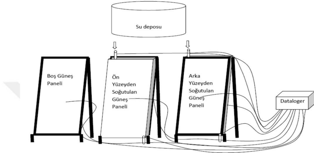
Şekil 3.11. Deney Düzenindeki Termokupl Bağlantıları
