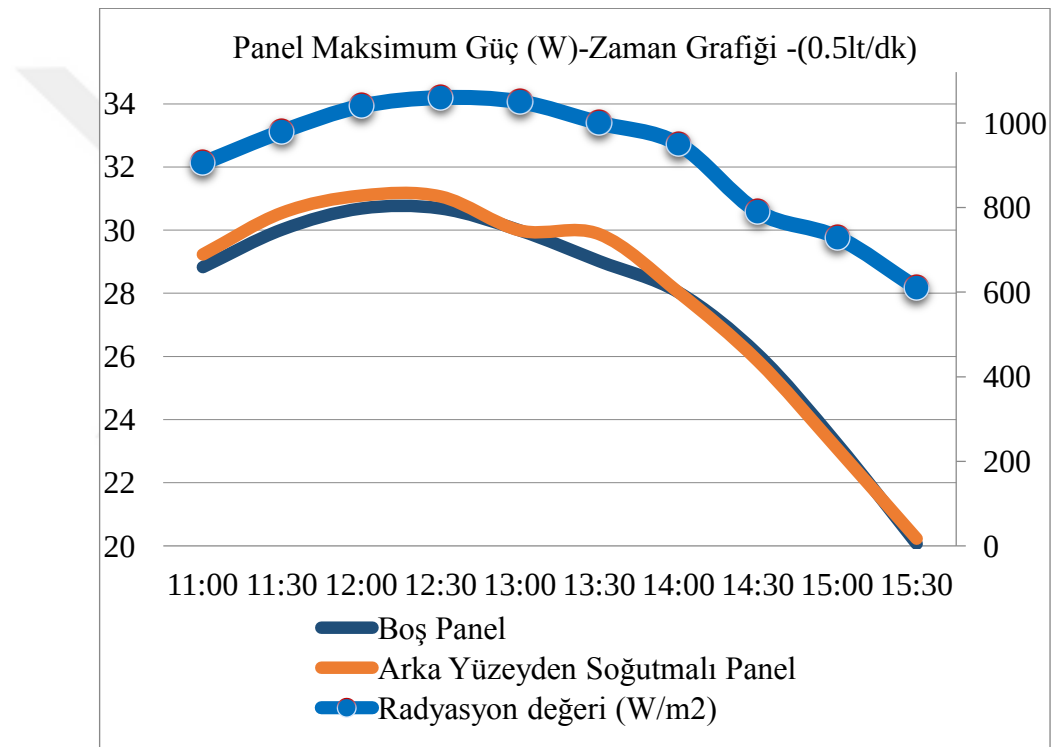
Şekil 4.6. Su Debisi 0.5 lt/dk iken Arka Yüzeyden Soğutulan Panel ile Boş Panelde Oluşan Güç Farkları
