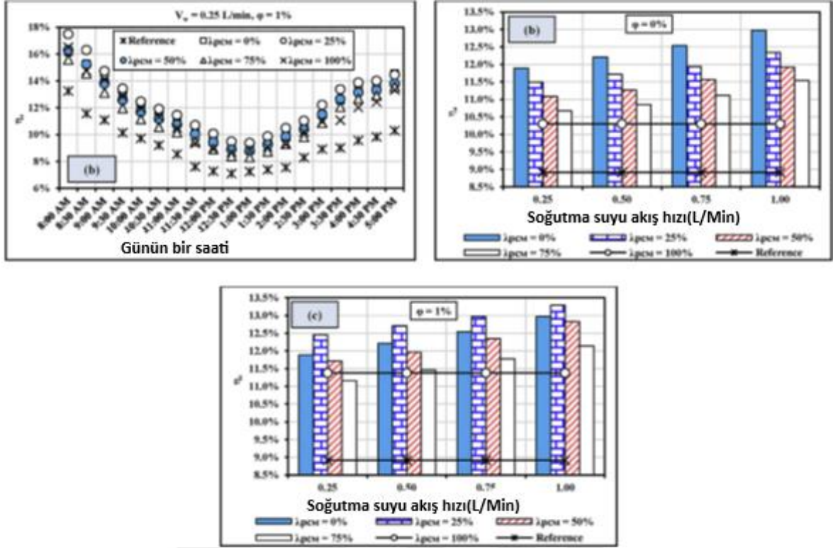
Şekil 2.7. Farklı FDM işgal oranlarında PV elektrik verimliliği; (a) V_w = 0.25 L/dk, \phi = 1\% 'de anlık değerler, (b) Ortalama değerler \phi = 0\% , (c) Ortalama değerler \phi = 1\% . (Salem ve ark., 2019)
