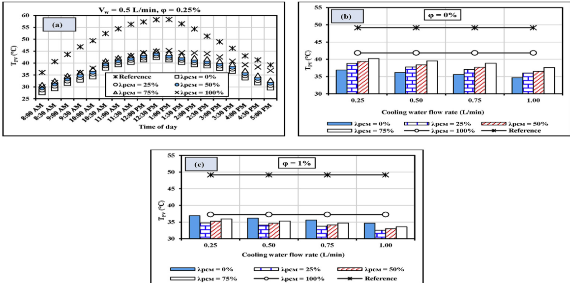
Şekil 2.5. Farklı FDM işgal oranlarında panel sıcaklığı; (a) Anlık sıcaklık, (b) Ortalama sıcaklık % 4 ¼, (c) Ortalama sıcaklık 4°C (Salem ve ark., 2019)
