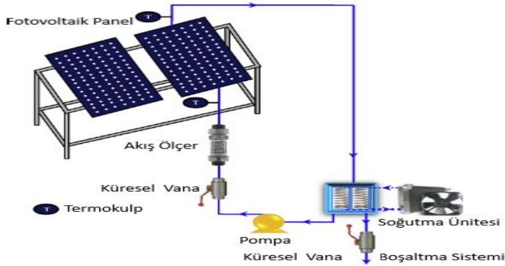
Şekil 2.1. Deneysel tesisin şematik gösterimi (Salem ve ark., 2019)
