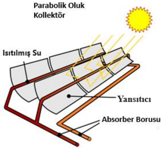
Şekil 1.26. Çizgi odaklı güneş kolektörünün çalışma prensibi (Arslan, 2015)
