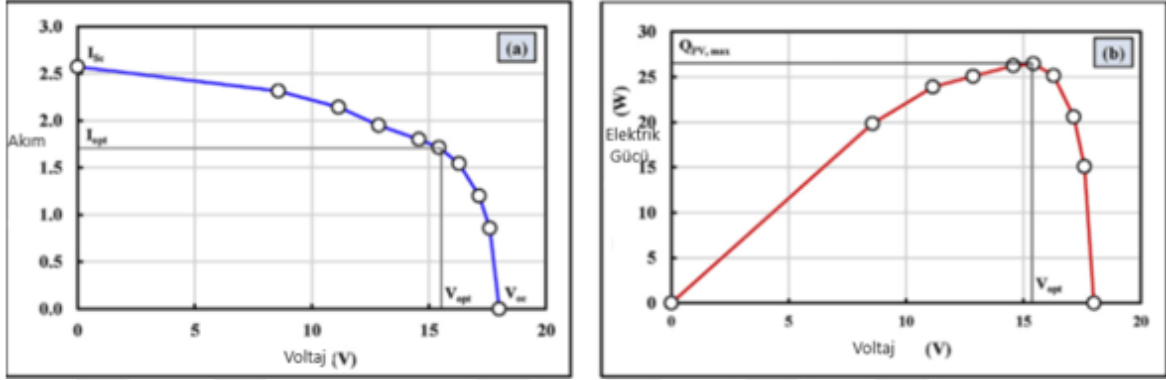
Şekil 2.4. Hücre için karakteristik eğriler; (a) I-V, (b) PPV-V (Salem ve ark., 2019)
