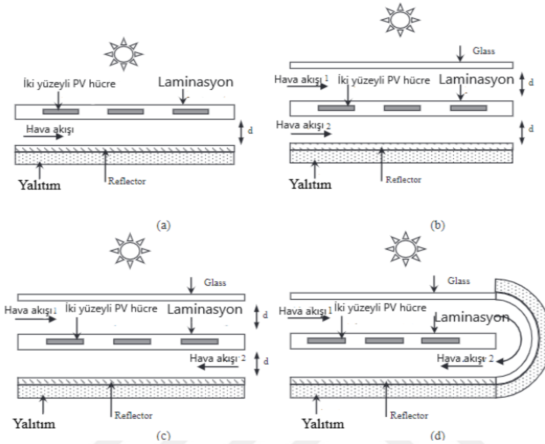
Şekil 2.22. Tek geçişli b) Paralel çift geçişli c) Çift geçişli karşı akışlı d) Çift geçişli geri dönüşlü (Ooshaksaraei ve ark., 2017)
