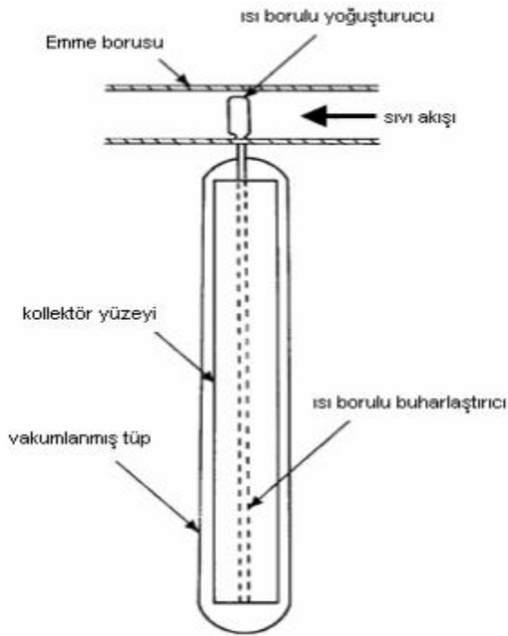
Şekil 1.25. Vakumlanmış güneş kolektörünün görünüşü (Şener, 2013)
