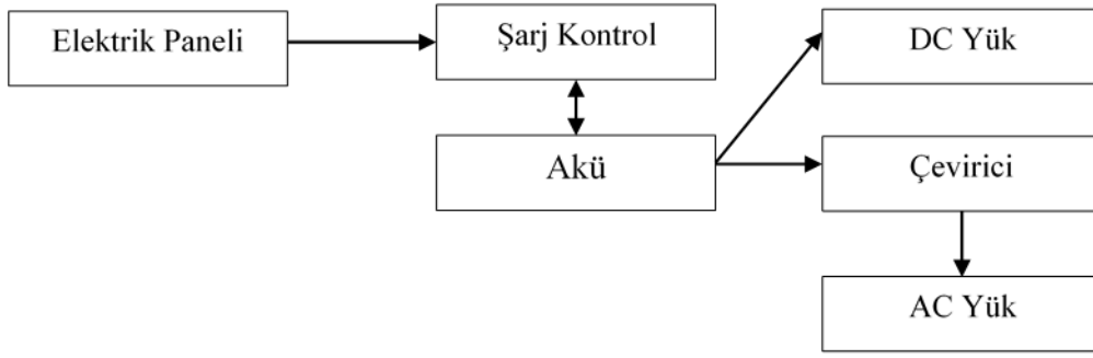
Şekil 1.15. PV sistem ekipman şeması (Kantaroğlu, 2010)
