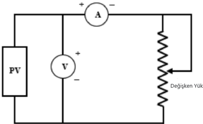
Şekil 2.3. Hücre özellikleri için ölçüm devresi (Salem ve ark., 2019)
