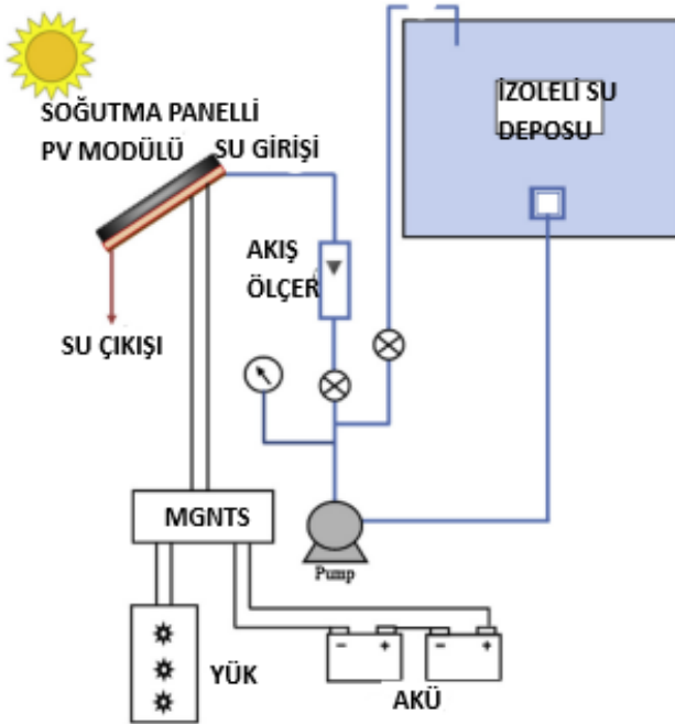
Şekil 2.21. Deney düzeneğinin şematik diyagramı (Bahaidarah ve ark., 2013)
