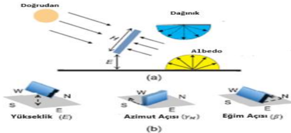
Şekil 2.26. (a) Doğrudan, dağınık ve soğurma ile iki yüzeyli bir güneş modülünün şeması yerden yansıyan albedo ışığı. Bu ışınım bileşenlerini hesaplamak için kullanılan denklemler burada etiketlenir. E ve H, nesnenin yüksekliğini (kağıtta 1m olarak ayarlanmıştır) belirtir. (b) İki yüzeyliyi optimize etmek için bu yazıda tartışılan üç parametre modülleri (Sun ve ark., 2018)
