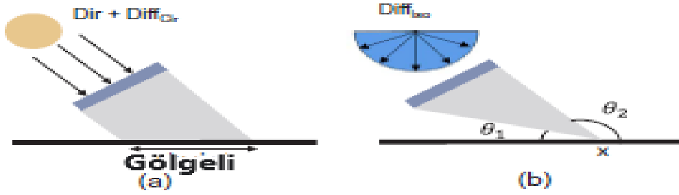
Şekil 2.27. Albedo ışığının (a) doğrudan (Dir) ve dairesel güneş ışığının kendi kendine gölgelenmesi ( Diff_{cir} ) ve (b) izotropik dağınık ışık (Diffiso) (Sun ve ark., 2018)
