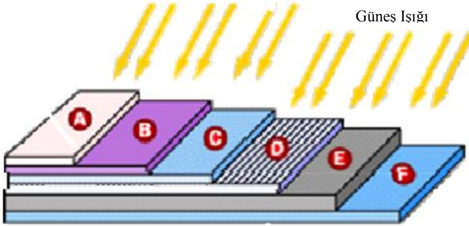
Şekil 1.20. Fotovoltaik hücrenin yapısı (URL-4, 2019)
