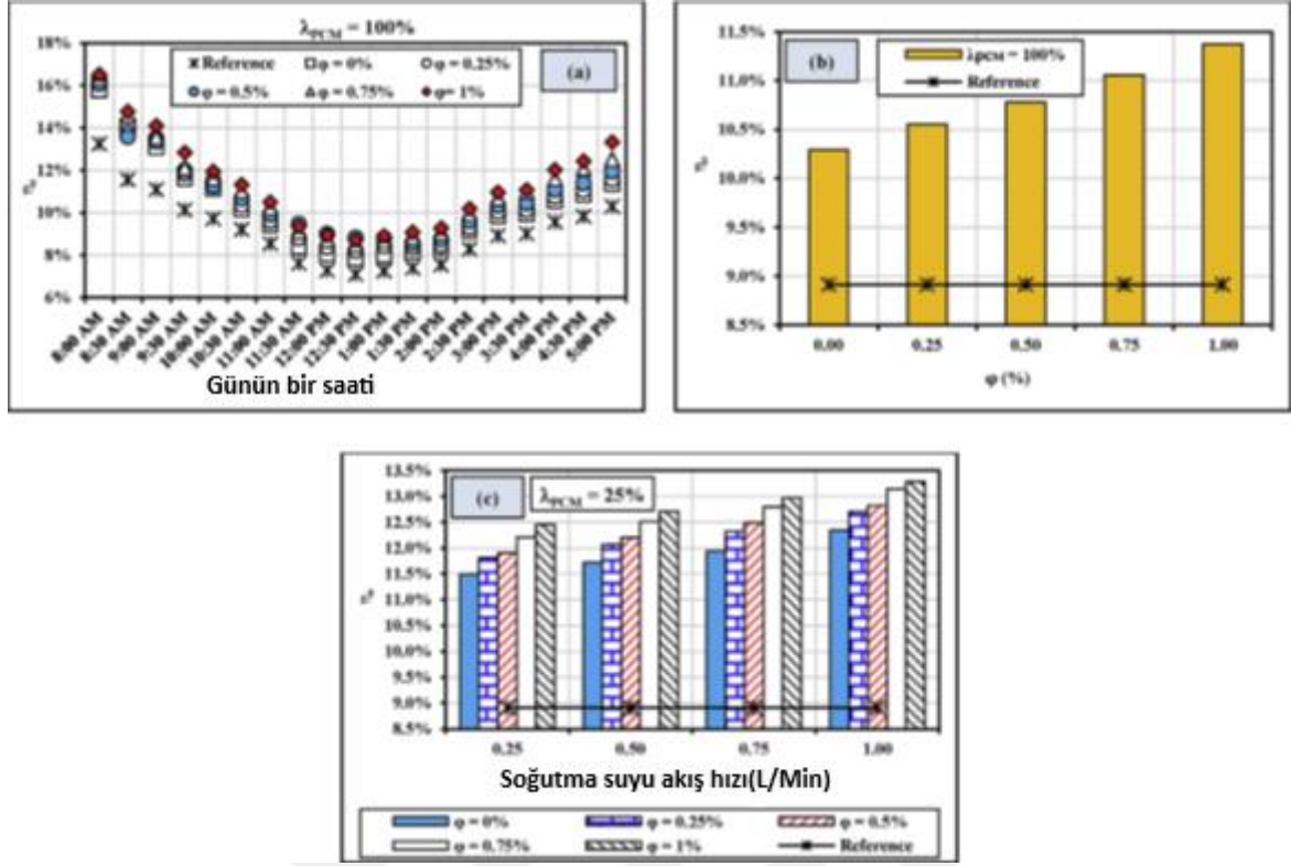
Şekil 2.8. Farklı nanoparçacık konsantrasyonlarında PV elektrik verimliliği; (a) Anlık değerler, (b) IFDM = %100'deki ortalama değerler, (c) IFDM = %25'teki ortalama değerler (Salem ve ark., 2019)
