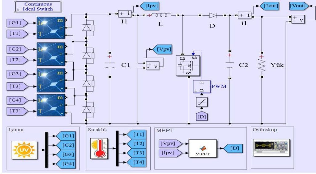
Şekil 2.34. Sistemin MATLAB/SIMULINK modeli (Gümüş ve Demirtaş, 2021)
