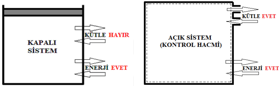
Şekil 1.5. Kapalı ve açık sistemin şematik görünümü (Ünal, 2009)
