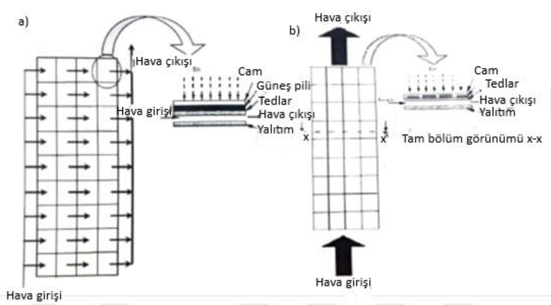
Şekil 2.24. a) Kare kanallı b) Düz kanallı kollektör (Agrawal ve Tiwari, 2013)
