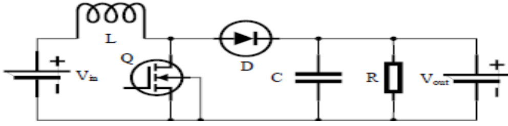
Şekil 2.30. DA-DA yükselten dönüştürücü devresi (Gümüş ve Demirtaş, 2021)
