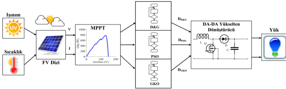
Şekil 2.29. Sistemin blok diyagramı (Gümüş ve Demirtaş, 2021)
