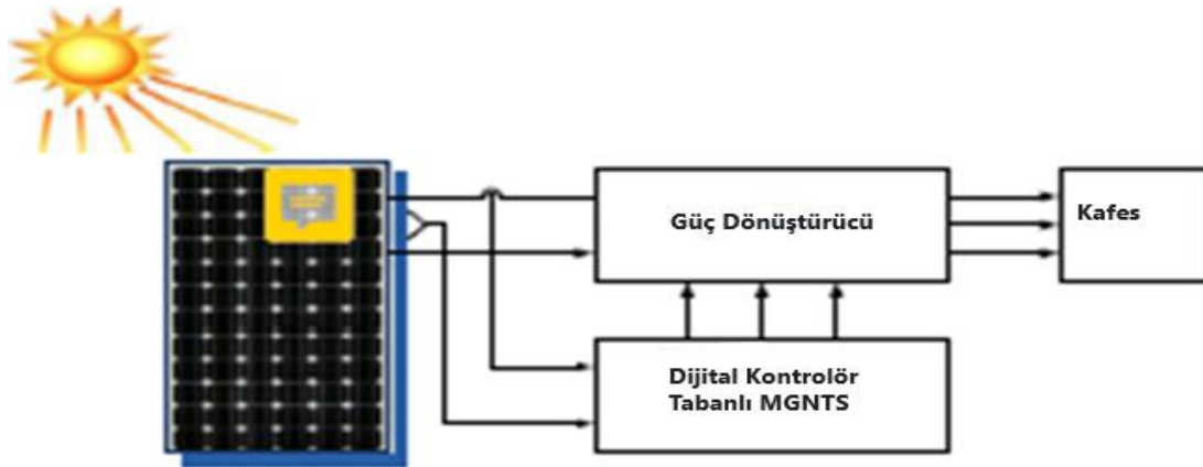
Şekil 2.35. Fotovoltaik sistem için MGNTS kontrolörünün blok şeması (Bhatnagar ve Nema 2013)
