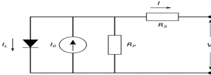
Şekil 1.18. Bir güneş pili için bir diyot modeli (Toprak ve ark., 2016)
