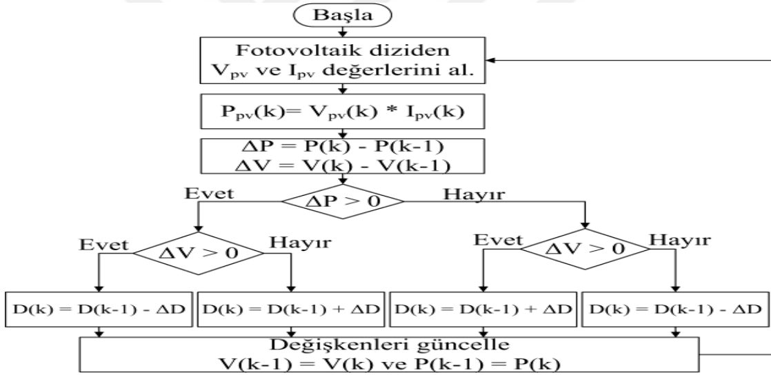
Şekil 2.31. D&G algoritmasının akış diyagramı (Gümüş ve Demirtaş, 2021)
