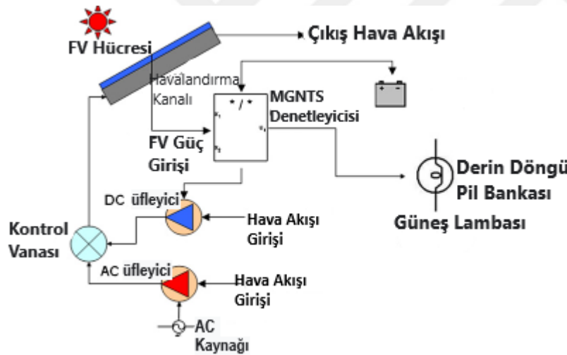
Şekil 2.18. Fotovoltaik modüller için aktif bir soğutma sistemi (Teo ve ark., 2012)
