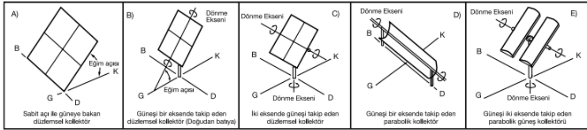
Şekil 1.22. Düzlemsel ve toplayıcı güneş kolektörlerinin konuşlandırılmaları (Değirmencioğlu ve İlken, 2003)
