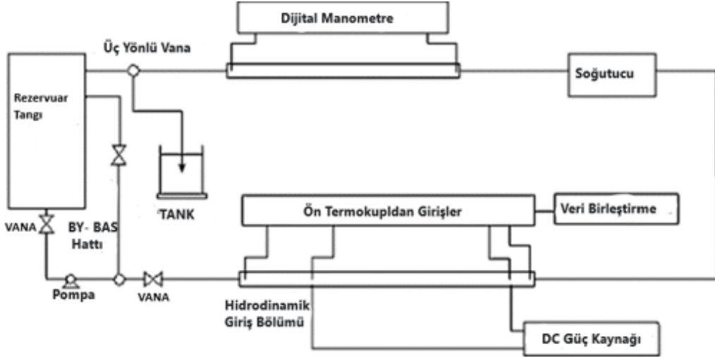
Şekil 2.19. Nanoakışkan için ısı transferi ve akış karakteristiklerinin deneysel sistemi (Li ve Xuan, 2002)
