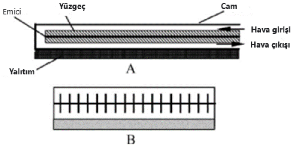
Şekil 2.28. Güneş enerjili hava ısıtıcısının şematik diyagramı (Naphon, 2005)
