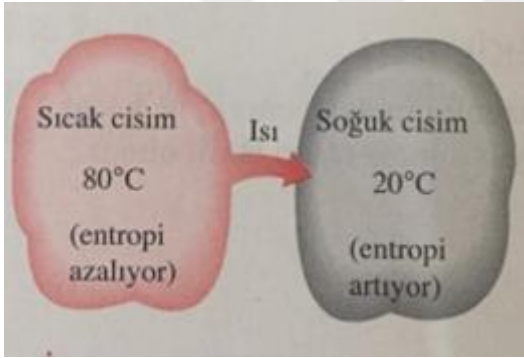
Şekil 1.8. Isı geçişi sırasında net entropi artışı (Çengel ve Boles, 2008)
