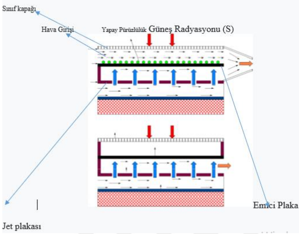
Şekil 2.23. (a) TGTKJPIGEHI solar hava ısıtıcısı, (b) TGTKJPIGEHI güneş hava ısıtıcısı, (c) Soğurucu plaka (d) Jet plakasının şematik kesit görünümü (Matheswaran ve ark., 2018)
