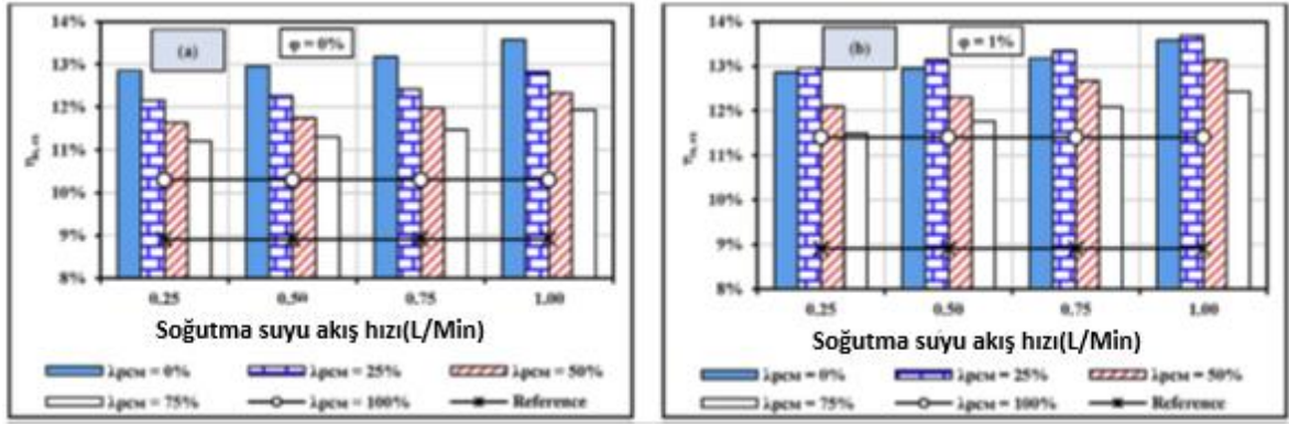
Şekil 2.11. Farklı FDM işgal oranlarında ortalama PV ekserji verimliliği; (a) %4 ¼ ve (b) 4 ¼ %1
