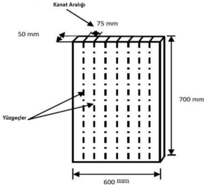
Şekil 2.14. Dikey olarak arkaya geri kanatçıklar takılı FDM konteynerlerinin şemaları (Hasan ve ark., 2014)
