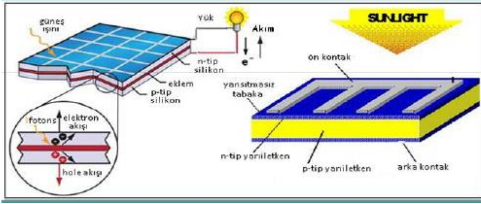
Şekil 1.14. Güneş pilinde fotovoltaik güç oluşumu (Cezim, 2013)
