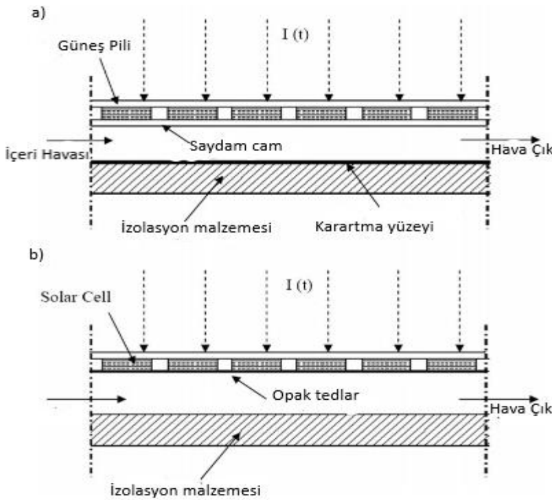
Şekil 2.25. Camdan a) Cama ve b) Mat yüzeye (Dubey ve ark., 2009)
