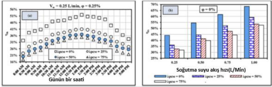
Şekil 2.9. Farklı Al_2O_3/FDM işgal oranlarında PV termal verimliliği; (a) Anlık değerler, (b) Ortalama değerler (Salem ve ark., 2019)
