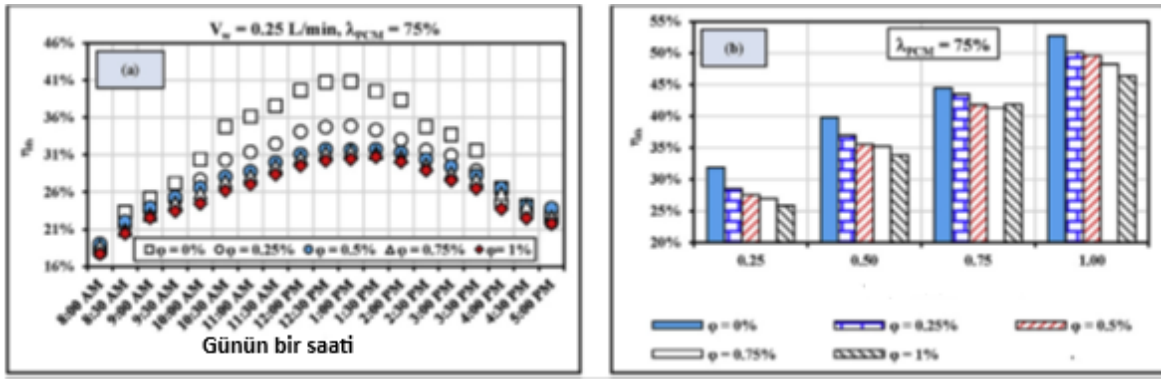
Şekil 2.10. Farklı Al_2O_3 nanoparçacık konsantrasyonlarında PV termal verimliliği; (a) Anlık değerler, (b) Ortalama değerler (Salem ve ark., 2019)
