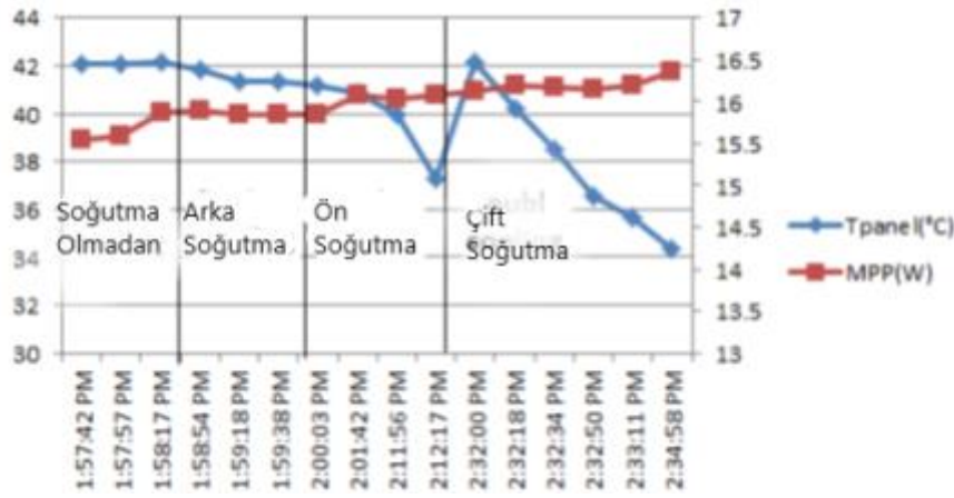
Şekil 2.17. Modül sıcaklığının deneysel test sırasında MGN'nin gelişimi (Hachicha ve ark., 2015)
