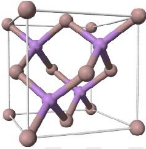
Şekil 1.21. Galyum Arsenit molekülün kristalik yapısı (Boz, 2011)
