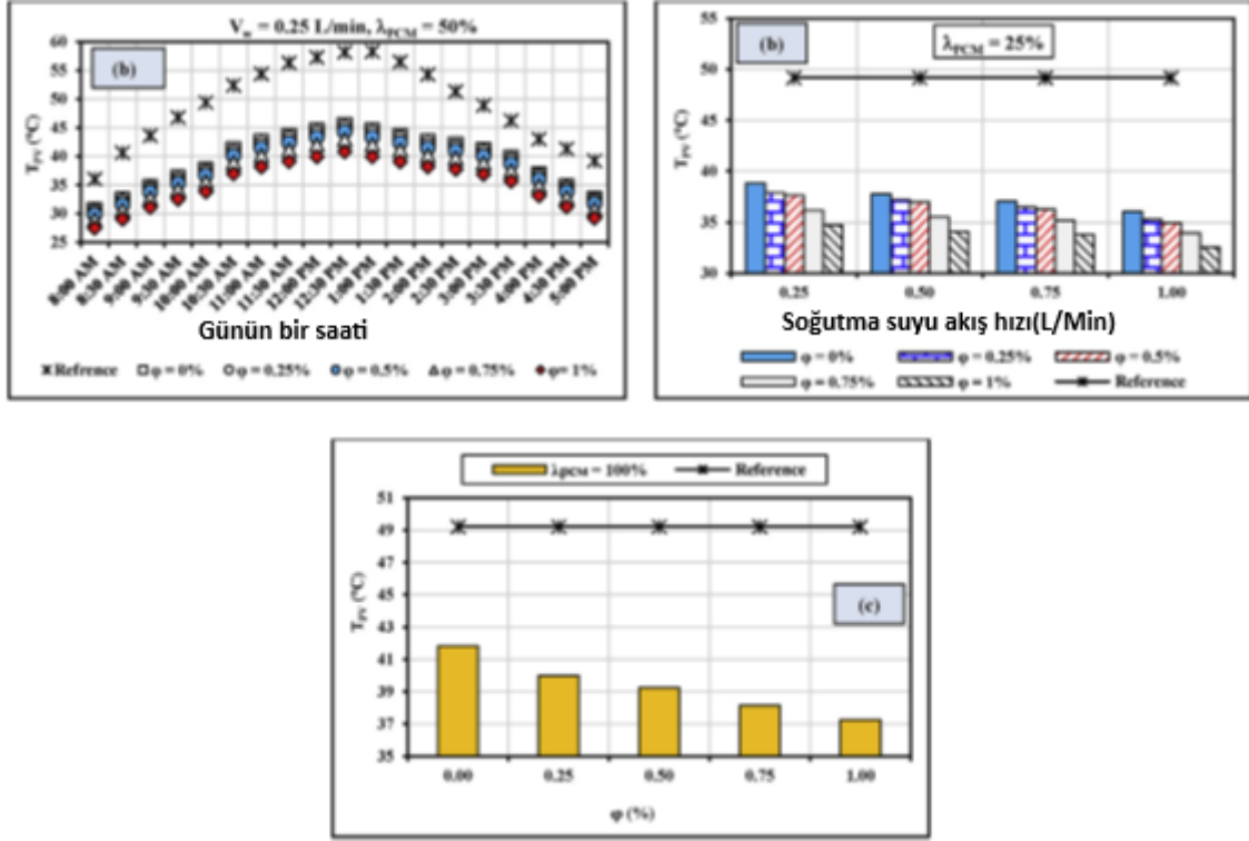
Şekil 2.6. Farklı nanopartikül konsantrasyonlarında panel sıcaklığı; (a) Anlık sıcaklık, (b) IFDM'de ortalama sıcaklık \frac{1}{4} %25, (c) IFDM'de ortalama sıcaklık \frac{1}{4} %100 (Salem ve ark., 2019)
