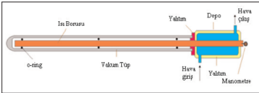
Şekil 1.24. Isı borulu vakum tüplü hava ısıtma güneş kolektörünün kesit görünüşü (Ersöz ve Yıldız, 2013)
