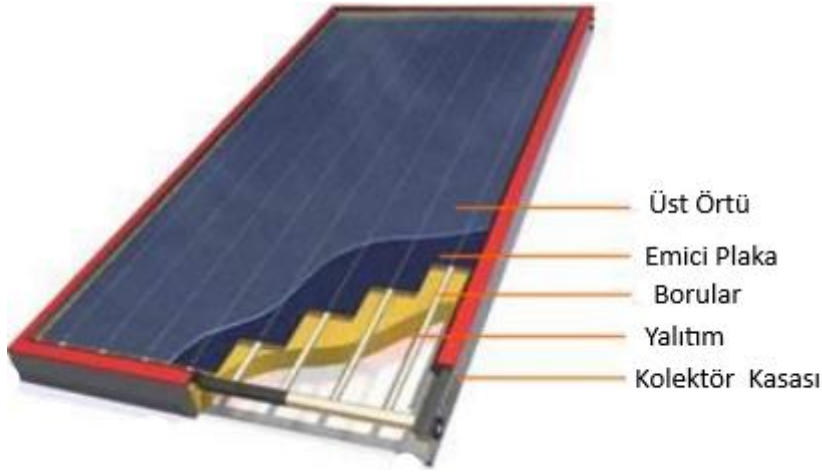
Şekil 1.23. Düz plakalı kolektörün görünüşü (Şener, 2013)
