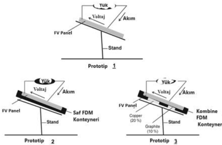
Şekil 2.15. Deneyde kullanılacak yöntemlere ait 3 prototip tip (Hachem ve ark., 2017)
