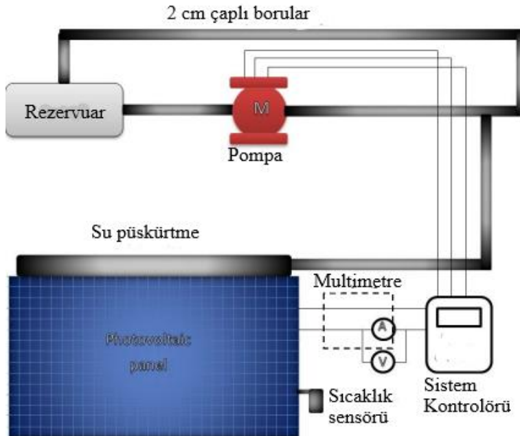
Şekil 2.16. Tam otomatik bir sistem için şematik diyagram (Dorobantu ve Popescu, 2013)
