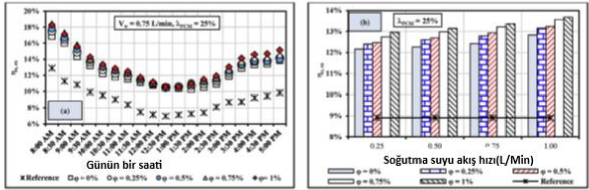
Şekil 2.12. Farklı nanoparçacık konsantrasyonlarında PV ekserji verimliliği; (a) Anlık değerler, (b) Ortalama değerler (Salem ve ark., 2019)
