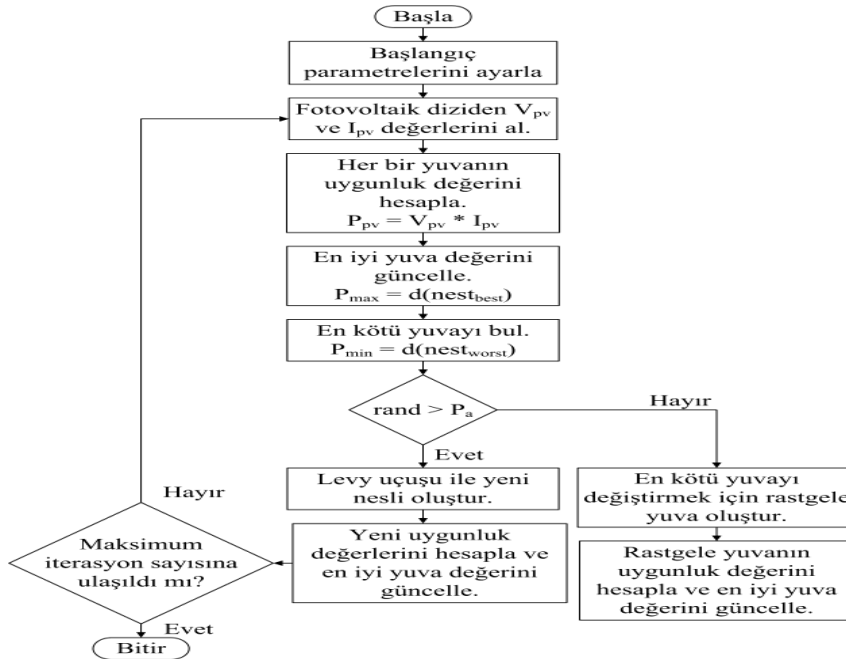
Şekil 2.33. GKO algoritmasının MGNTS’de işleminde kullanım diyagramı (Gümüş ve Demirtaş, 2021)
