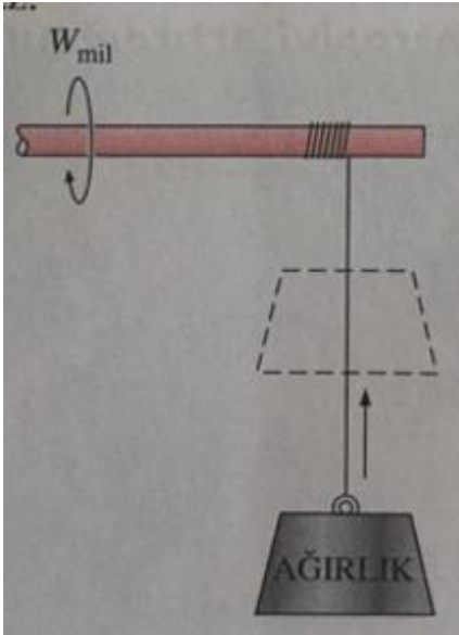
Şekil 1.10. Sürtünme oluşmaması durumu (Çengel ve Boles, 2008)
