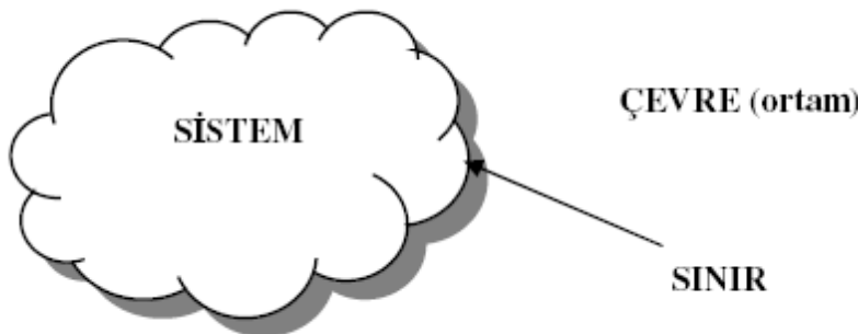
Şekil 1.4. Apak (2007)'ye göre sistem sınır ve çevre (Ünal, 2009)
