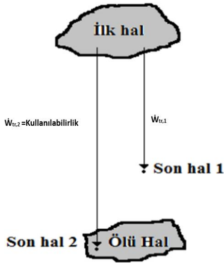
Şekil 1.11. Tersinir iş ve kullanılabilirlik arasındaki ilişki (Ünal, 2009)
