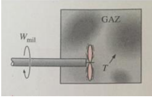
Şekil 1.7. Gaz üzerinde yapılan döner milin gazın düzensizliğini (entropisini) arttırması (Çengel ve Boles, 2008)
