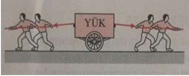
Şekil 1.9. Sürtünme durumunda entropinin varlığı (Çengel ve Boles, 2008)
