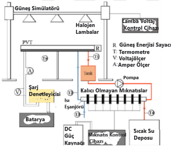
Şekil 2.20. Deney düzeneğinin diyagramı (Ghadiri ve ark., 2015)
