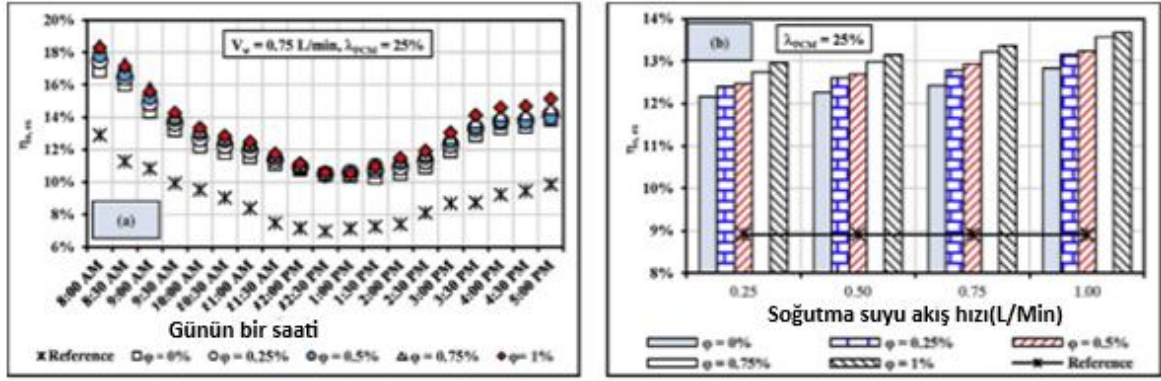
Şekil 2.13. Farklı nanoparçacık konsantrasyonlarında PV ekserji verimliliği; (a) Anlık değerler, (b) Ortalama değerler (Salem ve ark., 2019)
