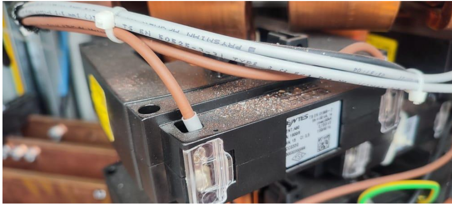
Şekil 4.26. Bakır kablo parçacıklarının neden olduğu kısa devre
