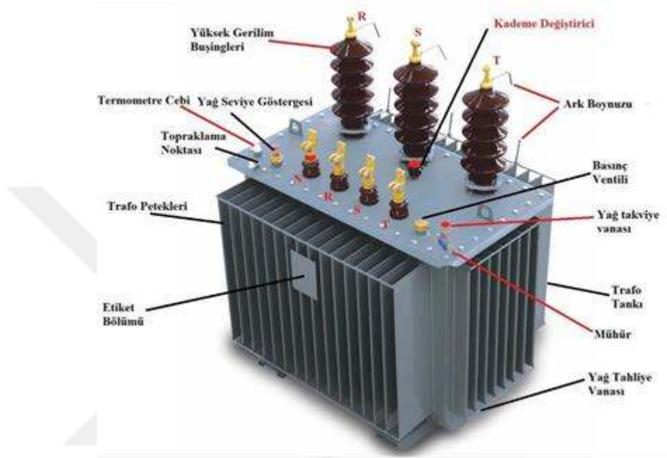
Şekil 2.16. 0,4-34kV trafo (URL-17, 2022)
