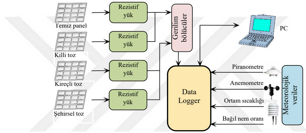
Şekil 6.1. Veri setinin elde edilmesine ait genel blok diyagramı
