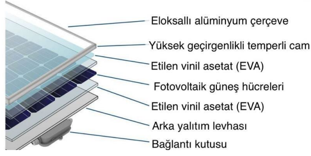
Şekil 3.2. Fotovoltaik panelin fiziksel yapısı [95]
