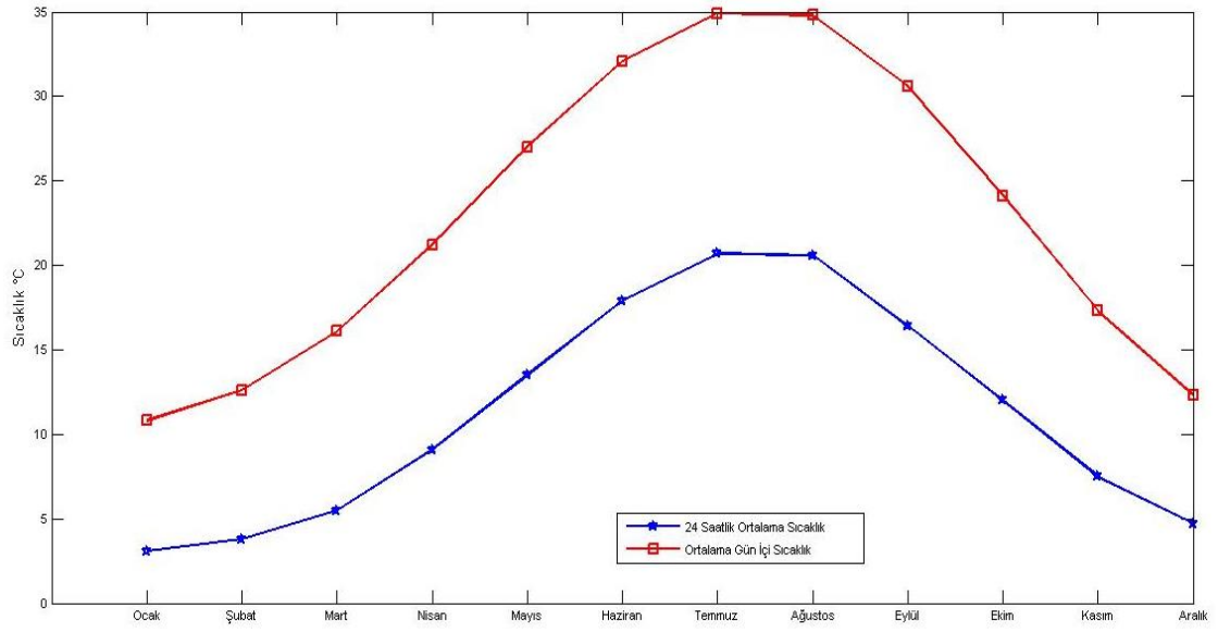
Şekil 1.5. Manisa/Turgutlu Sıcaklık Dağılım Grafiği
