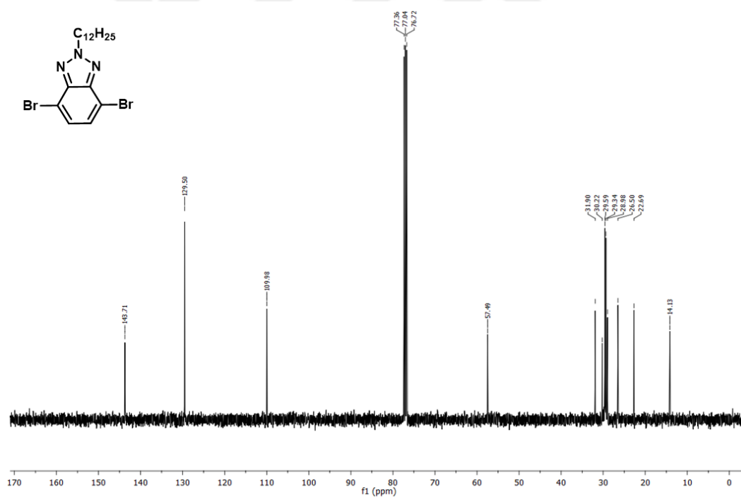
Figure A.10. 13 C NMR of 4,7-dibromo-2-dodecyl-2H-benzo[d][1,2,3]triazole
