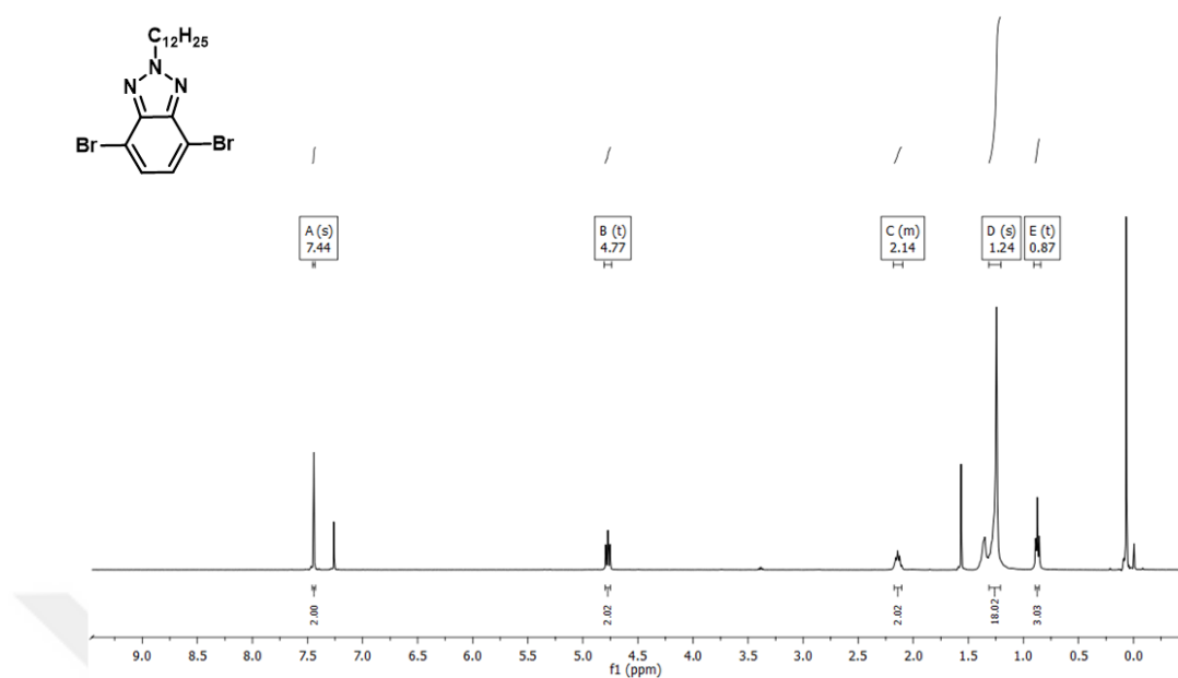
Figure A.9. 1 H NMR of 4,7-dibromo-2-dodecyl-2H-benzo[d][1,2,3]triazole
