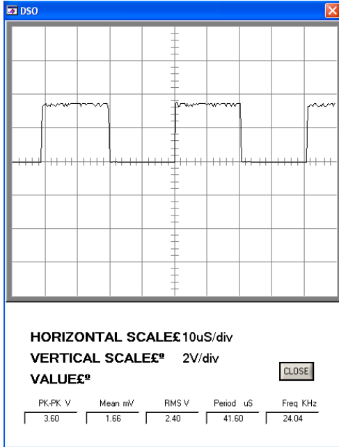
Şekil 7.9. R_L=50\Omega , D=0.5 (a) PWM sinyali, (b) V_o çıkış gerilimi
