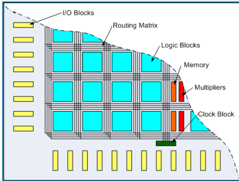
Şekil 2.10. FPGA Mimarisi [15]
