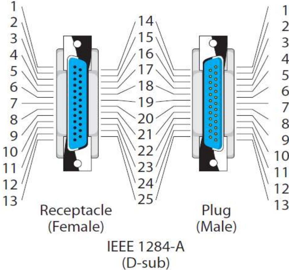
Şekil 6.2. IEEE 1284-A Paralel Port Şekli [27]
