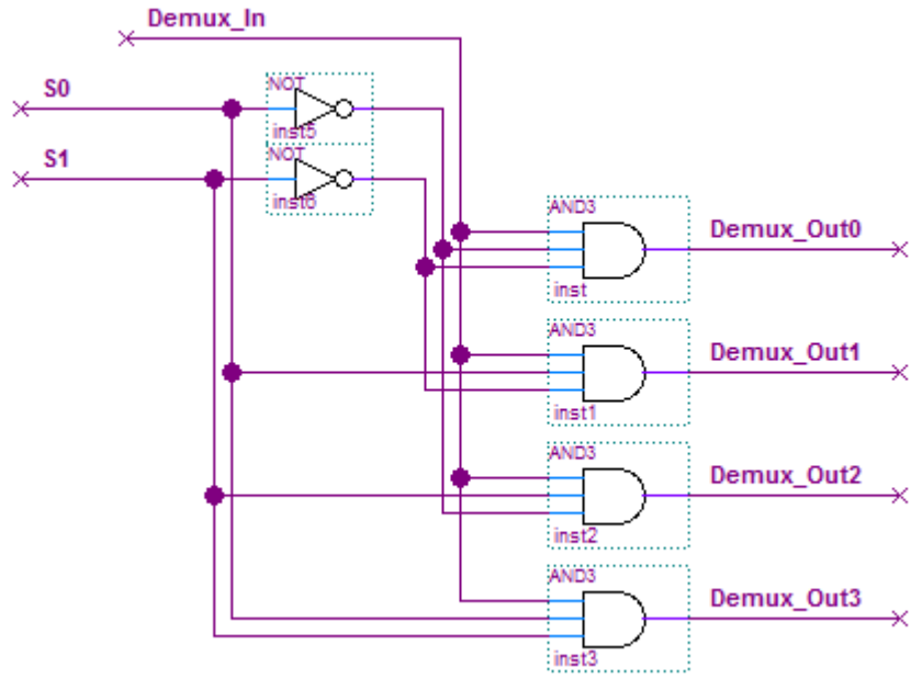
Şekil 7.4. 1x4 DeMultiplexer
