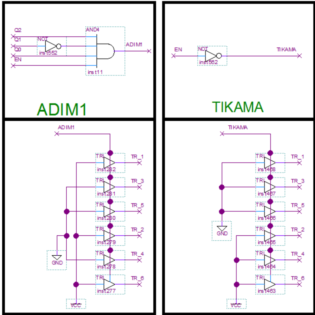
Şekil 7.17. Komütasyon Devresi
