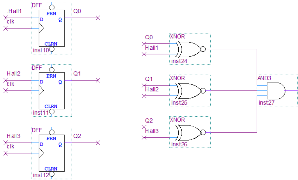
Şekil 7.12. Sensör Okuma Devresi
