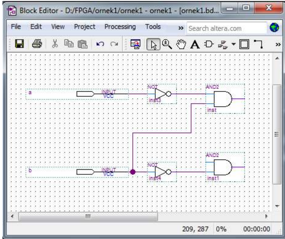
Şekil 3.14. Devrenin Genişletilmiş Görünümü
