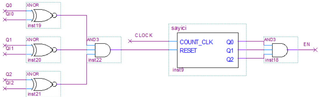
Şekil 7.13. Ölü zaman Üreticisi ve Karşılaştırıcı
