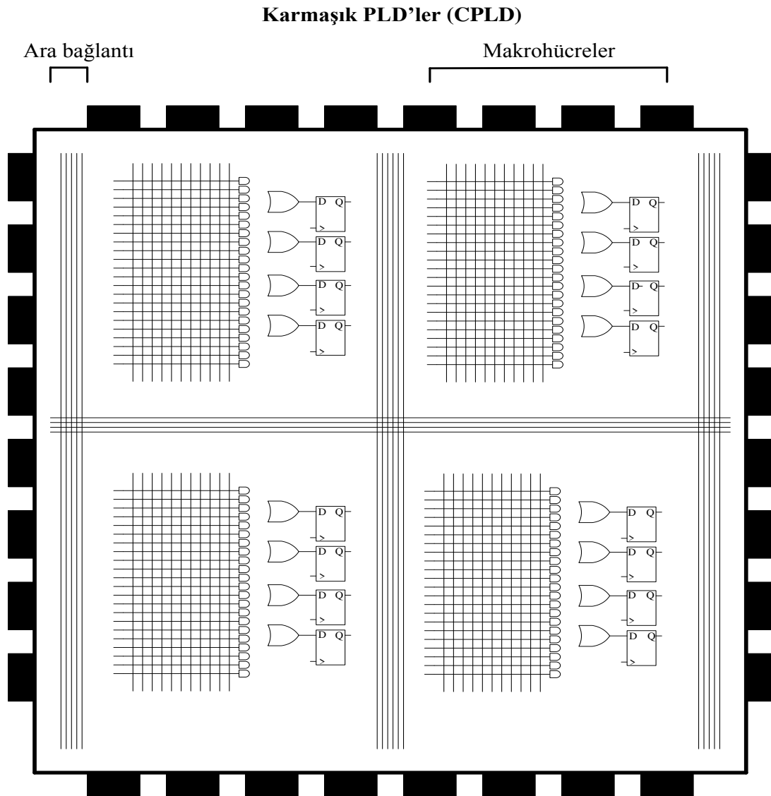
Şekil 2.4. CPLD Yapısı
