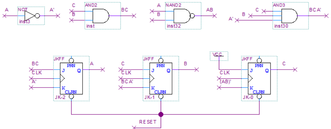
Şekil 7.16. Tamamlanmış Sayıcı Devre
