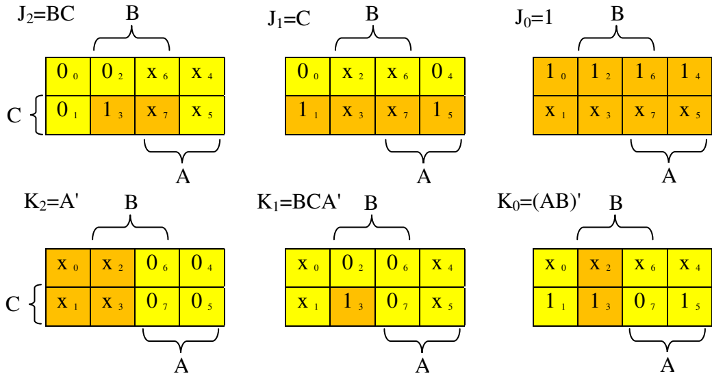
Şekil 7.15. Karnaugh Haritası
