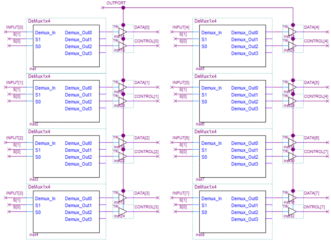
Şekil 7.6. 8x1x4 DeMultiplexer
