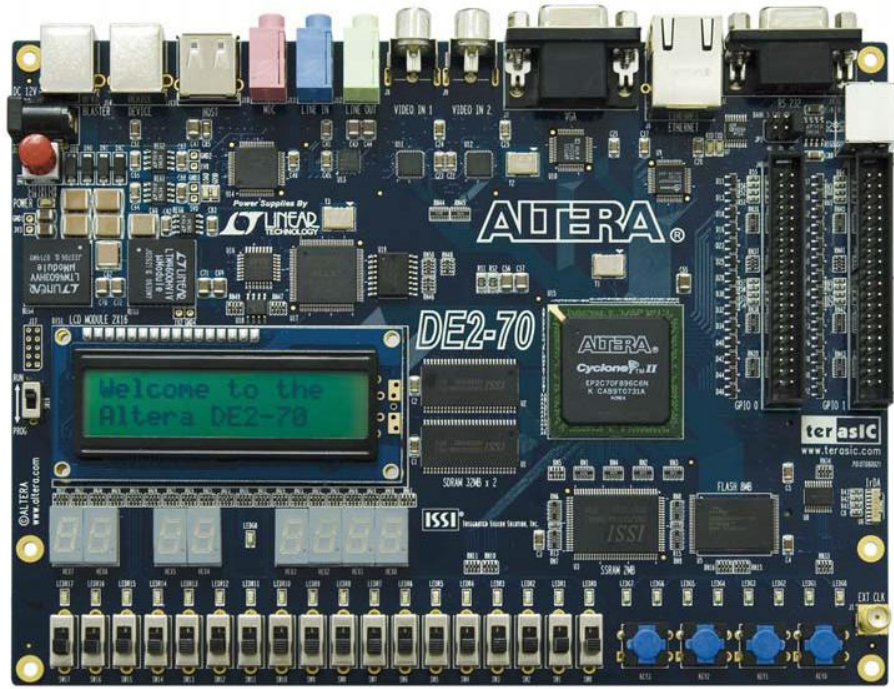
Şekil 2.15. Altera DE2-70 Board [16]
