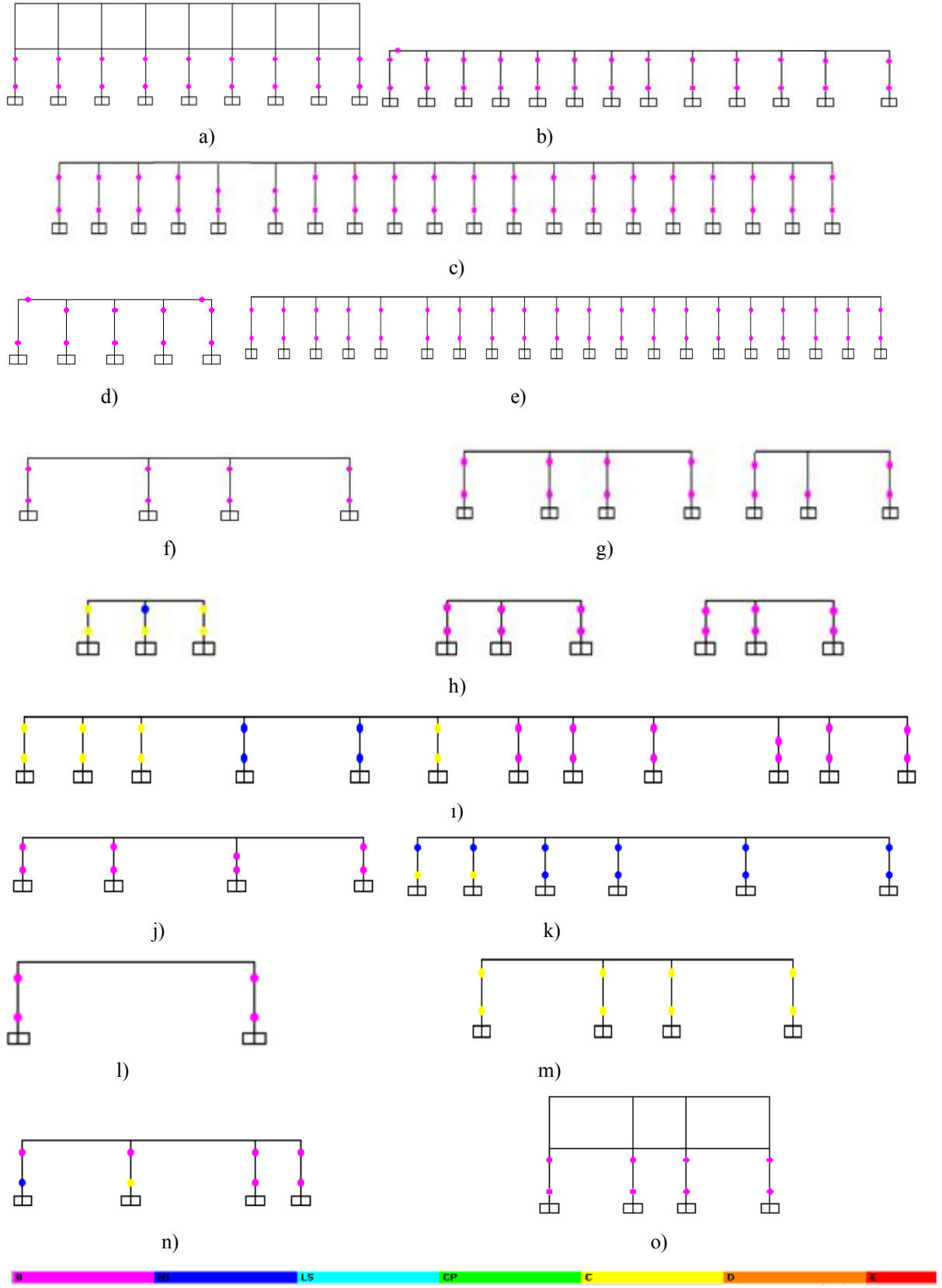
Şekil 5.5 Depremin x yönünde etkimesi için a) M, b) N, c) O, d) P, e) R, f) 1, g) 8, h) 11, ı) 12, j) 13, k) 14 , l) 15, m) 18, n) 19 ve o) 24 aksları hasar durumları
