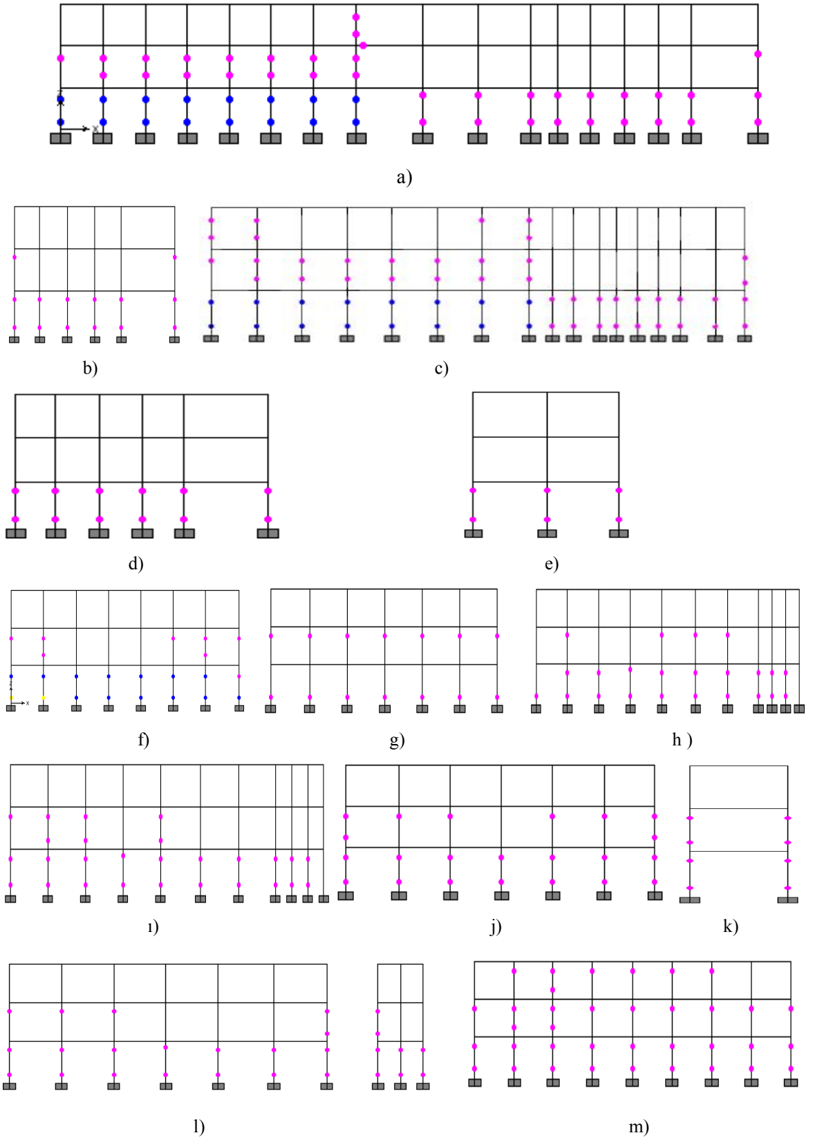
Şekil 5.34 Depremin y yönünde etkimesi için, a) E, b) F, c) G, d) H, e) I, f) K, g) O, h) P, i) R, j) S, k) T, l) U, m) Y aksları hasar durumları
