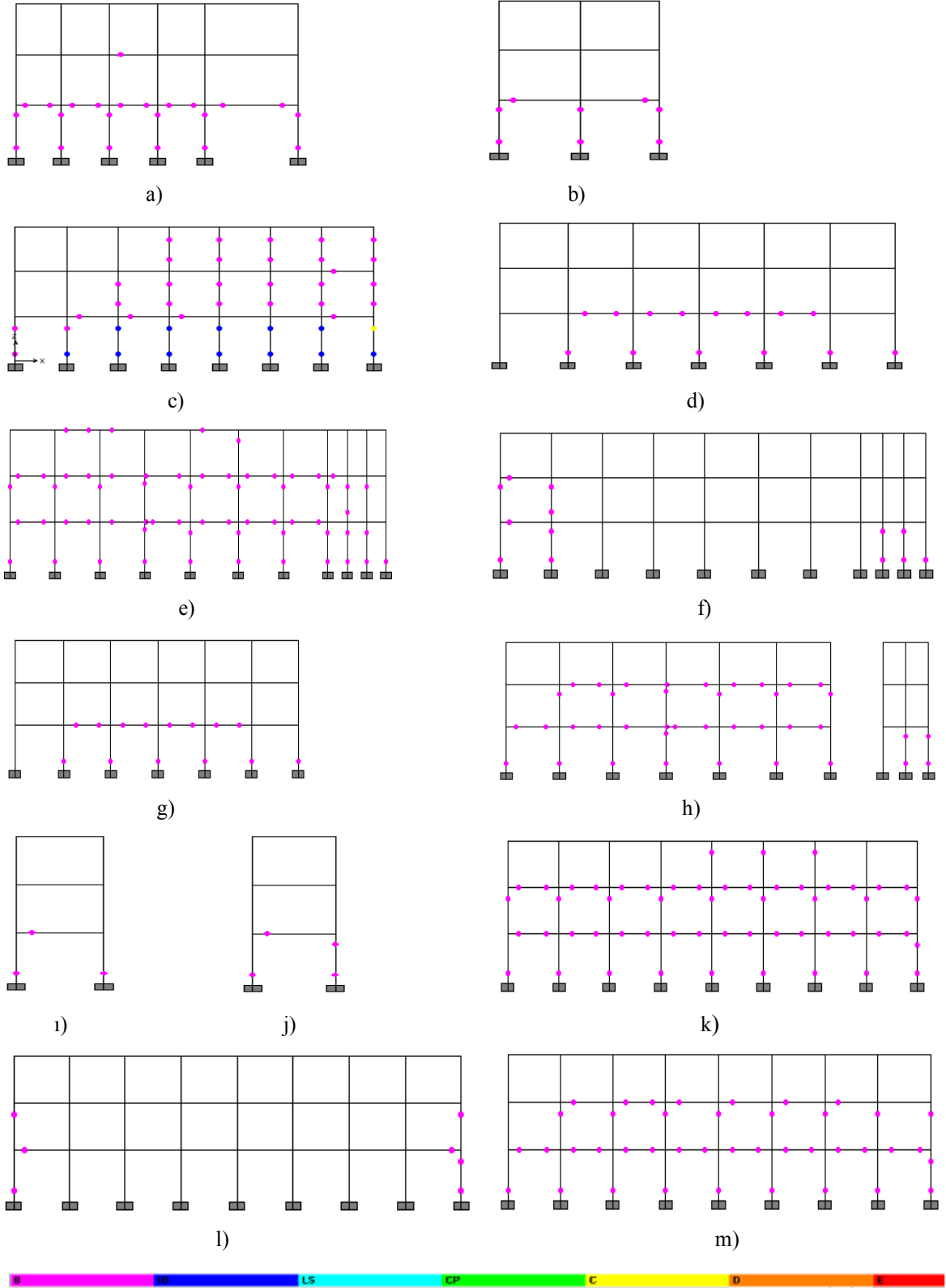
Şekil 5.30 Depremin x yönünde etkimesi için, a) H, b) I, c) K, d) O, e) P, f) R, g) S, h) T, ı) U, j) V, k) Y, l) Z ve m) Q aksları hasar durumları
