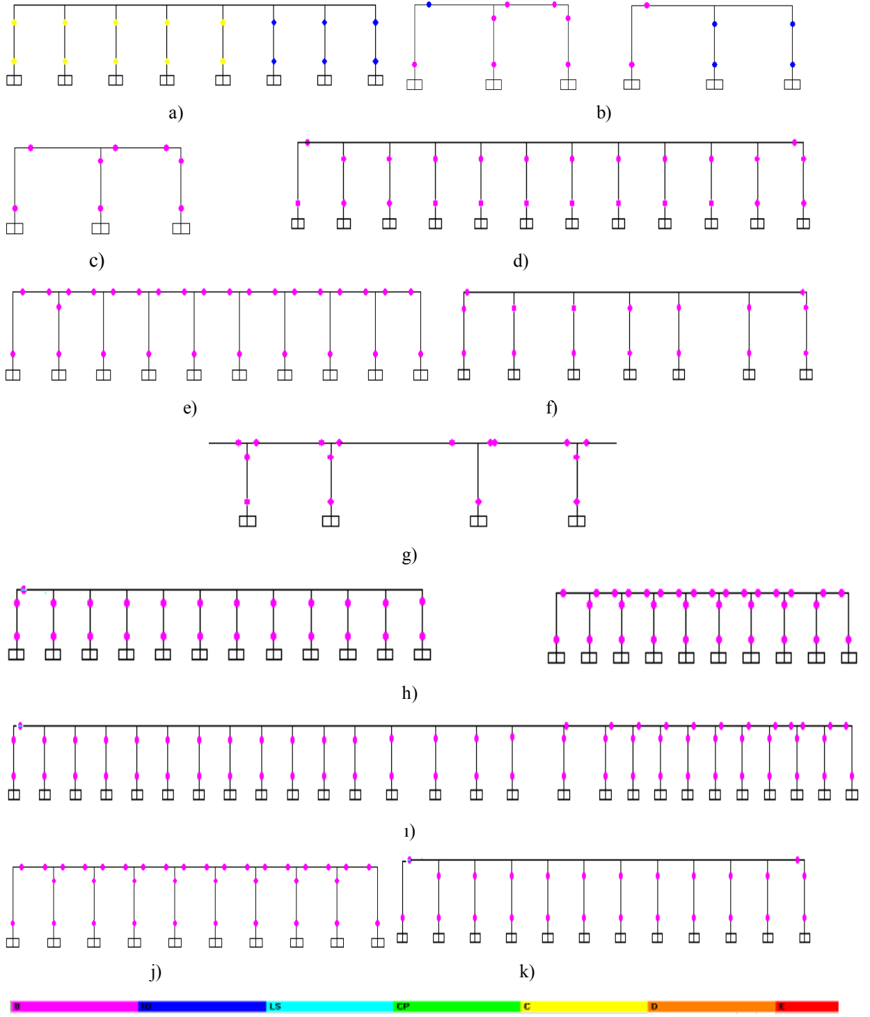
Şekil 5.14 Depremi x yönünde etkimesi için a) K, b) M, c) N, d) R, e) U, f) V, g) Y, h) Z, i) Q, j) W ve k) X aksları hasar durumları
