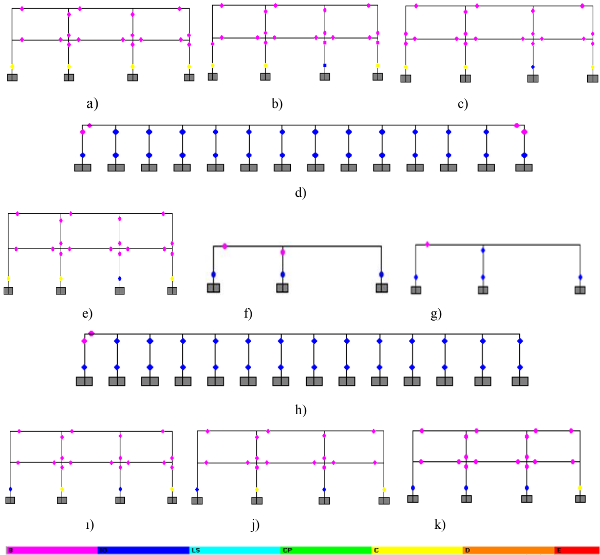
Şekil 5.41 Deprem'in x yönünde etkimesi için a) A, b) B, c) C, d) D, e) E, f) G, g) J, h) K, i) M, j) R, k) Y, aksları hasar durumları
