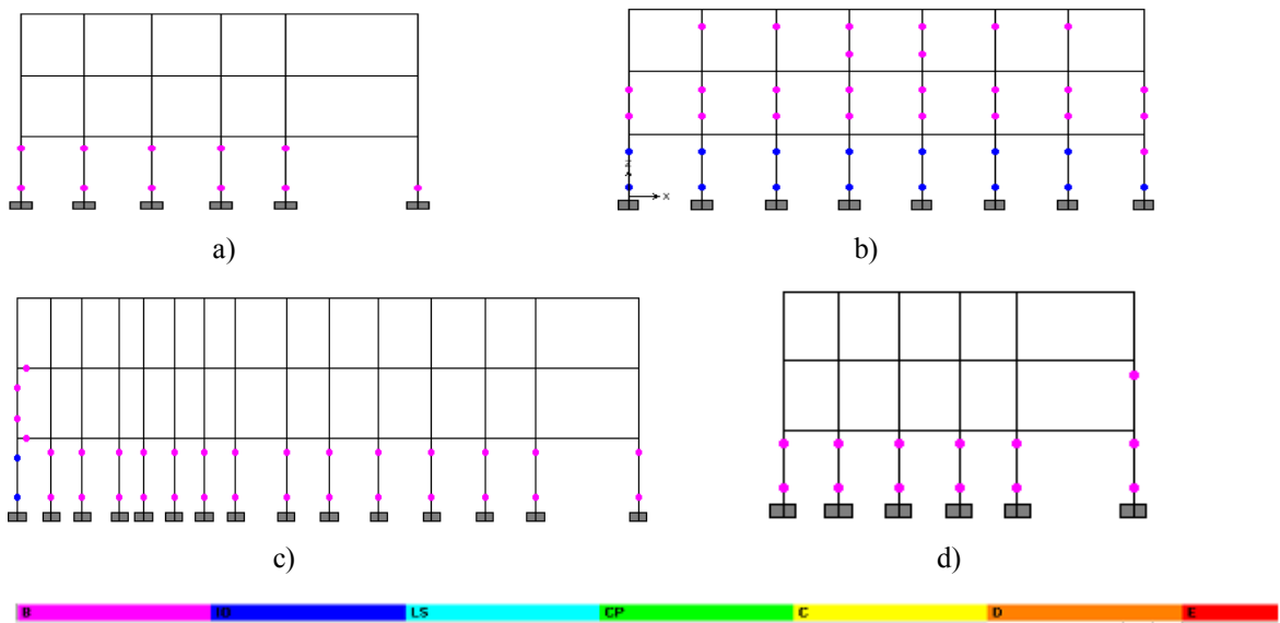
Şekil 5.33 Deprem y yönünde etkimesi için a) A, b) B, c) C ve d) D aksları hasar durumları
