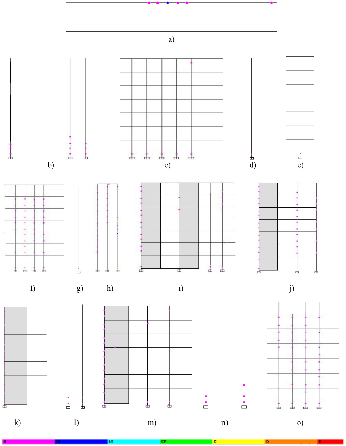
Şekil 5.53 Depremin y yönünde etkimesi için a) A, b) B, c) C, d) D, e) E, f) F, g) G, h) H, ı) J, j) K k) L, l) M, m) N, n) O ve o) P ağısları hasar durumları
