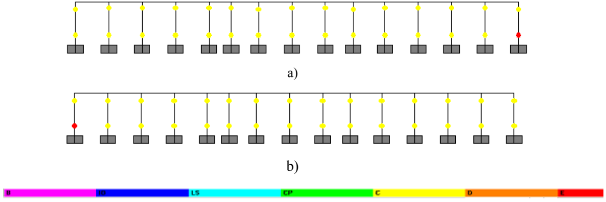
Şekil 5.47 Deprem y yönünde etkimesi için, a) 37, b) 38 aksları hasar durumları
