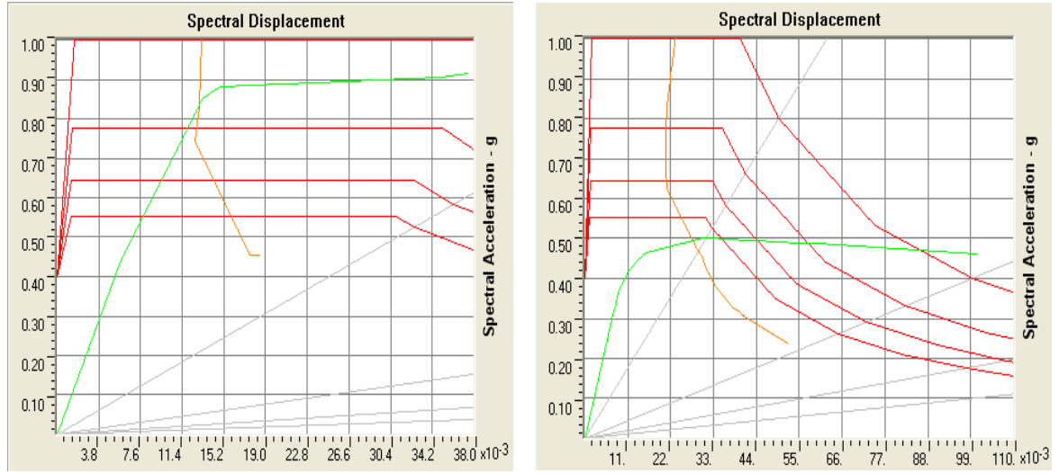
Şekil 5.48 Deprem x ve y yönlerinde etkimesi halinde ATC-40' a göre kapasite spektrum grafikleri
