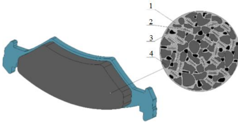
Şekil 2.3. Fren balatası yapısında kullanılan malzemeler: 1. bağlayıcı, 2. takviye, 3. dolgu, 4. sürtünme ayarlayıcı (Borawski, 2020)
