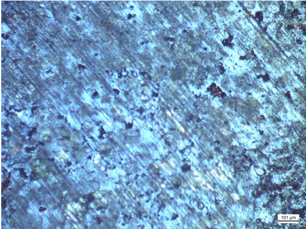
Şekil 3.13. %1,25 boraks dekahidrat kullanılan numunenin mikroyapısı
