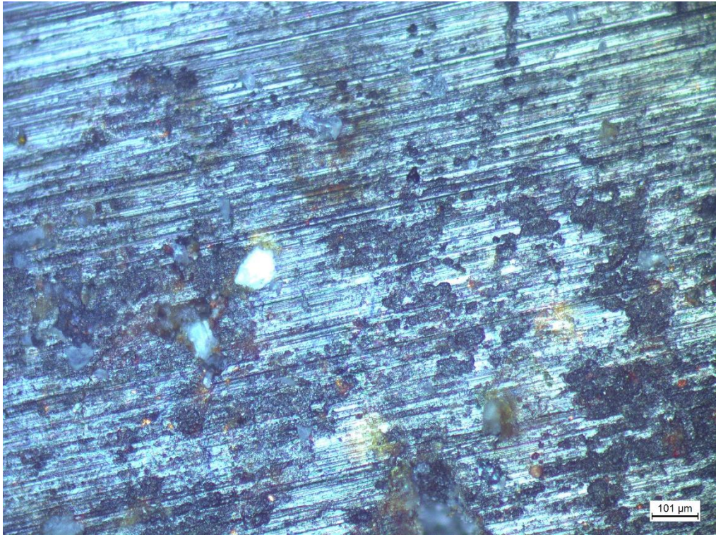
Şekil 3.15. %5 boraks dekahidrat kullanılan numunenin mikroyapısı
