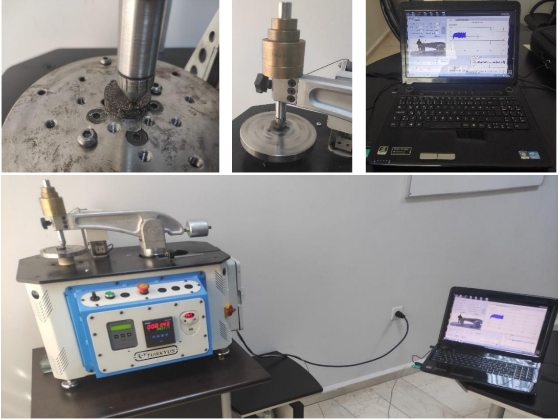
Şekil 3.5. Aşınma deney düzeneği
