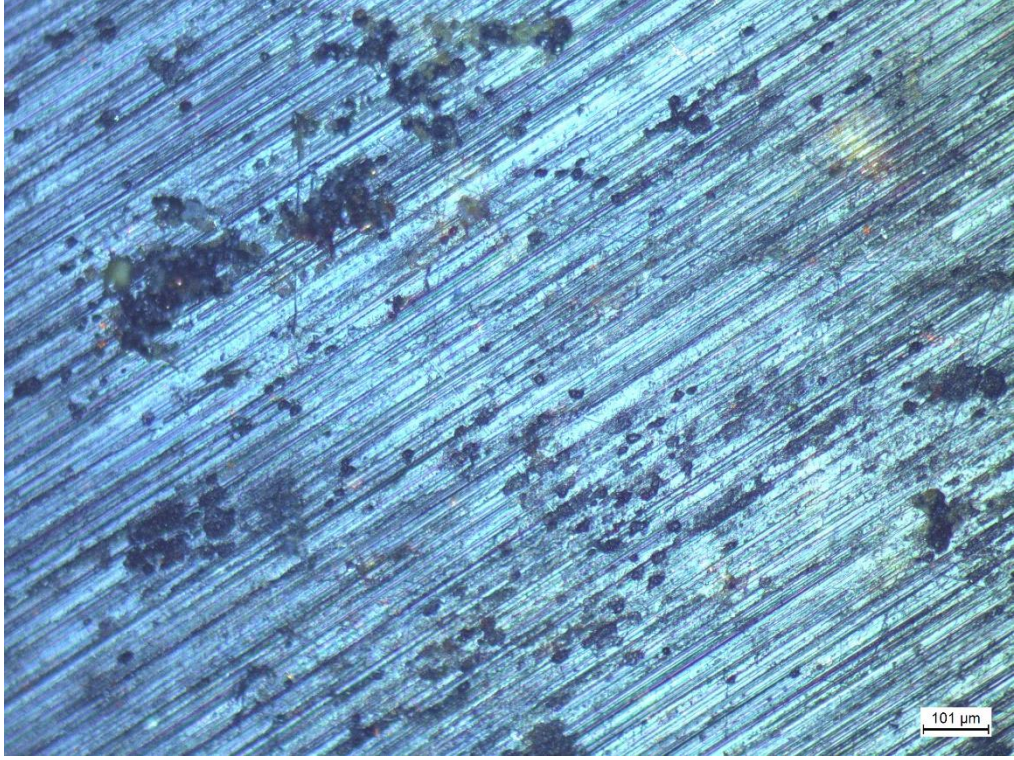
Şekil 3.14. %2,5 boraks dekahidrat kullanılan numunenin mikroyapısı
