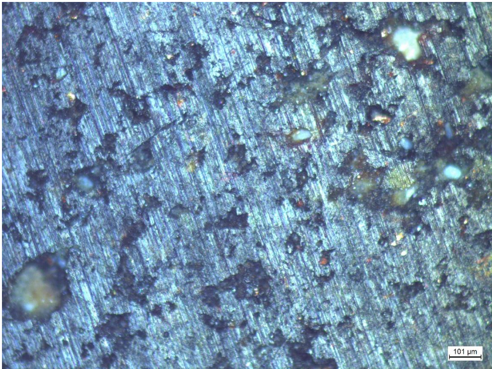
Şekil 3.9. %2,5 borik asit kullanılan numunenin mikroyapısı
