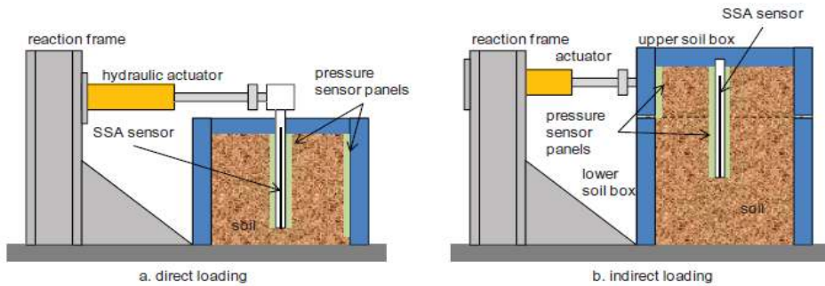
Şekil 2.1. Direkt ve Endirekt Yükleme
