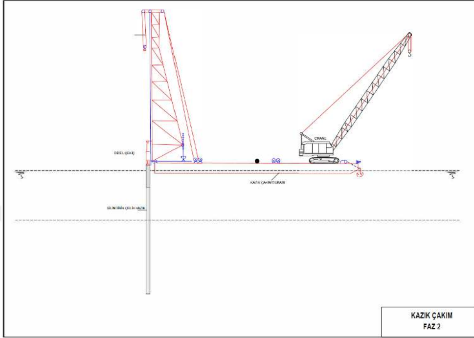
Şekil 3.13. Kazık Çakılması Faz-2
