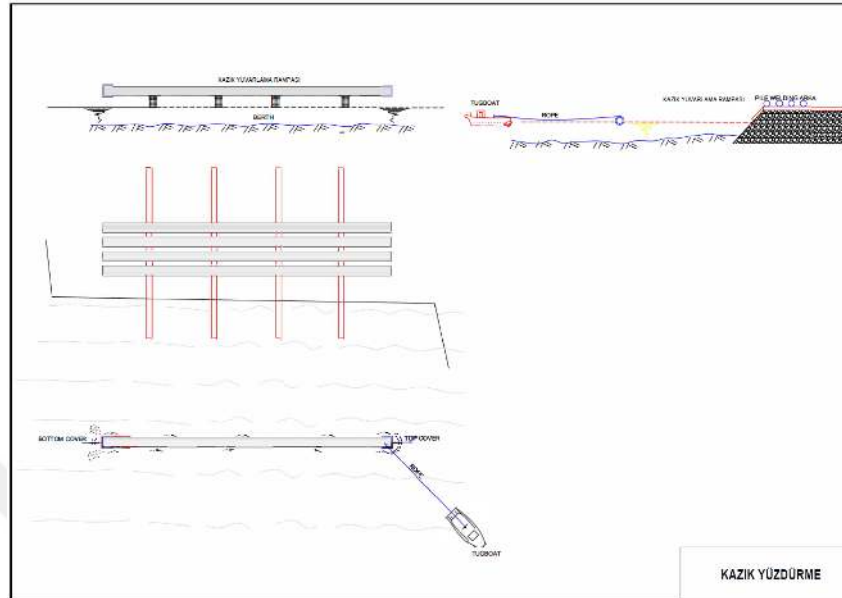
Şekil 3.9. Kazığın Yüzdürülmesi
