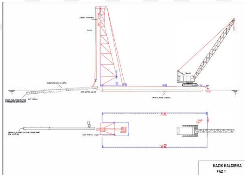
Şekil 3.10. Kazıgın Kaldırılması Faz-1
