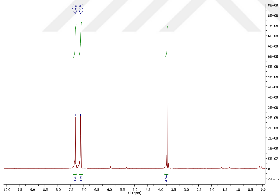
Figure A. 12 ^1\text{H} NMR spectrum of 29.
