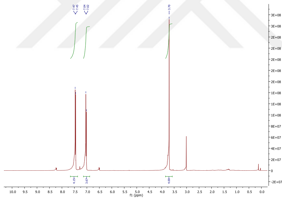
Figure A. ^1\text{H} NMR spectrum of 30.
