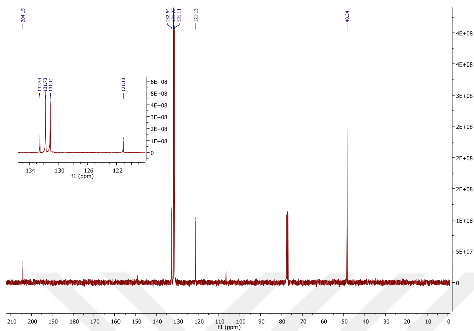
Figure A. 15 ^{13}\text{C} NMR spectrum of 30.
