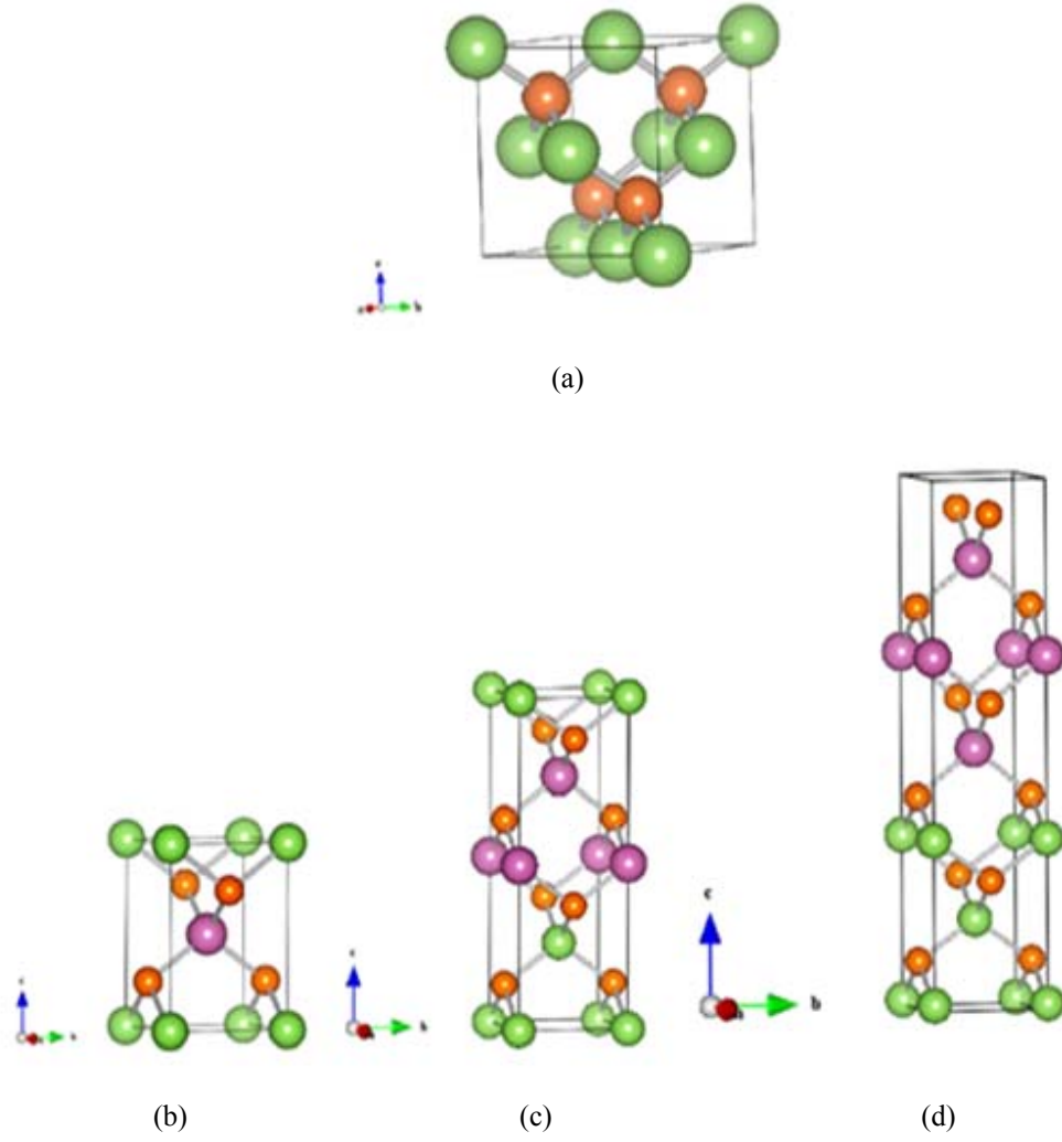
Şekil 4.1. a) GaAs(InAs), b) (\text{GaAs})_1/(\text{InAs})_1 , c) (\text{GaAs})_2/(\text{InAs})_2 , d) (\text{GaAs})_3/(\text{InAs})_3 yapıları. Yeşil atomlar As, mor atomlar In ve turuncu atomlar As
