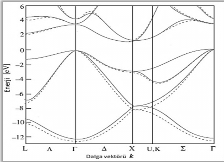
Şekil 3.2. Si ‘un pseudopotansiyel yöntemi kullanılarak hesaplanan bant yapısı grafiği.
