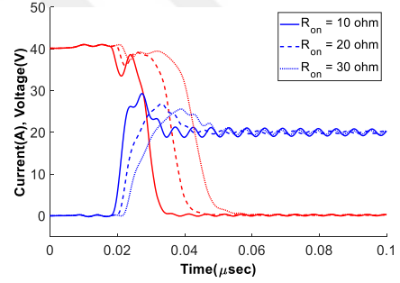
(d) Bottom switch turn-on[8]
