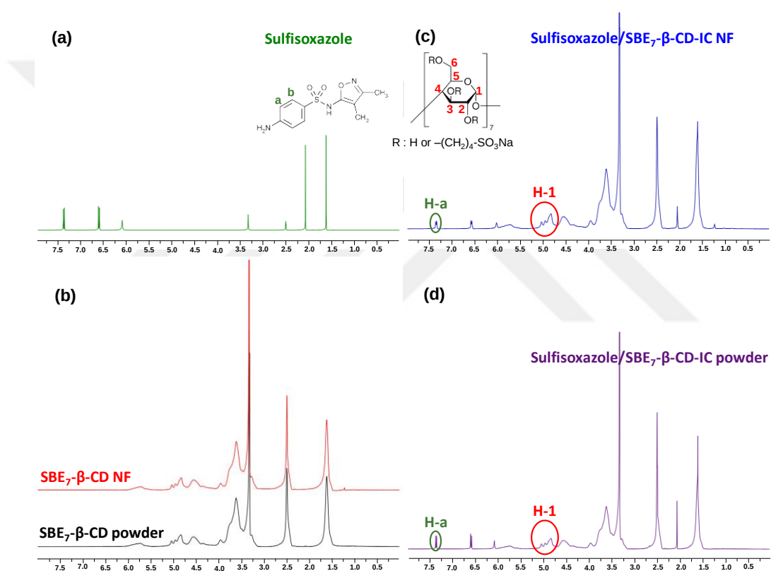
Figure 48. 1 H NMR spectra of (a) sulfisoxazole powder, (b) SBE 7 -β-CD NF and SBE 7 -β-CD powder, (c) sulfisoxazole/SBE 7 -β-CD-IC NF, (d) sulfisoxazole/SBE 7 -β-CD-IC powder.
