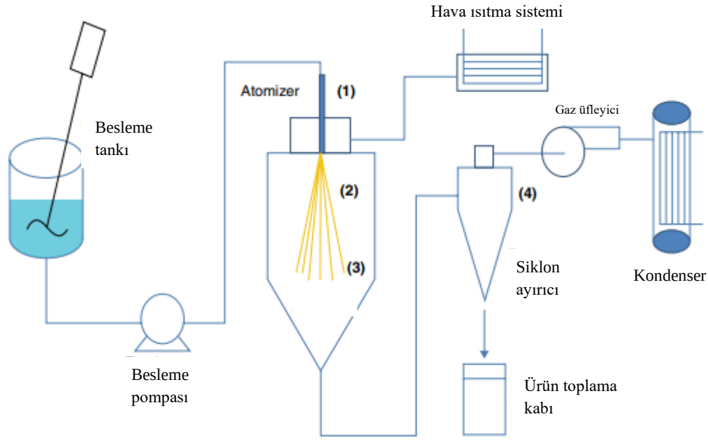
Şekil 2.4. Püskürterek kurutma aşamaları (Anandharamakrishnan 2015)
