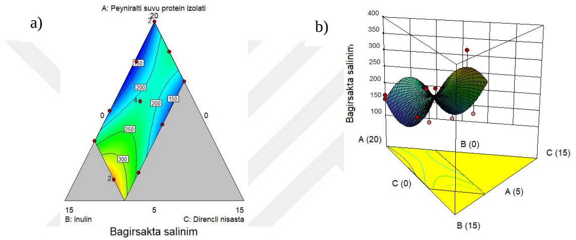
Şekil 4.5. PSP/IN/DN kombinasyonuna ait optimizasyon grafikleri a) Kontur grafiği ve b) 3 boyutlu yüzey grafiği
