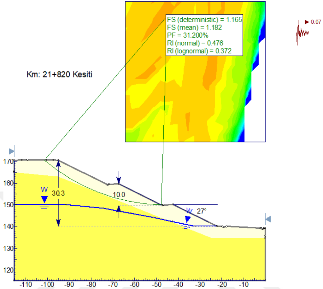
Şekil 9-19 27° basamak geometrisiyle oluşturulan km:21+820 şev profilinde kh=0.07 durumundaki olasılıklı duraylılık analizi
