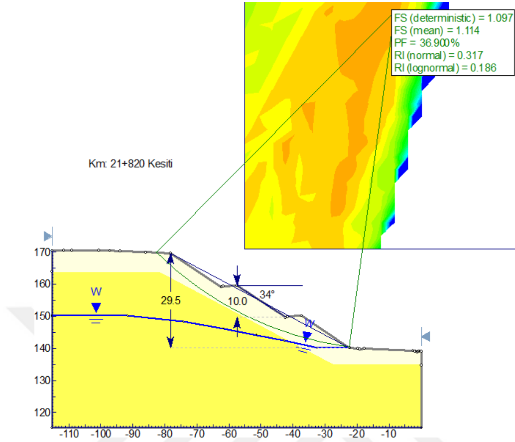
Şekil 9-9 Km:21+820 şev profilinde 34° basamak geometrisinin statik durum olasılıklı duraylılık analizi
