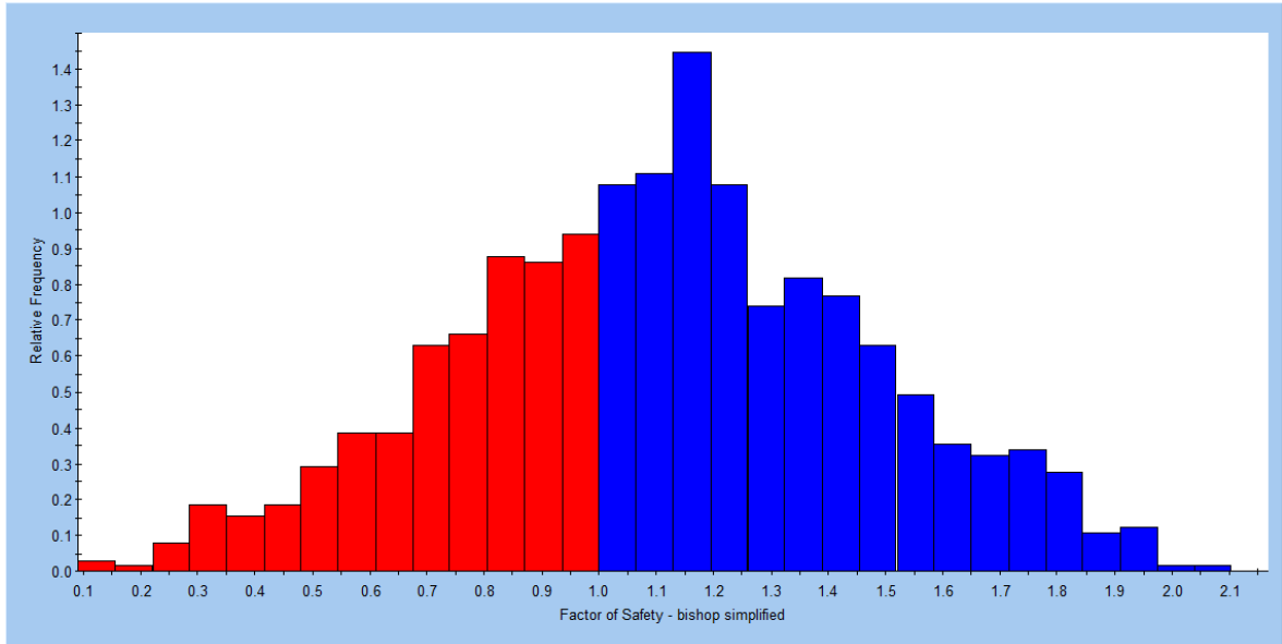
Şekil 9-10 Km:21+820 şev profilinde 34° basamak geometrisinin statik durum olasılıklı duraylılık analizinde belirlenen güvenlik katsayılarının (GK) histogram grafiği
