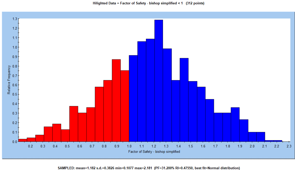
Şekil 9-20 27° basamak geometrisiyle oluşturulan km:21+820 şev profilinde kh=0.07 durumundaki olasılıklı duraylılık analizinde belirlenen güvenlik katsayılarının (GK) histogram grafiği
