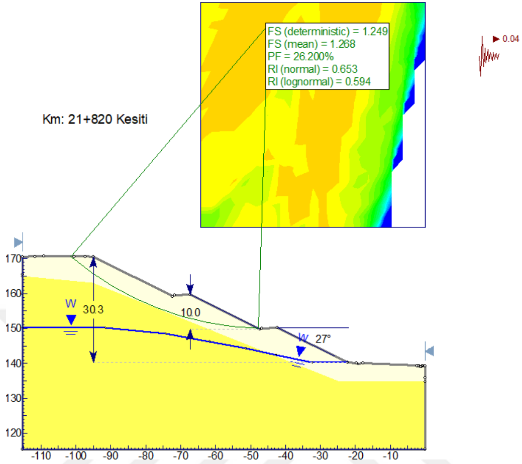
Şekil 9-27 27° basamak geometrisiyle oluşturulan km:21+820 şev profilinde kh=0.04 durumundaki olasılıklı duraylılık analizi
