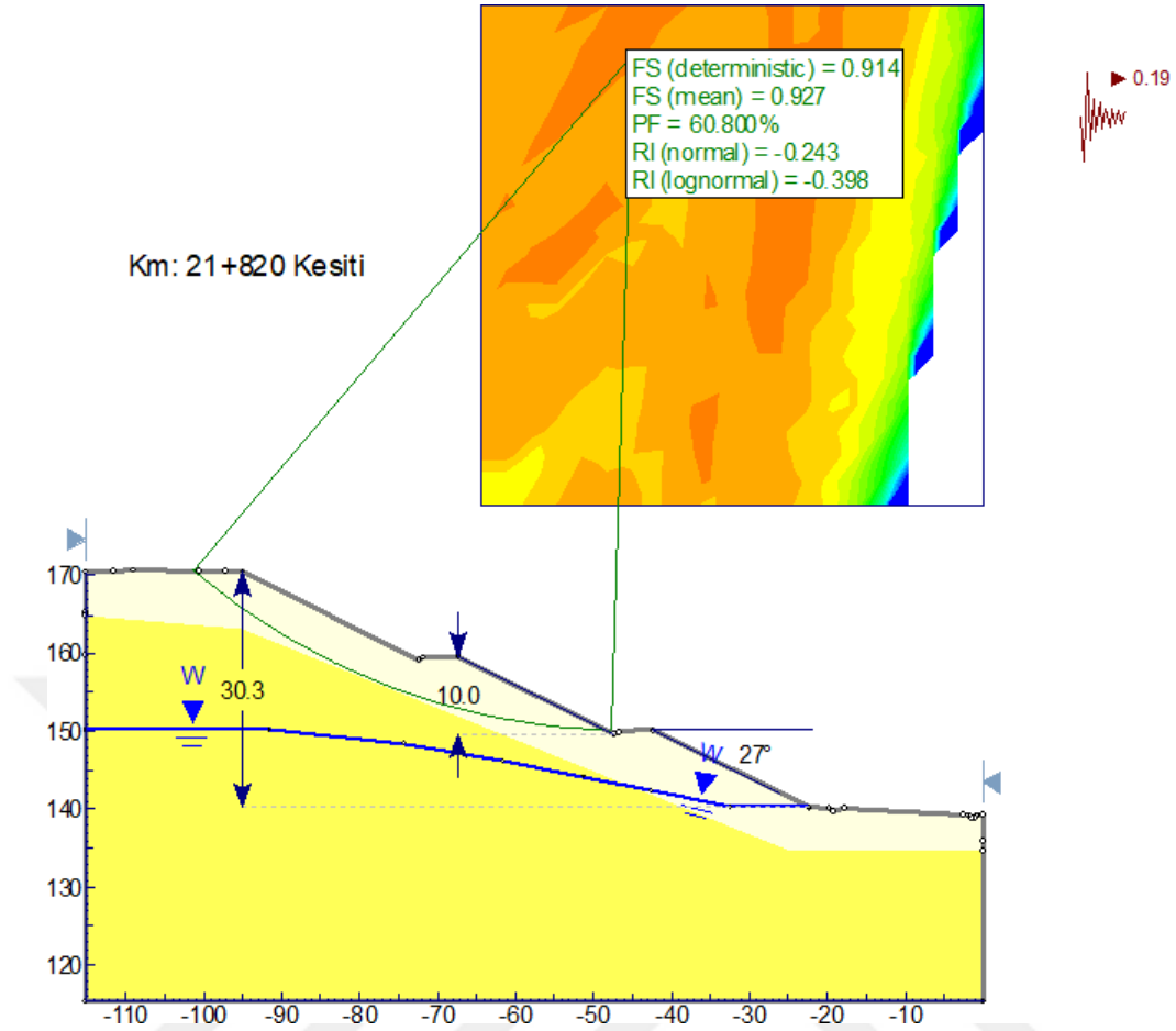
Şekil 9-13 27° basamak geometrisiyle oluşturulan km:21+820 şev profilinde k_h=0.19 durumundaki olasılıklı duraylılık analizi
