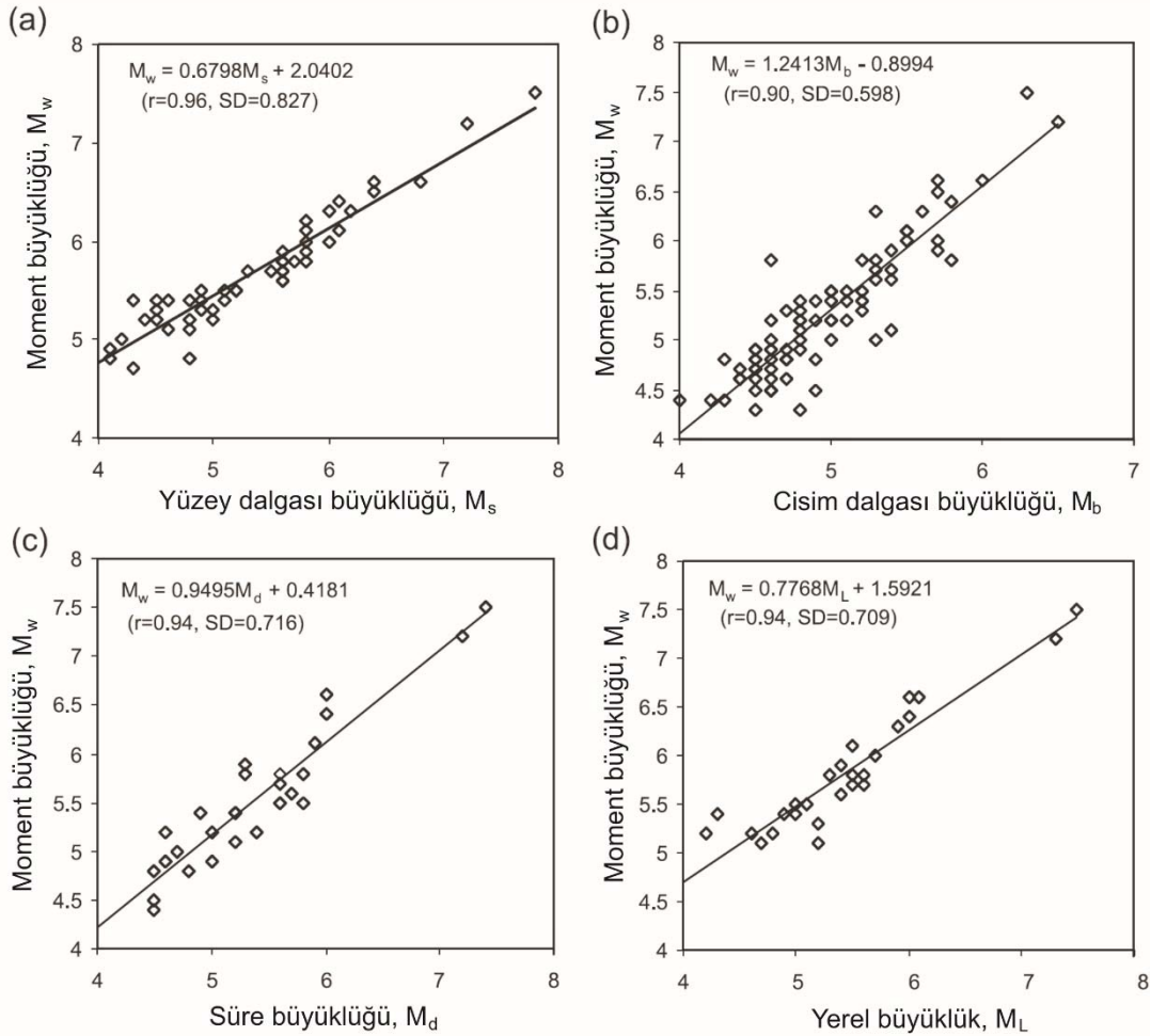
Şekil 5-8 Türkiye deprem verileri kullanılarak Ulusay vd. [15] tarafından önerilen farklı deprem büyüklük ölçekleriyle moment büyüklük arasındaki ilişkiler.
