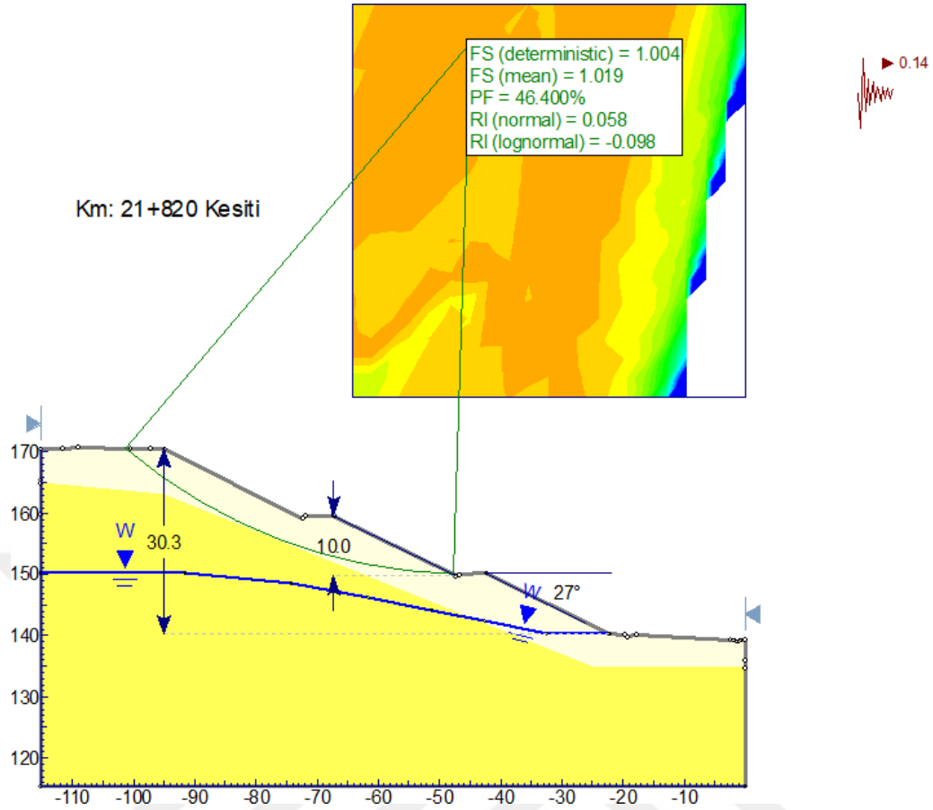
Şekil 9-15 27° basamak geometrisiyle oluşturulan km:21+820 şev profilinde kh=0.14 durumundaki olasılıklı duraylılık analizi
