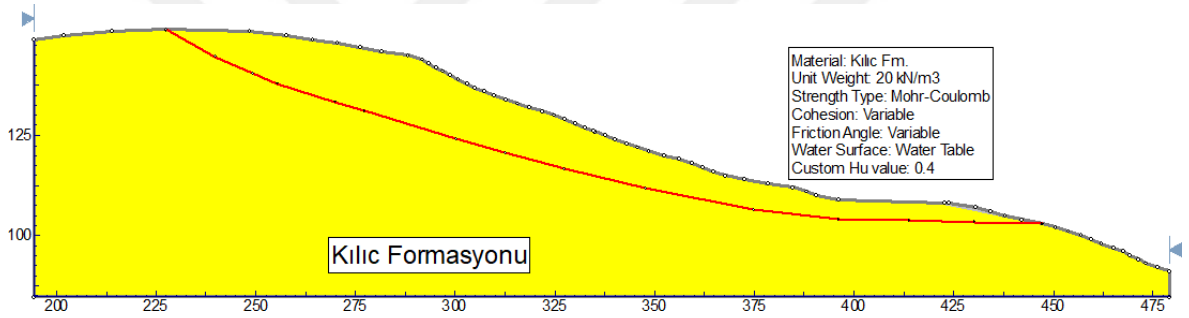
Şekil 8-2 B-B' kesiti geriye dönük analiz modeli
