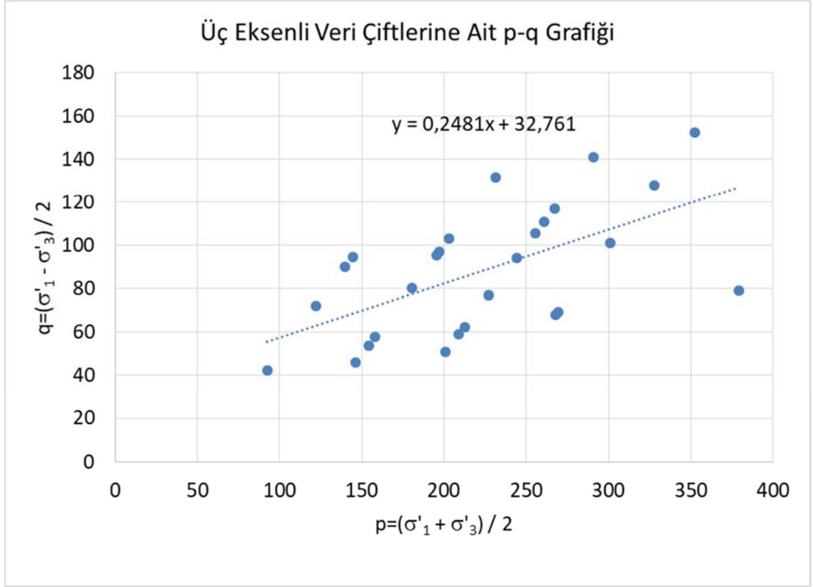
Şekil 7-5 Üç eksenli deney veri çiftlerine ait p-q grafiği
