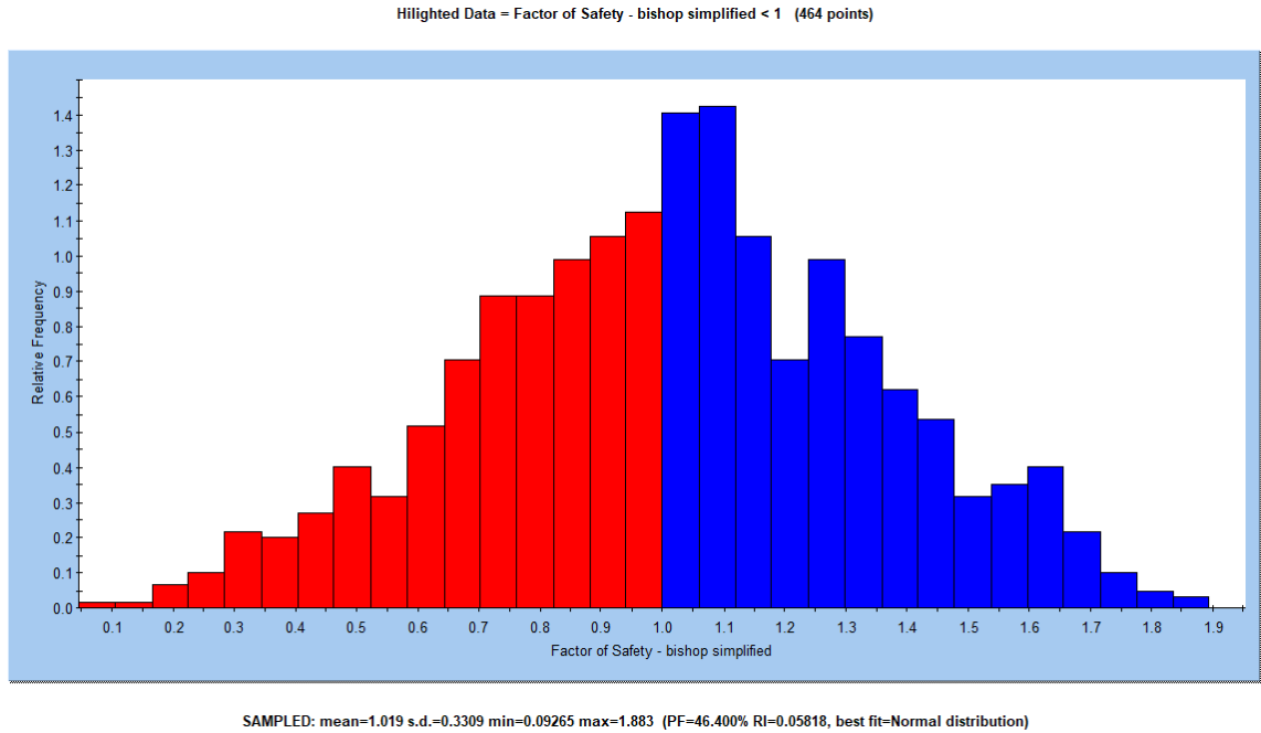
Şekil 9-16 27° basamak geometrisiyle oluşturulan km:21+820 şev profilinde kh=0.14 durumundaki olasılıklı duraylılık analizinde belirlenen güvenlik katsayılarının (GK) histogram grafiği
