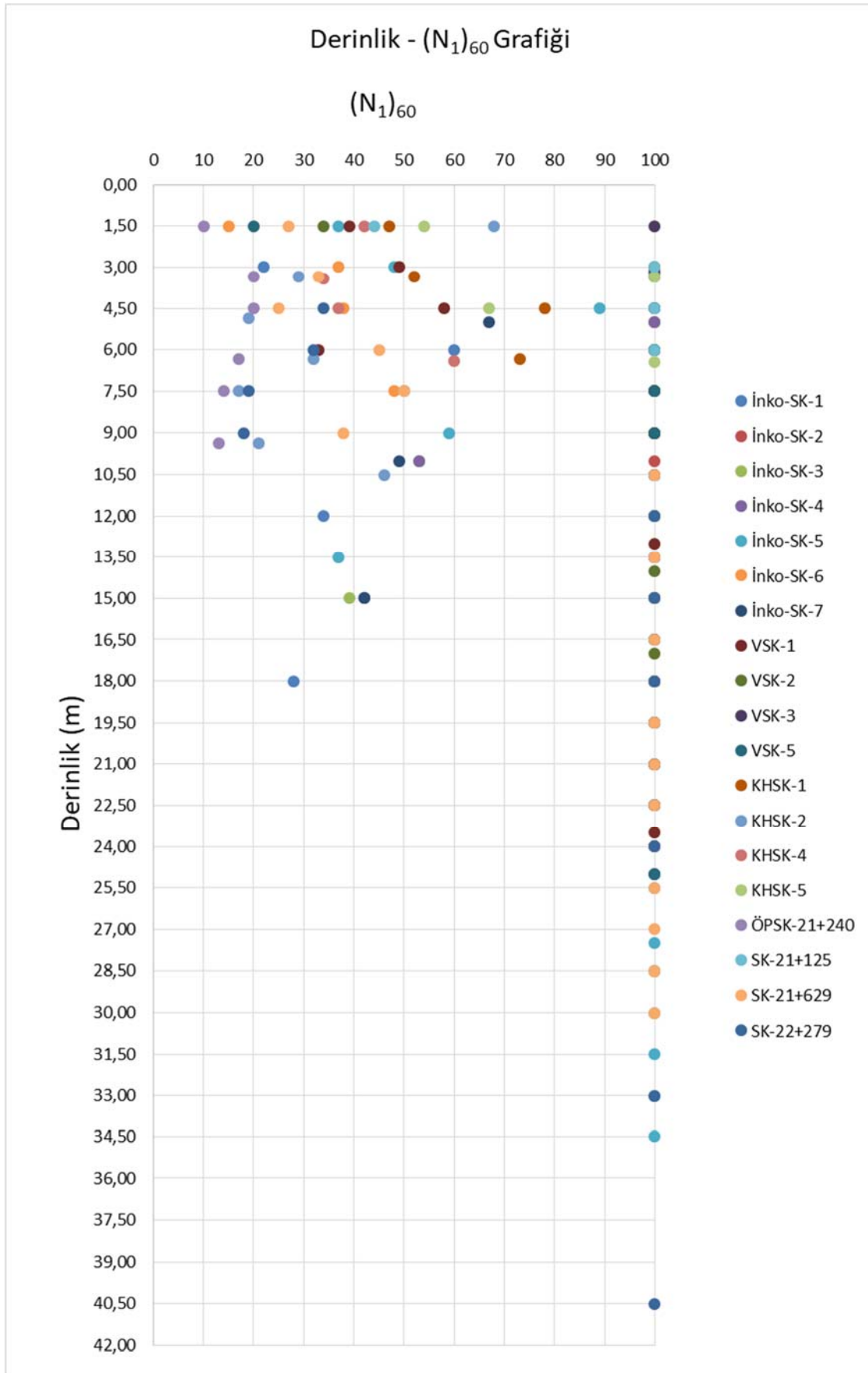
Şekil 6-10 Jeoteknik sondajlara ait (N_1)_{60} değerlerinin derinlik ile değişimi
