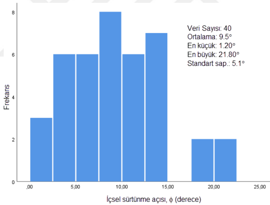
Şekil 9-3 Çalışma alanında kayan kütle için farklı yaklaşımlarla elde edilen makaslama dayanım parametresi çiftlerinin ( c ve \phi ) ayrı ayrı istatistiksel değerlendirmeleri ve histogram grafikleri (a) kohezyon ve (b) içsel sürtünme açısı
