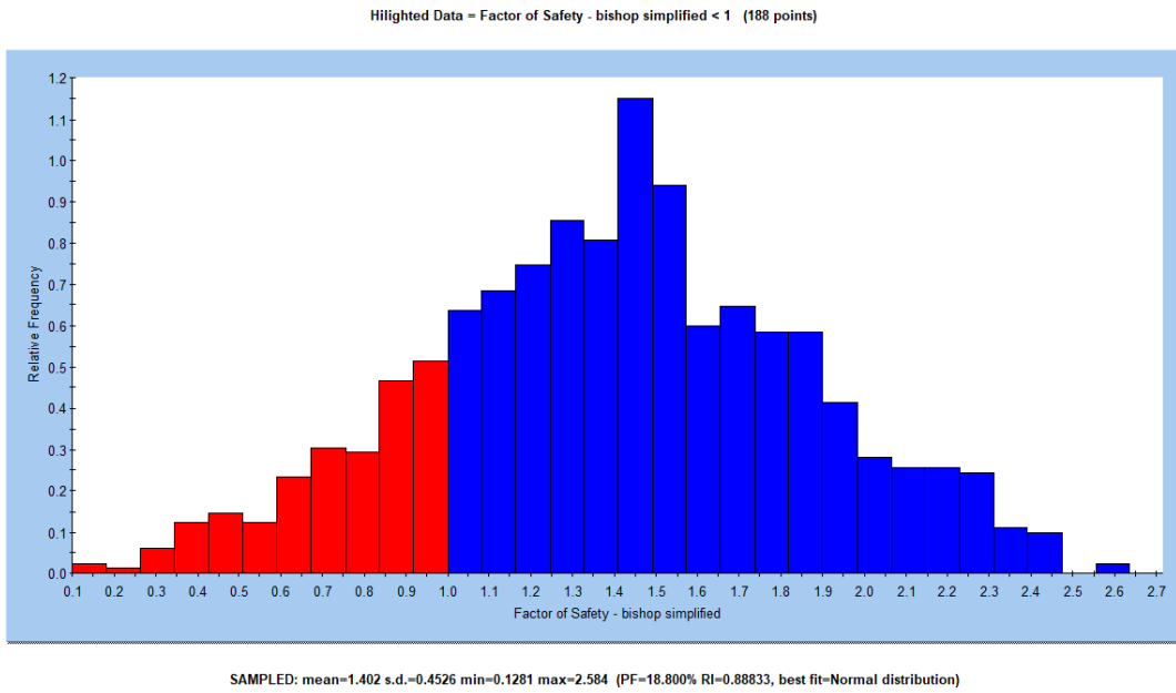
Şekil 9-12 Km:21+820 şev profilinde 27° basamak geometrisinin statik durum olasılıklı duraylılık analizinde belirlenen güvenlik katsayılarının (GK) histogram grafiği
