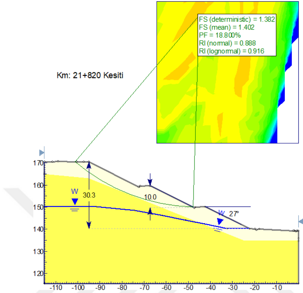
Şekil 9-11 Km:21+820 şev profilinde 27° basamak geometrisinin statik durum olasılıklı duraylılık analizi
