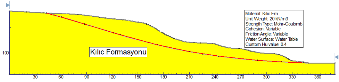
Şekil 8-3 C-C' kesiti geriye dönük analiz modeli
