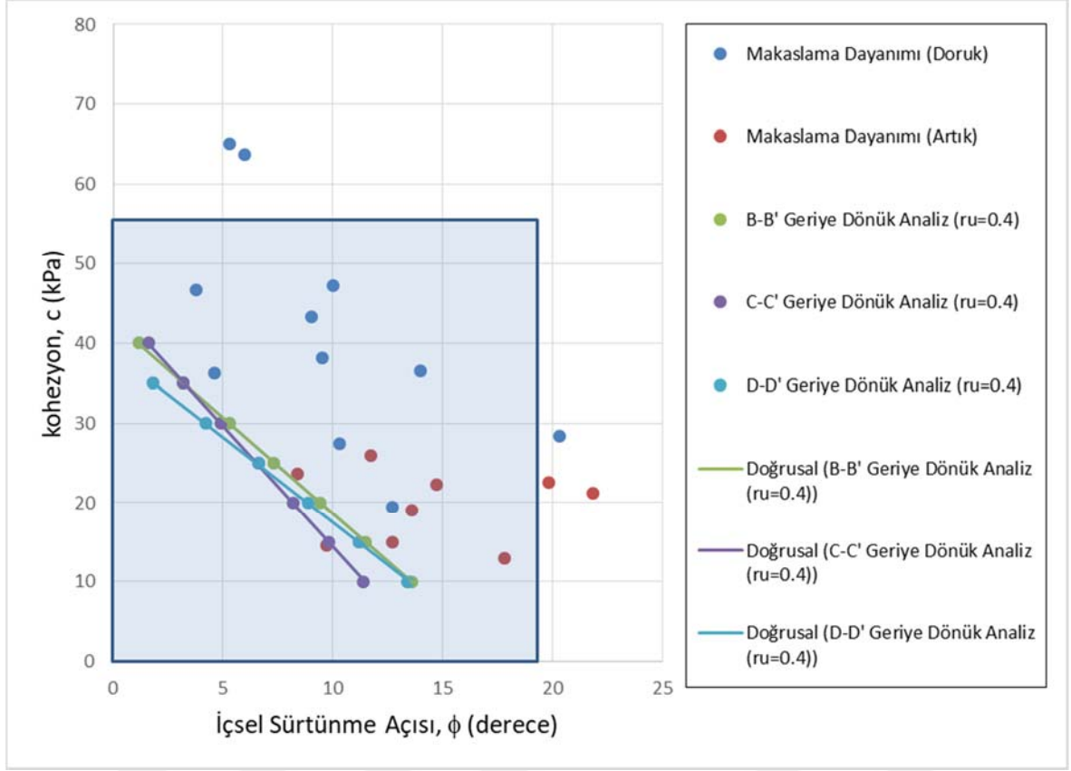
Şekil 9-2 Çalışma kapsamında derlenen tüm kohezyon ve içsel sürtünme açısı çiftlerinin c - \phi grafiği
