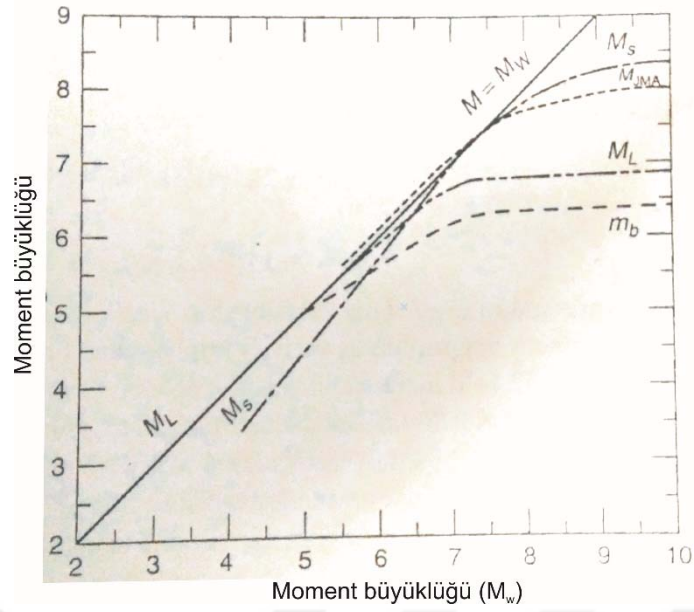
Şekil 5-7 Moment büyüklüğüne ( M_w ) göre diğer deprem büyüklük ölçeklerinin doygunluk grafiği [16]
