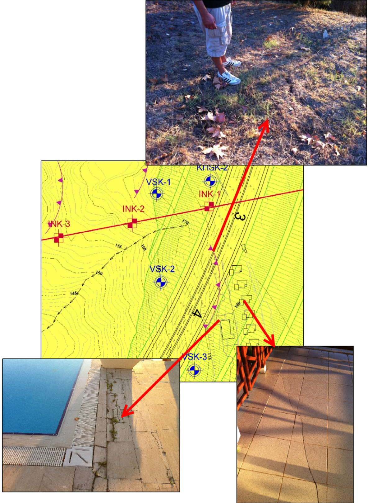
Şekil 6-1 Saha çalışmaları sırasında gözlenen bazı çatlak ve deformasyonlar
