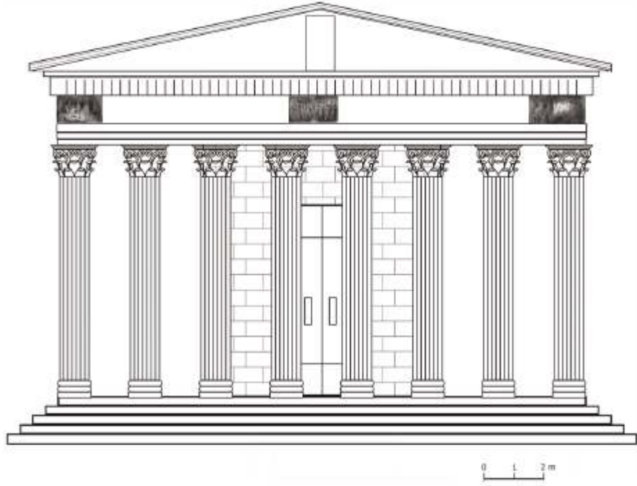
Resim Ek 1.7. Lagina Hekate Tapınağı'nın Doğu cephesi (Herring 2020, 252, figür 5)
