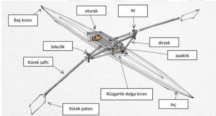
Şekil 2.1. Tekne üzerindeki donanımların gösterimi
