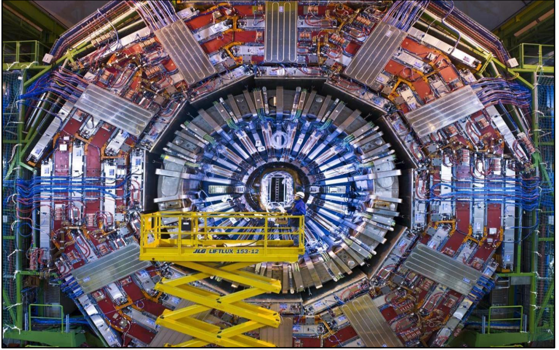
Şekil 1.5. CMS detektörü [17]
