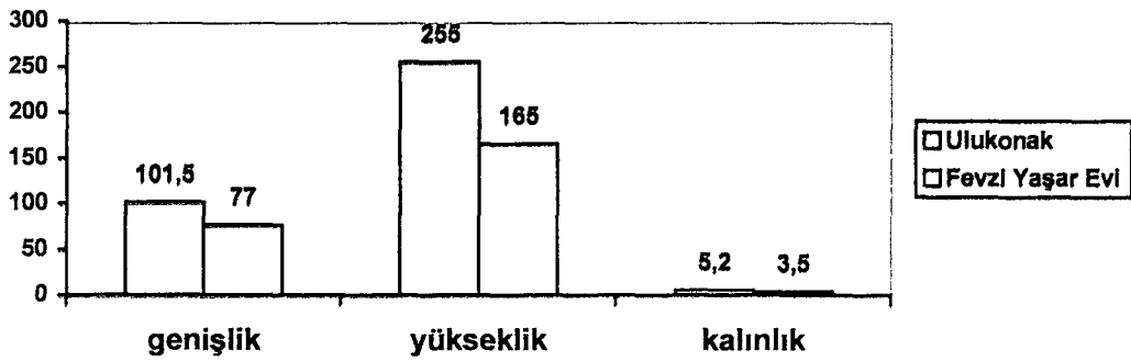
Şekil 5.8. Avlu Kapılarında Kanat Ölçüleri (cm)
