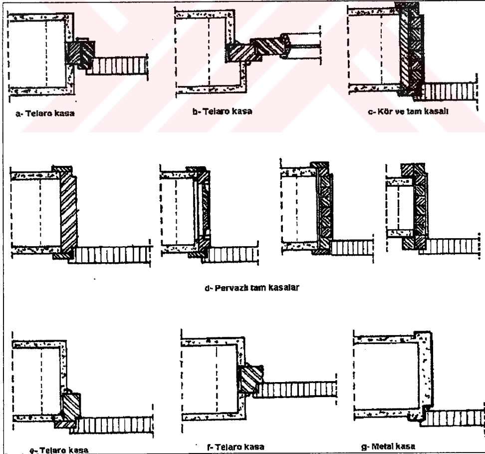
Şekil 3.1. Çeşitli kapı kasası türleri (7).
