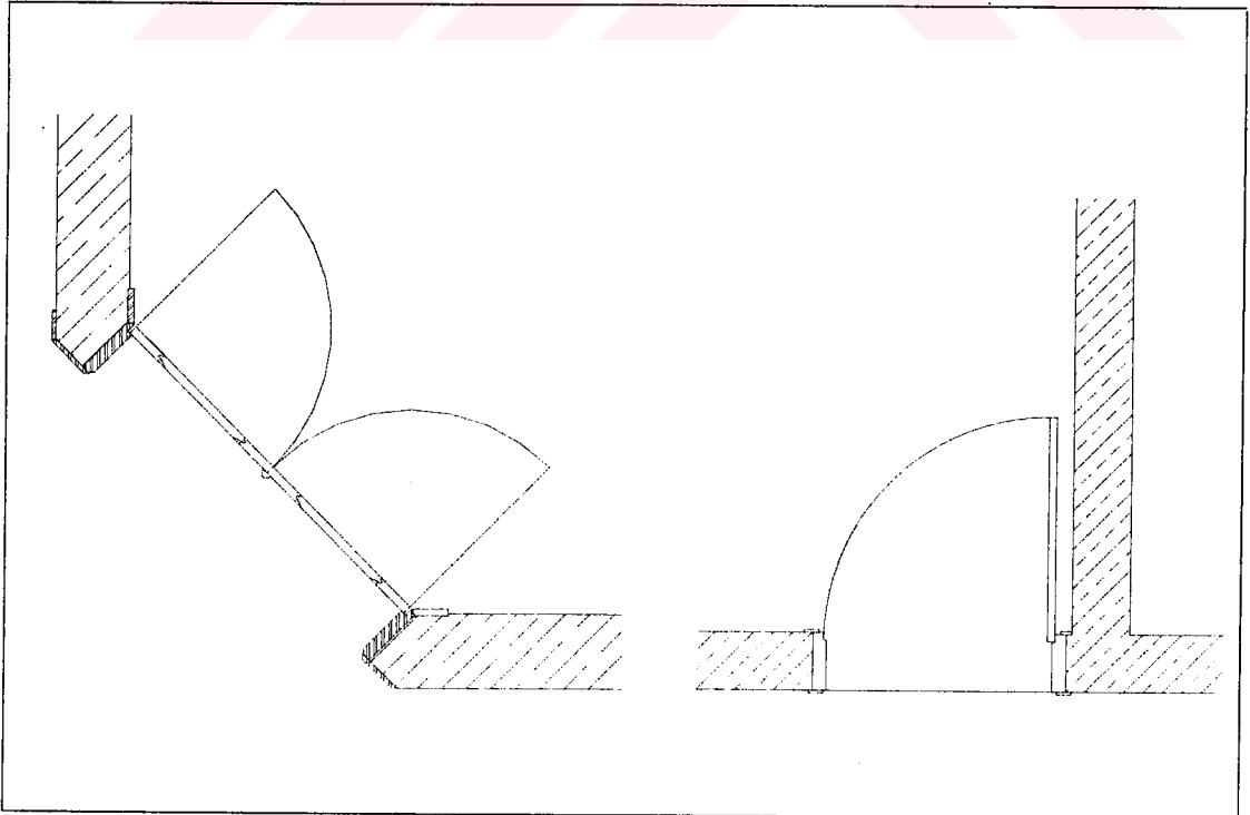
Şekil 5.3. Afyon ve İlçeleri Oda Kapılarının Plandaki Yeri
