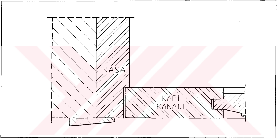
Şekil 5.1. Geleneksel Kapılarda Uygulanan Lambasız Tek Binili Kapı Kanadı
