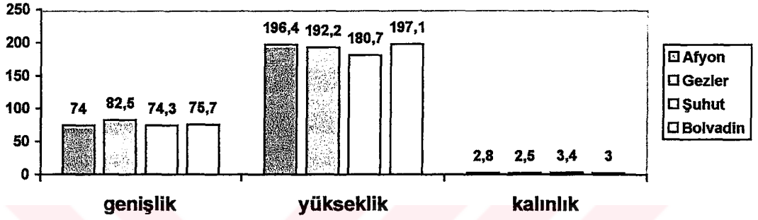
Şekil 5.10. İncelenen Oda Kapılarında Kanat Ölçüleri Ortalamaları (cm)
