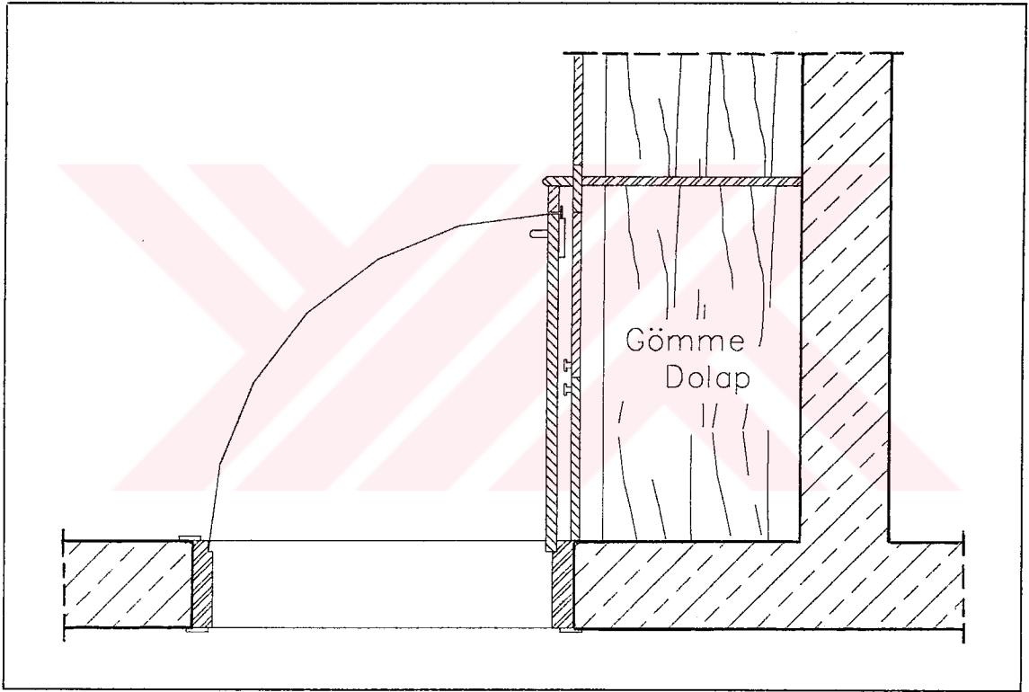
Şekil 5.4. Oda Kapısının Açık Halde Kapı Arkasında, Gömme Dolap Önündeki Özel Yuvasına Oturması
