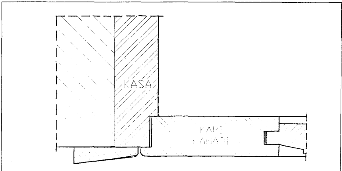
Şekil 5.2. Günümüz Kapılarında Uygulanan Lambalı Çift Binili Kapı Kanadı
