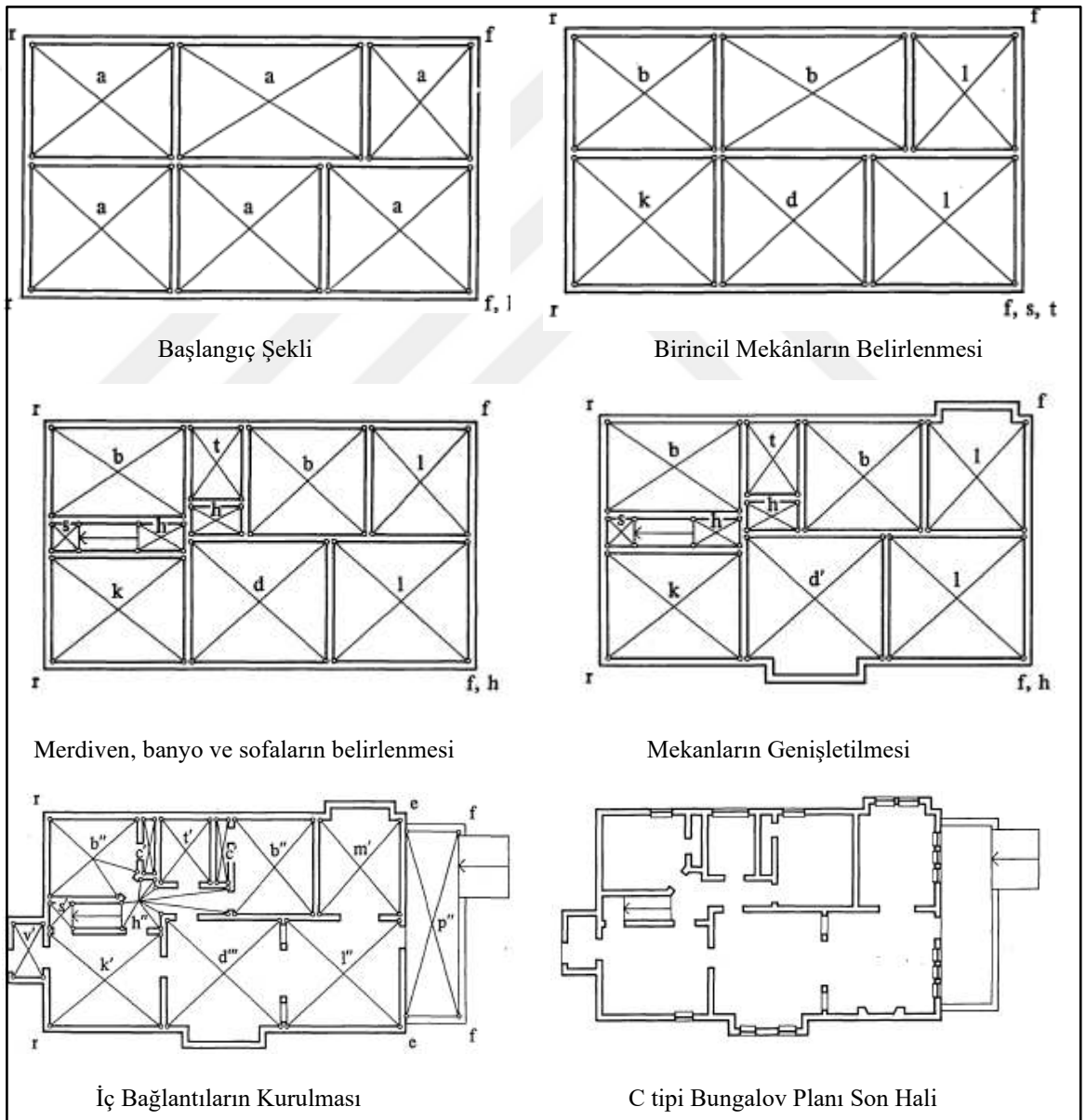
Şekil 3.62.C tipi Bungalov Üretim Aşamaları (Downing ve Flemming 1981)
