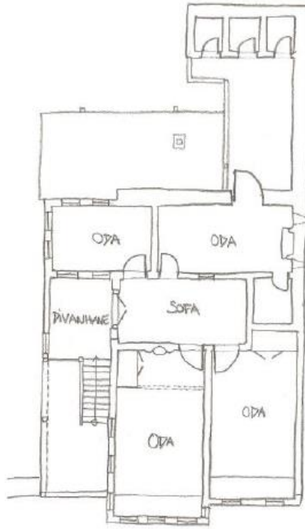
Şekil 3.30. Tapikler Evi Planında Oda Sofa İlişkisi (Çelimli 2016)
