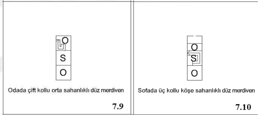
Şekil 4.26. İç Sofalı Plan Tipinde Merdiven Biçimi ve Yerleşimini Belirleyen Kurallar
