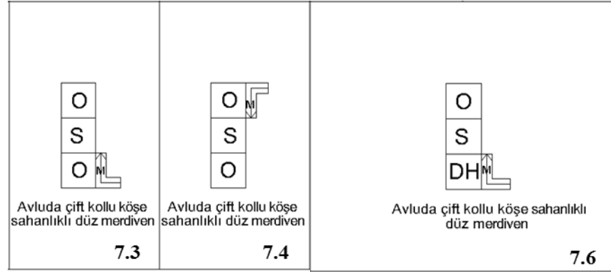
Şekil 4.25. İç Sofalı Plan Tipinde Merdiven Biçimi ve Yerleşimini Belirleyen Kurallar
