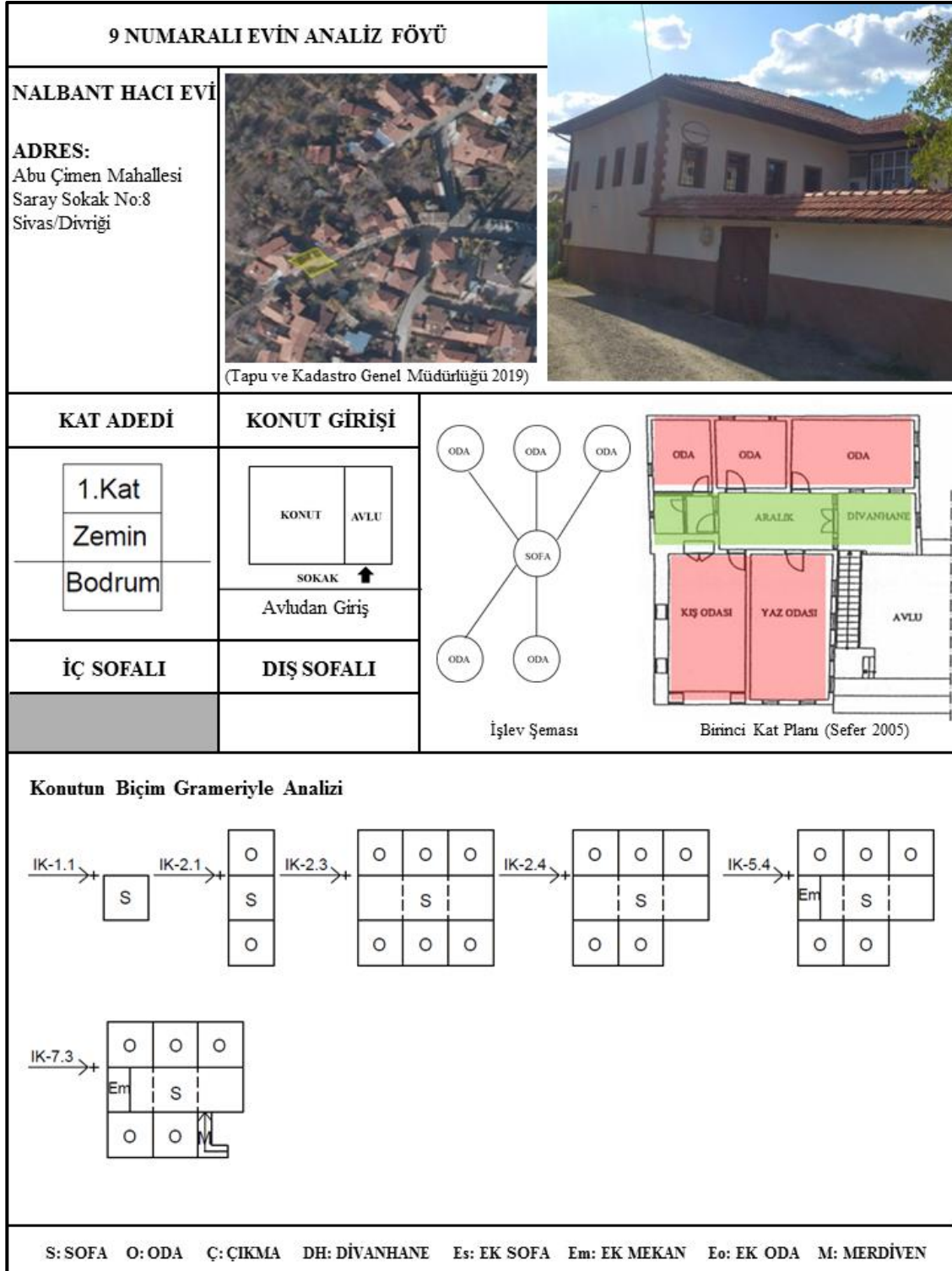
Şekil 4.37. 9 Numaralı Evin Analiz Föyü
