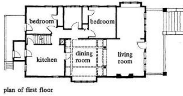
Şekil 3.61. C tipi Bungalova Ait 1. Kat Planı (Downing ve Flemming 1981)
