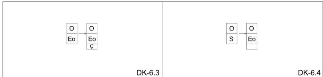
Şekil 4.22. Dış Sofalı Plan Tipinde Çıkmaları Belirleyen Kurallar (Çağdaş 1996'dan revize edilmiştir)
