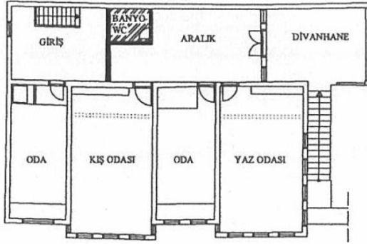
Şekil 3.31. Dış Sofalı Plan Tipi Örneği (Sefer 2005)
