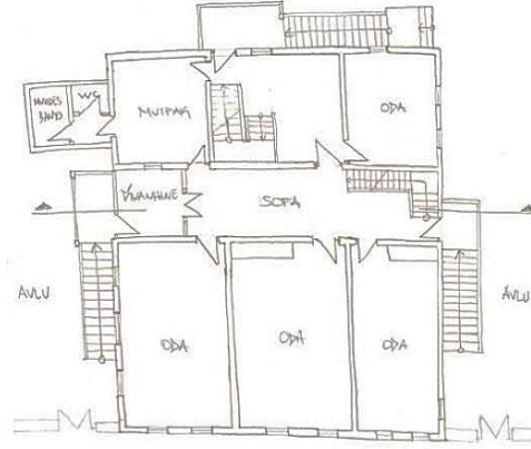
Şekil 3.32. İç Sofalı Plan Tipi Örneği (Çelimli 2016)
