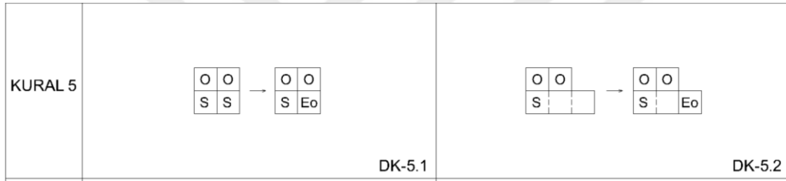
Şekil 4.17. Dış Sofalı Plan Tipinde Ek Oda ve Ek Mekânların Yerleşimini Belirleyen Kurallar (Çağdaş 1996'dan revize edilmiştir)
