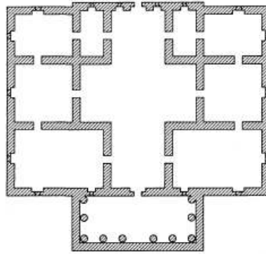
Şekil 3.55. Villa Malcotenta'ya Ait Planın Son Hali ( Stiny ve Mitchell1978)
