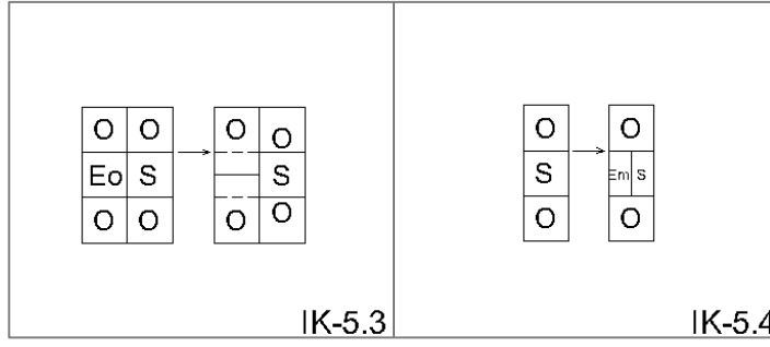
Şekil 4.16. İç Sofalı Plan Tipinde Ek Oda ve Ek Mekânların Yerleşimini Belirleyen Kurallar (Çağdaş 1996'dan revize edilmiştir)
