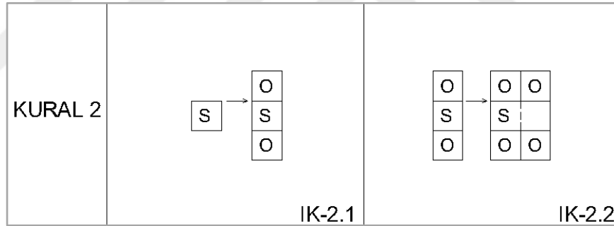
Şekil 4.3. İç Sofalı Plan Tipinde Oda Sayısı ve Yerleşimini Belirleyen Kurallar (Çağdaş 1996)
