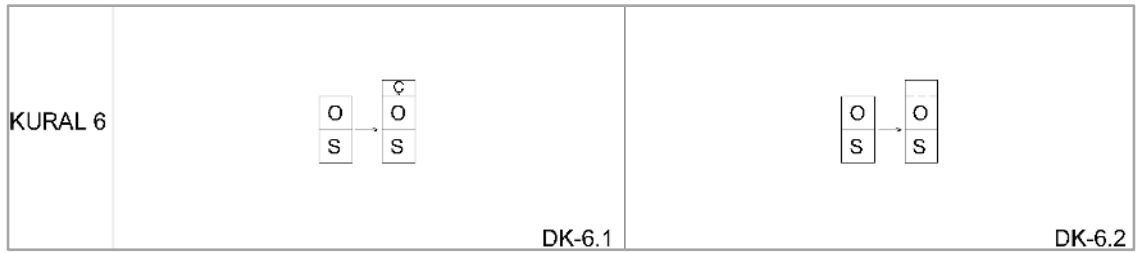
Şekil 4.21. Dış Sofalı Plan Tipinde Çıkmaları Belirleyen Kurallar (Çağdaş 1996'dan revize edilmiştir)
