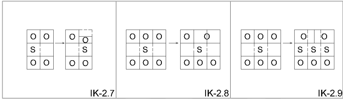
Şekil 4.6. İç Sofalı Plan Tipinde Oda Sayısı ve Yerleşimini Belirleyen Kurallar (Çağdaş 1996'dan revize edilmiştir)
