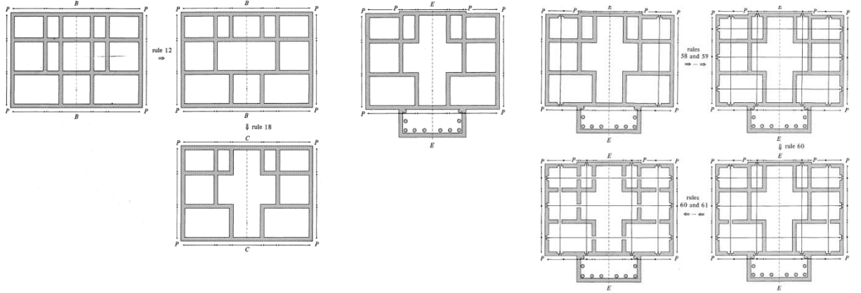
Şekil 3.54. Villa Malcontenta' nın Üretim Aşamaları ( Stiny ve Mitchell1978)
