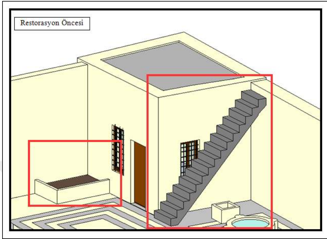
Ek 11 Emine Göğüş Mutfak Müzesi Rölöve ve Restorasyon Projesi Avlu Restorasyon Öncesi ve Sonrası
