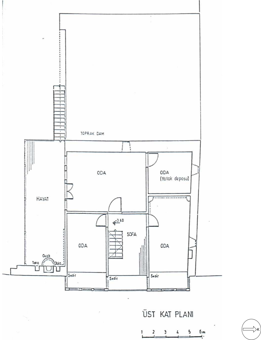
Şekil 1.6. Hacı Cumali Ağa evi üst kat planı-katalog no:3[33].
