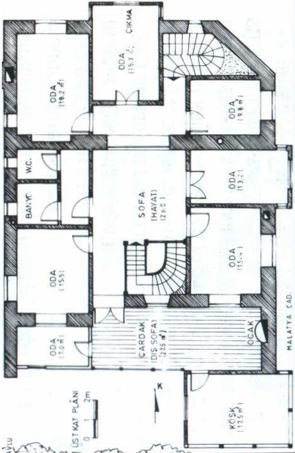
Şekil 1.54. Ahmet Kekevi evi üst kat planı-katalog no:27[33].
