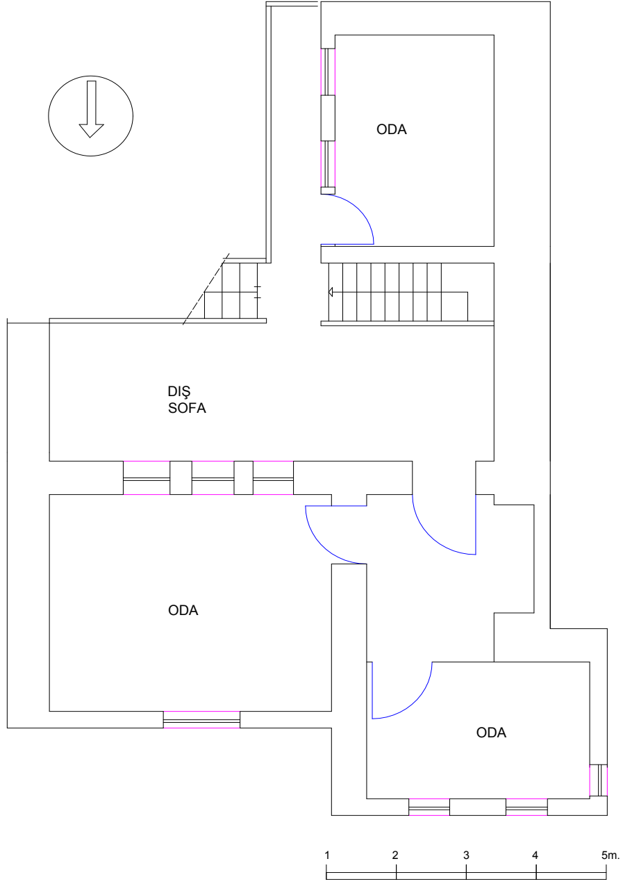
Şekil 1.38. 7 Nolu ev üst kat planı-katalog no:19
