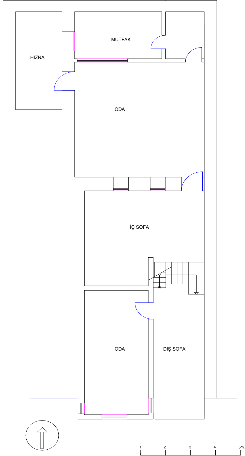
Şekil 1.46. 38 Nolu ev üst kat planı-katalog no:23
