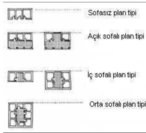
Şekil 3.1. 'Geleneksel Anadolu Evi' plan tipolojisi[5].
