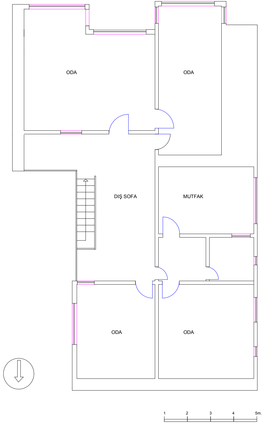
Şekil 1.50. 176 Nolu ev üst kat planı-katalog no:25
