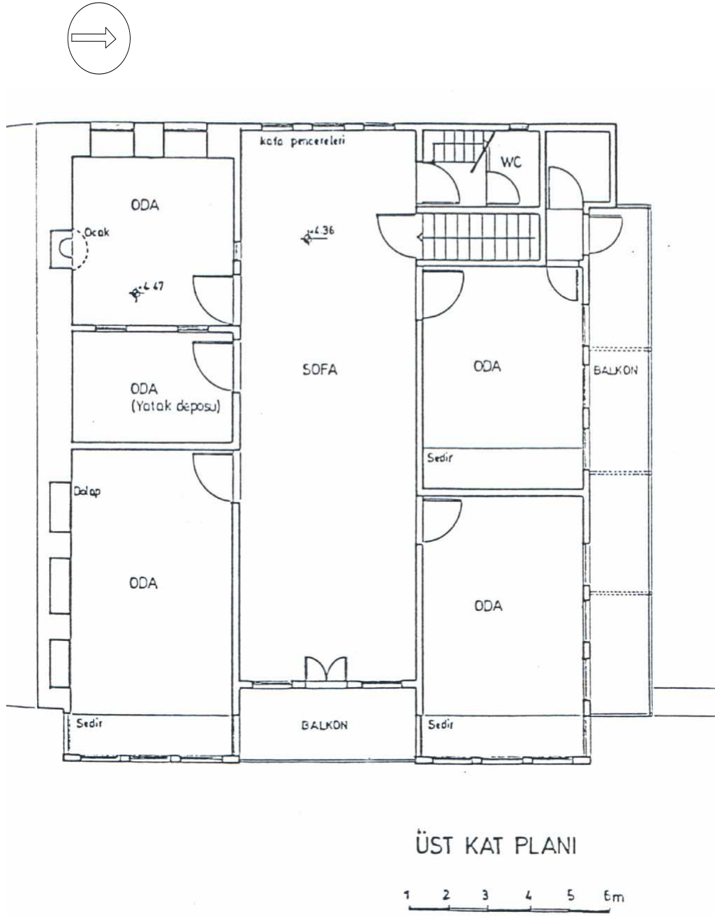
Şekil 1.24. Süheyla Hanım evi üst kat planı-katalog no:12[33].
