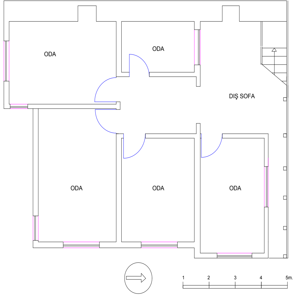
Şekil 1.52. 196 Nolu ev üst kat planı-katalog no:26
