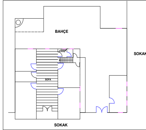
Şekil 4.1. Geleneksel evde çekirdek yaşama birimlerinin tekrarlarından oluşan yaşama katı örneği-katalog no:12
