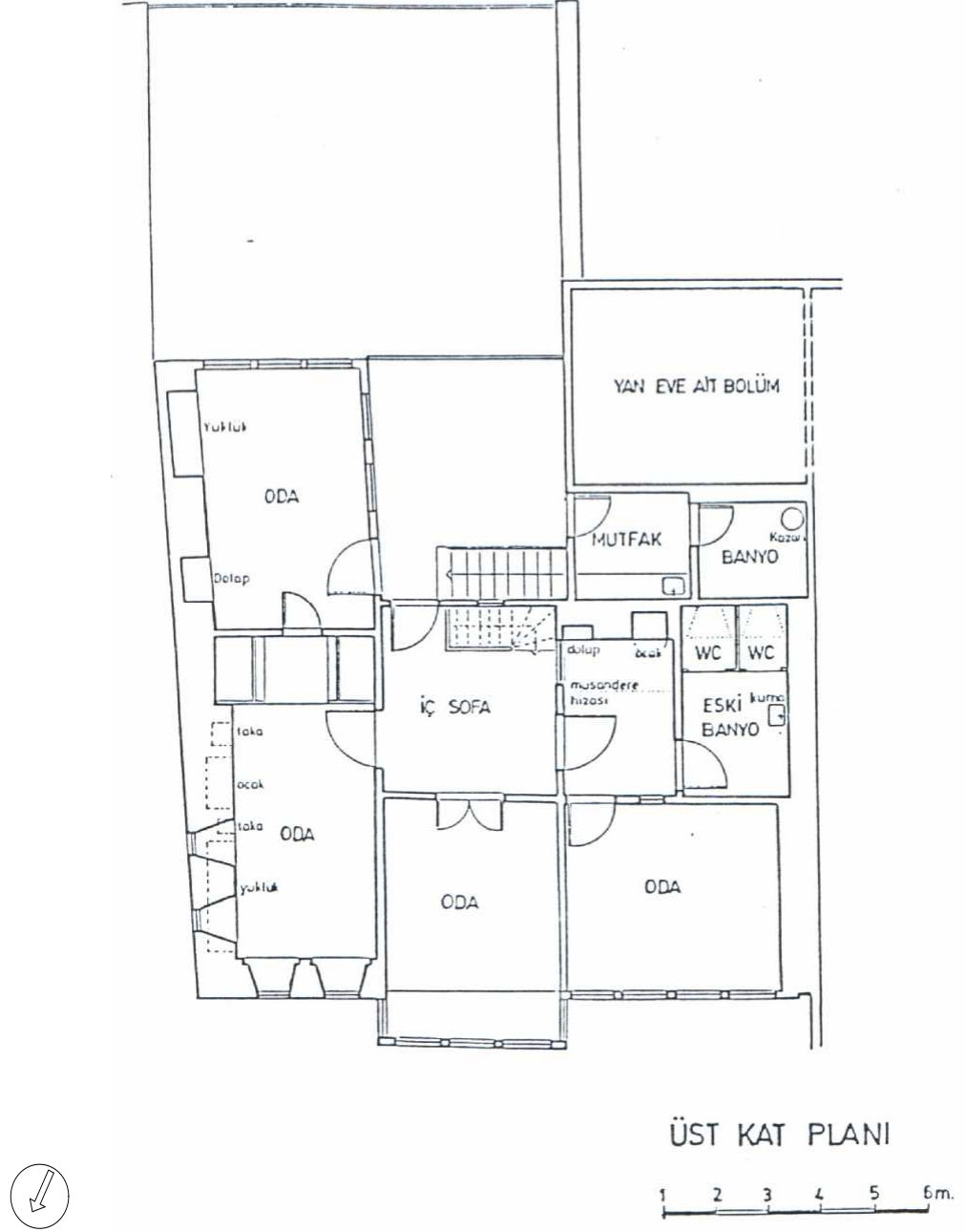
Şekil 1.12. Vahap Elgin evi üst kat planı-katalog no:6[33].
