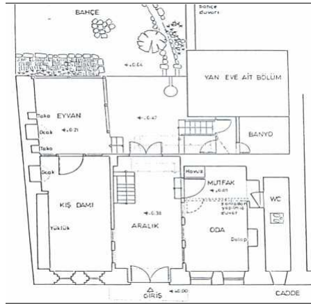
Şekil 3.3. Geleneksel Malatya evi zemin kat/ Aralık, Kış Damı, Hızna,Eyvan örneği- katalog no:6
