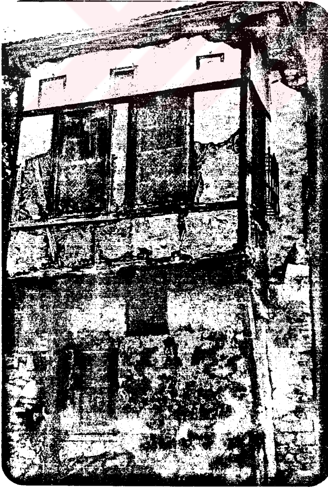
Fotoğraf 8. Payandaları duvar içindeki hatıllara veya dikmelere oturmuş çıkma (Yen. 1-1).
