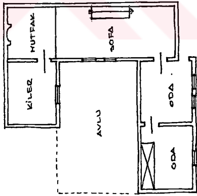
AVLU KİLEÇ MUTFAK SOFA ODA ODA ÜST KAT PLANI
