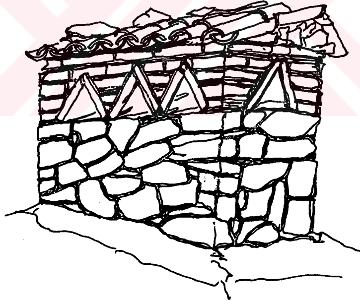
Şekil 2. Ocak veya tandır bacası. Tip 3
