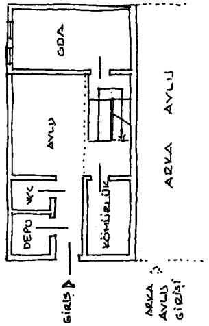
GİRİŞ KATI PLANI
