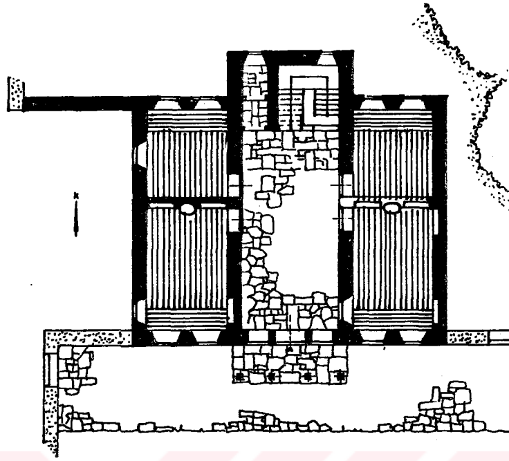
Şekil 6. Konya, Nakipoğulları evi planı.
