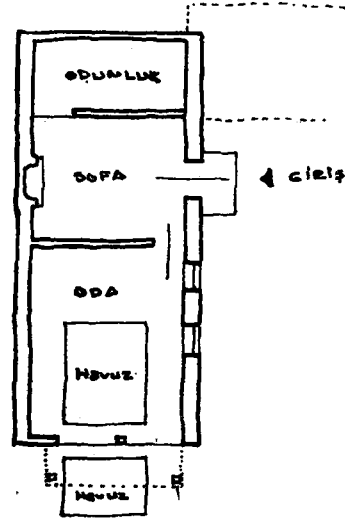
Şekil 5. Başayvaz bağ evi planı.
