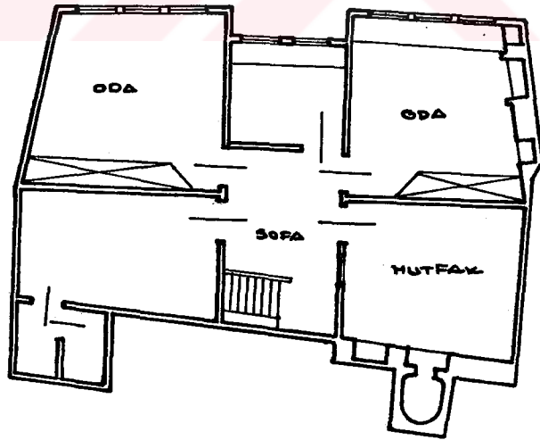
Şekil 7. Göynük, Süloğlu evi planı.
