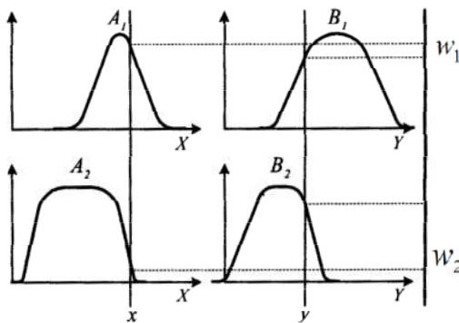
Şekil 3.21. Birinci dereceden iki girişli ve iki kurallı Sugeno bulanık modeli [84]
