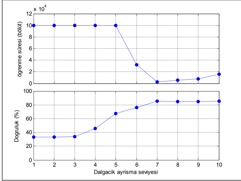
Şekil 4.29. Dalgacık ayrışma seviyesine göre YSA'nın öğrenme süresi ve doğruluğu
