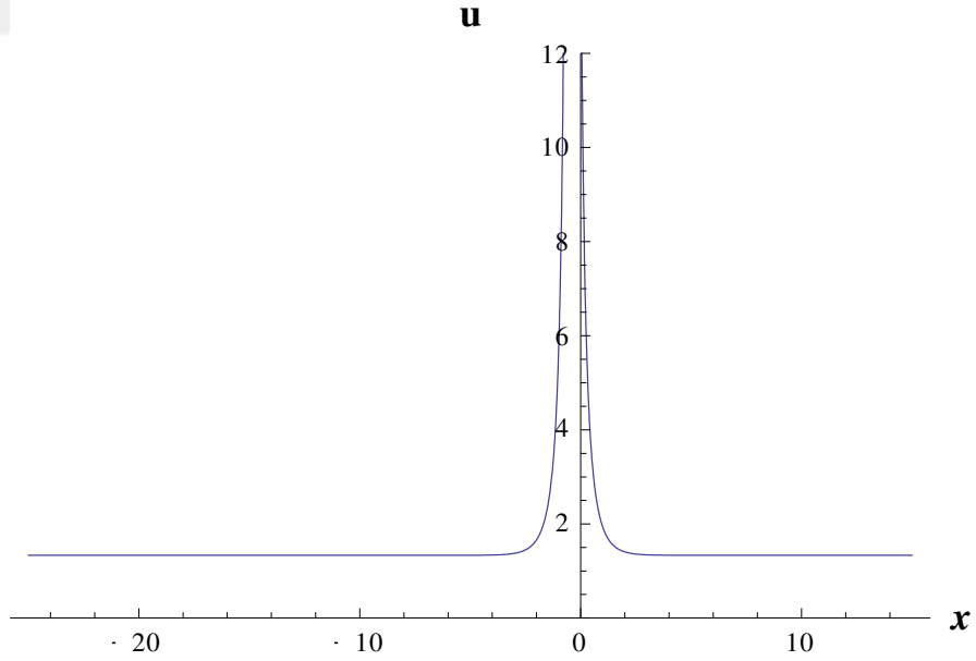
Şekil-4 (4.1.18) denkleminin 2 boyutlu yüzey grafiği
