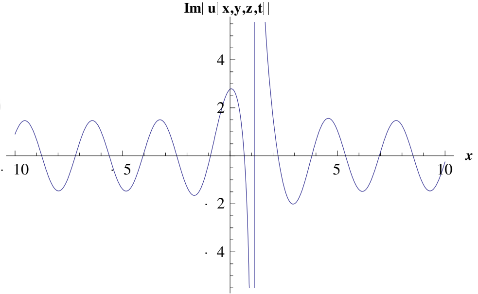
Şekil-8 (4.2.13) denkleminin sanal kısmının 2 boyutlu yüzey grafikleri w=0.5, a=2, b=0.25, c=0.35, d=0.2, E=0.3, y=0.8, z=0.9, -10 \leq x \leq 10, t=0.6
