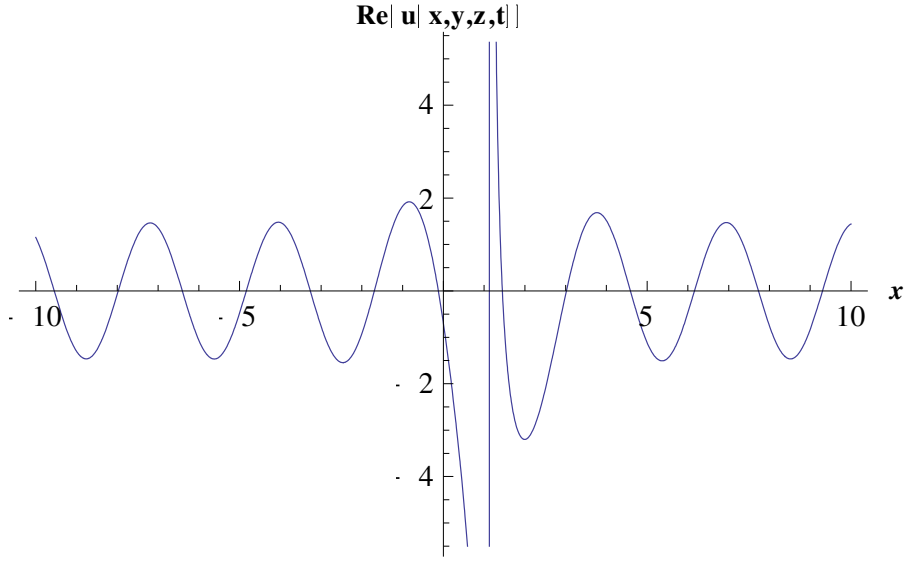
Şekil-7 (4.2.13) denkleminin reel kısmının 2 boyutlu yüzey grafikleri w=0.5, a=2, b=0.25, c=0.35, d=0.2, E=0.3, y=0.8, z=0.9, -10 \leq x \leq 10, t=0.6
