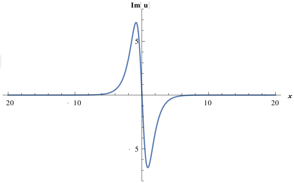
Şekil-28 (4.6.8) denkleminin sanal kısmının 2 boyutlu yüzey grafiği v = 0.1, \quad p = 0.2, \quad t = 0.3, -20 \leq x \leq 20
