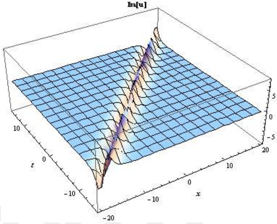
Şekil-30 (4.6.10) denkleminin sanal kısmının 3 boyutlu yüzey grafiği p = 0.1, \quad q = 0.2, \quad t = 0.3, -20 \leq x \leq 20, -15 \leq t \leq 15
