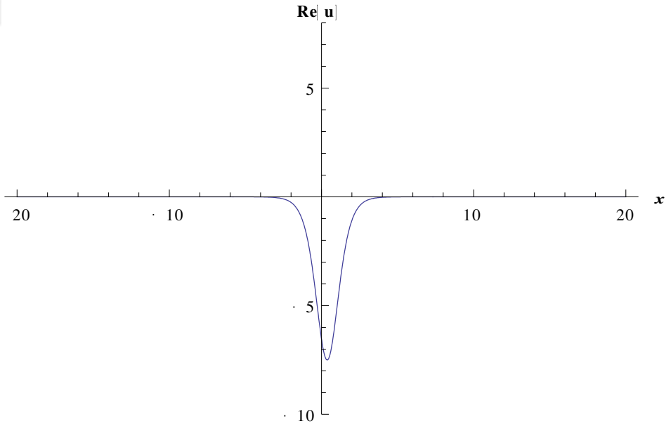
Şekil-31 (4.6.10) denkleminin reel kısmının 2 boyutlu yüzey grafiği p = 0.1, \quad q = 0.2, \quad t = 0.3, -20 \leq x \leq 20.
