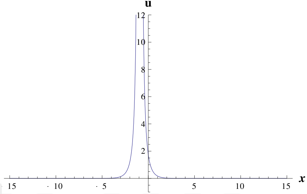
Şekil-2 (4.1.16) denkleminin 2 boyutlu yüzey grafiği
