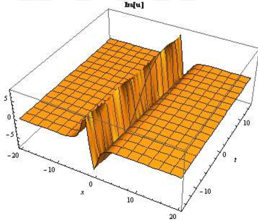
Şekil-26 (4.6.8) denkleminin sanal kısmının 3 boyutlu yüzey grafiği v = 0.1, \quad p = 0.2, \quad t = 0.3, -20 \leq x \leq 20, -15 \leq t \leq 15
