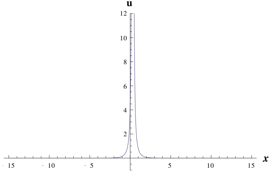
Şekil-10 (4.3.10) denkleminin 2 boyutlu yüzey grafiği
