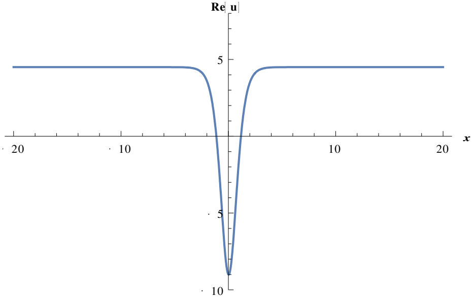
Şekil-27 (4.6.8) denkleminin reel kısmının 2 boyutlu yüzey grafiği v = 0.1, \quad p = 0.2, \quad t = 0.3, -20 \leq x \leq 20
