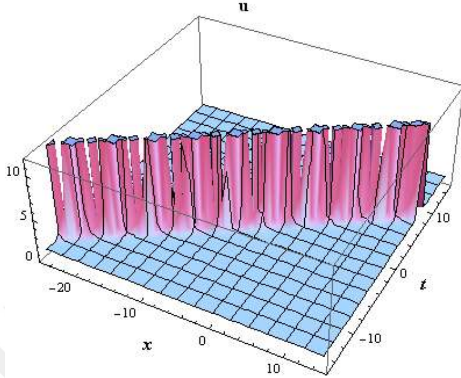
Şekil-3 (4.1.18) denkleminin 3 boyutlu yüzey grafiği
