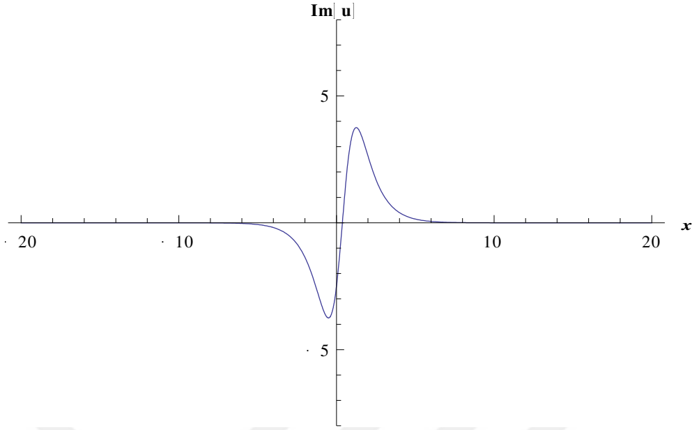
Şekil-32 (4.6.10) denkleminin sanal kısmının 2 boyutlu yüzey grafiği p = 0.1, \quad q = 0.2, \quad t = 0.3, -20 \leq x \leq 20.
