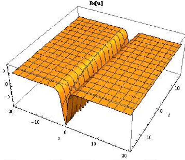
Şekil-25 (4.6.8) denkleminin reel kısmının 3 boyutlu yüzey grafiği v = 0.1, \quad p = 0.2, \quad t = 0.3, -20 \leq x \leq 20, -15 \leq t \leq 15
