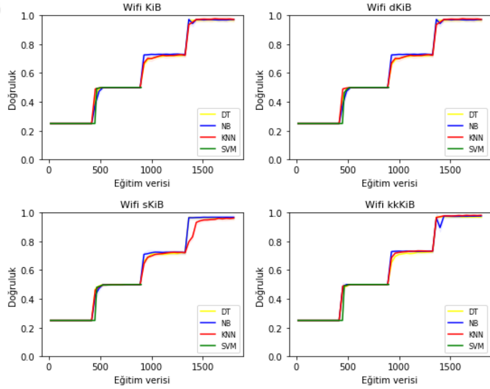
Şekil 4.16. Wifi veri setinin KiB, dKiB, sKiB ve kkKiB için sınıflama başarımlarını gösteren grafik
