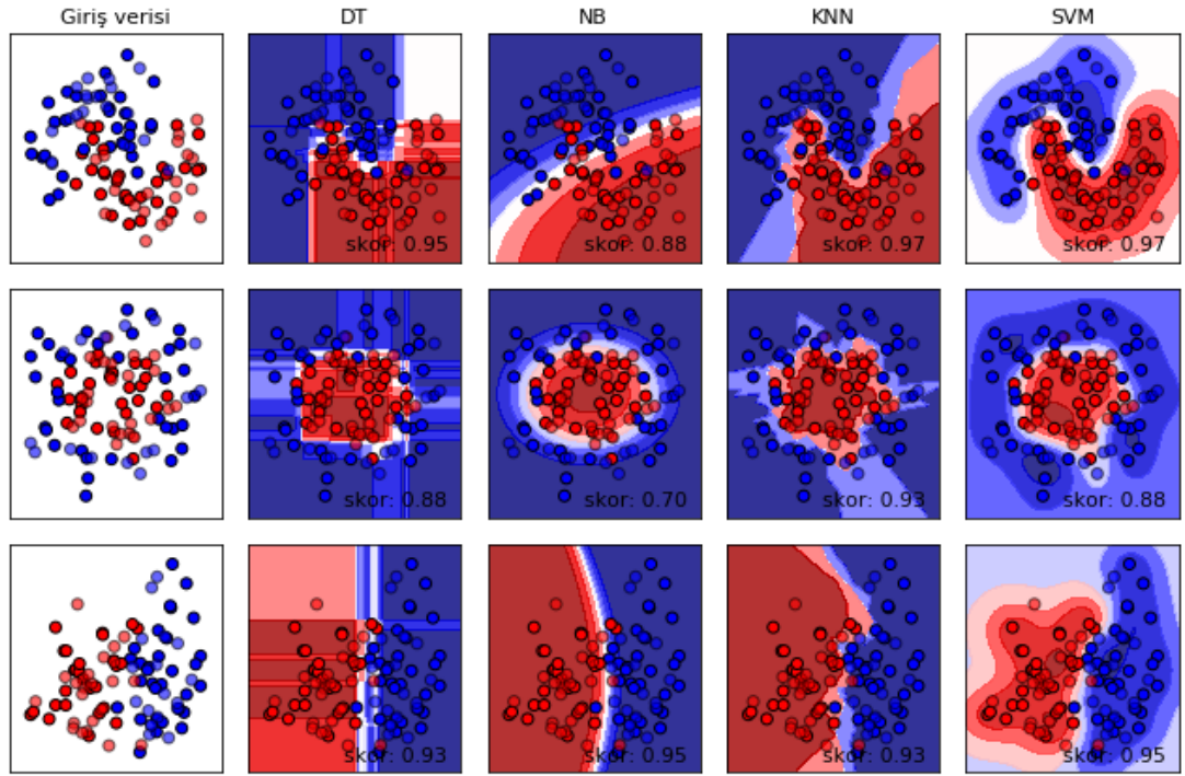
Şekil 3.3. Sınıflama algoritmalarının örnek veri kümeleri üzerinde başarımları
