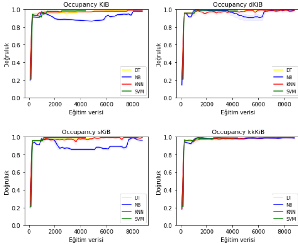
Şekil 4.14. Occupancy veri setinin KiB, dKiB, sKiB ve kkKiB için sınıflama başarımlar grafiği
