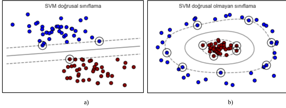
Şekil 3.6. SVM'nin doğrusal (a) ve doğrusal olmayan (b) veri için destek vektörleri
