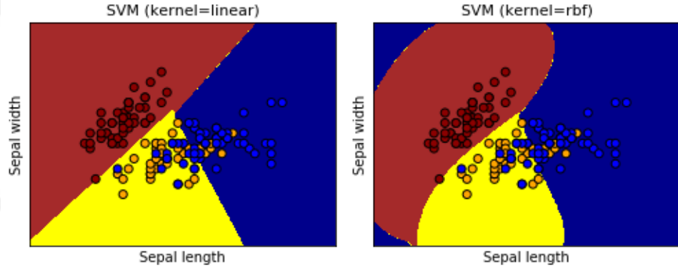
Şekil 3.7. Iris veri setinin farklı iki kernel değeri için SVM ile sınıflandırılması
