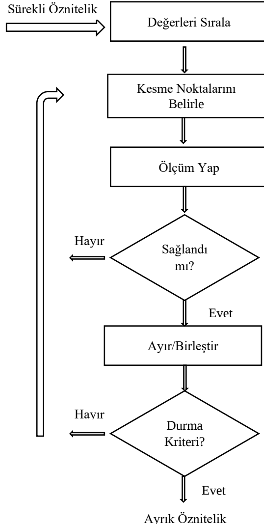
Şekil 1.2. Veri ayırıklaştırma akış diyagramı
