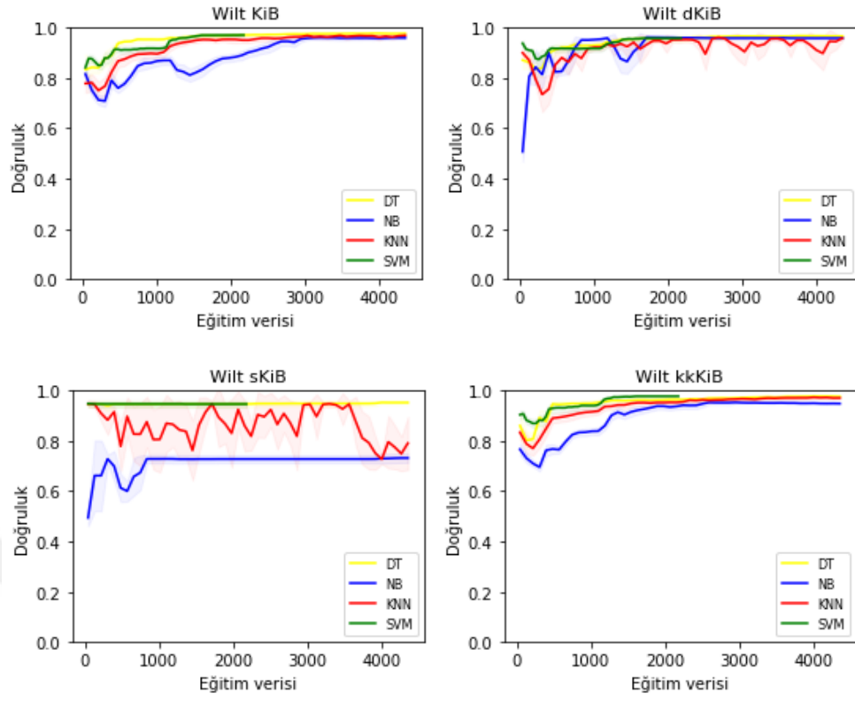
Şekil 4.15. Wilt veri setinin KiB, dKiB, sKiB ve kkKiB için sınıflama başarımlarını gösteren grafik
