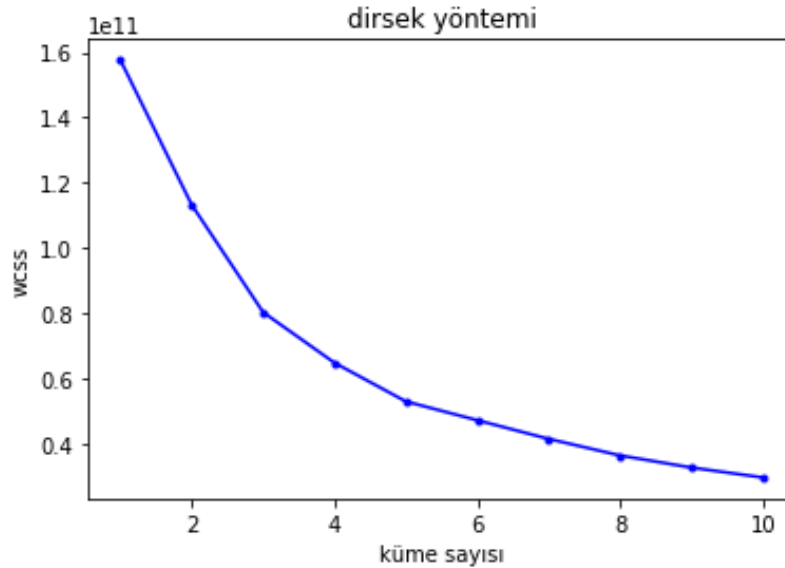
Şekil 3.1. Dirsek yöntemi
