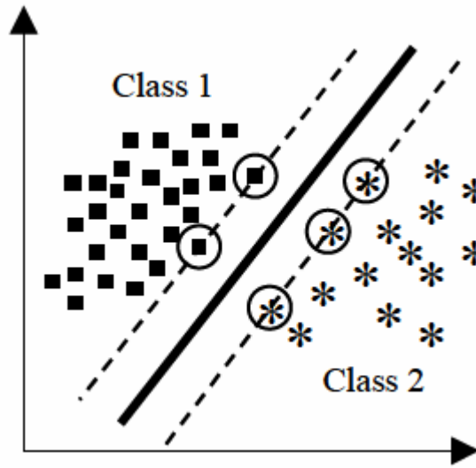
Şekil 6.1 Bir İkili DVM'nin Hiper Düzlem Şeması
