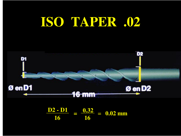
Şekil 1: Taper değerinin şematik gösterimi (Taper =D2-D1/16mm) (Dentsply Maillefer'den temin edilmiştir.)
