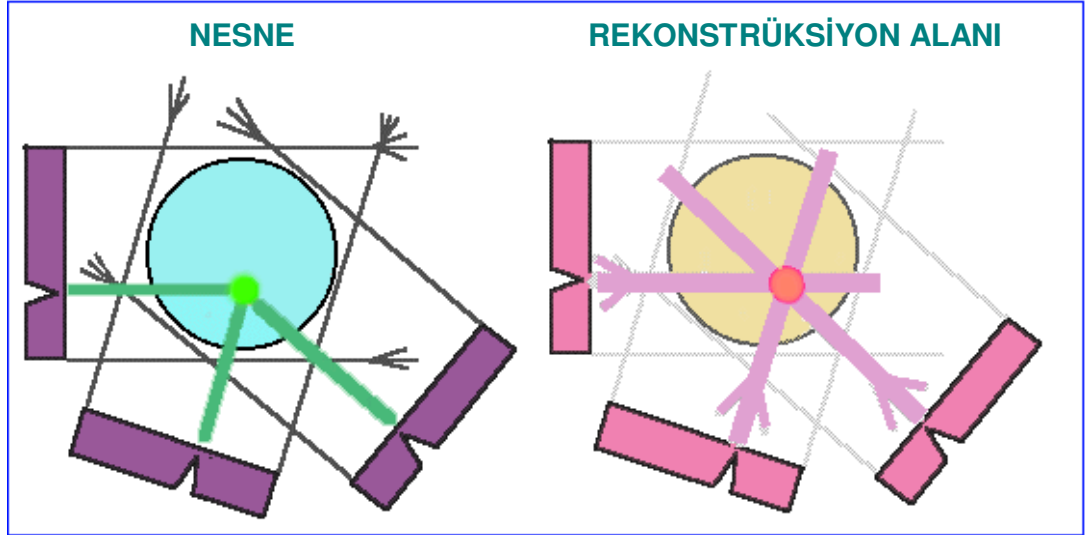
Şekil 5: µBT’de yeniden yapılandırma (SkyScan Kullanıcı kılavuzu)
