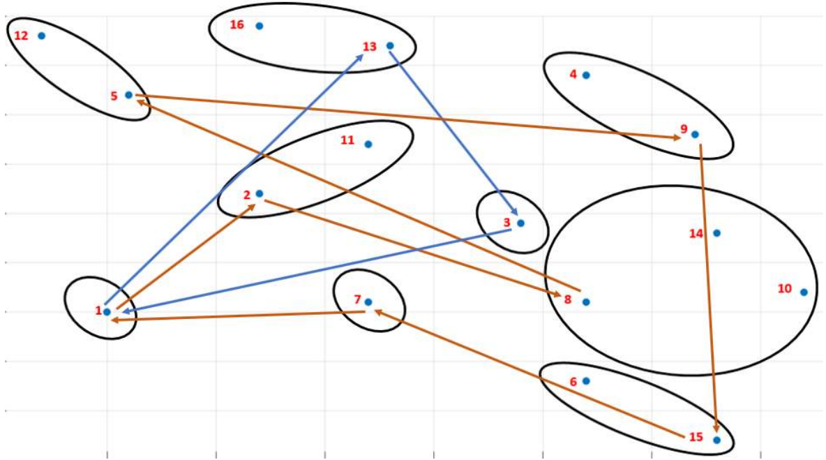
Şekil 11.2 C_AB Çözüm Örneği – İki Gezginli
