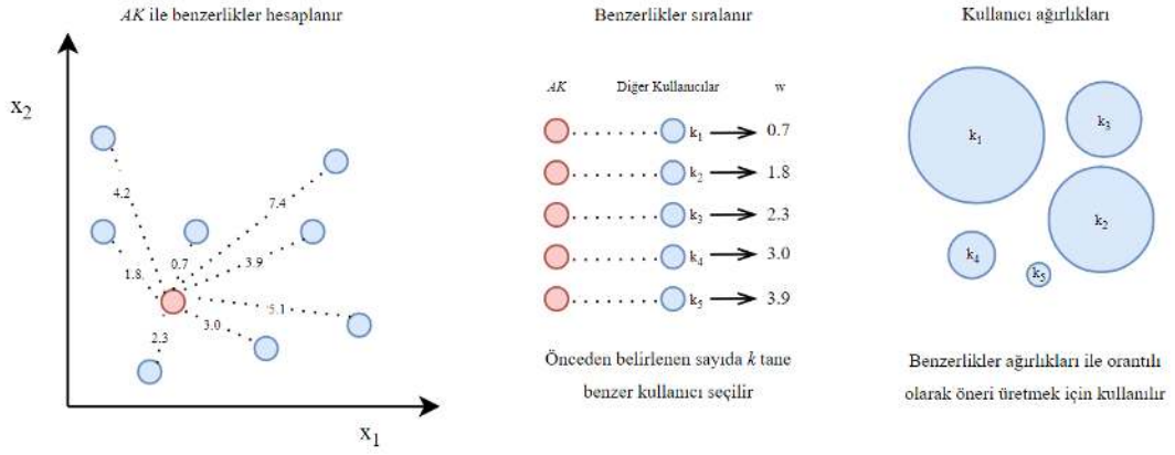
Şekil 4.2. kNN Algoritması
