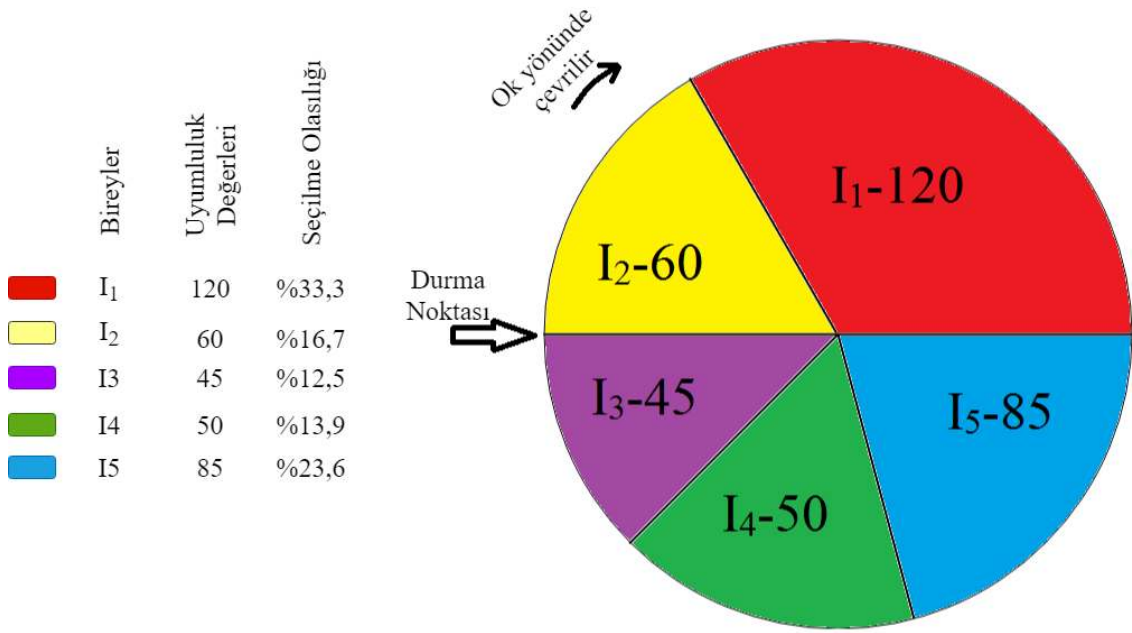
Şekil 6.4. Roulette-Wheel Algoritması
