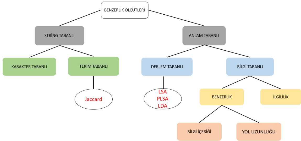
Şekil 2.2. Benzerlik ölçütleri
