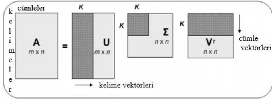
Şekil.2.4. SVD [42]
