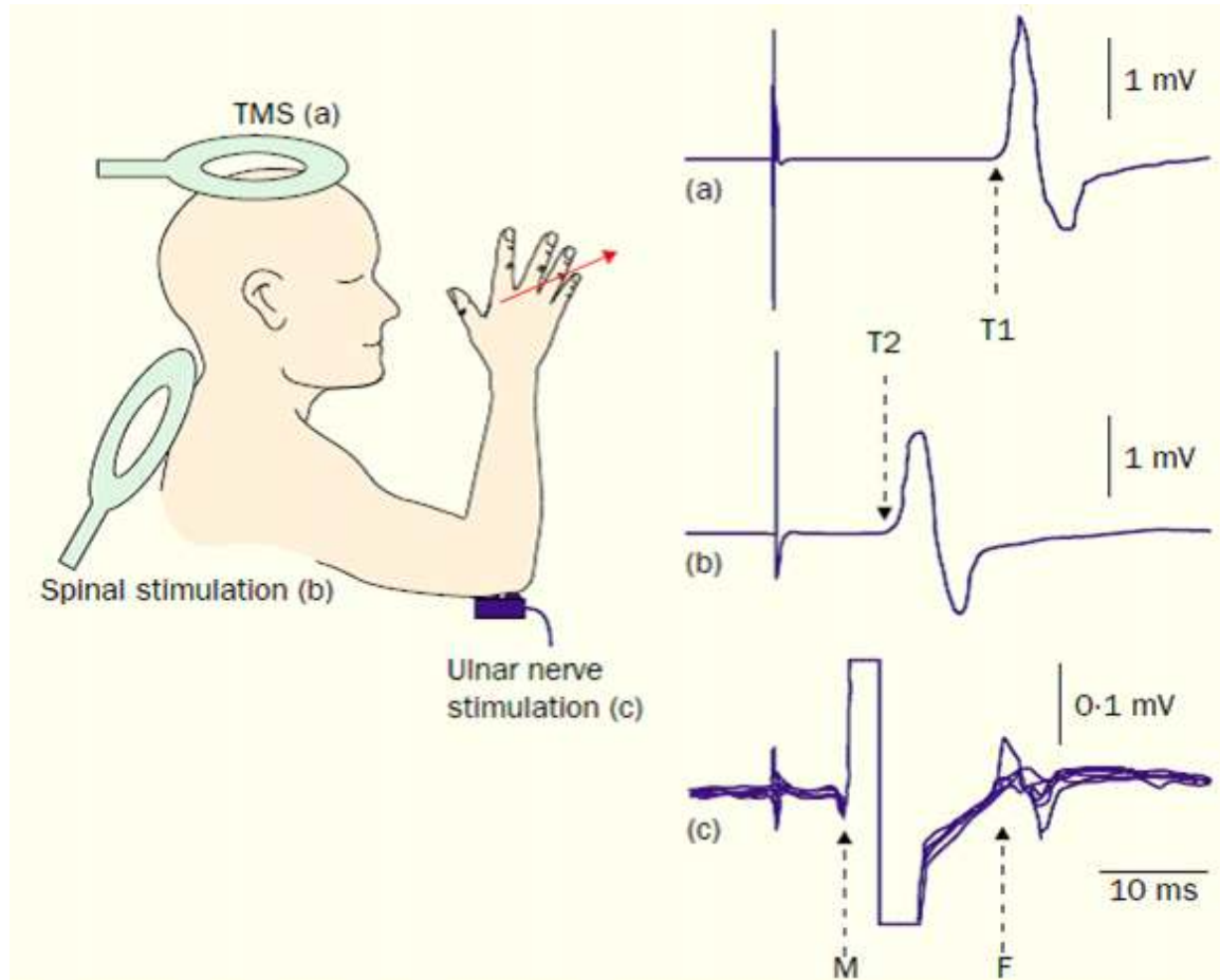
Şekil 3-2: Merkezi motor iletim zamanının (CMTC) hesaplanmasının şematik görüntüsü. (a) TMS tarafından indüklenen motor harekete geçmiş potansiyel.(b) Servikal spinal kök uyarımı sonrasında MUP (c) Ulnar sinir elektrik uyarımından sonra F-dalgaları. F dalgası gecikmesi kullanımı ile CMTC kolayca T1 - (F + M - 1) / 2 . T1= MUP başlangıç gecikmesi TMS tarafından ortaya çıkarılan; T2 cervical omurganın arkası üzerine yerleştirilen bobin tarafından ortaya çıkarılan MUP başlangıç gecikmesi M= elektrik ulnar uyarımı tarafından ortaya çıkarılan M-dalgası başlangıç gecikmesi F: elektrik ulnar uyarımı tarafından ortaya çıkarılan F-dalgası başlangıç gecikmesi olarak hesaplanabilir. Şekil referans: [A]
