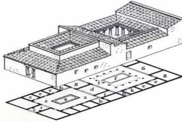
Abb. 12b. domus : 1 Fauces. 2 Atrium. 3 Peristyl. 6 Exedra. a Impluvium. b Alae. c Vestibulum. d Tablinum. e Cubicula. f Piscina. g Triclinia. h, k Nebenräume am Peristyl. j Durchgangsraum [198] 65, Abb. 77, 78.
