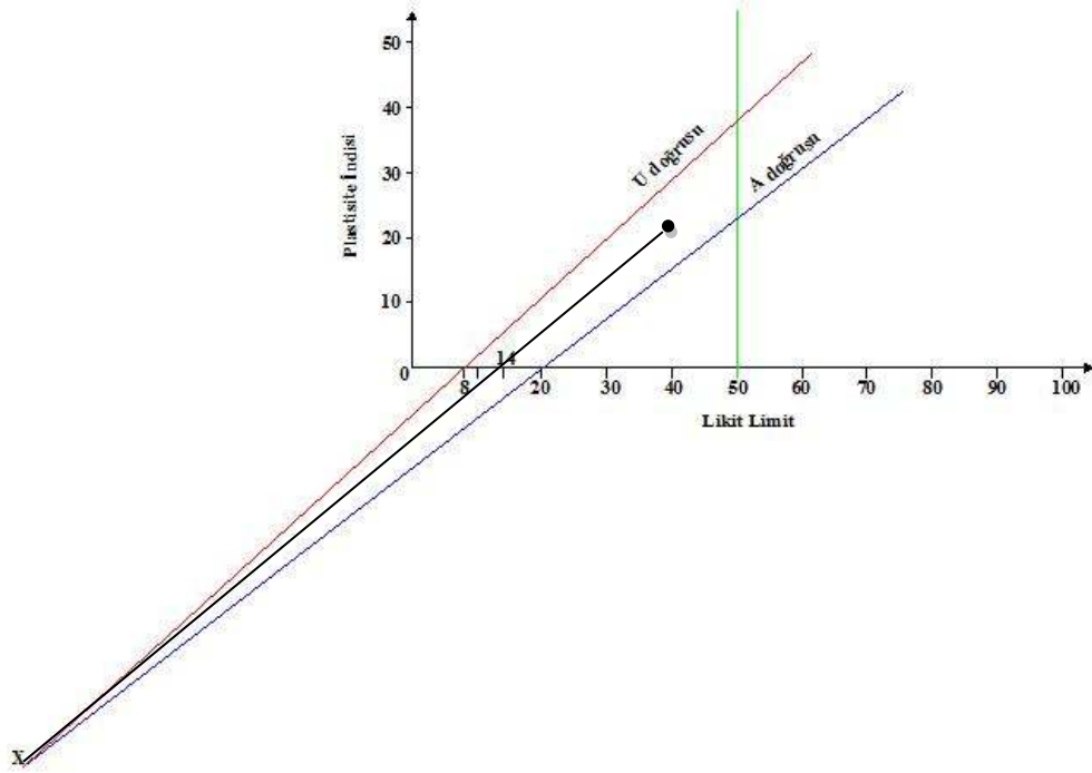
Şekil 5. Rötire limitin plastisite kartından bulunması (Önalp, A. 2002)
