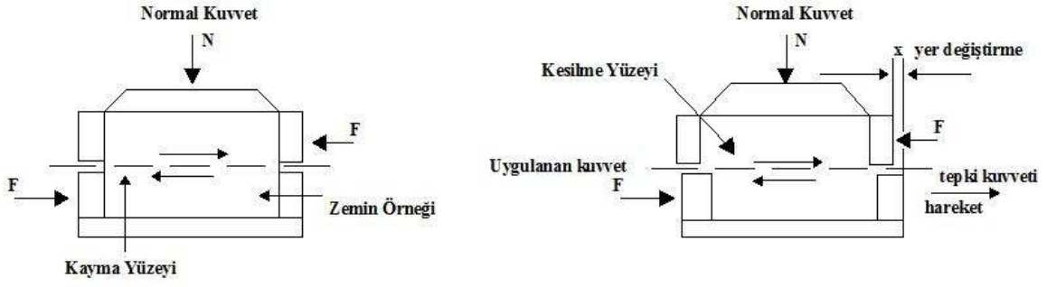
Şekil 12. Kesme kutusu deneyinin yapıma prensibi
