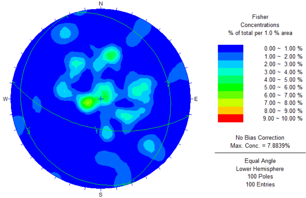
Şekil 31. Çağlayan Formasyonuna ait çatlak kontur diyagramı
