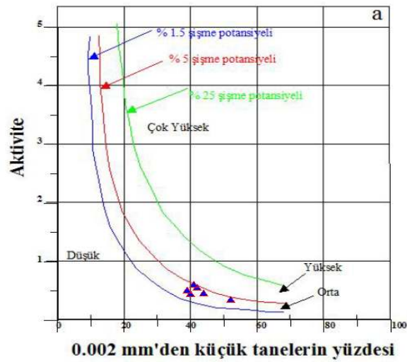
Şekil 43. Şişme potansiyeli
