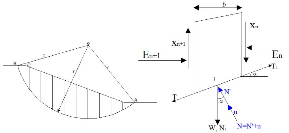
Şekil 19. Sadeleştirilmiş Janbu yönteminde bir dilime etkiyen kuvvetler
