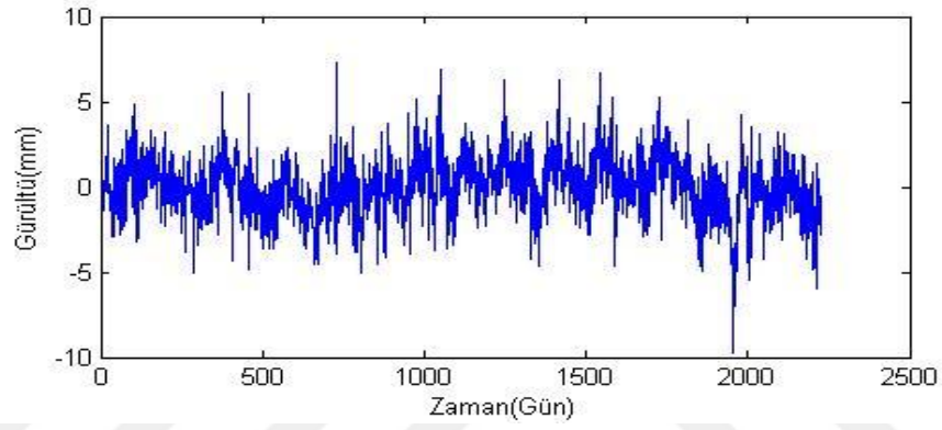
Şekil B.32. NEVS istasyonu doğu bileşeni gürültü-zaman grafiği.
