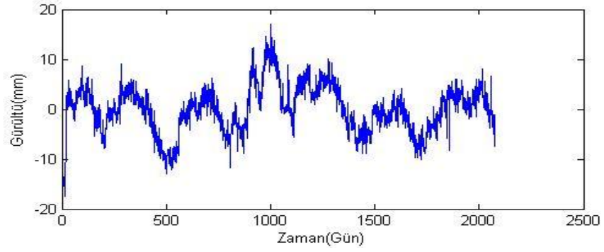
Şekil B.1. AKSI istasyonu kuzey bileşeni gürültü-zaman grafiği.
