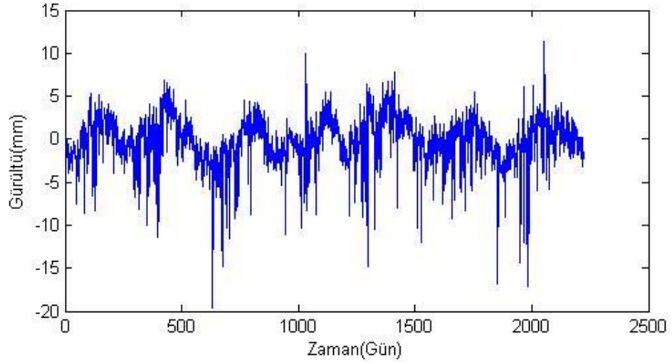
Şekil 5.6. AKHR istasyonu kuzey bileşeni gürültü-zaman grafiği.
