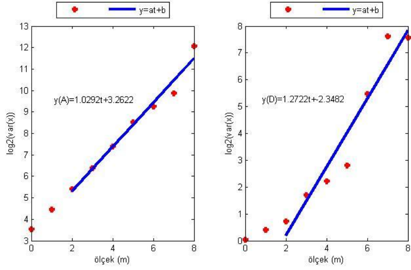
Şekil E.13. CIHA istasyonu kuzey bileşeninin Dalgacık Tabanlı Yöntem ile parametre kestiriminin ölçek boyutunda gösterimi (soldaki şekil yaklaşıklık, sağdaki şekil detay katsayılarına aittir).
