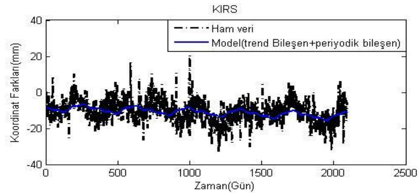
Şekil A.26. KIRS istasyonu doğu ham koordinatları ve modelden elde edilen koordinatlar.
