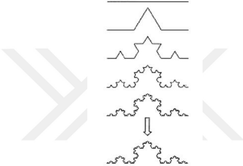
Şekil 3.7. Koch eğrisi üretimindeki adımlar (Bektaş, 2007).
