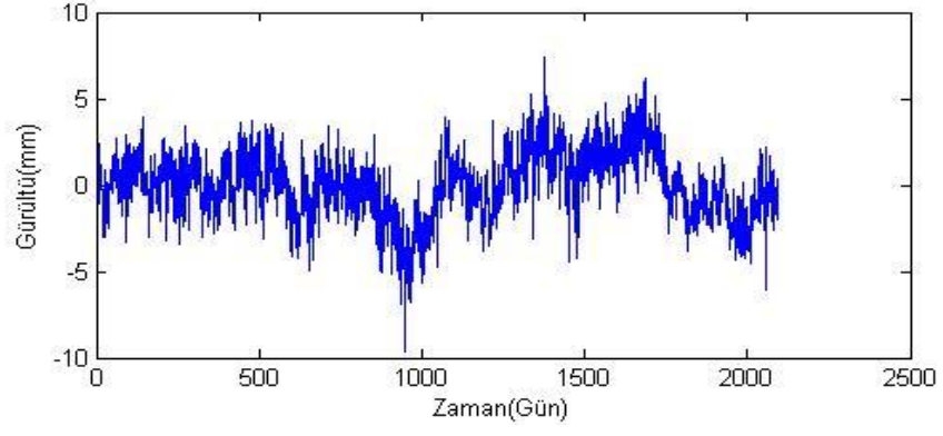
Şekil B.7. ANRK istasyonu kuzey bileşeni gürültü-zaman grafiği.
