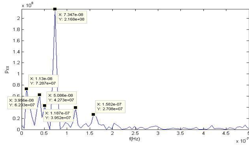
Şekil 5.10. AKHR istasyonu doğu bileşeni güç izgesi – frekans grafiği.
