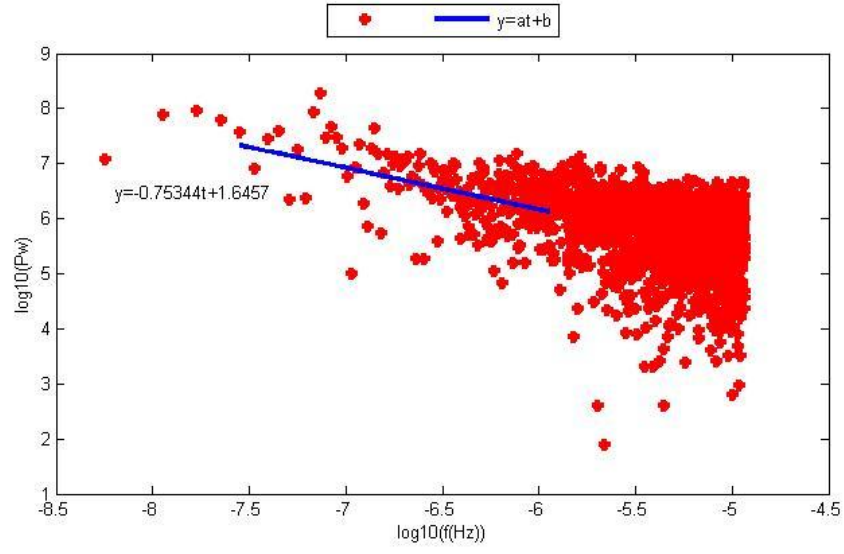
Şekil D.15. CIHA istasyonu yükseklik bileşeninin Periyodogram yöntemi ile parametre kestirim sonuçları.
