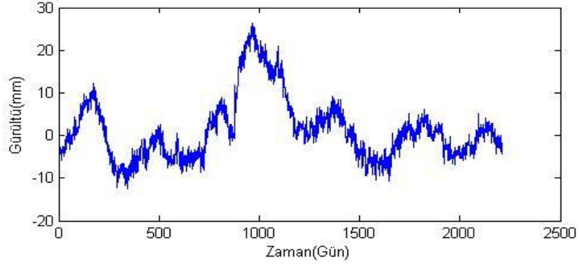
Şekil B.22. KAPN istasyonu kuzey bileşeni gürültü-zaman grafiği.
