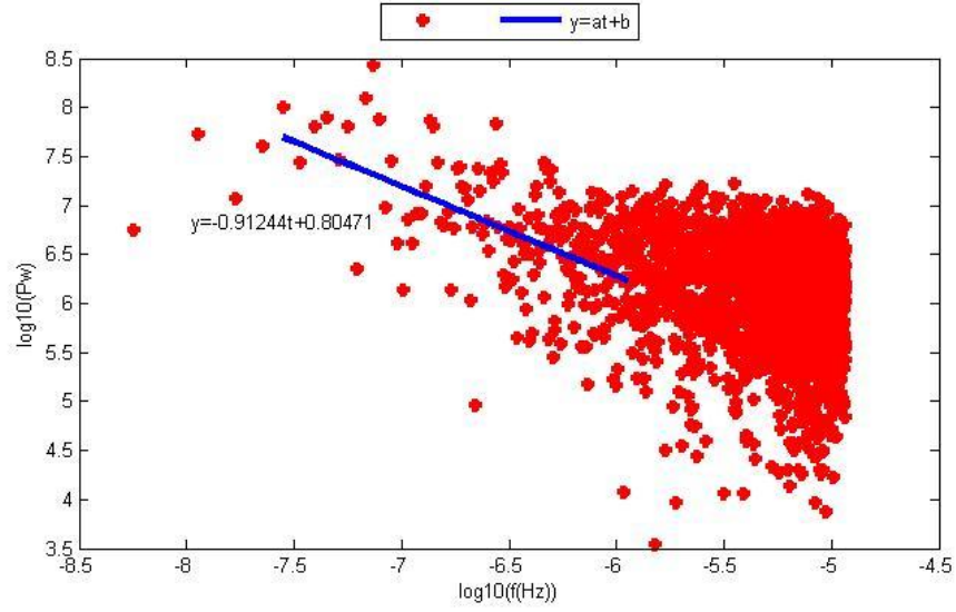
Şekil D.12. BEYS istasyonu yükseklik bileşeninin Periyodogram yöntemi ile parametre kestirim sonuçları.
