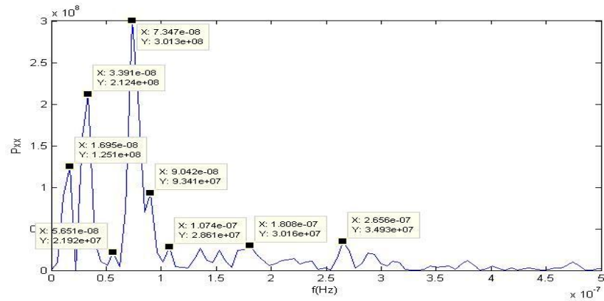
Şekil C.17. HYMN istasyonu doğu bileşeni güç izgesi – frekans grafiği.
