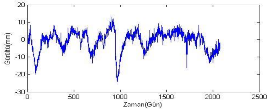
Şekil B.3. AKSI istasyonu yükseklik bileşeni gürültü-zaman grafiği.
