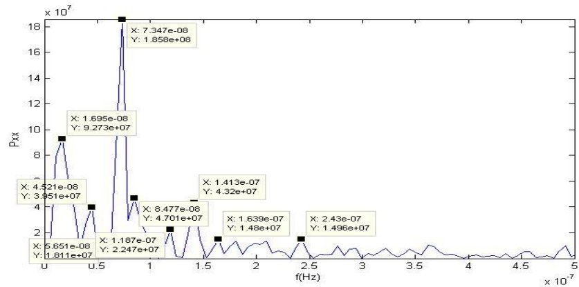
Şekil C.14. CIHA istasyonu doğu bileşeni güç izgesi – frekans grafiği.
