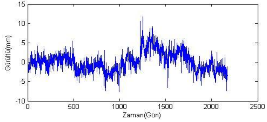
Şekil B.34. NIGD istasyonu kuzey bileşeni gürültü-zaman grafiği.
