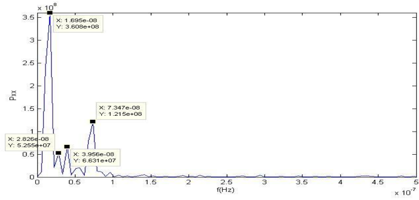
Şekil C.13. CIHA istasyonu kuzey bileşeni güç izgesi – frekans grafiği.
