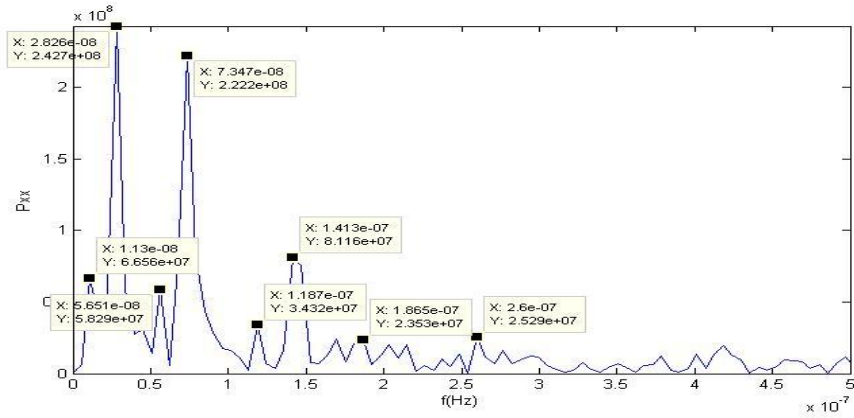
Şekil C.5. AKSR istasyonu doğu bileşeni güç izgesi – frekans grafiği.
