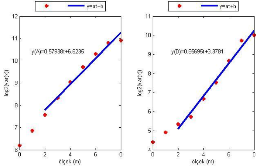
Şekil E.9. ANRK istasyonu yükseklik bileşeninin Dalgacık Tabanlı Yöntem ile parametre kestiriminin ölçek boyutunda gösterimi (soldaki şekil yaklaşıklık, sağdaki şekil detay katsayılarına aittir).
