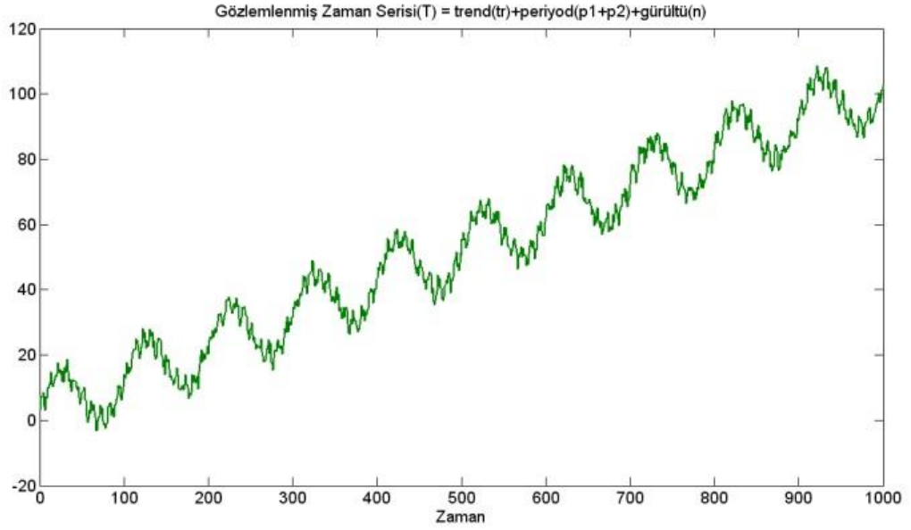
Şekil 3.2. Gözlemlenmiş bir zaman serisi (Yiğit, 2010).
