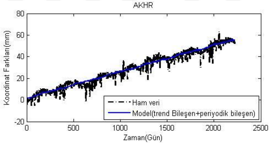
Şekil 5.2. AKHR istasyonu kuzey ham koordinatları ve modelden elde edilen koordinatlar.
