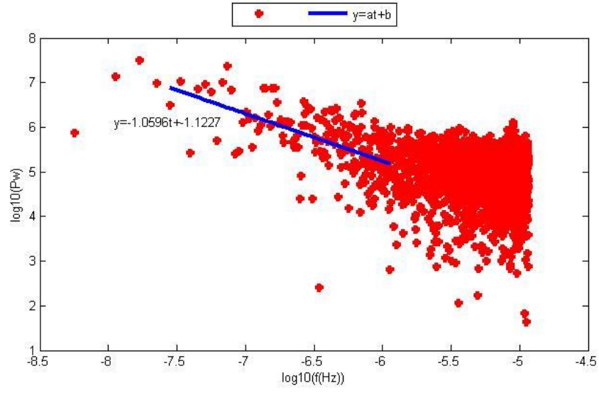
Şekil D.5. AKSR istasyonu doğu bileşeninin Periyodogram yöntemi ile parametre kestirim sonuçları.
