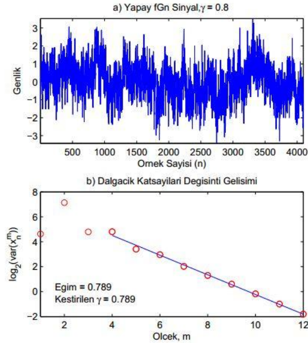
Şekil 4.3. Yapay bir fGn sinyalinin dalgacık tabanı ile kestirimi (Baykut, 2012).
