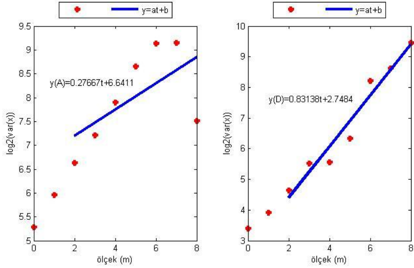
Şekil E.6. AKSR istasyonu yükseklik bileşeninin Dalgacık Tabanlı Yöntem ile parametre kestiriminin ölçek boyutunda gösterimi (soldaki şekil yaklaşıklık, sağdaki şekil detay katsayılarına aittir).
