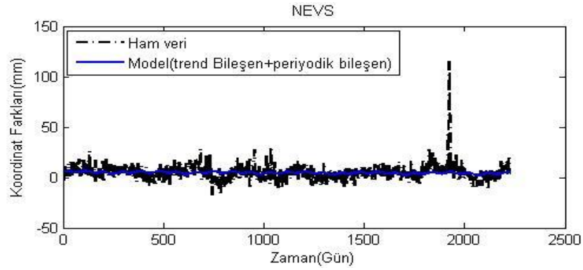
Şekil A.32. NEVS istasyonu doğu ham koordinatları ve modelden elde edilen koordinatlar.
