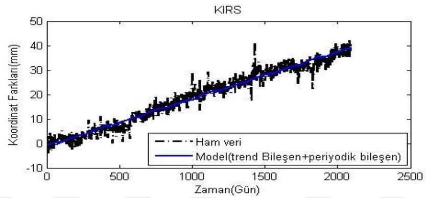
Şekil A.25. KIRS istasyonu kuzey ham koordinatları ve modelden elde edilen koordinatlar.
