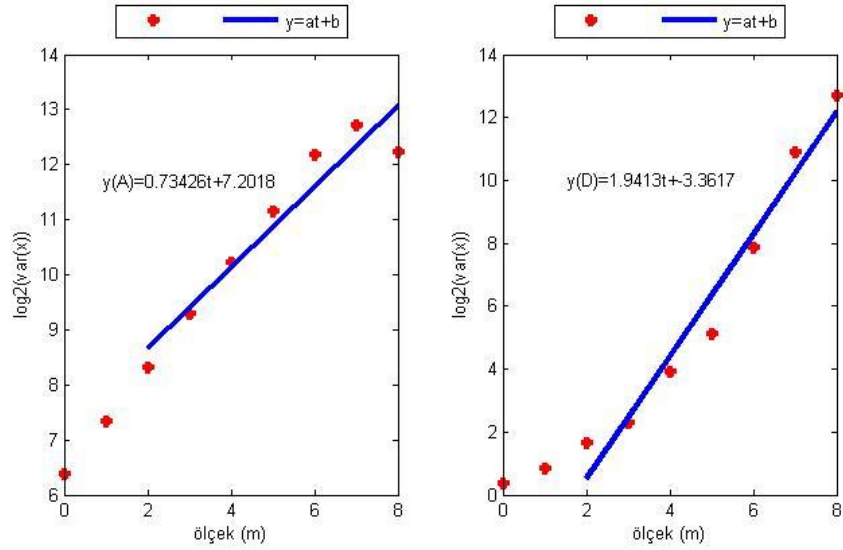
Şekil E.22. KAPN istasyonu kuzey bileşeninin Dalgacık Tabanlı Yöntem ile parametre kestiriminin ölçek boyutunda gösterimi (soldaki şekil yaklaşıklık, sağdaki şekil detay katsayılarına aittir).
