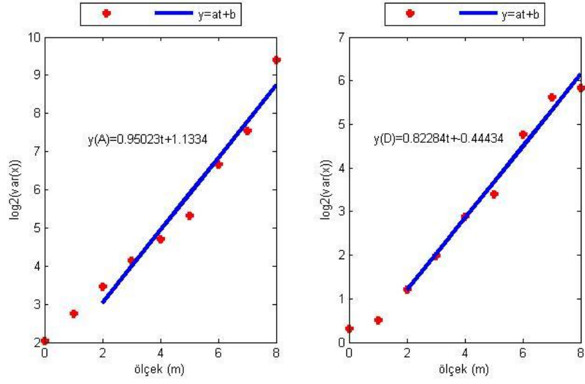
Şekil E.31. NEVS istasyonu kuzey bileşeninin Dalgacık Tabanlı Yöntem ile parametre kestiriminin ölçek boyutunda gösterimi (soldaki şekil yaklaşıklık, sağdaki şekil detay katsayılarına aittir).
