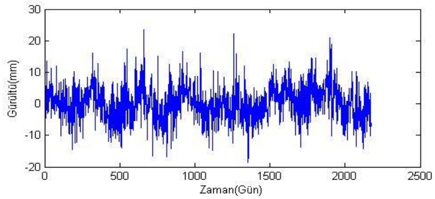
Şekil B.36. NIGD istasyonu kuzey bileşeni gürültü-zaman grafiği.
