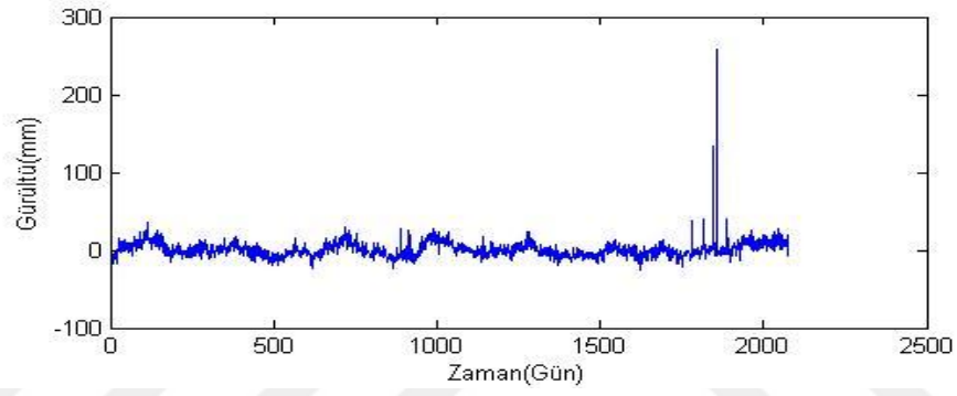
Şekil B.1. AKSI istasyonu kuzey bileşeni gürültü-zaman grafiği.
