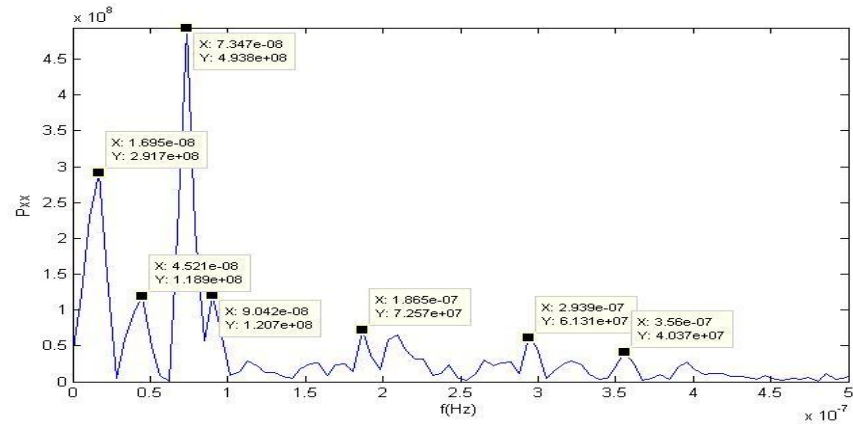
Şekil C.11. BEYS istasyonu doğu bileşeni güç izgesi – frekans grafiği.
