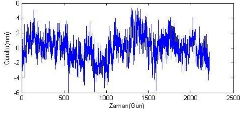
Şekil B.4. AKSR istasyonu kuzey bileşeni gürültü-zaman grafiği.
