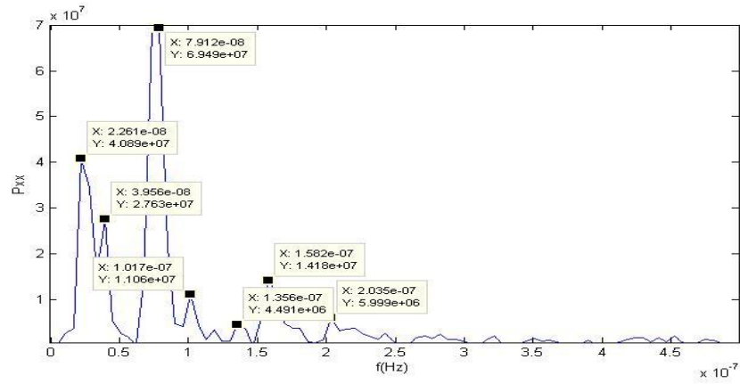
Şekil C.28. KLUU istasyonu kuzey bileşeni güç izgesi – frekans grafiği.
