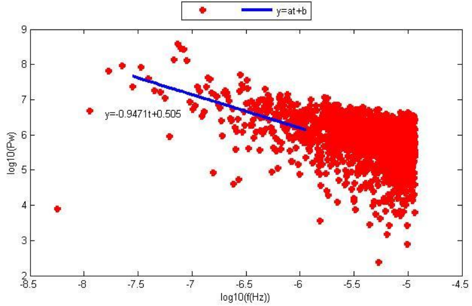
Şekil D.30. KLUU istasyonu yükseklik bileşeninin Periyodogram yöntemi ile parametre kestirim sonuçları.
