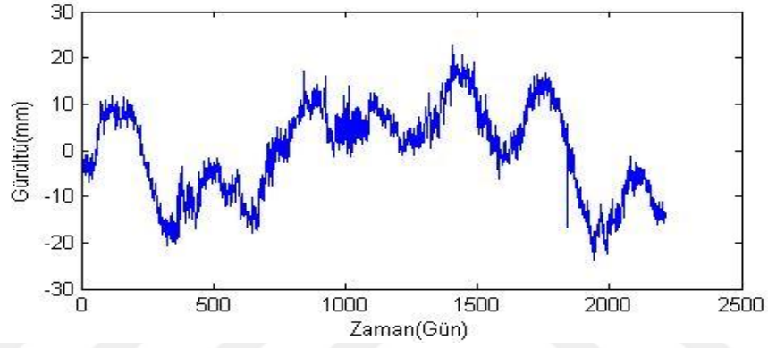
Şekil B.23. KAPN istasyonu doğu bileşeni gürültü-zaman grafiği.
