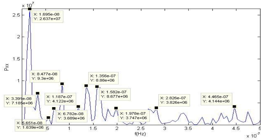
Şekil C.32. NEVS istasyonu doğu bileşeni güç izgesi – frekans grafiği.
