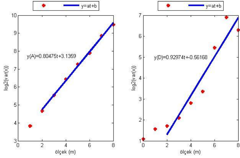
Şekil E.11. BEYS istasyonu doğu bileşeninin Dalgacık Tabanlı Yöntem ile parametre kestiriminin ölçek boyutunda gösterimi (soldaki şekil yaklaşıklık, sağdaki şekil detay katsayılarına aittir).
