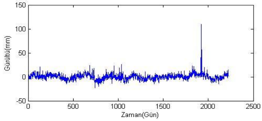
Şekil B.33. NEVS istasyonu yükseklik bileşeni gürültü-zaman grafiği.
