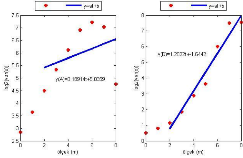
Şekil E.29. KLUU istasyonu doğu bileşeninin Dalgacık Tabanlı Yöntem ile parametre kestiriminin ölçek boyutunda gösterimi (soldaki şekil yaklaşıklık, sağdaki şekil detay katsayılarına aittir).
