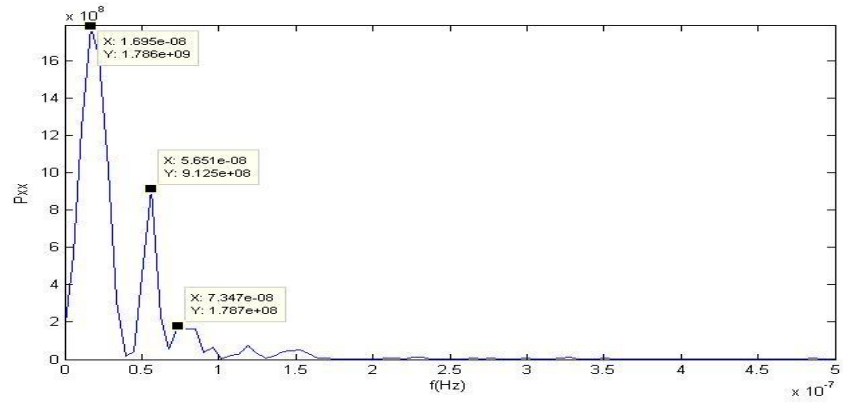
Şekil C.22. KAPN istasyonu kuzey bileşeni güç izgesi – frekans grafiği.
