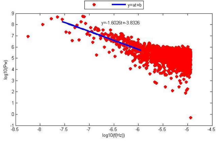
Şekil D.1. AKSI istasyonu kuzey bileşeninin Periyodogram yöntemi ile parametre kestirim sonuçları.
