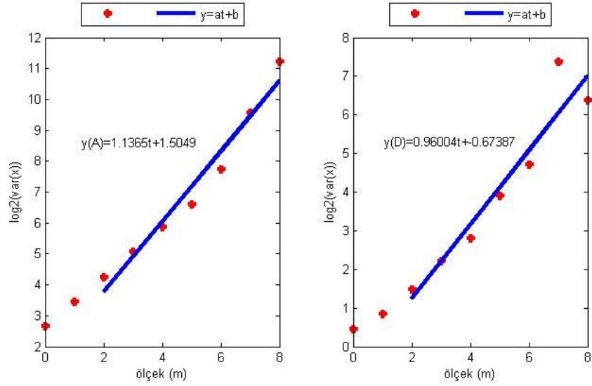
Şekil E.16. HYMN istasyonu kuzey bileşeninin Dalgacık Tabanlı Yöntem ile parametre kestiriminin ölçek boyutunda gösterimi (soldaki şekil yaklaşıklık, sağdaki şekil detay katsayılarına aittir).
