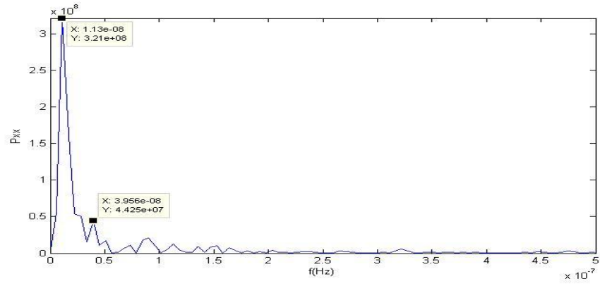
Şekil C.28. KLUU istasyonu kuzey bileşeni güç izgesi – frekans grafiği.
