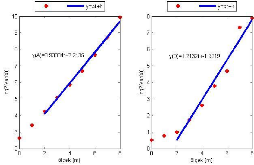
Şekil E.34. NIGD istasyonu kuzey bileşeninin Dalgacık Tabanlı Yöntem ile parametre kestiriminin ölçek boyutunda gösterimi (soldaki şekil yaklaşıklık, sağdaki şekil detay katsayılarına aittir).
