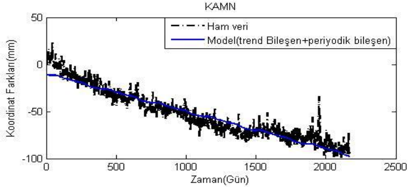
Şekil A.20. KAMN istasyonu kuzey ham koordinatları ve modelden elde edilen koordinatlar.
