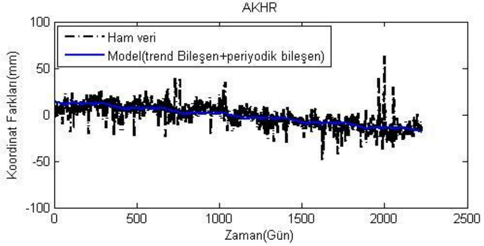
Şekil 5.4. AKHR istasyonu yükseklik ham koordinatları ve modelden elde edilen koordinatlar.
