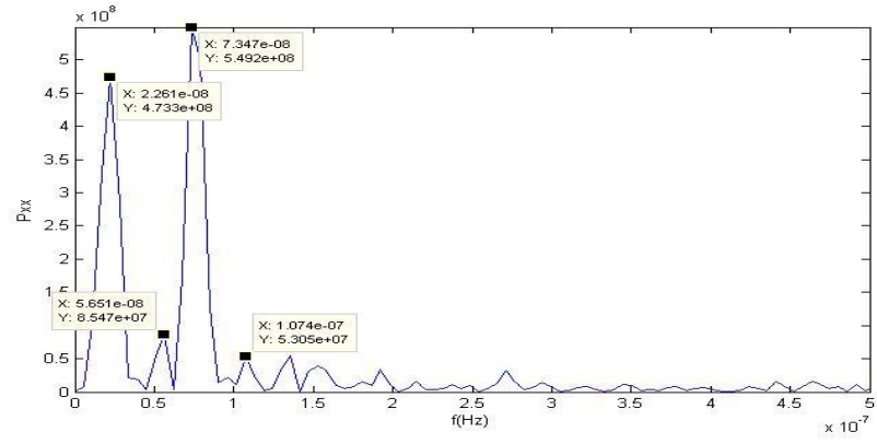
Şekil C.1. AKSI istasyonu kuzey bileşeni güç izgesi – frekans grafiği.
