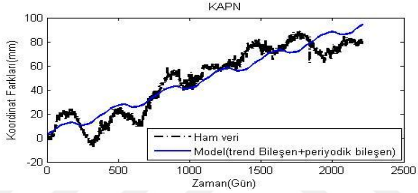
Şekil A.22. KAPN istasyonu kuzey ham koordinatları ve modelden elde edilen koordinatlar.
