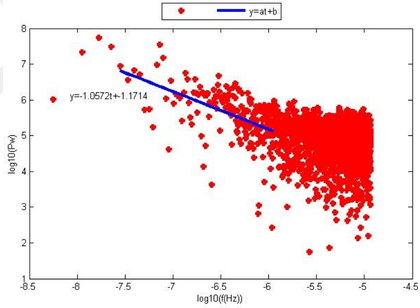
Şekil D.4. AKSR istasyonu kuzey bileşeninin Periyodogram yöntemi ile parametre kestirim sonuçları.
