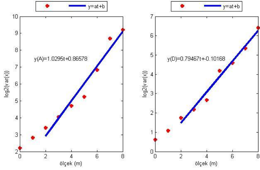
Şekil E.17. HYMN istasyonu doğu bileşeninin Dalgacık Tabanlı Yöntem ile parametre kestiriminin ölçek boyutunda gösterimi (soldaki şekil yaklaşıklık, sağdaki şekil detay katsayılarına aittir).
