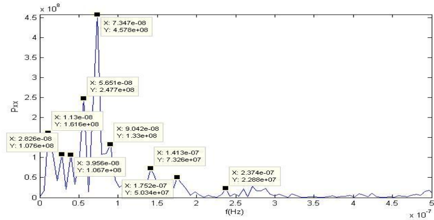
Şekil C.33. NEVS istasyonu yükseklik bileşeni güç izgesi – frekans grafiği.
