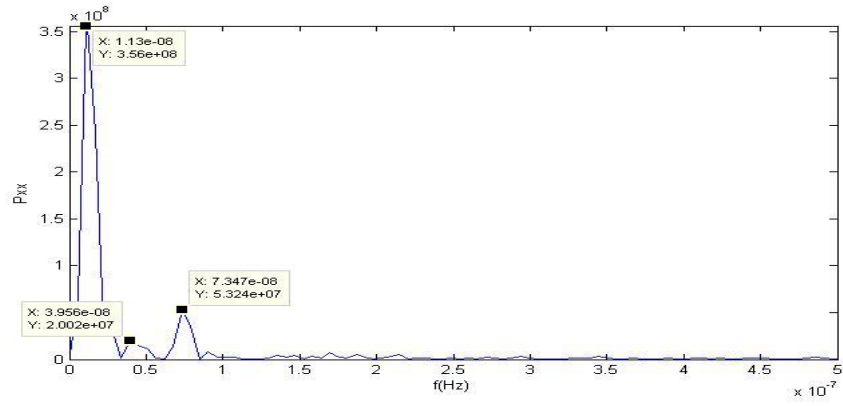
Şekil C.25. KIRS istasyonu kuzey bileşeni güç izgesi – frekans grafiği.
