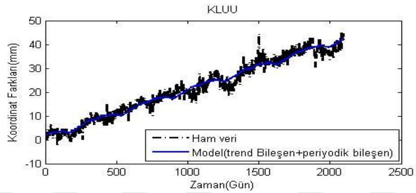
Şekil A.28. KLUU istasyonu kuzey ham koordinatları ve modelden elde edilen koordinatlar.
