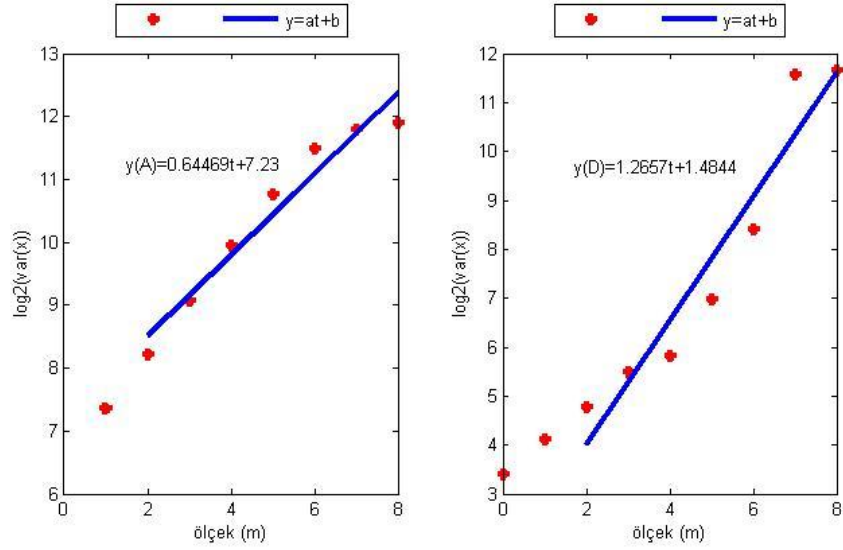
Şekil E.24. KAPN istasyonu yükseklik bileşeninin Dalgacık Tabanlı Yöntem ile parametre kestiriminin ölçek boyutunda gösterimi (soldaki şekil yaklaşıklık, sağdaki şekil detay katsayılarına aittir).
