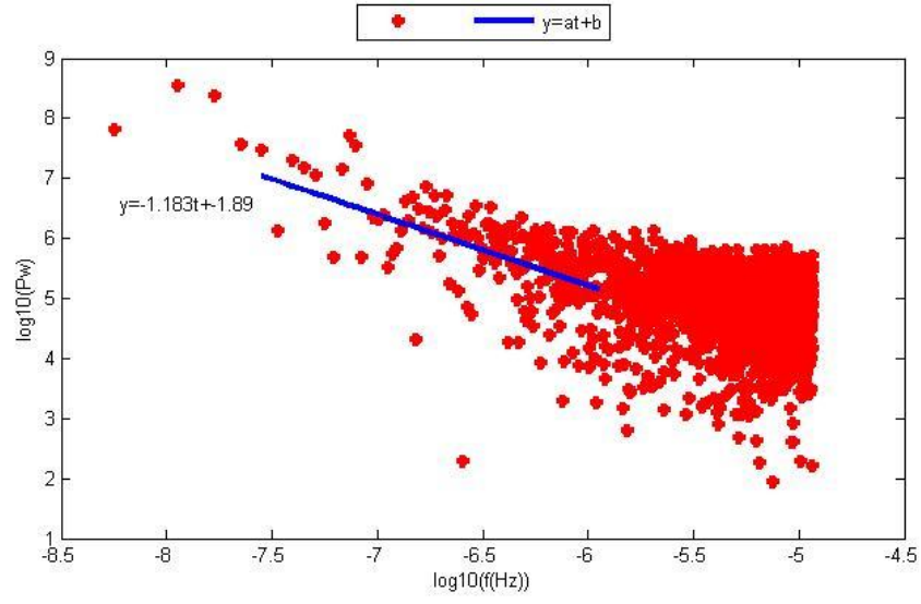
Şekil D.25. KIRS istasyonu kuzey bileşeninin Periyodogram yöntemi ile parametre kestirim sonuçları.
