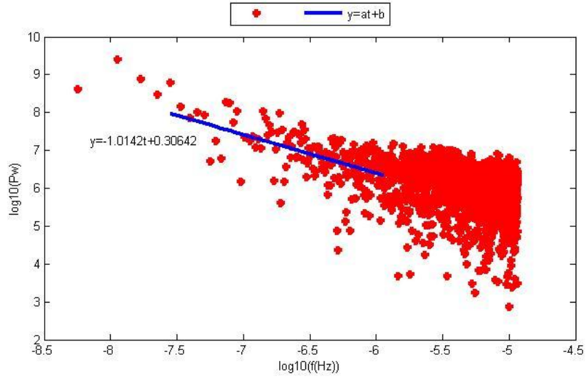
Şekil D.21. KAMN istasyonu yükseklik bileşeninin Periyodogram yöntemi ile parametre kestirim sonuçları.
