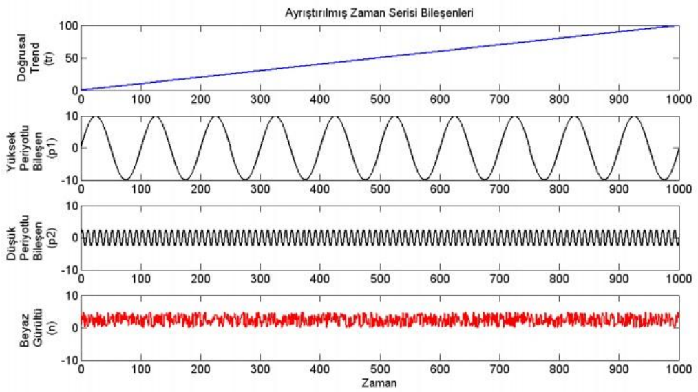
Şekil 3.3. Ayrıştırılmış zaman serisi bileşenleri (Yiğit, 2010).
