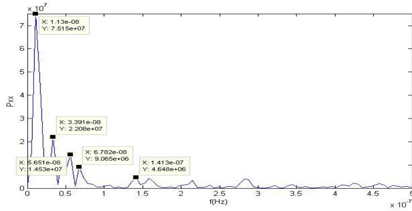
Şekil C.13. CIHA istasyonu kuzey bileşeni güç izgesi – frekans grafiği.
