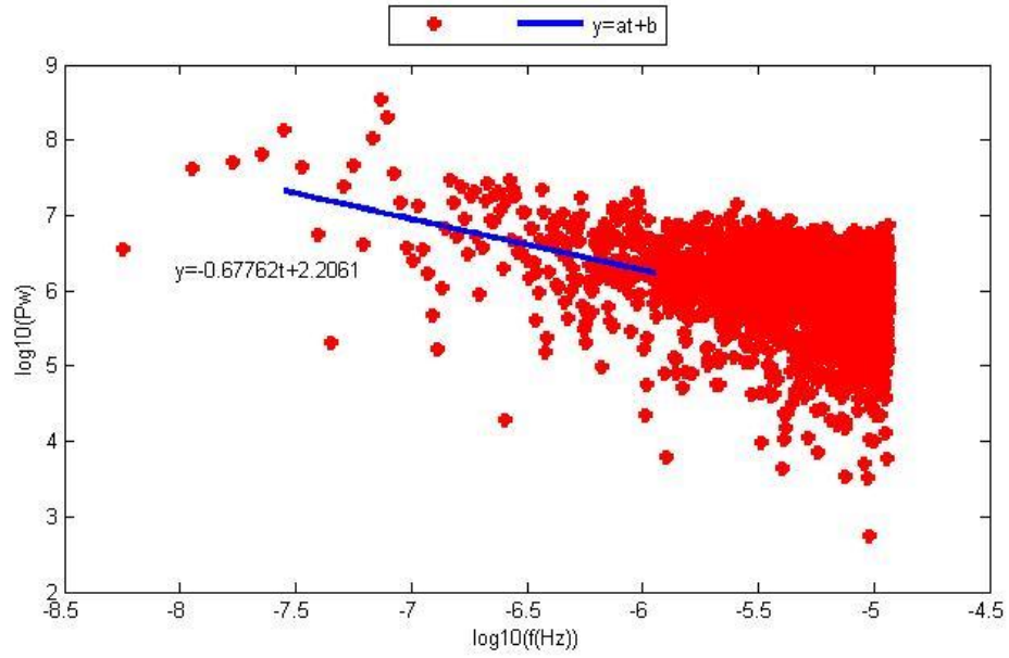
Şekil D.36. NIGD istasyonu yükseklik bileşeninin Periyodogram yöntemi ile parametre kestirim sonuçları.
