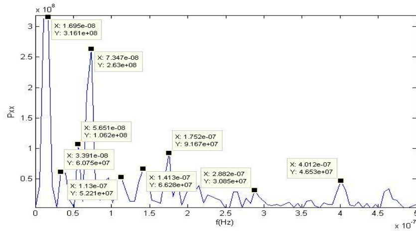
Şekil 5.11. AKHR istasyonu yükseklik bileşeni güç izgesi – frekans grafiği.
