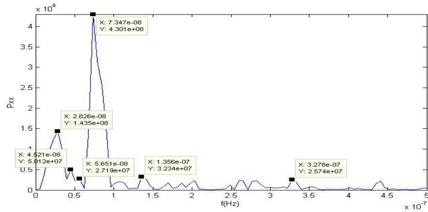
Şekil C.26. KIRS istasyonu doğu bileşeni güç izgesi – frekans grafiği.
