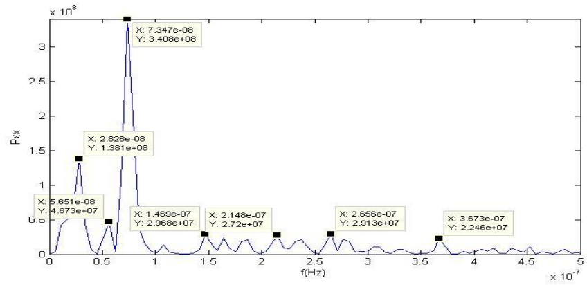
Şekil C.35. NIGD istasyonu doğu bileşeni güç izgesi – frekans grafiği.
