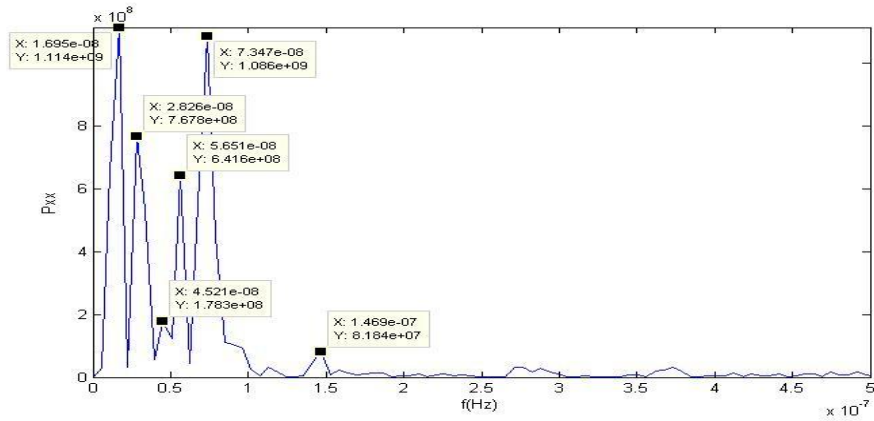
Şekil C.23. KAPN istasyonu doğu bileşeni güç izgesi – frekans grafiği.
