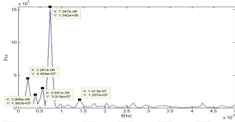
Şekil 5.9. AKHR istasyonu kuzey bileşeni güç izgesi – frekans grafiği.
