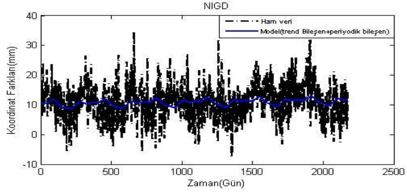
Şekil A.35. NIGD istasyonu kuzey ham koordinatları ve modelden elde edilen koordinatlar.
