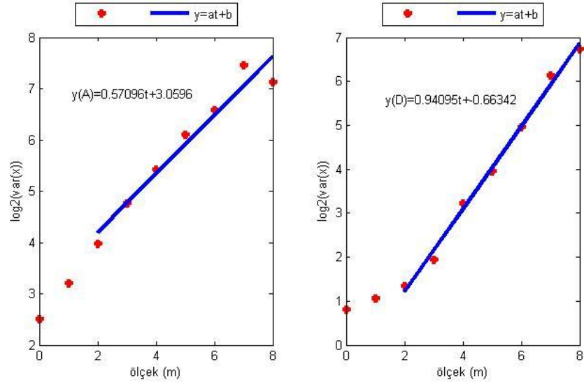
Şekil E.35. NIGD istasyonu doğu bileşeninin Dalgacık Tabanlı Yöntem ile parametre kestiriminin ölçek boyutunda gösterimi (soldaki şekil yaklaşıklık, sağdaki şekil detay katsayılarına aittir).
