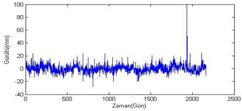
Şekil B.12. BEYS istasyonu yükseklik bileşeni gürültü-zaman grafiği.
