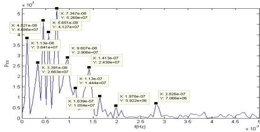
Şekil C.19. KAMN istasyonu kuzey bileşeni güç izgesi – frekans grafiği.
