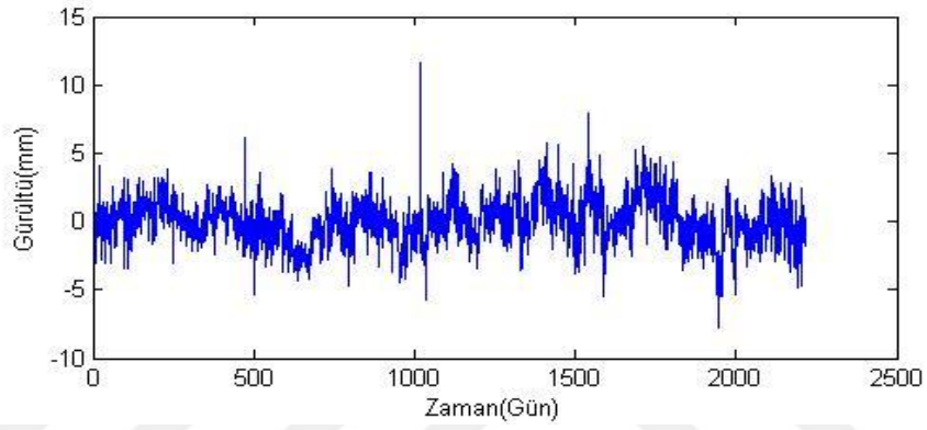
Şekil B.5. AKSR istasyonu doğu bileşeni gürültü-zaman grafiği.
