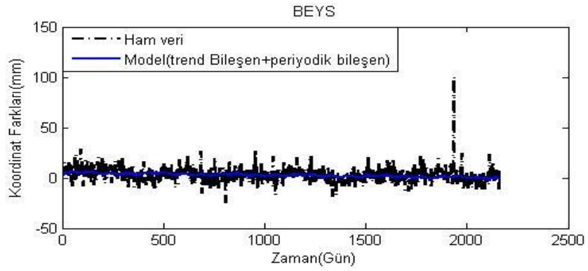
Şekil A.12. BEYS istasyonu yükseklik ham koordinatları ve modelden elde edilen koordinatlar.
