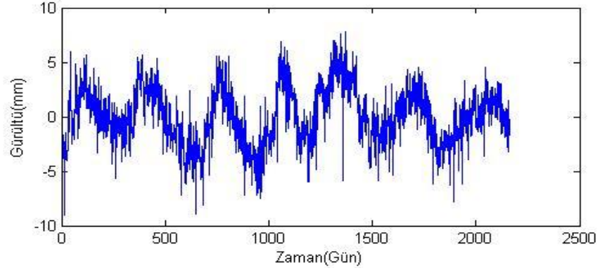
Şekil B.10. BEYS istasyonu kuzey bileşeni gürültü-zaman grafiği.
