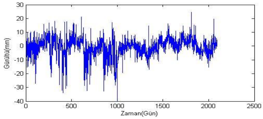
Şekil B.9. ANRK istasyonu yükseklik bileşeni gürültü-zaman grafiği.
