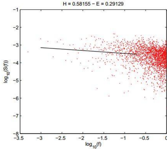
Şekil 4.1. Bir fGn sinyalin periyodogram ile kestirim sonuçları (Baykut, 2012).
