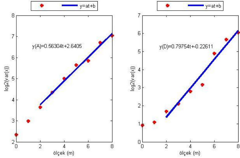
Şekil E.26. KIRS istasyonu doğu bileşeninin Dalgacık Tabanlı Yöntem ile parametre kestiriminin ölçek boyutunda gösterimi (soldaki şekil yaklaşıklık, sağdaki şekil detay katsayılarına aittir).
