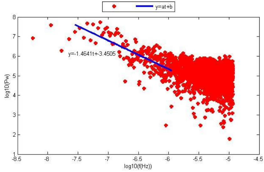
Şekil D.20. KAMN istasyonu doğu bileşeninin Periyodogram yöntemi ile parametre kestirim sonuçları.
