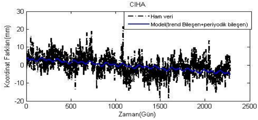
Şekil A.14. CIHA istasyonu kuzey ham koordinatları ve modelden elde edilen koordinatlar.
