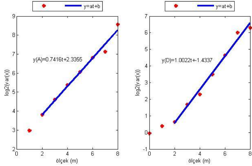
Şekil E.4. AKSR istasyonu kuzey bileşeninin Dalgacık Tabanlı Yöntem ile parametre kestiriminin ölçek boyutunda gösterimi (soldaki şekil yaklaşıklık, sağdaki şekil detay katsayılarına aittir).
