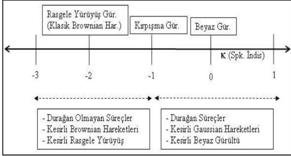
Şekil 3.6. Gürültü çeşitlerinin spektral indis eksenindeki konumları (Kurt, 2009).
