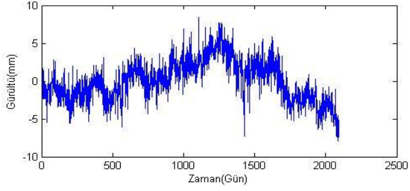
Şekil B.25. KIRS istasyonu kuzey bileşeni gürültü-zaman grafiği.
