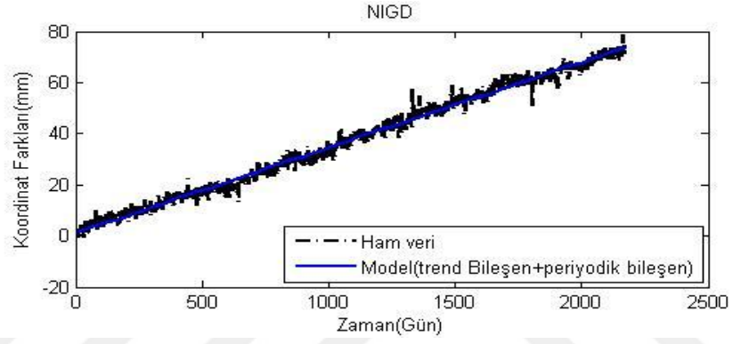
Şekil A.34. NIGD istasyonu kuzey ham koordinatları ve modelden elde edilen koordinatlar.
