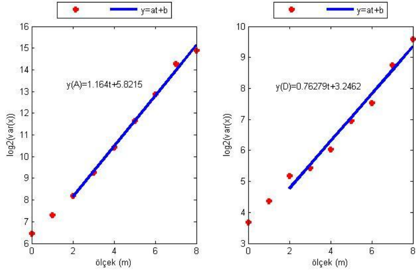
Şekil E.21. KAMN istasyonu yükseklik bileşeninin Dalgacık Tabanlı Yöntem ile parametre kestiriminin ölçek boyutunda gösterimi (soldaki şekil yaklaşıklık, sağdaki şekil detay katsayılarına aittir).
