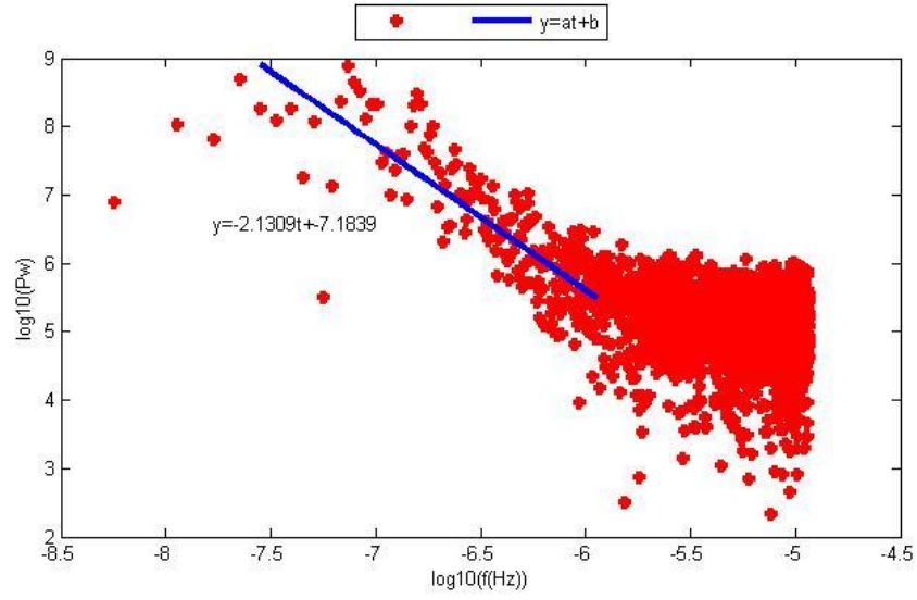
Şekil D.2. AKSI istasyonu doğu bileşeninin Periyodogram yöntemi ile parametre kestirim sonuçları.
