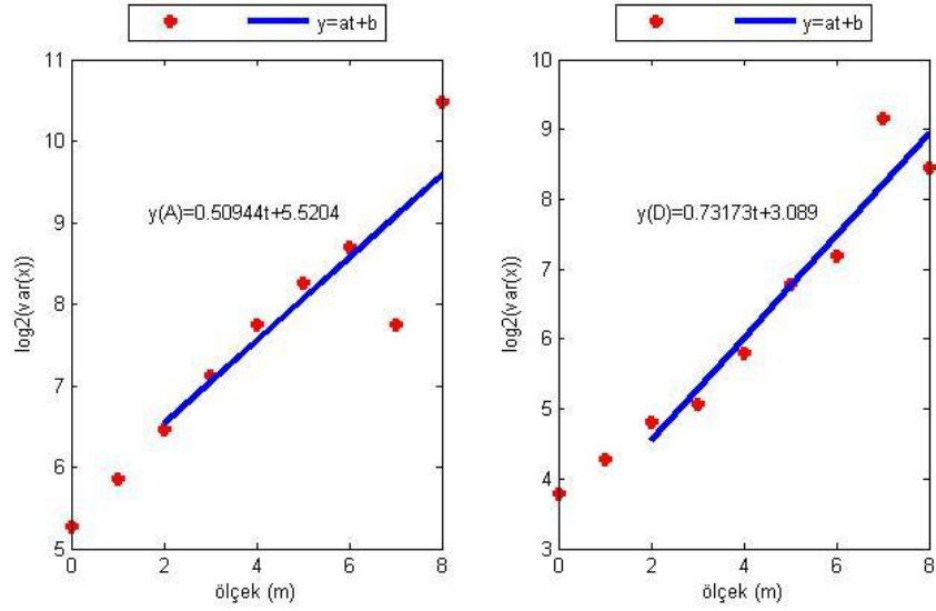
Şekil E.36. NIGD istasyonu yükseklik bileşeninin Dalgacık Tabanlı Yöntem ile parametre kestiriminin ölçek boyutunda gösterimi (soldaki şekil yaklaşıklık, sağdaki şekil detay katsayılarına aittir).
