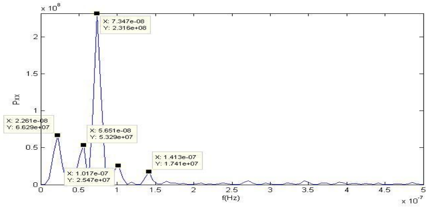
Şekil C.10. BEYS istasyonu kuzey bileşeni güç izgesi – frekans grafiği.
