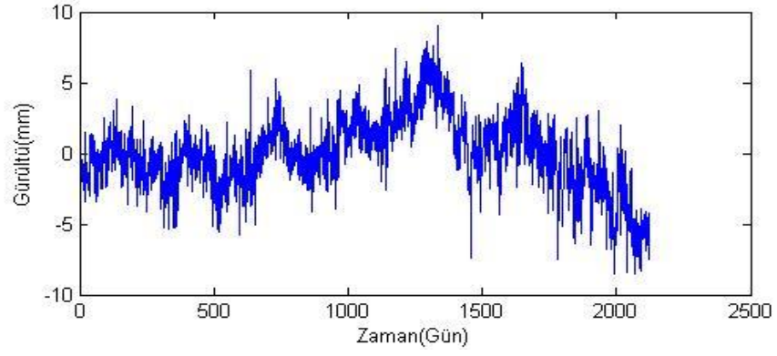
Şekil B.16. HYMN istasyonu kuzey bileşeni gürültü-zaman grafiği.
