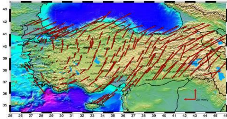
Şekil 5.5. TUSAGA-Aktif nokta hızları (ITRF) (Cingöz vd., 2013).
