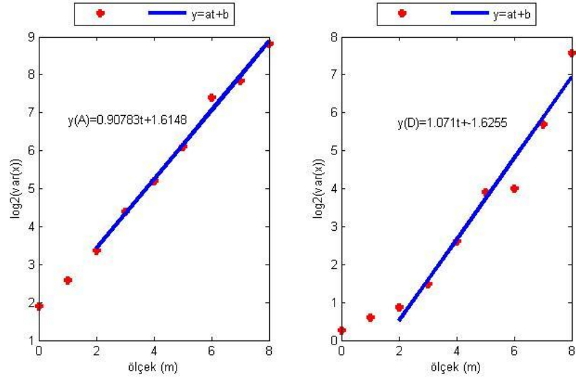
Şekil E.14. CIHA istasyonu doğu bileşeninin Dalgacık Tabanlı Yöntem ile parametre kestiriminin ölçek boyutunda gösterimi (soldaki şekil yaklaşıklık, sağdaki şekil detay katsayılarına aittir).
