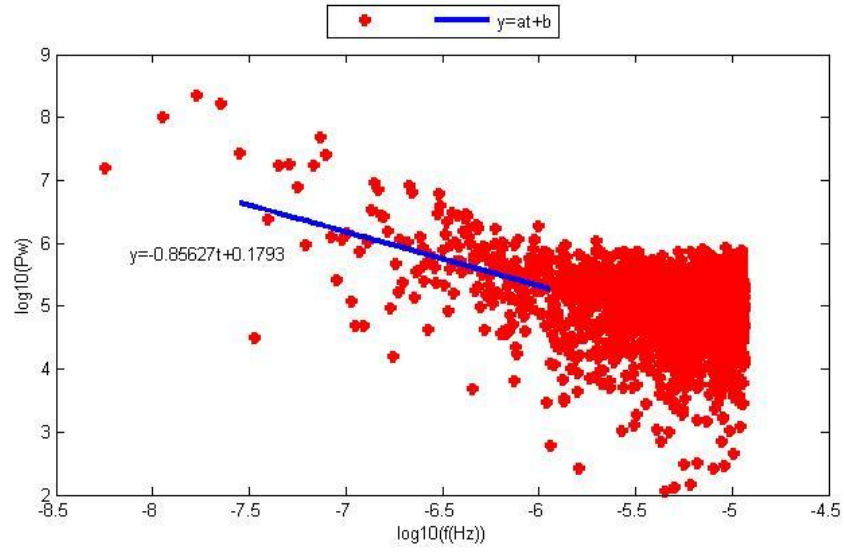
Şekil D.34. NIGD istasyonu kuzey bileşeninin Periyodogram yöntemi ile parametre kestirim sonuçları.
