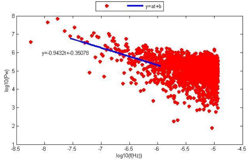
Şekil D.26. KIRS istasyonu doğu bileşeninin Periyodogram yöntemi ile parametre kestirim sonuçları.
