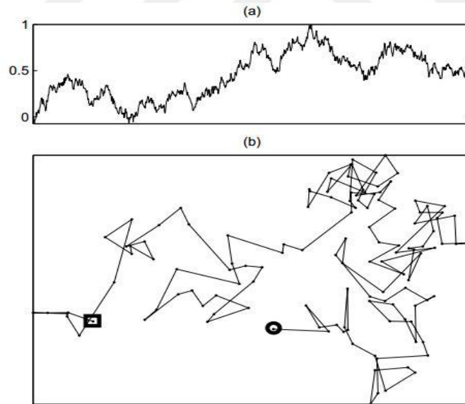
Şekil 3.9. (a) Bir boyutlu, (b) İki boyutlu Brown hareketleri (Baykut, 2012).
