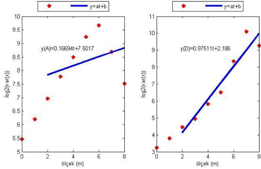
Şekil E.30. KLUU istasyonu yükseklik bileşeninin Dalgacık Tabanlı Yöntem ile parametre kestiriminin ölçek boyutunda gösterimi (soldaki şekil yaklaşıklık, sağdaki şekil detay katsayılarına aittir).
