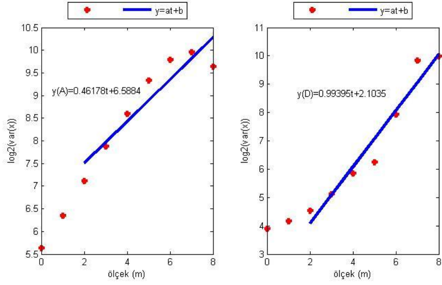
Şekil E.27. KIRS istasyonu yükseklik bileşeninin Dalgacık Tabanlı Yöntem ile parametre kestiriminin ölçek boyutunda gösterimi (soldaki şekil yaklaşıklık, sağdaki şekil detay katsayılarına aittir).
