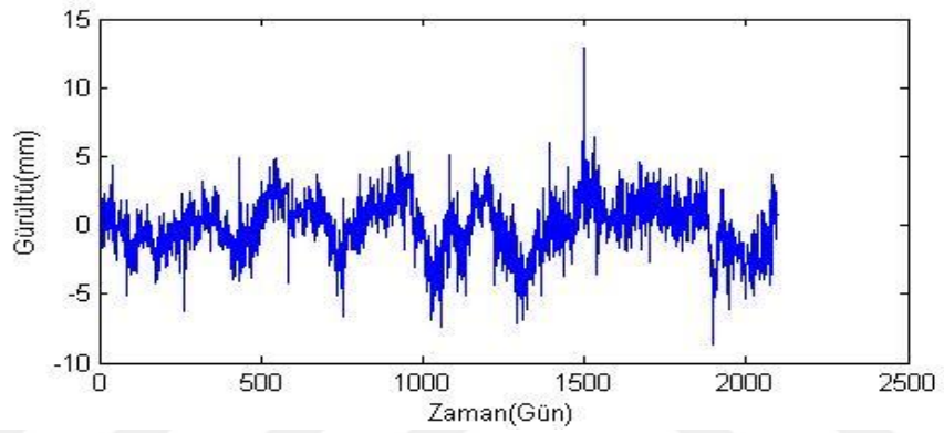
Şekil B.28. KLUU istasyonu kuzey bileşeni gürültü-zaman grafiği.
