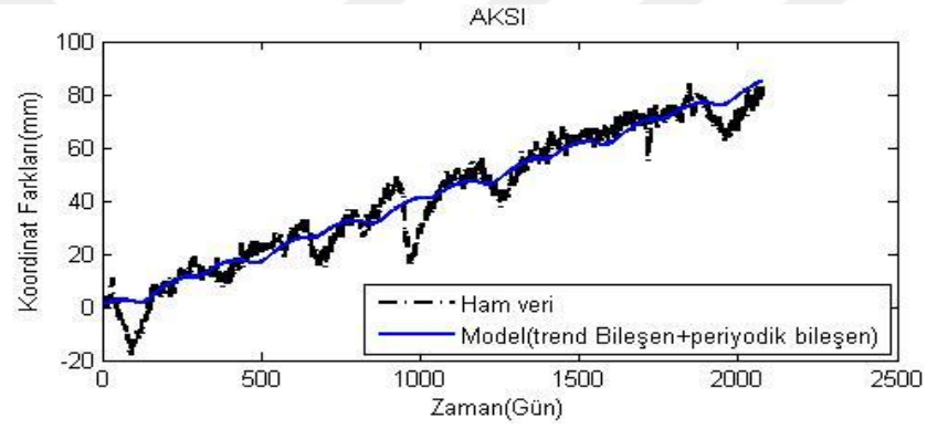
Şekil A.2. AKSI istasyonu doğu ham koordinatları ve modelden elde edilen koordinatlar.
