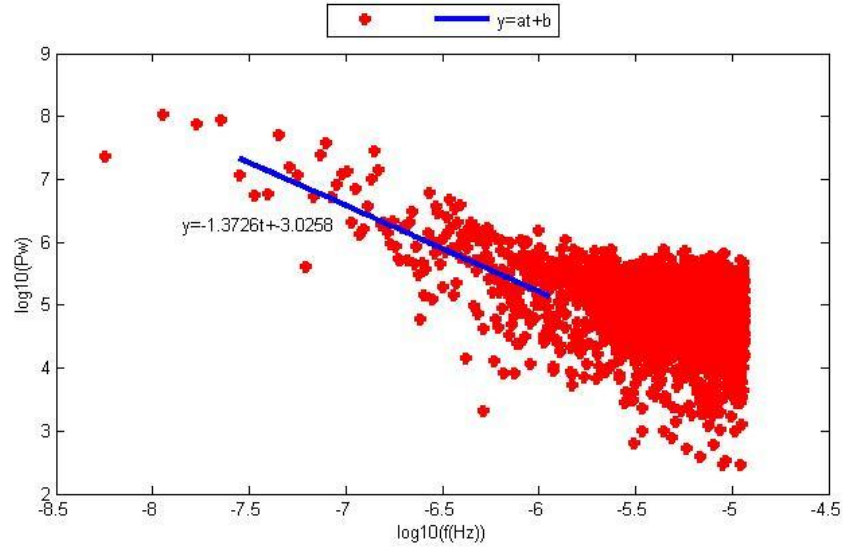
Şekil D.19. KAMN istasyonu kuzey bileşeninin Periyodogram yöntemi ile parametre kestirim sonuçları.
