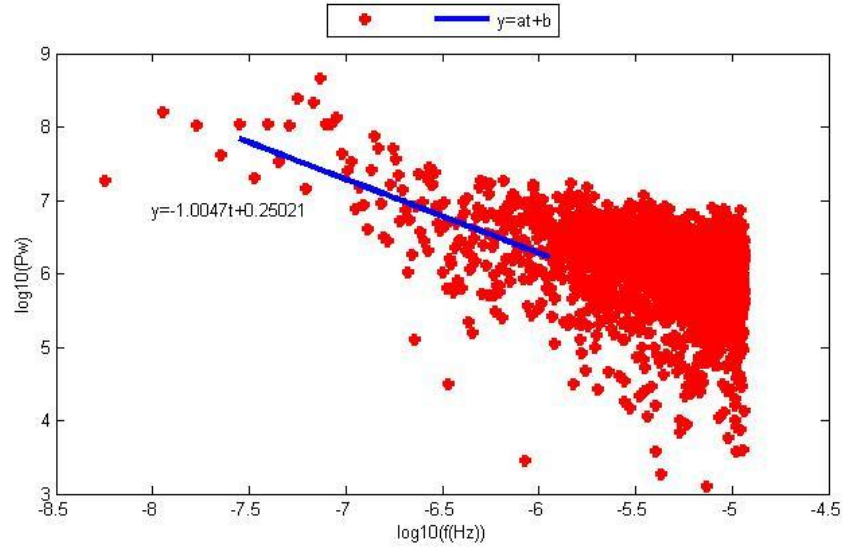
Şekil D.33. NEVS istasyonu yükseklik bileşeninin Periyodogram yöntemi ile parametre kestirim sonuçları.
