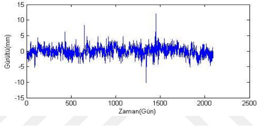
Şekil B 8. ANRK istasyonu doğu bileşeni gürültü-zaman grafiği.
