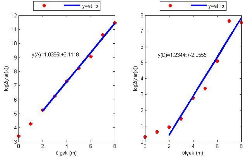
Şekil E.19. KAMN istasyonu kuzey bileşeninin Dalgacık Tabanlı Yöntem ile parametre kestiriminin ölçek boyutunda gösterimi (soldaki şekil yaklaşıklık, sağdaki şekil detay katsayılarına aittir).
