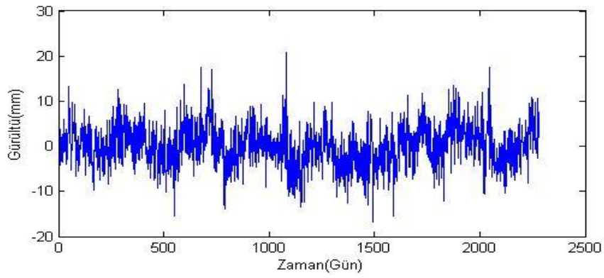
Şekil B.15. CIHA istasyonu yükseklik bileşeni gürültü-zaman grafiği.
