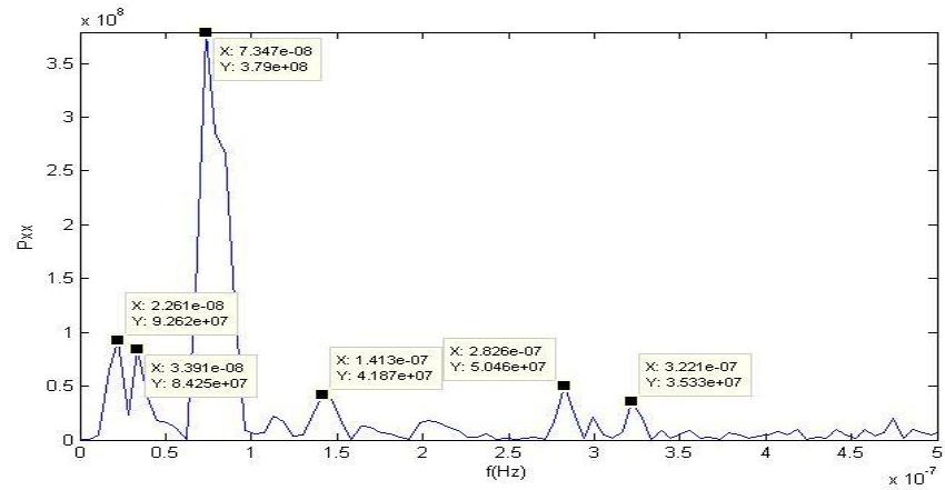
Şekil C.29. KLUU istasyonu doğu bileşeni güç izgesi – frekans grafiği.
