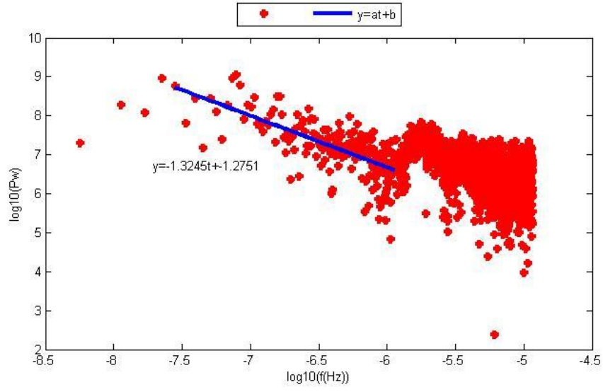
Şekil D.3. AKSI istasyonu yükseklik bileşeninin Periyodogram yöntemi ile parametre kestirim sonuçları.
