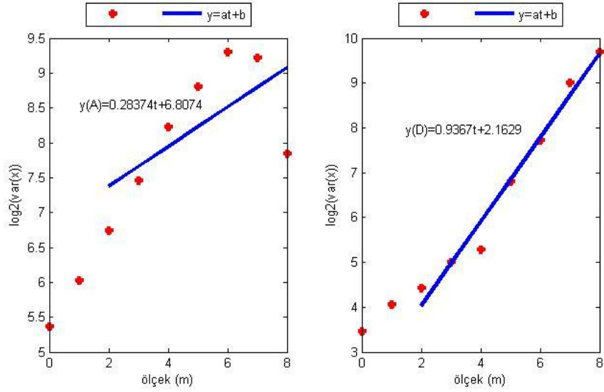
Şekil E.18. HYMN istasyonu yükseklik bileşeninin Dalgacık Tabanlı Yöntem ile parametre kestiriminin ölçek boyutunda gösterimi (soldaki şekil yaklaşıklık, sağdaki şekil detay katsayılarına aittir).
