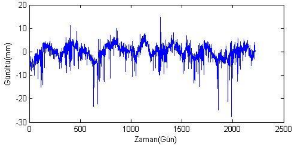
Şekil 5.8. AKHR istasyonu yükseklik bileşeni gürültü-zaman grafiği.
