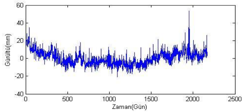
Şekil B.21. KAMN istasyonu yükseklik bileşeni gürültü-zaman grafiği.
