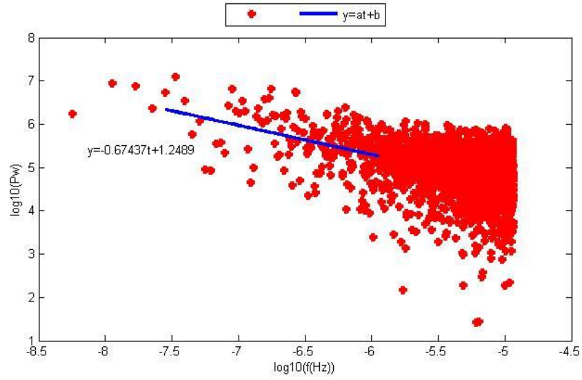
Şekil D.8. ANRK istasyonu doğu bileşeninin Periyodogram yöntemi ile parametre kestirim sonuçları.
