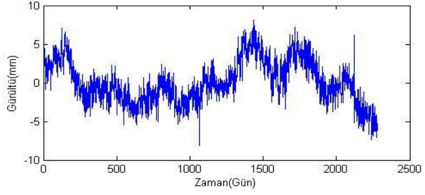
Şekil B.13. CIHA istasyonu kuzey bileşeni gürültü-zaman grafiği.
