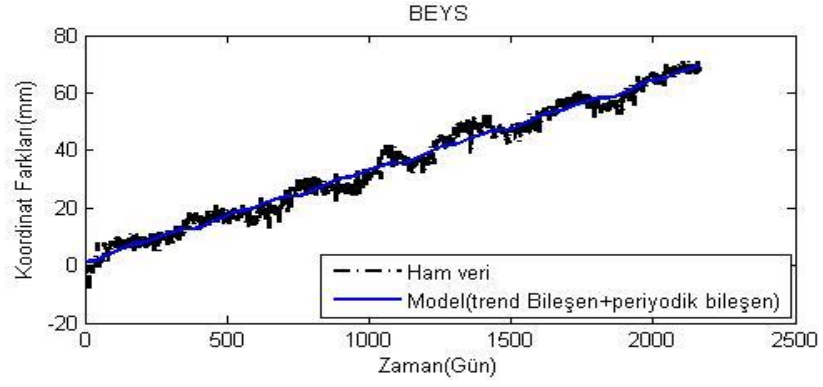
Şekil A.10. BEYS istasyonu kuzey ham koordinatları ve modelden elde edilen koordinatlar.
