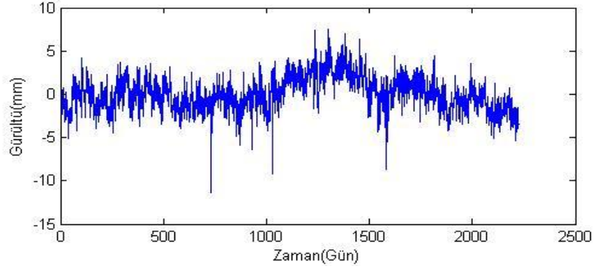
Şekil B.31. NEVS istasyonu kuzey bileşeni gürültü-zaman grafiği.
