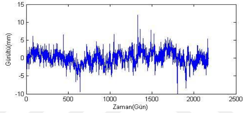
Şekil B.35. NIGD istasyonu kuzey bileşeni gürültü-zaman grafiği.
