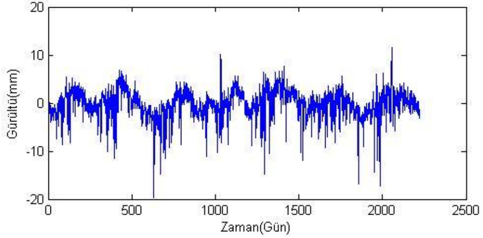
Şekil 5.7. AKHR istasyonu doğu bileşeni gürültü-zaman grafiği.
