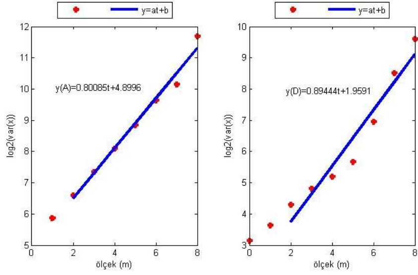
Şekil E.15. CIHA istasyonu yükseklik bileşeninin Dalgacık Tabanlı Yöntem ile parametre kestiriminin ölçek boyutunda gösterimi (soldaki şekil yaklaşıklık, sağdaki şekil detay katsayılarına aittir).
