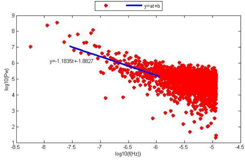
Şekil D.13. CIHA istasyonu kuzey bileşeninin Periyodogram yöntemi ile parametre kestirim sonuçları.
