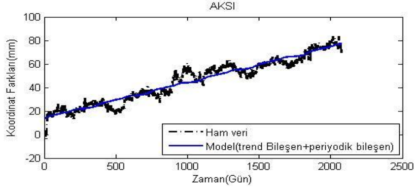
Şekil A.1. AKSI istasyonu kuzey ham koordinatları ve modelden elde edilen koordinatlar.
