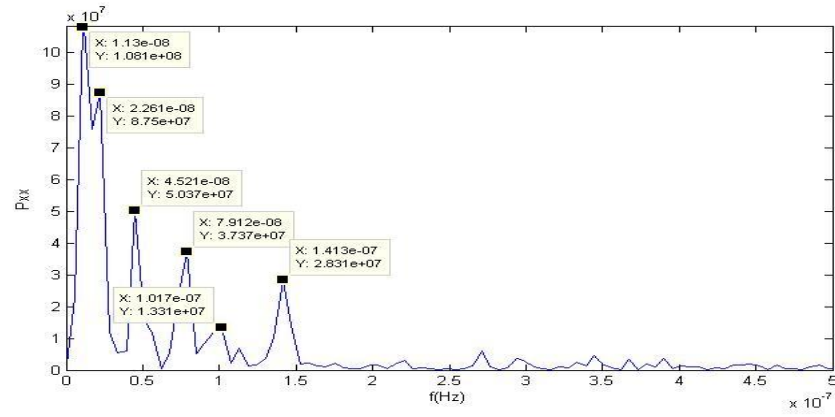
Şekil C.19. KAMN istasyonu kuzey bileşeni güç izgesi – frekans grafiği.
