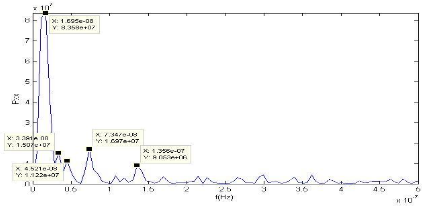
Şekil C.31. NEVS istasyonu kuzey bileşeni güç izgesi – frekans grafiği.
