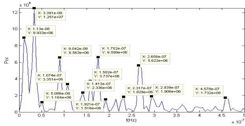
Şekil C.7. ANRK istasyonu kuzey bileşeni güç izgesi – frekans grafiği.
