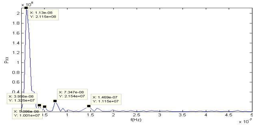
Şekil C.16. HYMN istasyonu kuzey bileşeni güç izgesi – frekans grafiği.
