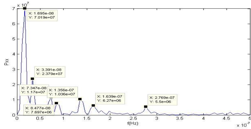
Şekil C.25. KIRS istasyonu kuzey bileşeni güç izgesi – frekans grafiği.
