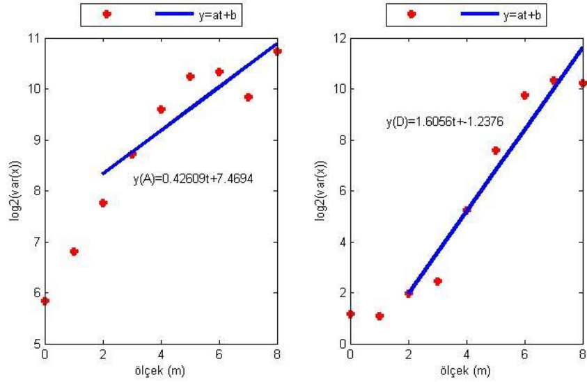
Şekil E.2. AKSI istasyonu doğu bileşeninin Dalgacık Tabanlı Yöntem ile parametre kestiriminin ölçek boyutunda gösterimi (soldaki şekil yaklaşıklık, sağdaki şekil detay katsayılarına aittir).
