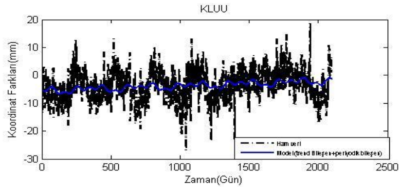
Şekil A.29. KLUU istasyonu doğu ham koordinatları ve modelden elde edilen koordinatlar.
