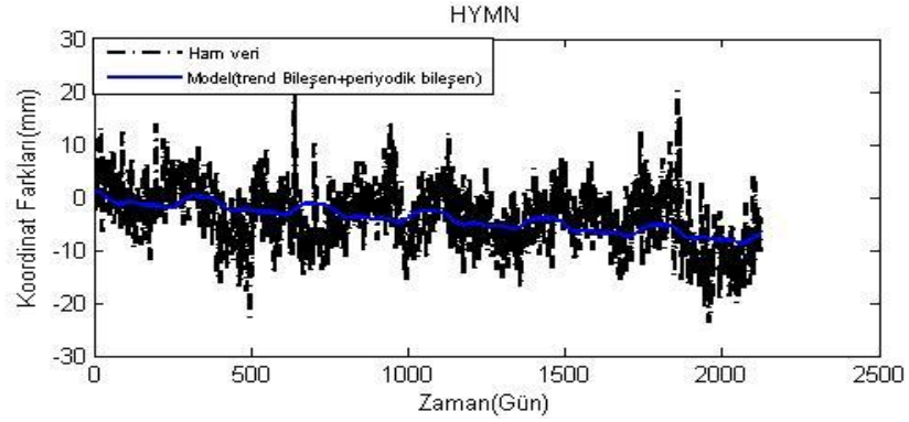
Şekil A.17. HYMN istasyonu doğu ham koordinatları ve modelden elde edilen koordinatlar.
