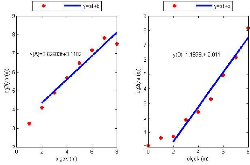
Şekil E.7. ANRK istasyonu kuzey bileşeninin Dalgacık Tabanlı Yöntem ile parametre kestiriminin ölçek boyutunda gösterimi (soldaki şekil yaklaşıklık, sağdaki şekil detay katsayılarına aittir).
