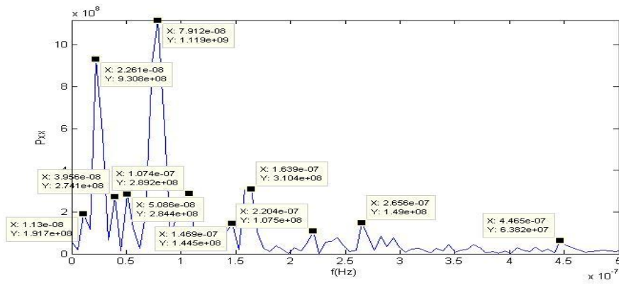
Şekil C.2. AKSI istasyonu kuzey bileşeni güç izgesi – frekans grafiği.
