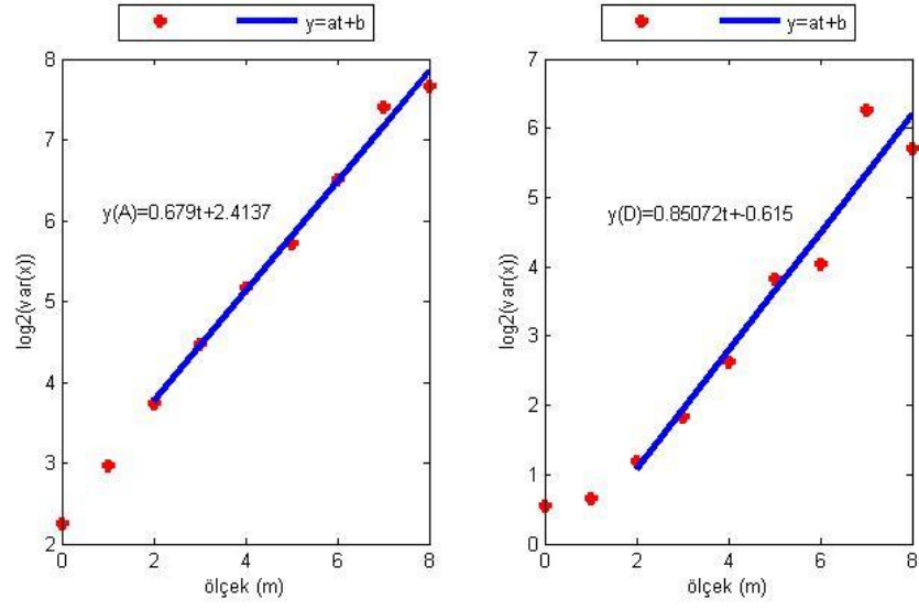
Şekil E.5. AKSR istasyonu doğu bileşeninin Dalgacık Tabanlı Yöntem ile parametre kestiriminin ölçek boyutunda gösterimi (soldaki şekil yaklaşıklık, sağdaki şekil detay katsayılarına aittir).
