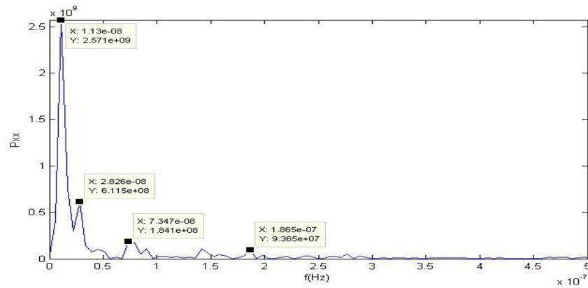
Şekil C.20. KAMN istasyonu doğu bileşeni güç izgesi – frekans grafiği.
