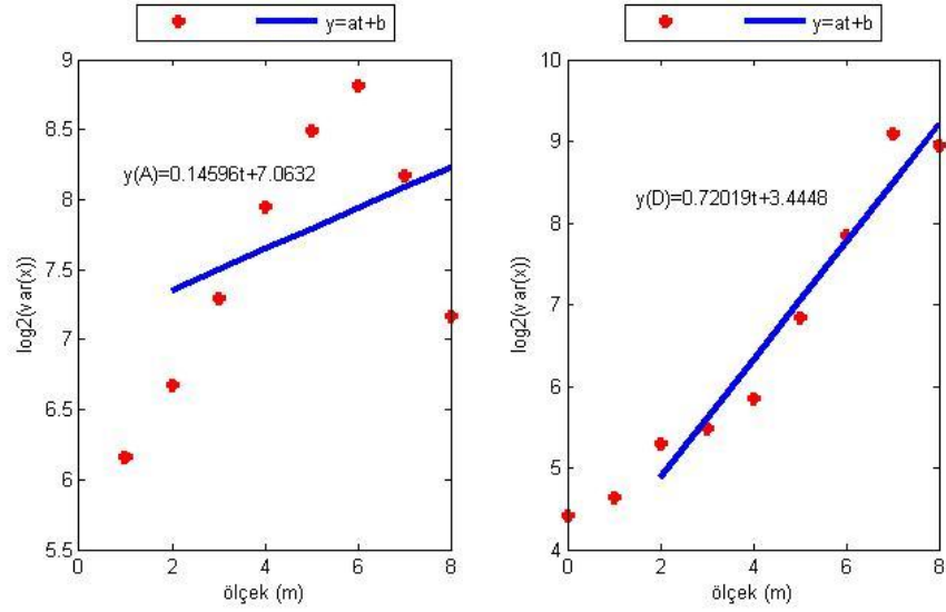
Şekil E.12. BEYS istasyonu yükseklik bileşeninin Dalgacık Tabanlı Yöntem ile parametre kestiriminin ölçek boyutunda gösterimi (soldaki şekil yaklaşıklık, sağdaki şekil detay katsayılarına aittir).
