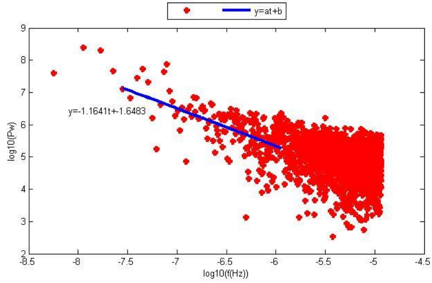
Şekil D.16. HYMN istasyonu kuzey bileşeninin Periyodogram yöntemi ile parametre kestirim sonuçları.
