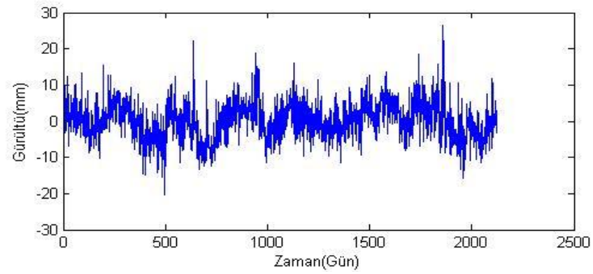
Şekil B.18. HYMN istasyonu yükseklik bileşeni gürültü-zaman grafiği.
