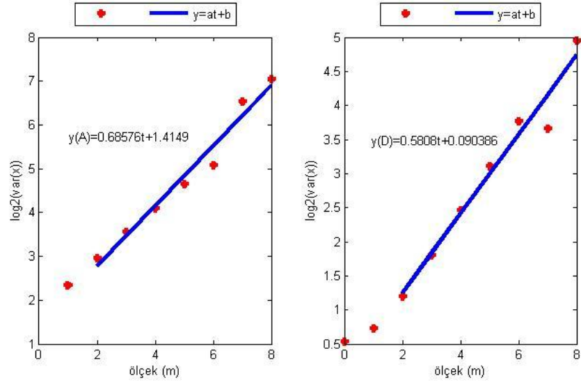
Şekil E.8. ANRK istasyonu doğu bileşeninin Dalgacık Tabanlı Yöntem ile parametre kestiriminin ölçek boyutunda gösterimi (soldaki şekil yaklaşıklık, sağdaki şekil detay katsayılarına aittir).
