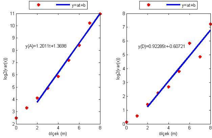
Şekil E.28. KLUU istasyonu kuzey bileşeninin Dalgacık Tabanlı Yöntem ile parametre kestiriminin ölçek boyutunda gösterimi (soldaki şekil yaklaşıklık, sağdaki şekil detay katsayılarına aittir).
