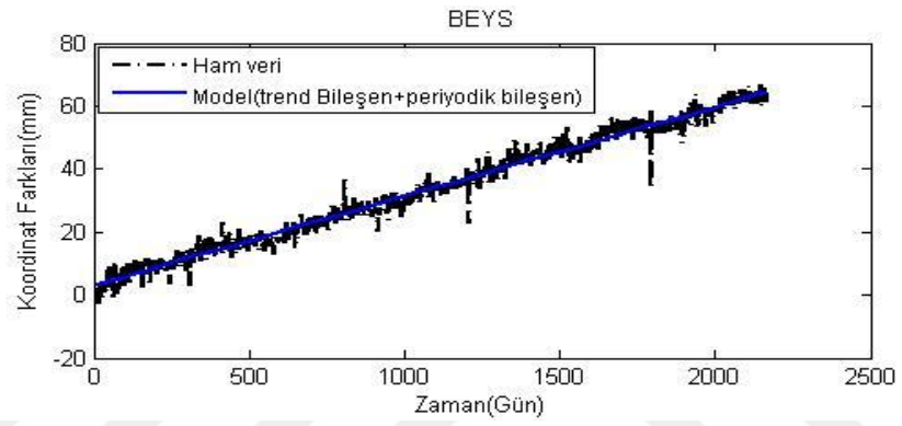
Şekil A.11. BEYS istasyonu doğu ham koordinatları ve modelden elde edilen koordinatlar.
