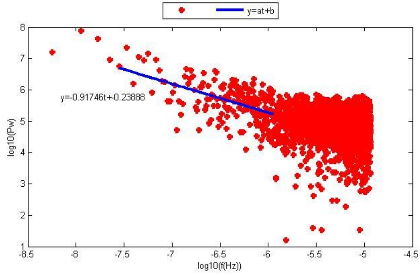
Şekil D.14. CIHA istasyonu doğu bileşeninin Periyodogram yöntemi ile parametre kestirim sonuçları.
