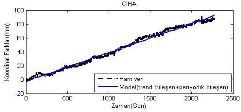
Şekil A.13. CIHA istasyonu kuzey ham koordinatları ve modelden elde edilen koordinatlar.
