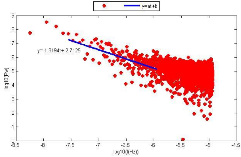
Şekil D.28. KLUU istasyonu kuzey bileşeninin Periyodogram yöntemi ile parametre kestirim sonuçları.
