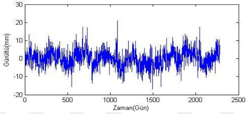
Şekil B.14. CIHA istasyonu doğu bileşeni gürültü-zaman grafiği.
