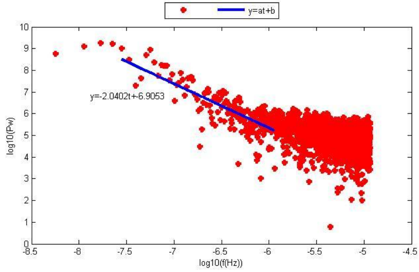
Şekil D.22. KAPN istasyonu kuzey bileşeninin Periyodogram yöntemi ile parametre kestirim sonuçları.
