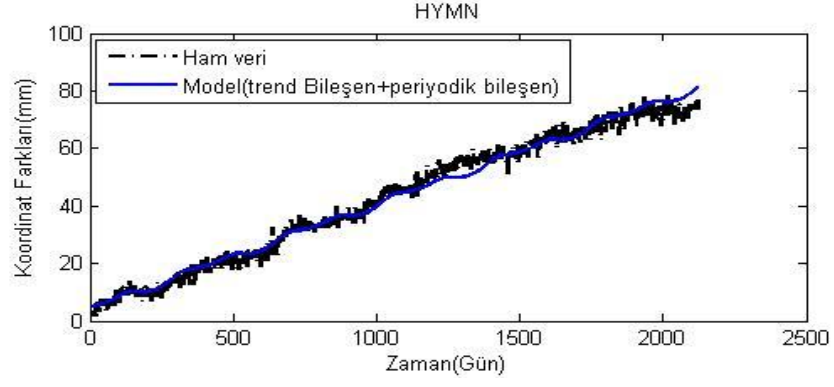
Şekil A.16. HYMN istasyonu kuzey ham koordinatları ve modelden elde edilen koordinatlar.
