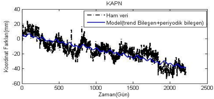
Şekil A.23. KAPN istasyonu doğu ham koordinatları ve modelden elde edilen koordinatlar.
