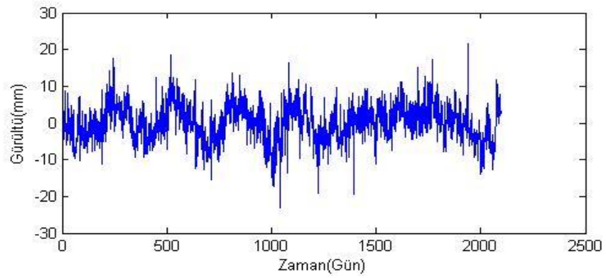
Şekil B.30. KLUU istasyonu yükseklik bileşeni gürültü-zaman grafiği.
