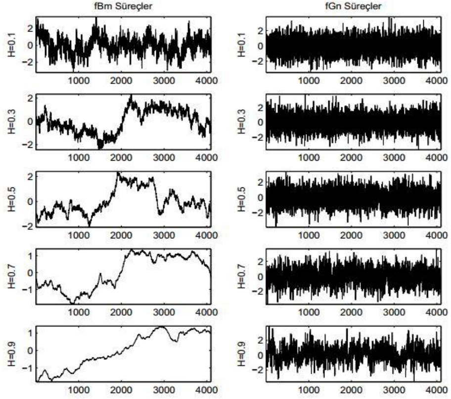
Şekil 3.10. Değişik H değerleri için süreç gösterimleri (soldaki şekil fBm, sağdaki şekil fGn süreçleri göstermektedir) (Baykut, 2012).
