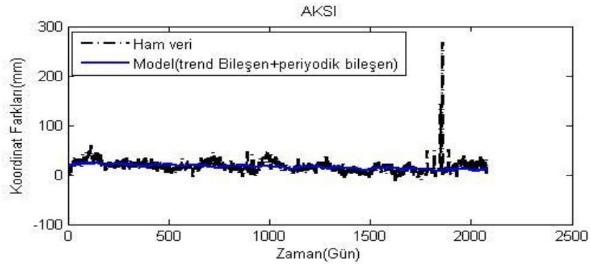
Şekil A.3. AKSI istasyonu yükseklik ham koordinatları ve modelden elde edilen koordinatlar.
