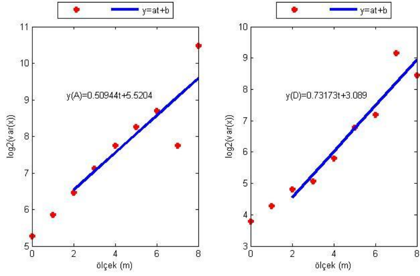
Şekil E.33. NEVS istasyonu yükseklik bileşeninin Dalgacık Tabanlı Yöntem ile parametre kestiriminin ölçek boyutunda gösterimi (soldaki şekil yaklaşıklık, sağdaki şekil detay katsayılarına aittir).
