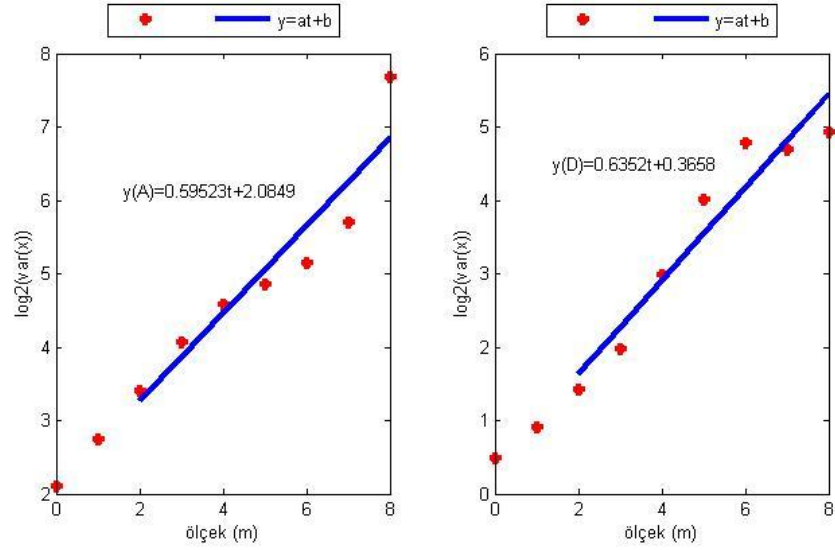
Şekil E.32. NEVS istasyonu doğu bileşeninin Dalgacık Tabanlı Yöntem ile parametre kestiriminin ölçek boyutunda gösterimi (soldaki şekil yaklaşıklık, sağdaki şekil detay katsayılarına aittir).
