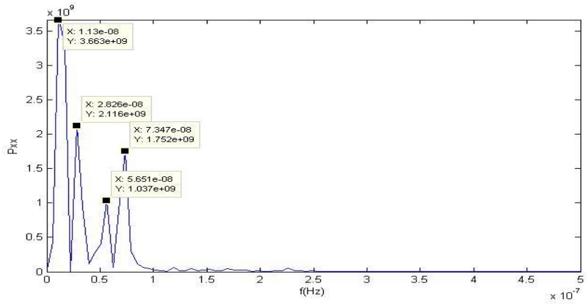
Şekil C.22. KAPN istasyonu kuzey bileşeni güç izgesi – frekans grafiği.
