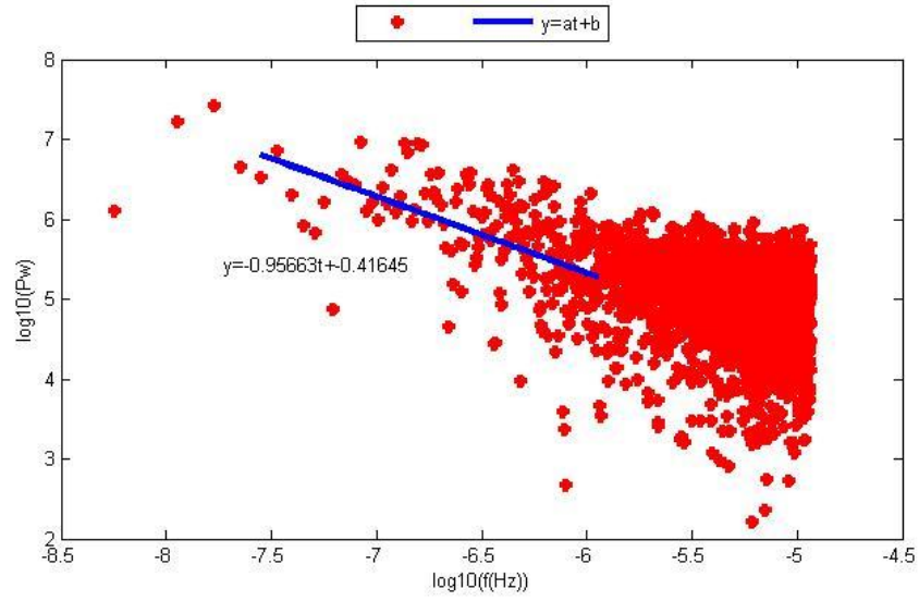
Şekil D.32. NEVS istasyonu doğu bileşeninin Periyodogram yöntemi ile parametre kestirim sonuçları.
