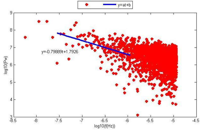
Şekil 5.14. AKHR istasyonu yükseklik bileşeninin Periyodogram yöntemi ile parametre kestirim sonuçları.
