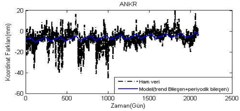
Şekil A.9. ANRK istasyonu yükseklik ham koordinatları ve modelden elde edilen koordinatlar.
