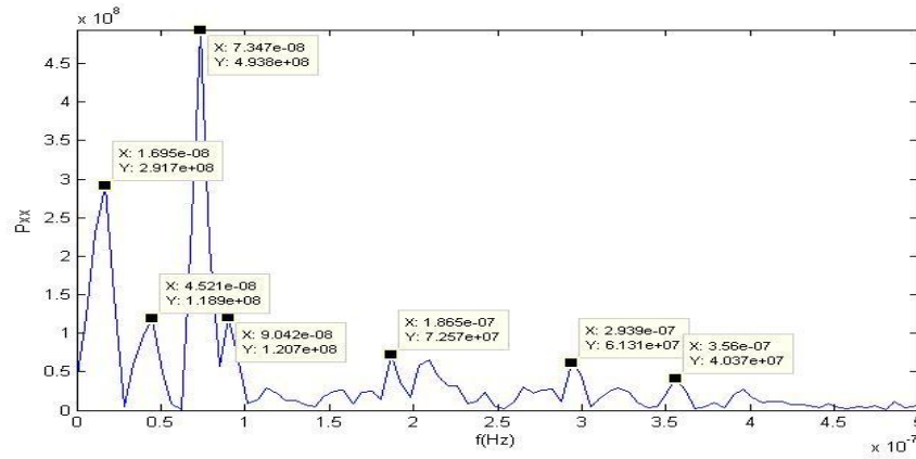
Şekil C.8. ANRK istasyonu doğu bileşeni güç izgesi – frekans grafiği.
