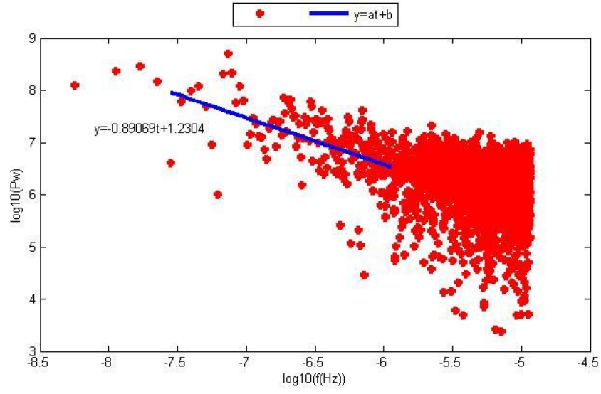
Şekil D.9. ANRK istasyonu yükseklik bileşeninin Periyodogram yöntemi ile parametre kestirim sonuçları.
