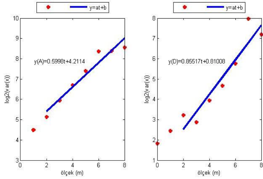
Şekil 5.15. AKHR istasyonu kuzey bileşeninin Dalgacık Tabanlı Yöntem ile parametre kestiriminin ölçek boyutunda gösterimi (soldaki şekil yaklaşıklık, sağdaki şekil detay katsayılarına aittir).
