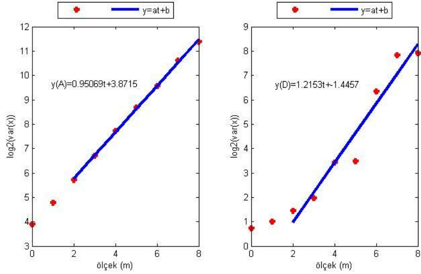
Şekil E.20. KAMN istasyonu doğu bileşeninin Dalgacık Tabanlı Yöntem ile parametre kestiriminin ölçek boyutunda gösterimi (soldaki şekil yaklaşıklık, sağdaki şekil detay katsayılarına aittir).
