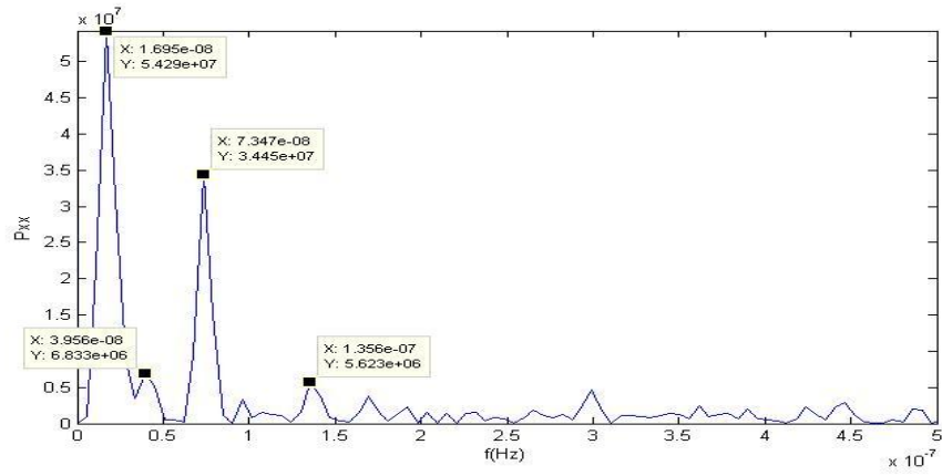
Şekil C.4. AKSR istasyonu kuzey bileşeni güç izgesi – frekans grafiği.
