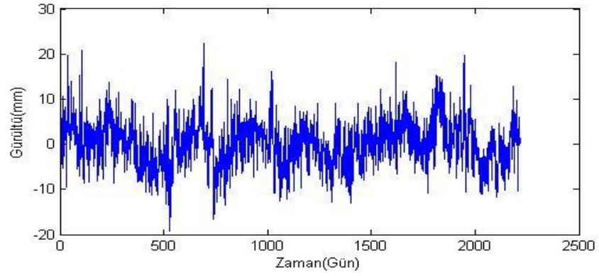
Şekil B.6. AKSR istasyonu yükseklik bileşeni gürültü-zaman grafiği.
