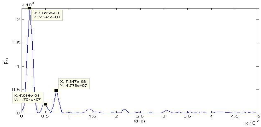
Şekil C.34. NIGD istasyonu kuzey bileşeni güç izgesi – frekans grafiği.
