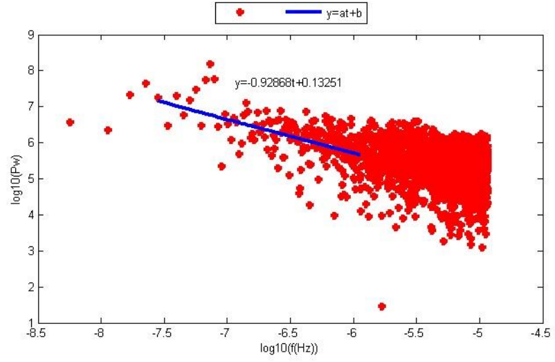
Şekil 5.12. AKHR istasyonu kuzey bileşeninin Periyodogram yöntemi ile parametre kestirim sonuçları.
