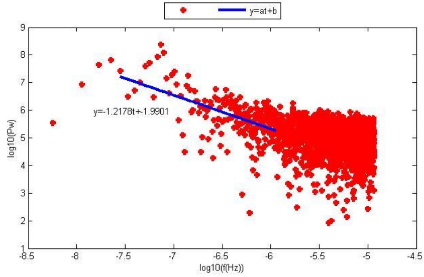
Şekil D.10. BEYS istasyonu kuzey bileşeninin Periyodogram yöntemi ile parametre kestirim sonuçları.
