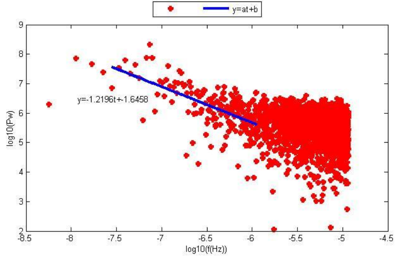
Şekil 5.13. AKHR istasyonu doğu bileşeninin Periyodogram yöntemi ile parametre kestirim sonuçları.
