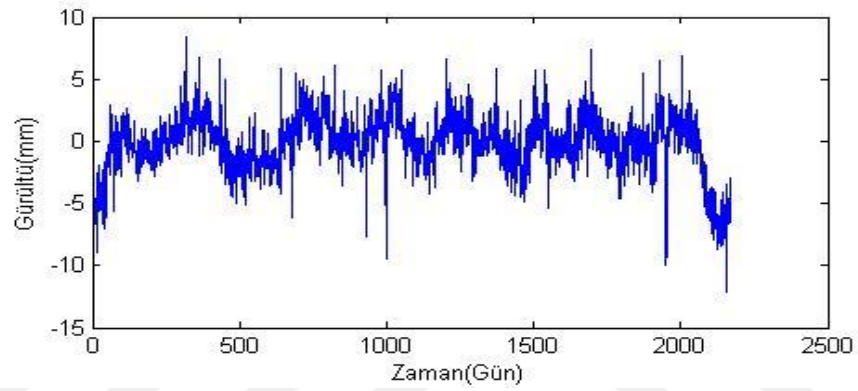
Şekil B.19. KAMN istasyonu kuzey bileşeni gürültü-zaman grafiği.
