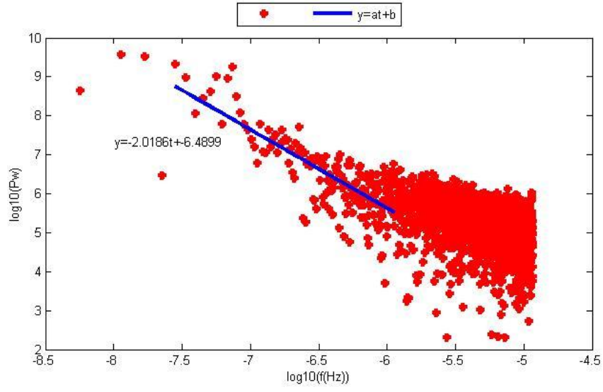
Şekil D.23. KAPN istasyonu doğu bileşeninin Periyodogram yöntemi ile parametre kestirim sonuçları.
