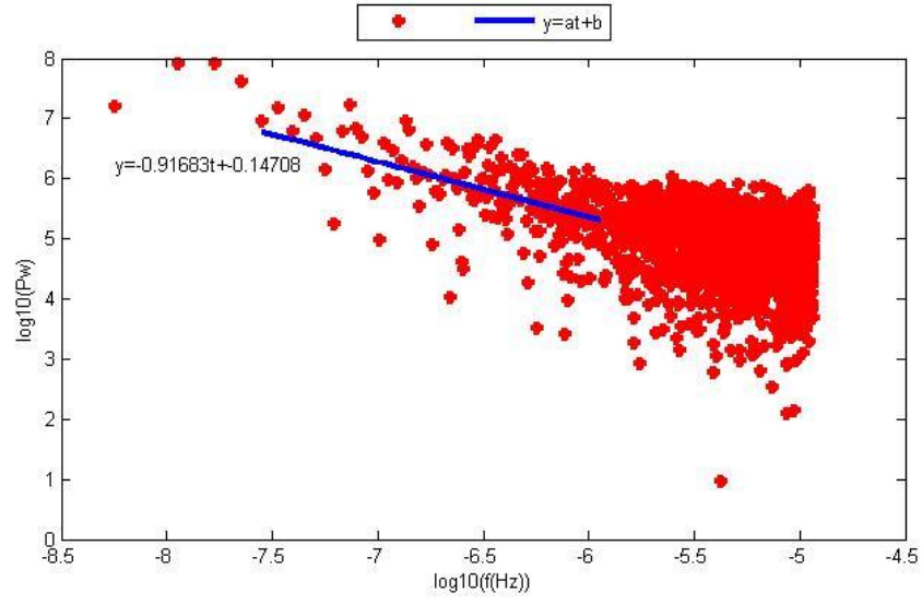
Şekil D.31. NEVS istasyonu kuzey bileşeninin Periyodogram yöntemi ile parametre kestirim sonuçları.
