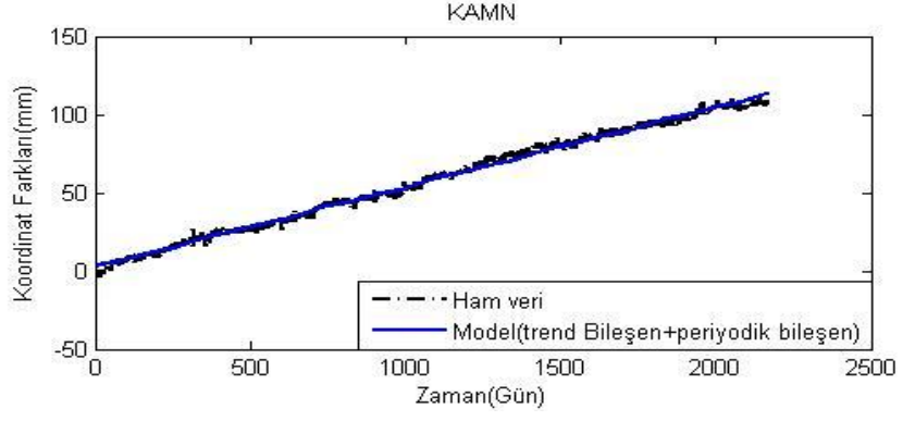
Şekil A.19. KAMN istasyonu kuzey ham koordinatları ve modelden elde edilen koordinatlar.
