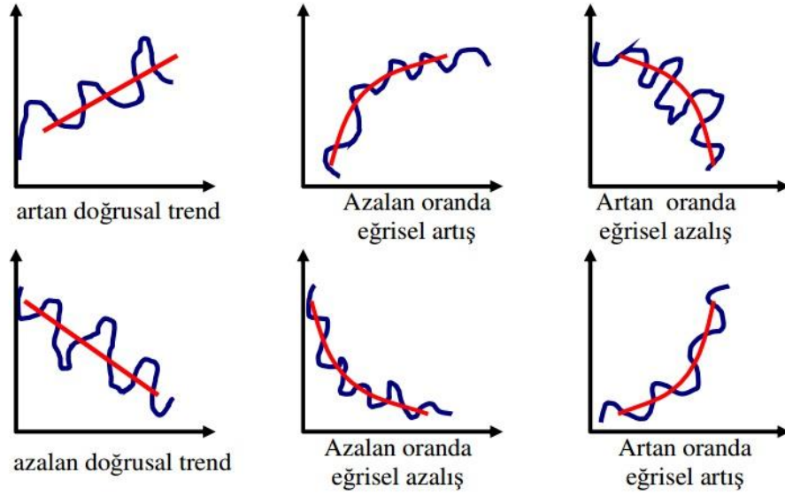
Şekil 3.4. Gerçekleşmesi olası trendlerin gösterimleri (Yiğit, 2010).
