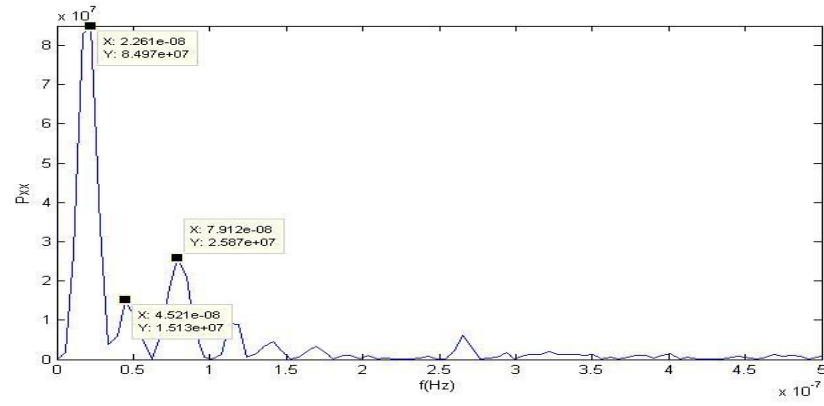
Şekil C.7. ANRK istasyonu kuzey bileşeni güç izgesi – frekans grafiği.
