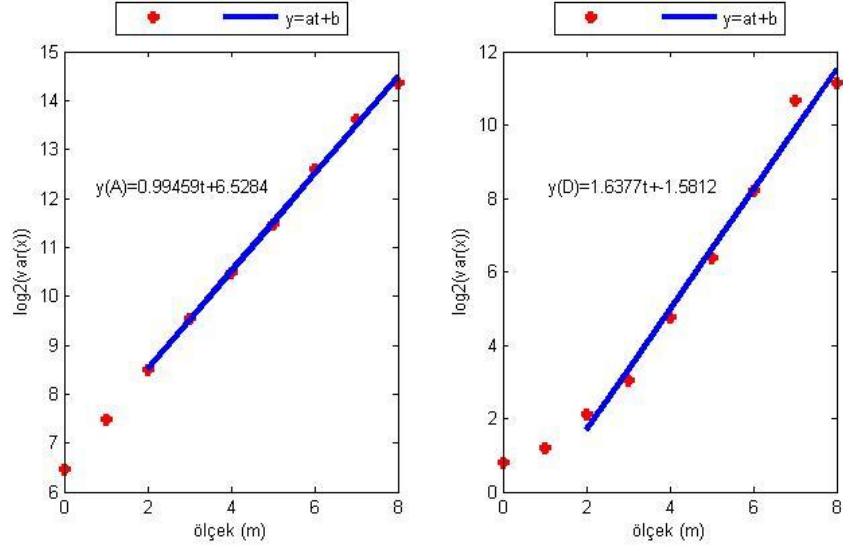
Şekil E.1. AKSI istasyonu kuzey bileşeninin Dalgacık Tabanlı Yöntem ile parametre kestiriminin ölçek boyutunda gösterimi (soldaki şekil yaklaşıklık, sağdaki şekil detay katsayılarına aittir).
