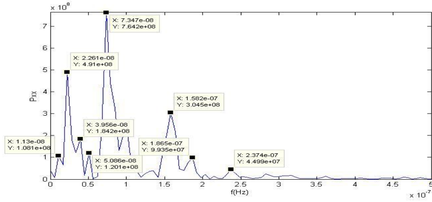
Şekil C.1. AKSI istasyonu kuzey bileşeni güç izgesi – frekans grafiği.
