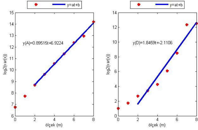
Şekil E.23. KAPN istasyonu doğu bileşeninin Dalgacık Tabanlı Yöntem ile parametre kestiriminin ölçek boyutunda gösterimi (soldaki şekil yaklaşıklık, sağdaki şekil detay katsayılarına aittir).
