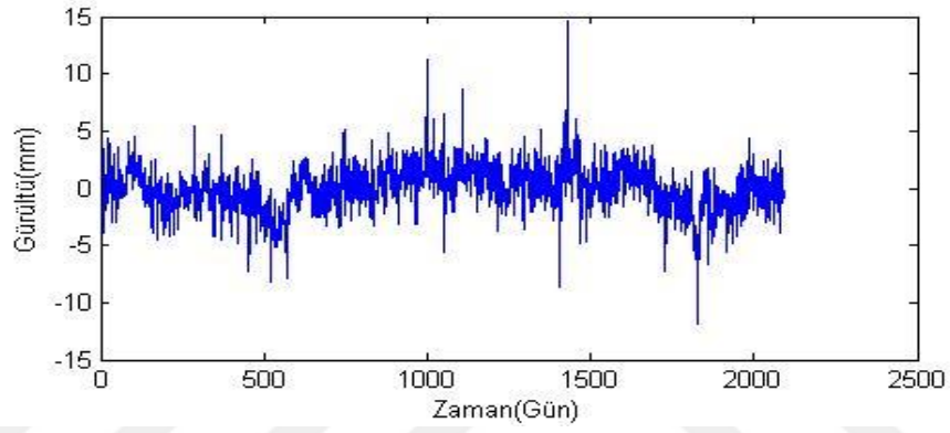
Şekil B.26. KIRS istasyonu doğu bileşeni gürültü-zaman grafiği.
