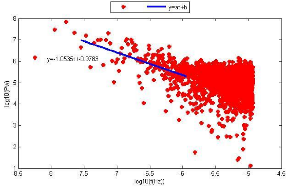
Şekil D.35. NIGD istasyonu doğu bileşeninin Periyodogram yöntemi ile parametre kestirim sonuçları.
