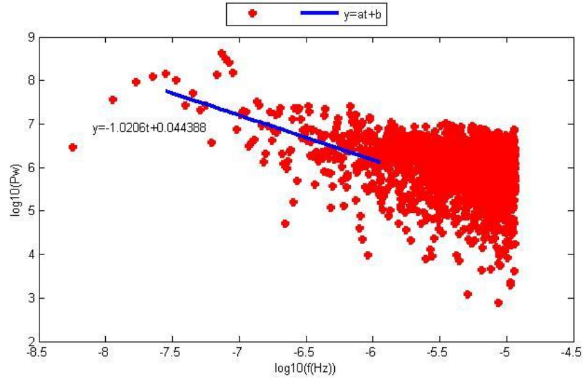
Şekil D.27. KIRS istasyonu yükseklik bileşeninin Periyodogram yöntemi ile parametre kestirim sonuçları.
