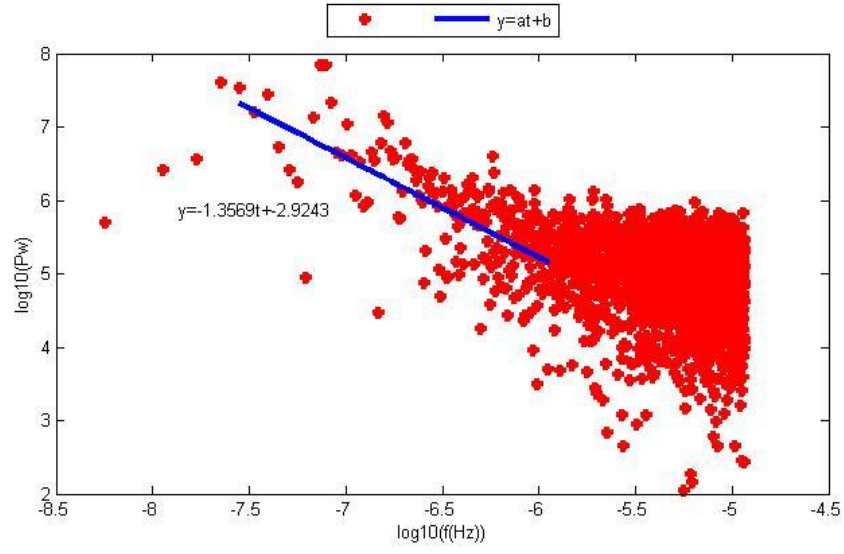
Şekil D.29. KLUU istasyonu doğu bileşeninin Periyodogram yöntemi ile parametre kestirim sonuçları.
