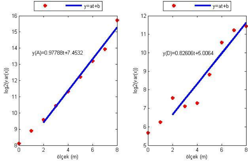
Şekil E.3. AKSI istasyonu yükseklik bileşeninin Dalgacık Tabanlı Yöntem ile parametre kestiriminin ölçek boyutunda gösterimi (soldaki şekil yaklaşıklık, sağdaki şekil detay katsayılarına aittir).
