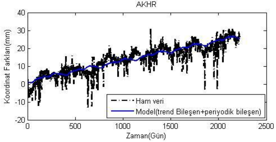
Şekil 5.3. AKHR istasyonu doğu ham koordinatları ve modelden elde edilen koordinatlar.
