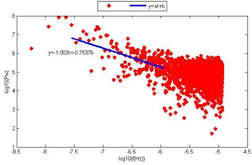
Şekil D.7. ANRK istasyonu kuzey bileşeninin Periyodogram yöntemi ile parametre kestirim sonuçları.
