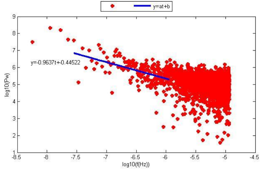
Şekil D.17. HYMN istasyonu doğu bileşeninin Periyodogram yöntemi ile parametre kestirim sonuçları.
