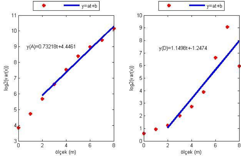
Şekil E.10. BEYS istasyonu kuzey bileşeninin Dalgacık Tabanlı Yöntem ile parametre kestiriminin ölçek boyutunda gösterimi (soldaki şekil yaklaşıklık, sağdaki şekil detay katsayılarına aittir).
