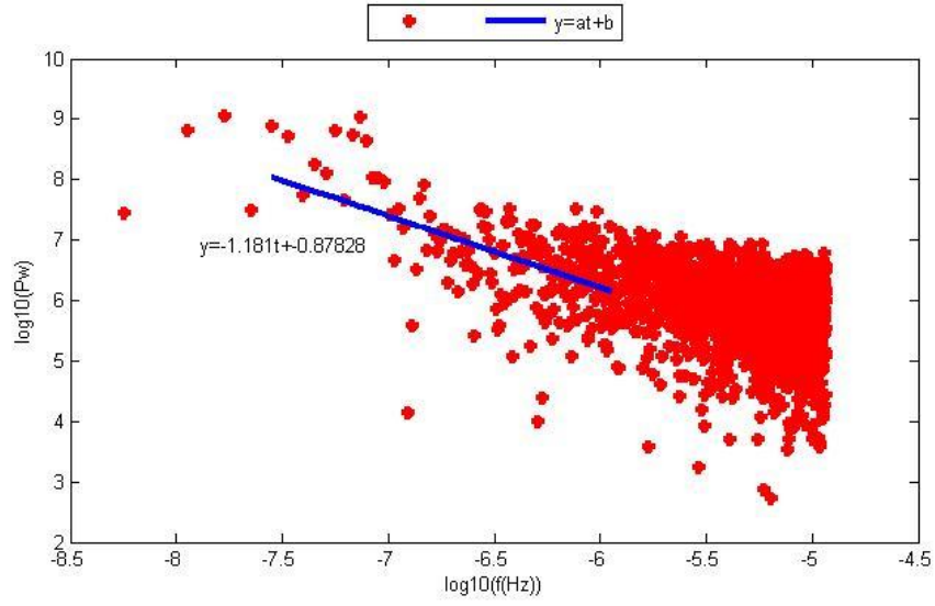
Şekil D.24. KAPN istasyonu yükseklik bileşeninin Periyodogram yöntemi ile parametre kestirim sonuçları.
