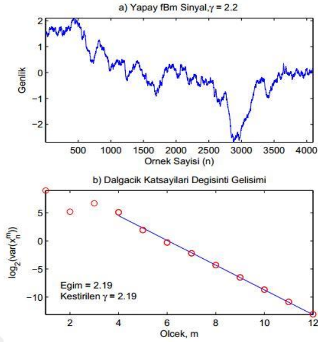
Şekil 4.2. Yapay bir fBm sinyalinin dalgacık tabanı ile kestirimi (Baykut, 2012).
