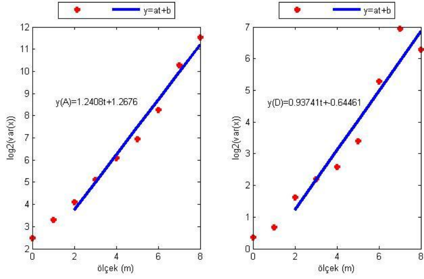
Şekil E.25. KIRS istasyonu kuzey bileşeninin Dalgacık Tabanlı Yöntem ile parametre kestiriminin ölçek boyutunda gösterimi (soldaki şekil yaklaşıklık, sağdaki şekil detay katsayılarına aittir).
