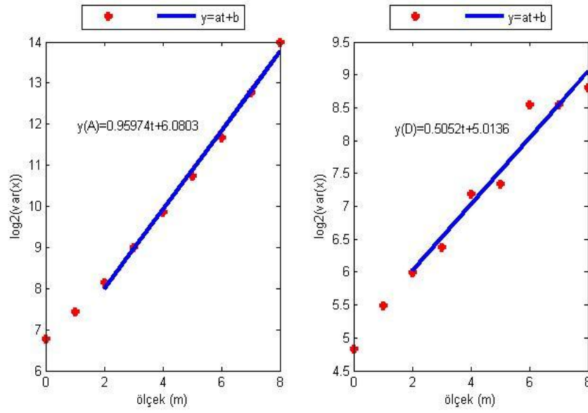
Şekil 5.17. AKHR istasyonu yükseklik bileşeninin Dalgacık Tabanlı Yöntem ile parametre kestiriminin ölçek boyutunda gösterimi (soldaki şekil yaklaşıklık, sağdaki şekil detay katsayılarına aittir).
