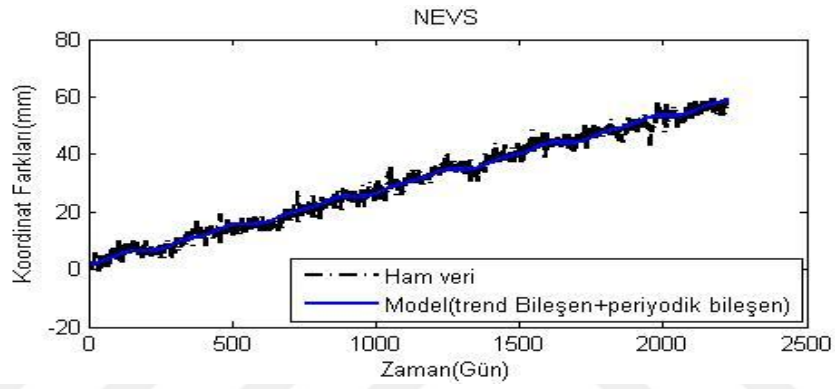
Şekil A.31. NEVS istasyonu kuzey ham koordinatları ve modelden elde edilen koordinatlar.
