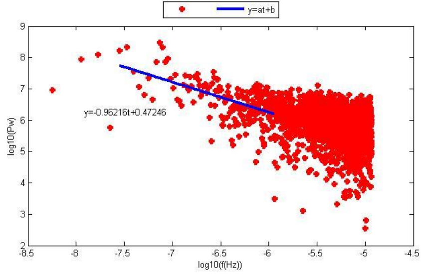
Şekil D.18. HYMN istasyonu yükseklik bileşeninin Periyodogram yöntemi ile parametre kestirim sonuçları.
