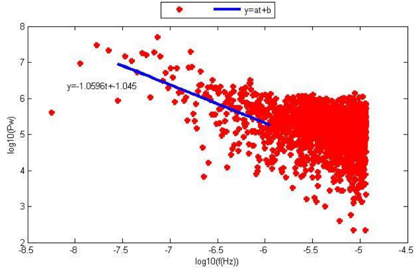
Şekil D.11. BEYS istasyonu doğu bileşeninin Periyodogram yöntemi ile parametre kestirim sonuçları.
