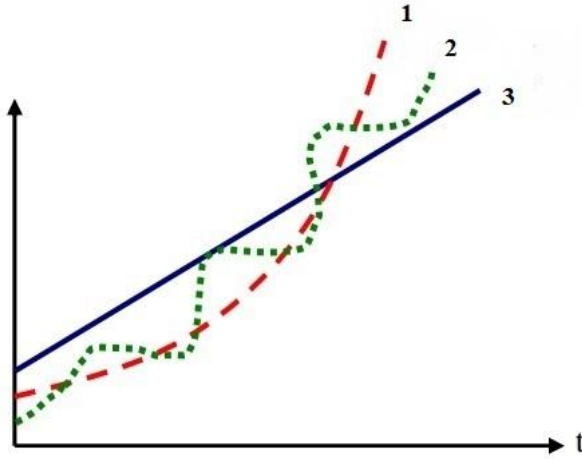
Şekil 3.5. Gerçekleşmesi olası deterministik trendler (1 ve 3 numaralı) ile stokastik bir trendin (2 numaralı) örnek gösterimi (Yiğit, 2010).
