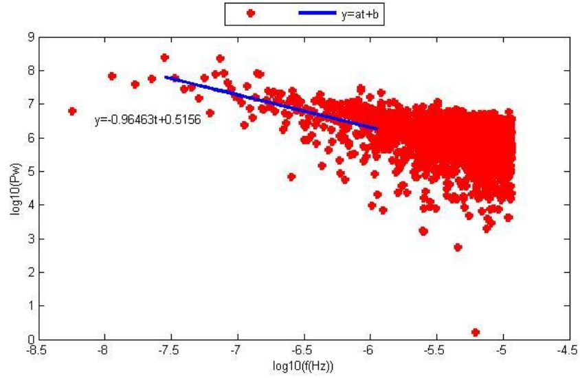
Şekil D.6. AKSR istasyonu yükseklik bileşeninin Periyodogram yöntemi ile parametre kestirim sonuçları.
