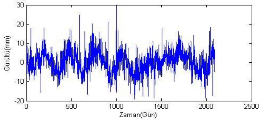
Şekil B.27. KIRS istasyonu yükseklik bileşeni gürültü-zaman grafiği.
