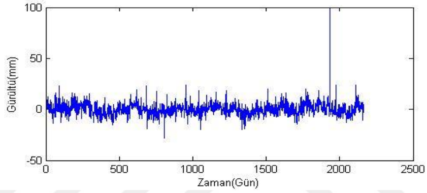
Şekil B.11. BEYS istasyonu doğu bileşeni gürültü-zaman grafiği.
