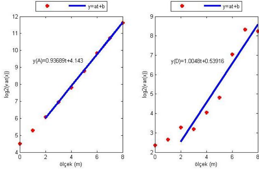
Şekil 5.16. AKHR istasyonu doğu bileşeninin Dalgacık Tabanlı Yöntem ile parametre kestiriminin ölçek boyutunda gösterimi (soldaki şekil yaklaşıklık, sağdaki şekil detay katsayılarına aittir).
