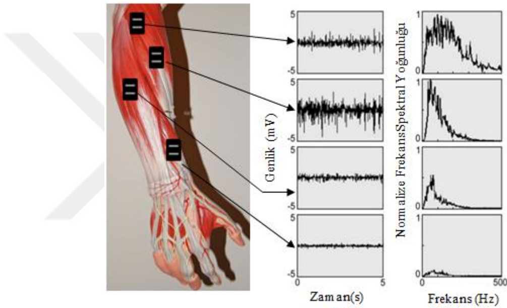
Şekil 3.9. Farklı kas konumlarında elektrotların sinyal üzerine etkisi [8]
