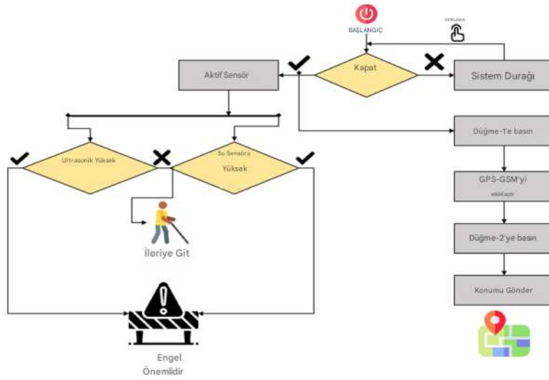
Şekil 9. Su ve GPS sensörü içeren elektronik baston çalışma prensibi (Biswas vd., 2022)
