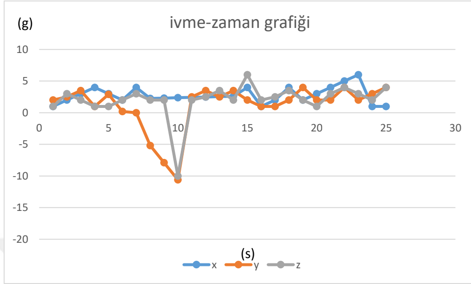
Şekil 17. Akıllı bastonumuz düştüğünde ivmelenme deęerleri
