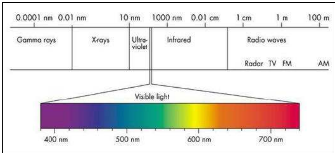
Şekil 2.3. Elektromanyetik spektrum
