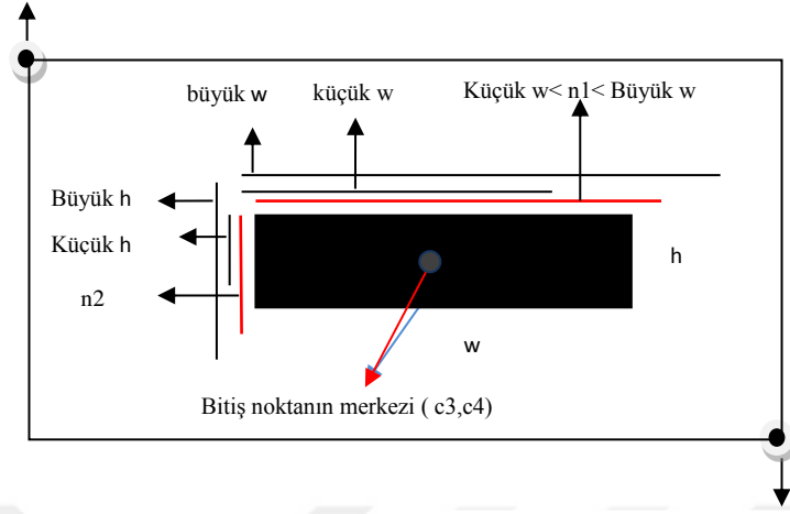
Şekil 3.10. Bitiş noktası algılama algoritması
