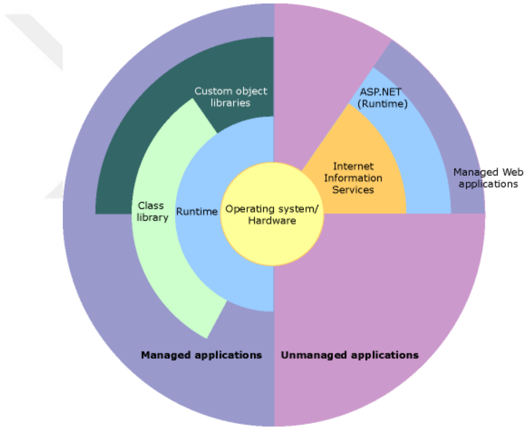
Şekil 2.1. CLR çalışma şeması
