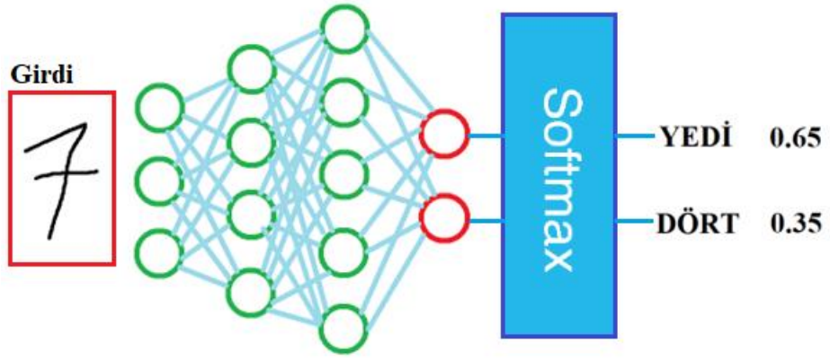
Şekil 3.21. Softmax aktivasyonu
