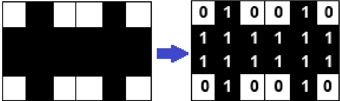
Şekil 3.11. Bitmap grafiği
