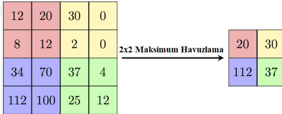
Şekil 3.19. 2x2 Filtre ile Maksimum Havuzlama
