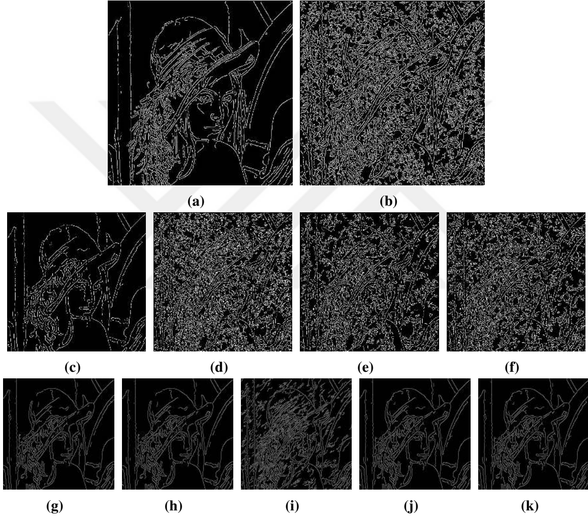
Ş ekil 4.6. Anonim bir görüntünün filtrelendikten sonra Canny kenarları: (a) Orijinal, (b) Gürültü; İzotropik filtreler: (c) Beltrami, (d) Gauss, (e) Mean, (f) Median; Anizotropik filtreler: (g) Yeni Randers, (h) Ingarden, (i) N. Miron, (j) Yeni N.Miron, (k) Yeni Metrik.
