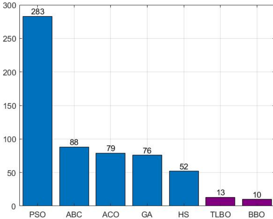
Şekil 2.23. Kullanılan sezgisel algoritmaların yayın sayıları (Hussain vd., 2019: 2191)
