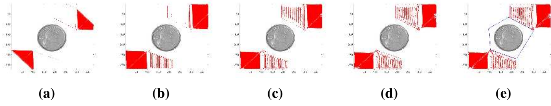
Şekil 2.4. Deney 4: c = 0, \sigma = 1, \rho = 2 . [a, b, c, d] : Sırasıyla 50,100,150,200 üncü tekrarlardaki aktif konturlar, e : Tekrar sonunda oluşan son durum, mavi ile başlangıç eğrisi, kırmızı ile aktif kontur görüntülenmektedir.
