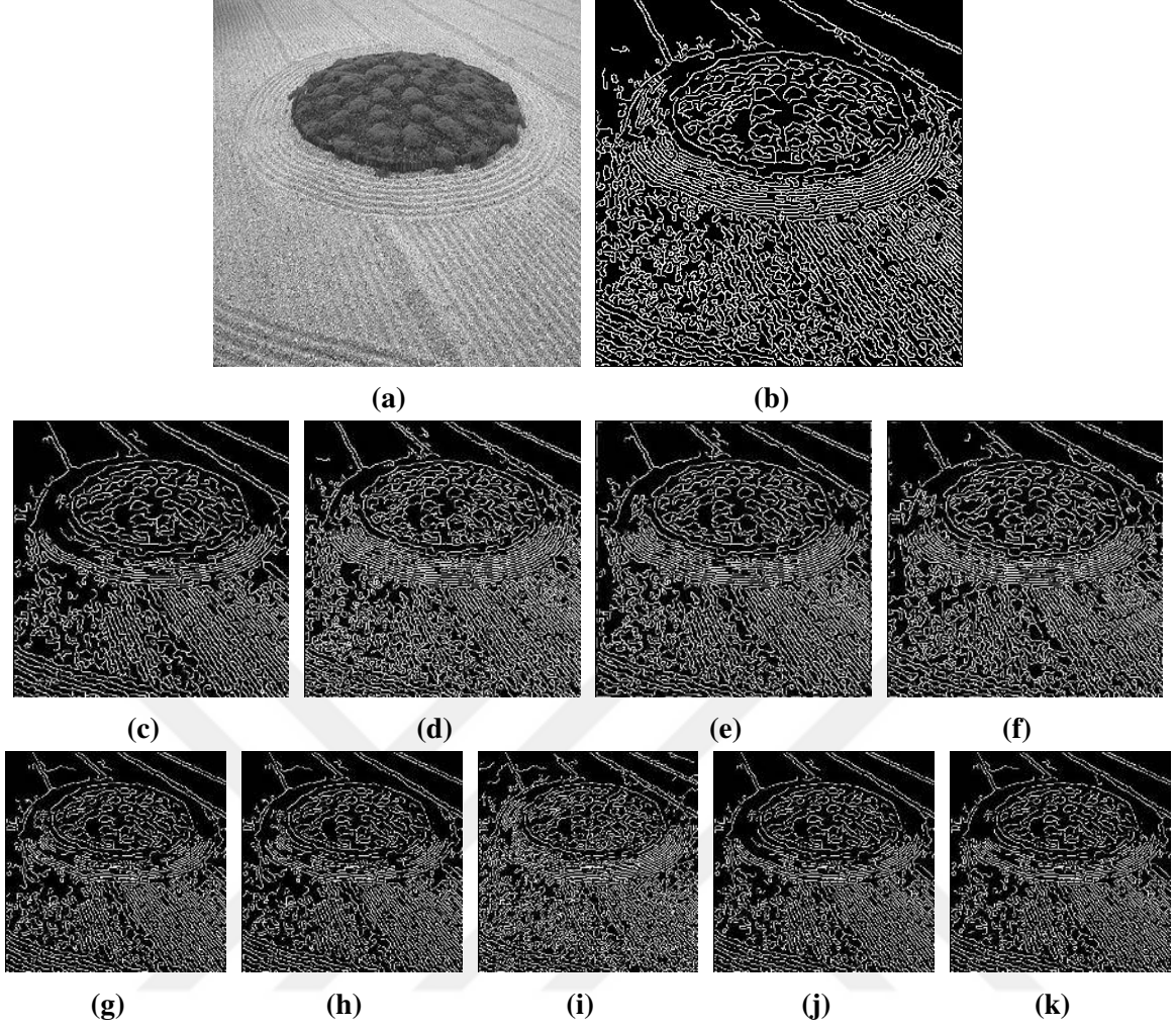
Şekil 4.8. Kamufle bir görüntünün filtrelendikten sonra Canny kenarları: (a) Orijinal, (b) Gürültülü; İzotropik filtreler: (c) Beltrami, (d) Gauss, (e) Mean, (f) Median; Anizotropik filtreler: (g) Yeni Randers, (h) Ingarden, (i) N. Miron, (j) Yeni N.Miron, (k) Yeni Metrik.
