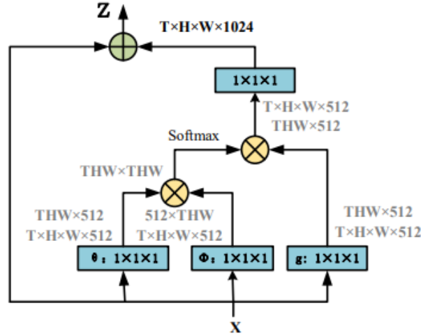
Şekil 1.6. Yerel olmayan sinir ağı [10].
