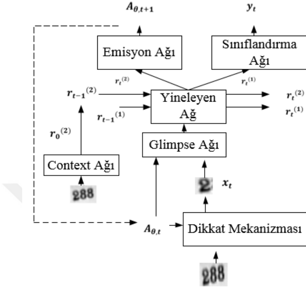
Şekil 1.8. EDRAM model mimarisi [17].
