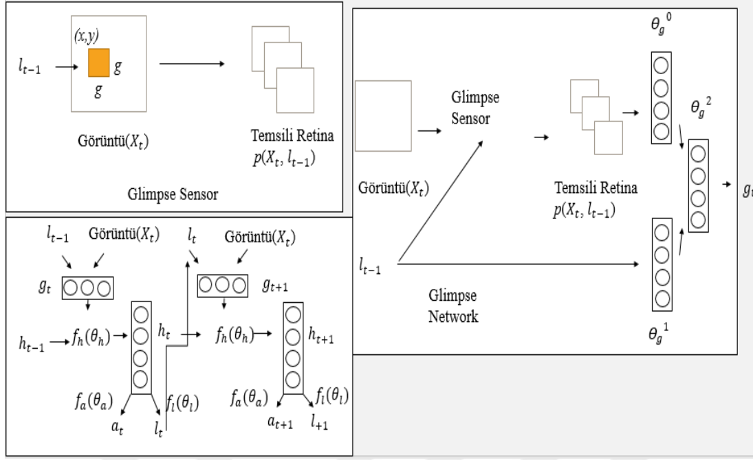
Şekil 1.7. Yineleyen dikkat modeli [15].
