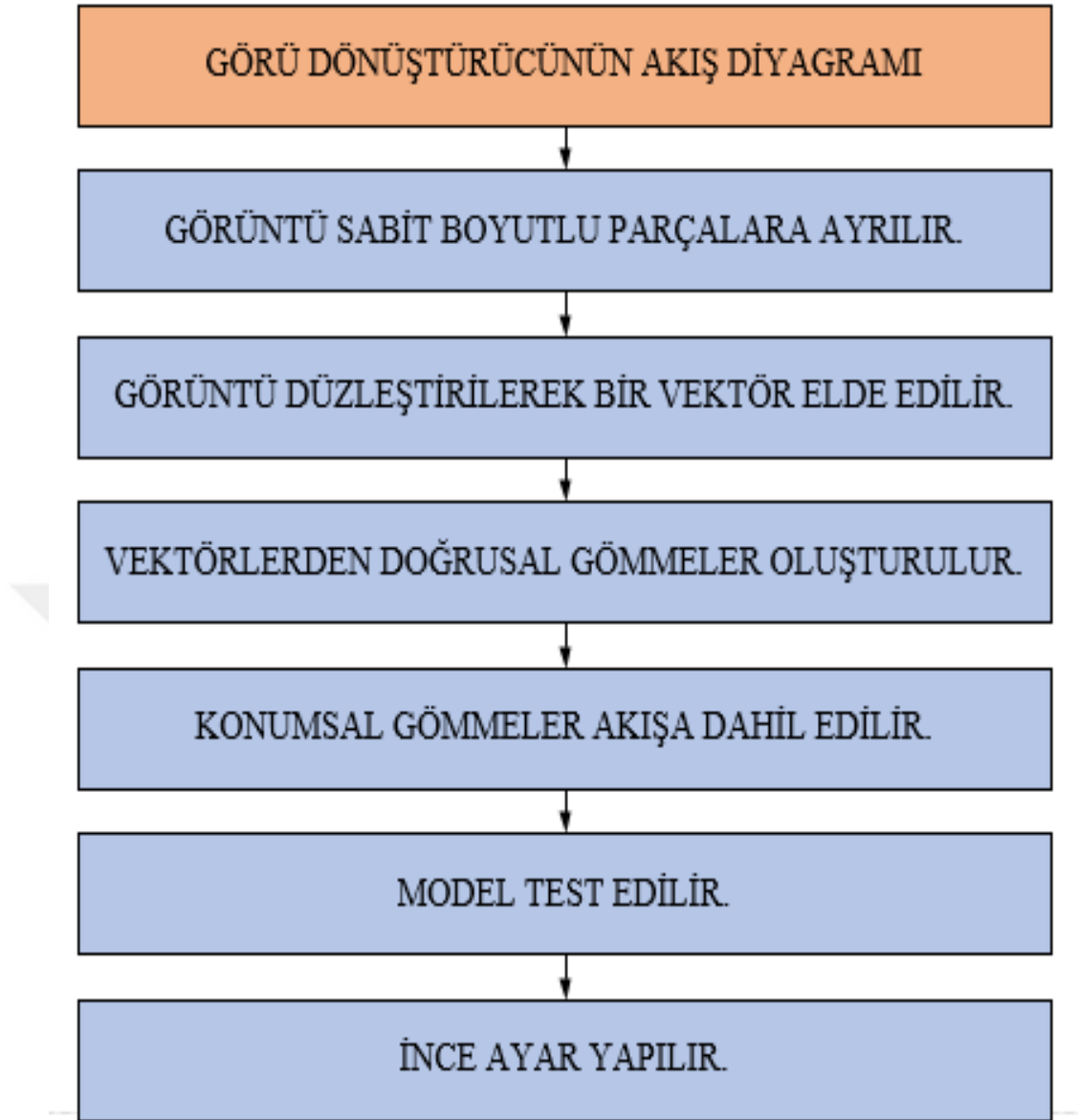
Şekil 4.3. Görü dönüştürücünün akış diyagramı.
