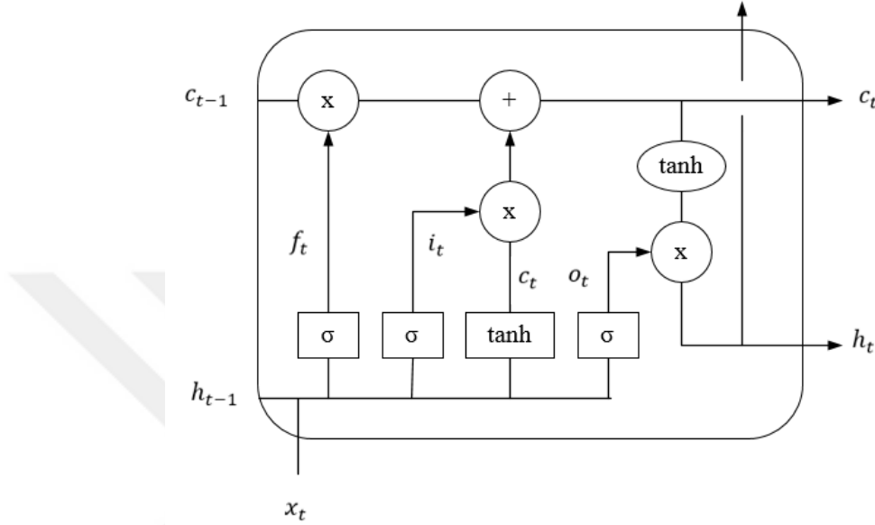
Şekil 2.9. LSTM yapısı.
