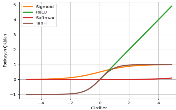
Şekil 2.10. Aktivasyon fonksiyonları değer aralıkları.
