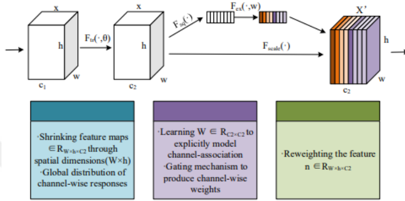
Şekil 1.4. SENet prensibi [10].
