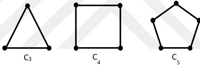
Şekil 1.11. C_3, C_4, C_5 devir grafları
