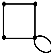
Şekil 1.5. Basit olmayan bir graf
