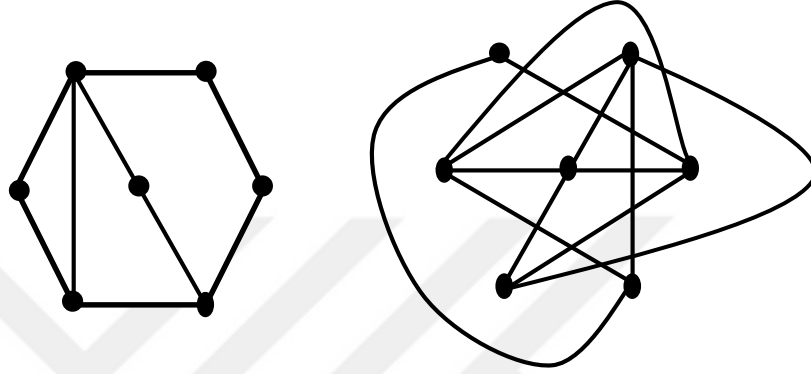
Şekil 1.7. G ve \bar{G} grafları
