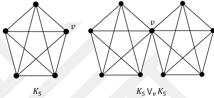
Şekil 6.2. K_5 ve K_5 \vee_v K_5 köşe birleşim grafi
