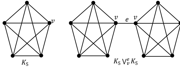
Şekil 6.7. K_5 ve K_5 \vee_v^e K_5 grafi
