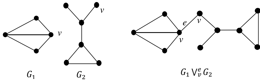
Şekil 6.6. G_1 , G_2 ve G_1 \vee_v^e G_2 grafları
