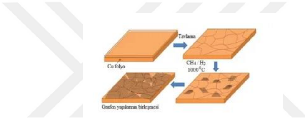
Şekil 2.4. Kimyasal Buhar Biriktirme Yöntemi [135]
