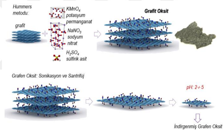
Şekil 2.3. Kimyasal İndirgeme Yöntemi [134]
