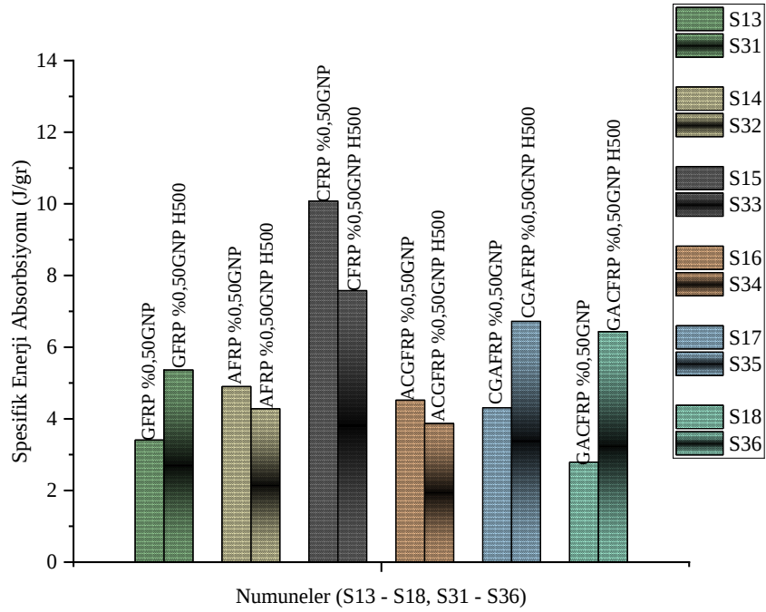
Şekil 4.57. %0,50 grafen ilaveli numunelerde 500 saat hidrotermal yaşlanmada spesifik enerji absorpsiyonları karşılaştırılması
