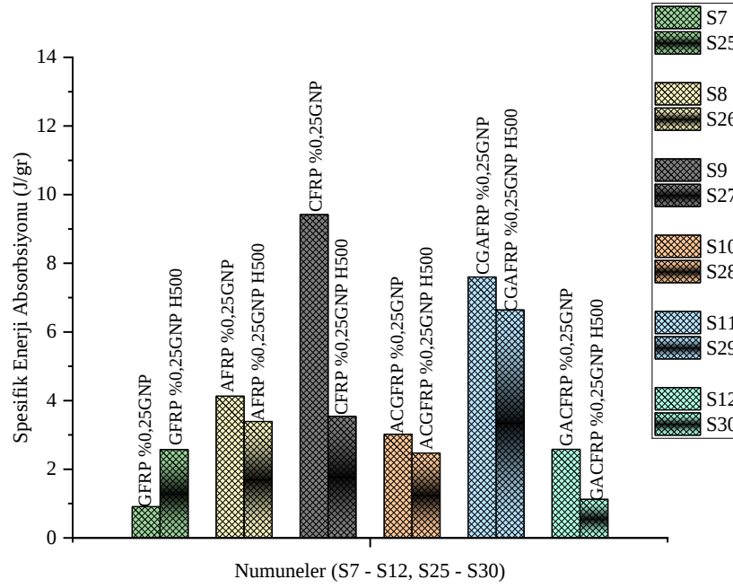
Şekil 4.51. %0,25 grafen ilaveli numunelerde 500 saat hidrotermal yaşlanmanın spesifik enerji absorpsiyonları karşılaştırılması
