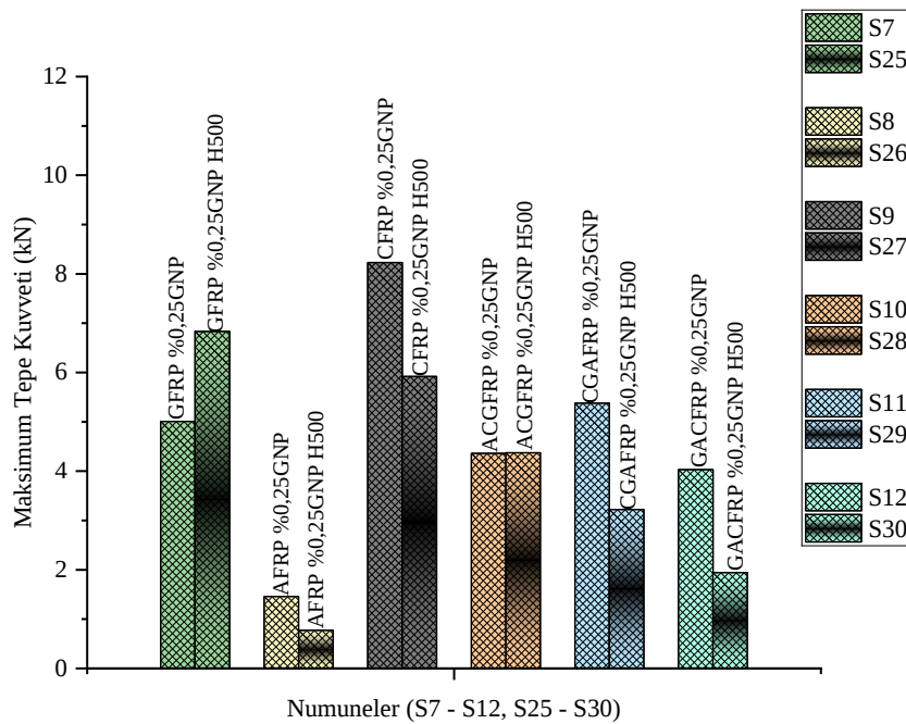
Şekil 4.49. %0,25 grafen ilaveli numunelerde 500 saat hidrotermal yaşlanmanın maksimum tepe kuvveti üzerinde yaptığı etki
