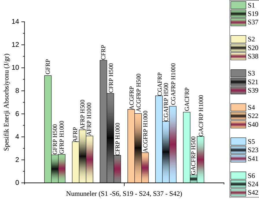
Şekil 4.48. 100 saat yaşlandırılmış numunelerin spesifik enerji absorbsiyonlarının karşılaştırılması
