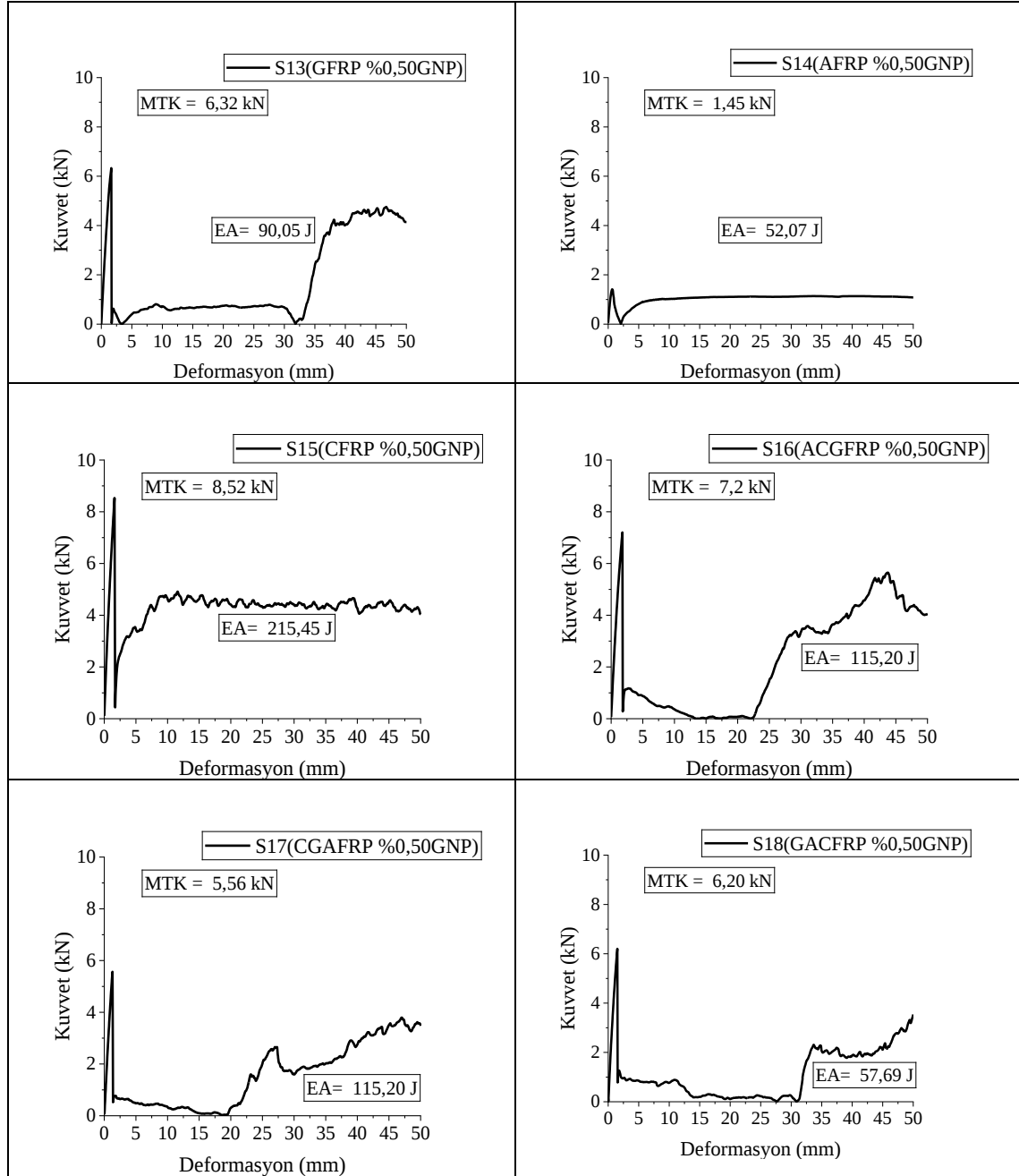
Şekil 4.9. % 0,50 grafen takviyeli hidrotermal yaşlandırılmamış numunelerin kuvvet-yer değişirme grafikleri
