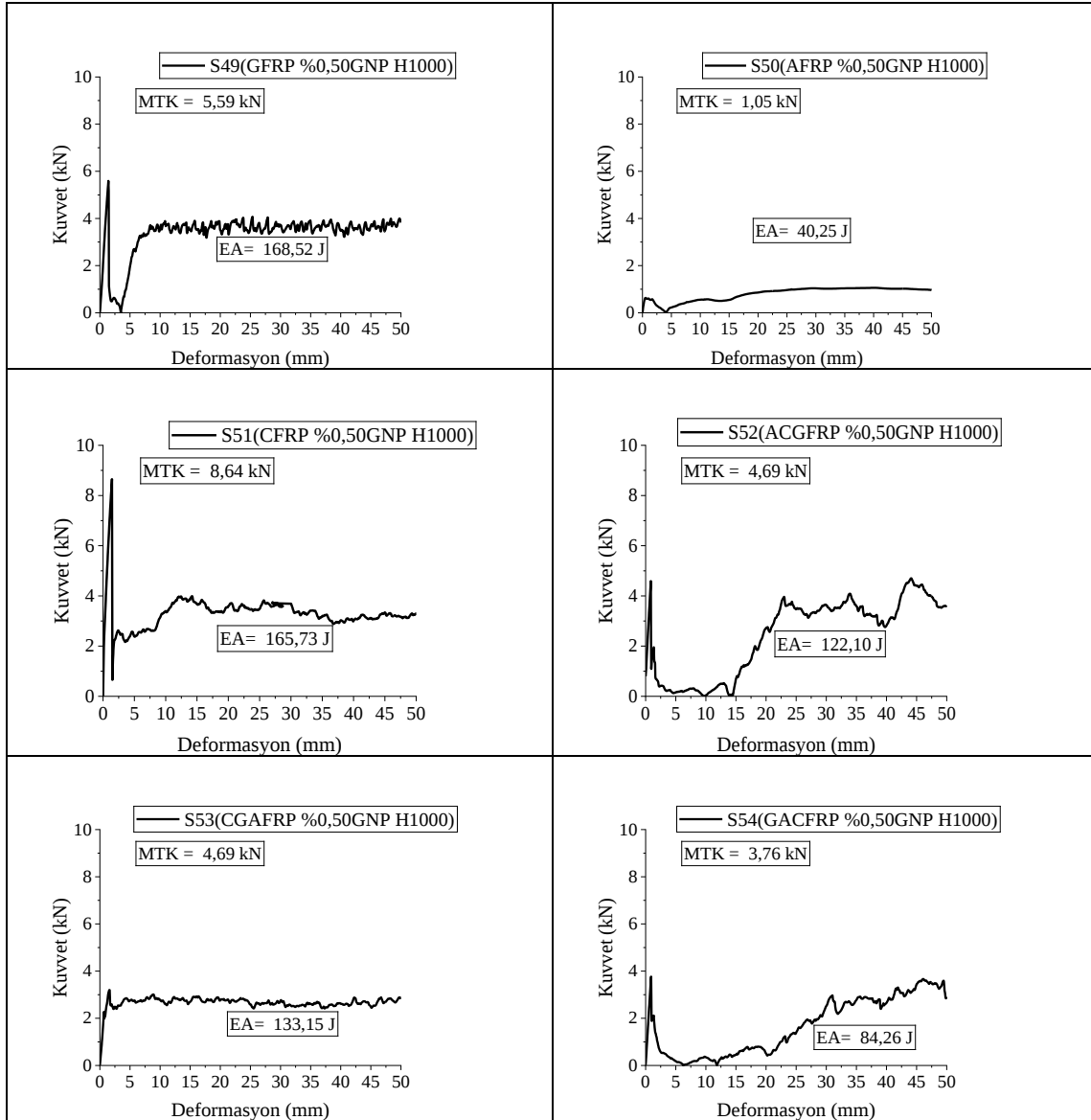
Şekil 4.33. %0,50 grafen ile takviye edilmiş 1000 saat süreyle hidrotermal olarak yaşlandırılmış numunelerin kuvvet-yer değiştirme grafikleri
