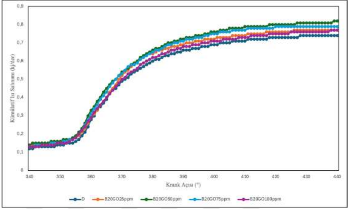
Şekil 15. 1 bar OEB göre krank açısına bağlı Kümülatif Isı Salınımı değişimi
