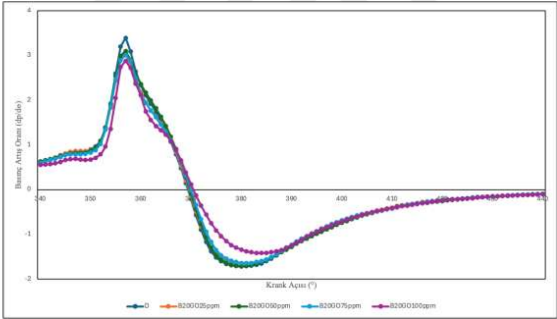
Şekil 21. 3 bar OEB göre krank açısına bağlı Basınç Artış Oranı değişimi ( dp/d\theta )
