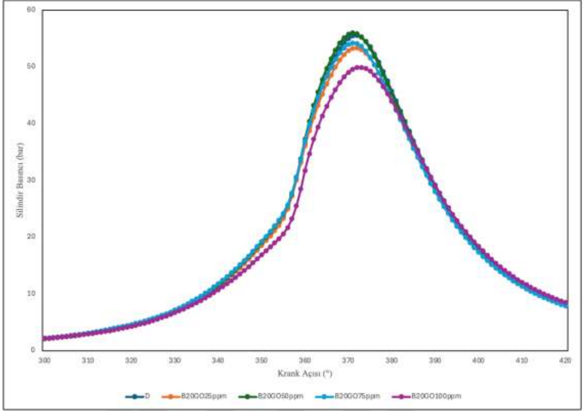
Şekil 9. 3 bar OEB göre krank açısına bağlı silindir basıncı değişimi (bar)
