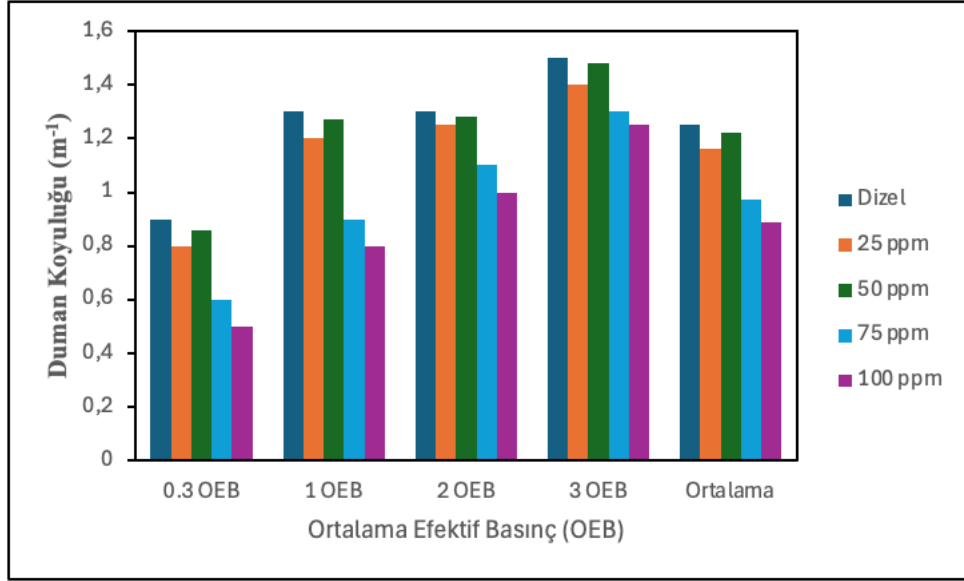
Şekil 25. Duman Koyuluğu
