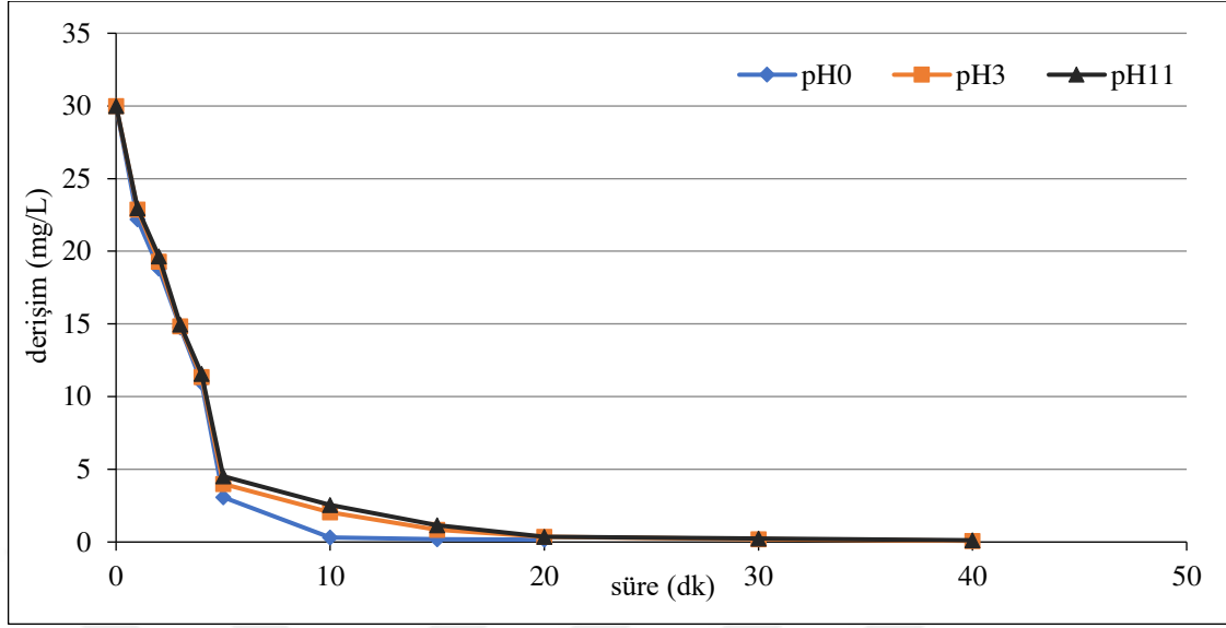
Şekil 6.118. %40IrO 2 -%60RuO 2 kaplı paralel plaka titanyum elektrotlarla, C 0 :30 mg/L, 75 A/m 2 akım yoğunluğunda, 155,84 mL/dk akış hızında, 0,05 M NaCl derişimlerinde, pH 0 (6,05), pH 3 ve pH 11 ’de olan koşullarda elde edilen arıtım verimleri
