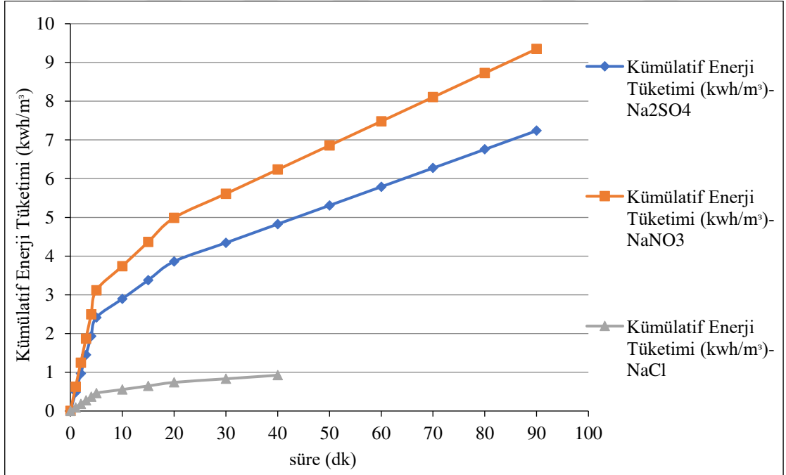
Şekil 6.186. Ti/RuO 2 kaplı paralel plaka elektrotlarla, başlangıç kirlilik derişimi 125 mg/L olduđu durumda Na 2 SO 4 , NaNO 3 ve NaCl elektrolitleri ile optimum kořullarda oluřan enerji tüketim grafięi
