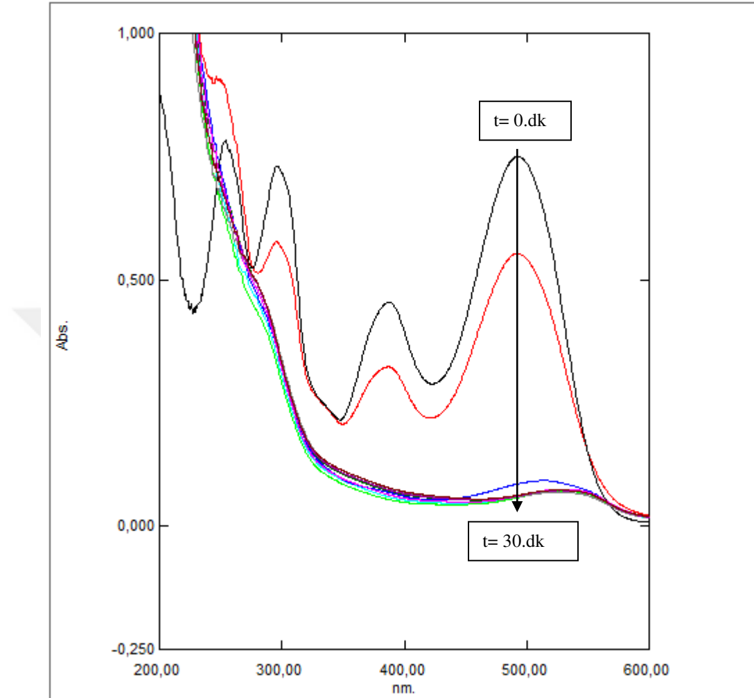
Şekil 6.125. Grafit paralel plaka elektrotlarla, 30 mg/L başlangıç kirlilik derişimi için; 8 A/m 2 akım yoğunluğunda, 155,84 mL/dk akış hızında, 0,01 M \text{Na}_2\text{SO}_4 elektroliti ve 0,5 mL \text{H}_2\text{O}_2 kullanılan pH 11 'de UV-Spektrum grafiğı
