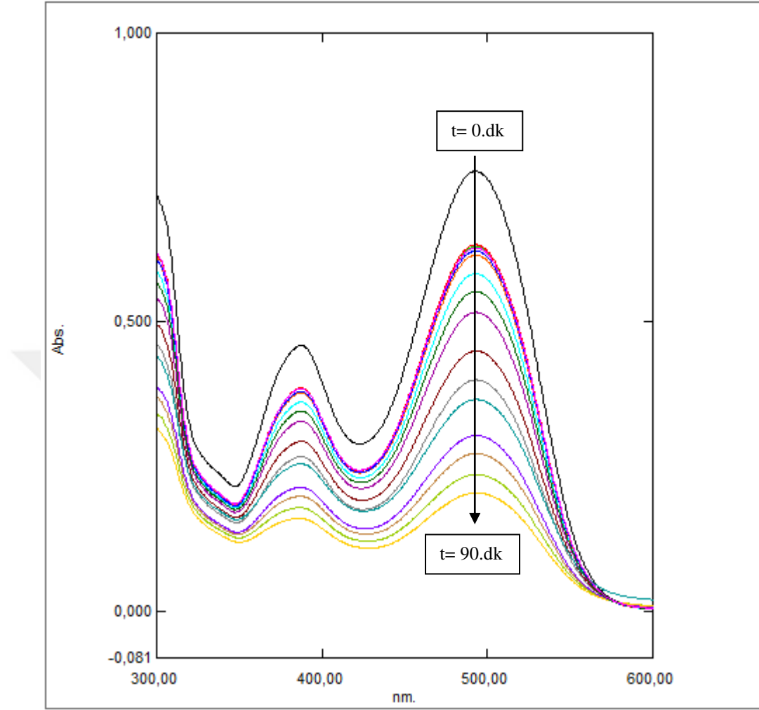
Şekil 6.147. %20IrO 2 -%80RuO 2 kaplı paralel plaka titanyum elektrotlarla, 125 mg/L başlangıç kirlilik derişimi için; 400 A/m 2 akım yoğunluğunda, 155,84 mL/dk akış hızında, 0,01 M NaNO 3 elektrolit miktarı ve pH 0 'de UV-Spektrum grafiğı
