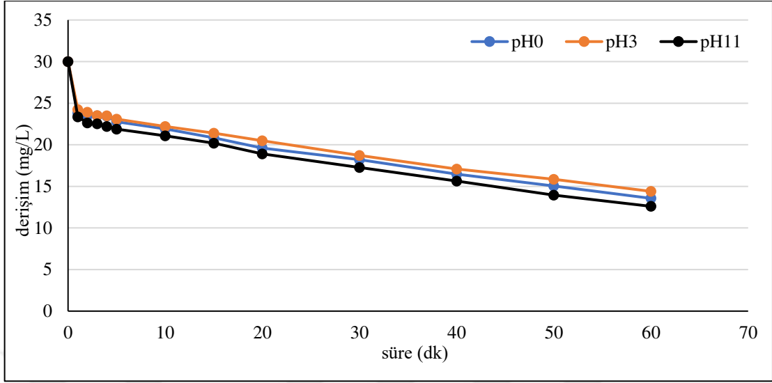
Şekil 6.74. %20IrO 2 -%80RuO 2 kaplı paralel plaka titanyum elektrotlarla, C_0 :30 mg/L, 200 A/m 2 akım yoğunluğunda, 155,84 mL/dk akış hızında, 0,01 M Na_2SO_4 derişiminde, pH 0 (6,15), pH 3 ve pH 11 'de olan koşullarda elde edilen arıtım verimleri
