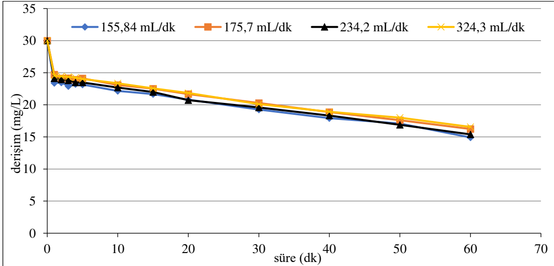
Şekil 6.44. Ti/RuO 2 kaplı paralel plaka elektrotlarla, C 0 :30 mg/L, 150 A/m 2 akım yoğunluğu, 155,84 mL/dk, 175,7 mL/dk, 234,2 mL/dk, 324,3 mL/dk akış hızlarında, 0,01 M NaNO 3 , pH 0 : 6,31-6,80 aralığında olan koşullarda elde edilen arıtım verimleri
