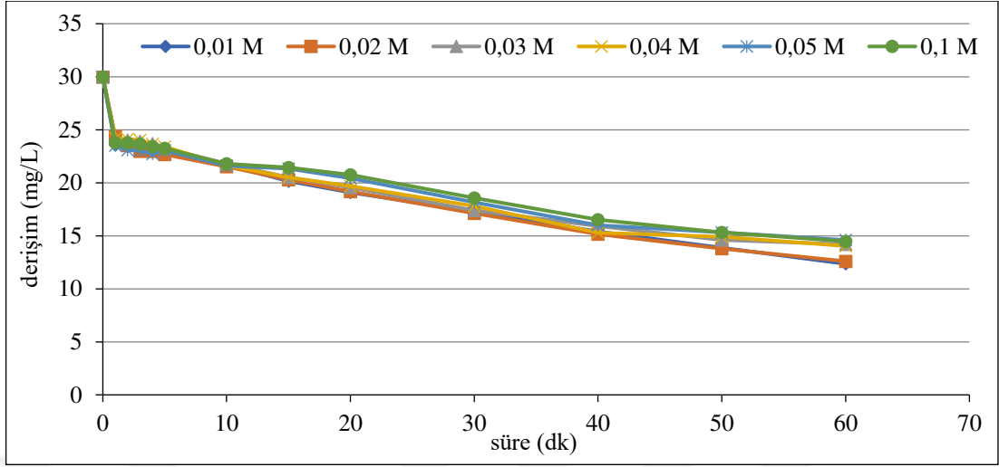
Şekil 6.89. %60IrO 2 -%40RuO 2 kaplı paralel plaka titanyum elektrotlarla, C_0 :30 mg/L, 400 A/m 2 akım yoğunluğunda, 155,84 mL/dk akış hızında, 0,01/0,02/0,03/0,04/0,05/0,1 M \text{Na}_2\text{SO}_4 derişimlerinde, pH 0 : 6,09-6,16 aralığında olan koşullarda elde edilen arıtım verimleri
