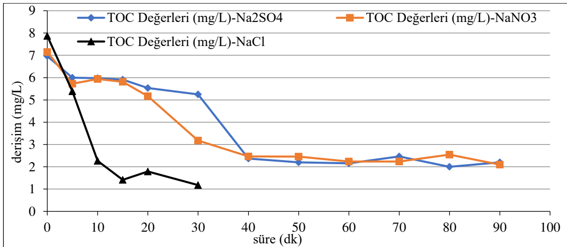
Şekil 6.167. %80IrO 2 -%20RuO 2 kaplı paralel plaka titanyum elektrotlarla, başlangıç kirlilik derişimi 30 mg/L, 200 A/m 2 akım yoğunluğu, 155,84 mL/dk hızı, 0,02 M Na 2 SO 4 elektrolit derişimi, pH 11 : 11'de; 400 A/m 2 akım yoğunluğu, 155,84 mL/dk akış hızı, 0,01 M NaNO 3 elektrolit derişimi, pH 0 'da; 75 A/m 2 akım yoğunluğu, 155,84 mL/dk akış hızı, 0,05 M NaCl elektrolit derişimi, pH 0 olan koşullarda elde edilen TOC sonuçları
