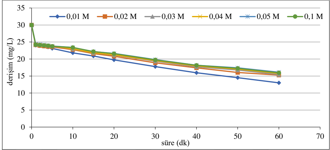
Şekil 6.106. %40IrO 2 -%60RuO 2 kaplı paralel plaka titanyum elektrotlarla, C o :30 mg/L, 300 A/m 2 akım yoğunluğunda, 155,84 mL/dk akış hızında, 0,01/0,02/0,03/0,04/0,05/0,1 M Na 2 SO 4 derişiminde, pH 0 : 6,11-6,16 aralığında olan koşullarda elde edilen arıtım verimleri
