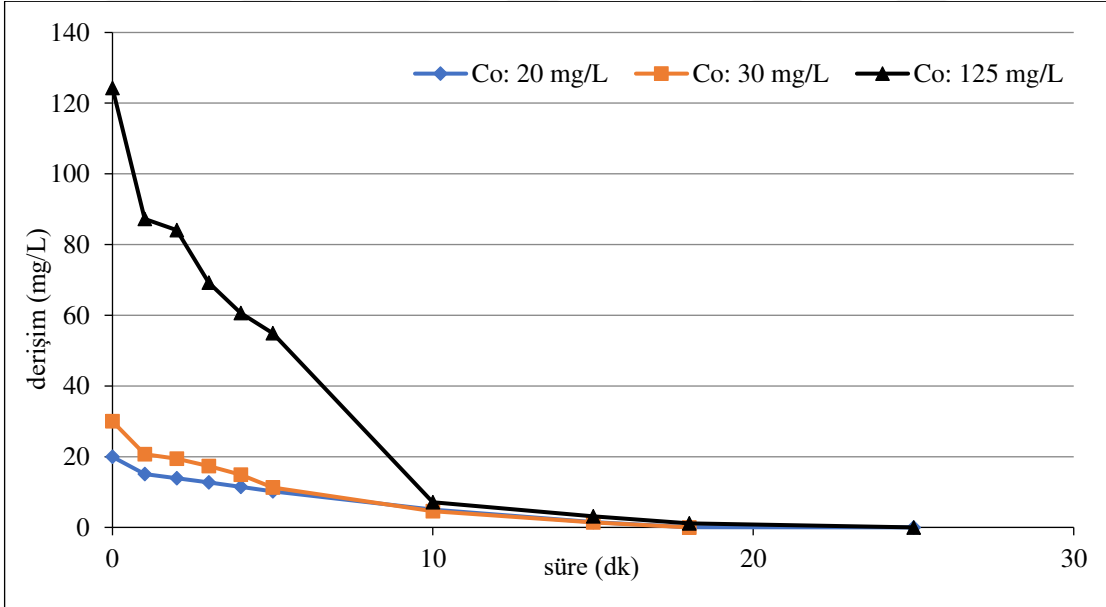
Şekil 6.34. Ti/IrO 2 kaplı paralel plaka elektrotlarla, 50 A/m 2 akım yoğunluğunda, 175,7 mL/dk akış hızında, başlangıç kirlilik derişimi 20 mg/L, 30 mg/L ve 125 mg/L, 0,05 M NaCl elektrolit derişimlerinde, pH 0 : 5,71-5,94'teki koşullarda elde edilen arıtım verimleri
