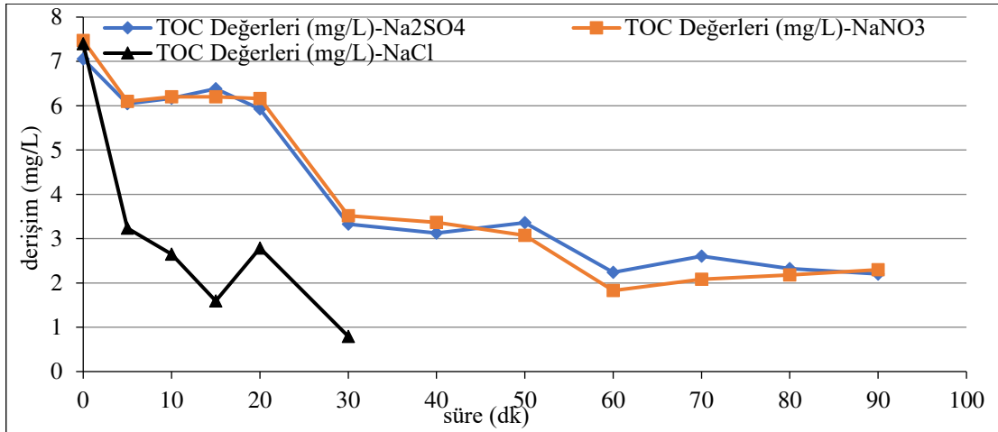
Şekil 6.169. %20IrO 2 -%80RuO 2 kaplı paralel plaka titanyum elektrotlarla, başlangıç kirlilik derişimi 30 mg/L, 200 A/m 2 akım yoğunluğu, 155,84 mL/dk akış hızı, 0,01 M Na 2 SO 4 elektrolit derişimi, pH 11 : 11'de; 400 A/m 2 akım yoğunluğu, 155,84 mL/dk akış hızı, 0,01 M NaNO 3 elektrolit derişimi, pH 0 'da; 75 A/m 2 akım yoğunluğu, 155,84 mL/dk akış hızı, 0,04 M NaCl elektrolit derişimi, pH 0 olan koşullarda elde edilen TOC sonuçları
