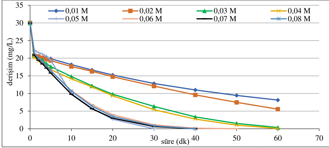
Şekil 6.31. Ti/IrO 2 kaplı paralel plaka elektrotlarla, C o :30 mg/L, 50 A/m 2 akım yoğunluğunda, 155,84 mL/dk akış hızında, 0,01/0,02/0,03/0,04/0,05/0,06/0,07/0,08 M NaCl elektrolit derişimlerinde, pH 0 koşullarında elde edilen arıtım verimleri
