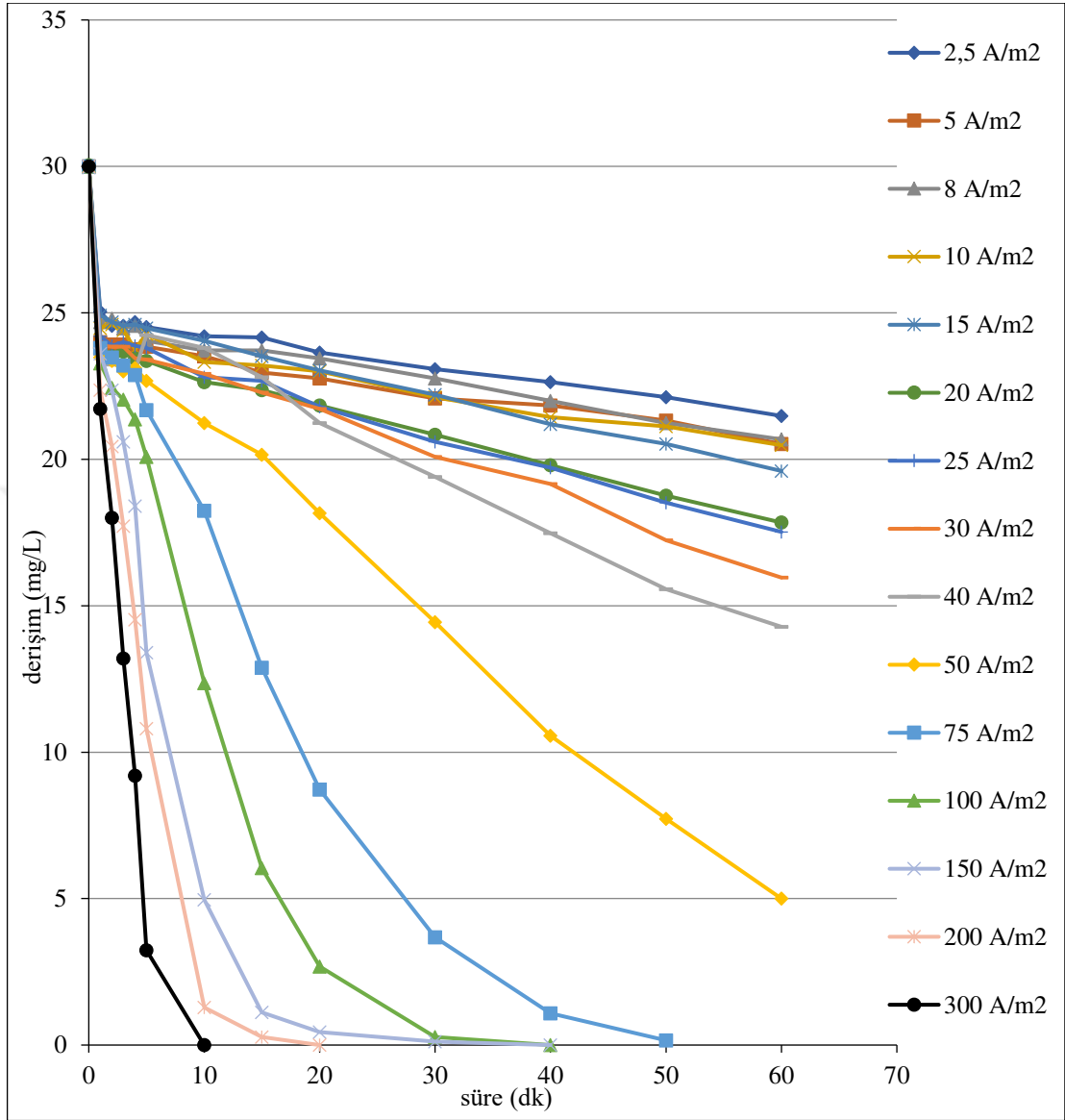
Şekil 6.64. %80IrO 2 -%20RuO 2 kaplı paralel plaka titanyum elektrotlarla, C o :30 mg/L, 2,5/5/8/10/15/20/25/30/40/50/75/100/150/200/300 A/m 2 akım yoğunluklarında, 155,84 mL/dk akış hızında, 0,01 M NaCl, pH 0 : 5,81-6,33 aralığında olan koşullarda elde edilen arıtım verimleri
