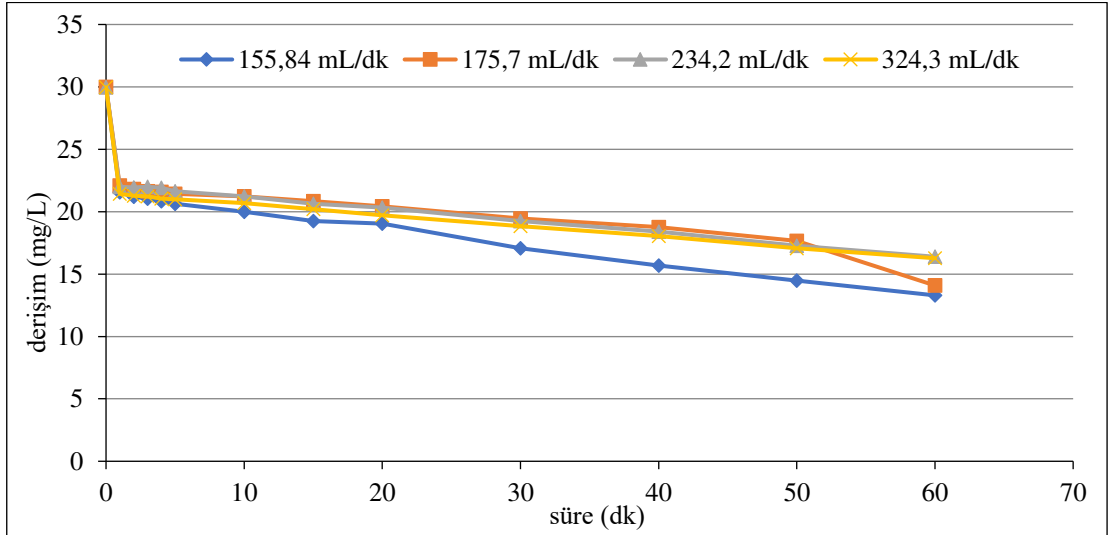
Şekil 6.22. Ti/IrO 2 kaplı paralel plaka elektrotlarla, C 0 :30 mg/L, 50 A/m 2 akım yoğunluğu, 155,84 mL/dk, 175,7 mL/dk, 234,2 mL/dk, 324,3 mL/dk akış hızlarında, 0,01 M Na 2 SO 4 , pH 11 olan koşullarda elde edilen arıtım verimleri
