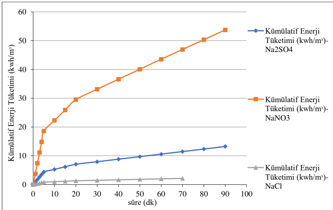
Şekil 6.190. %20IrO 2 -%80RuO 2 kaplı paralel plaka titanyum elektrotlarla, başlangıç kirlilik derişimi 125 mg/L olduđu durumda Na 2 SO 4 , NaNO 3 ve NaCl elektrolitleri ile optimum kořullarda oluřan enerji tüketim grafiđi
