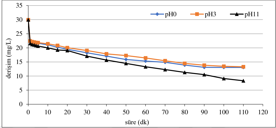
Şekil 6.23. \text{Ti}/\text{IrO}_2 kaplı paralel plaka elektrotlarla, C_0 :30 mg/L, 50 \text{ A/m}^2 akım yoğunluğunda, 155,84 \text{ mL/dk} akış hızında, 0,01 \text{ M Na}_2\text{SO}_4 derişiminde, \text{pH}_0 (6,90), \text{pH}_3 ve \text{pH}_{11} 'de olan koşullarda elde edilen arıtım verimleri
