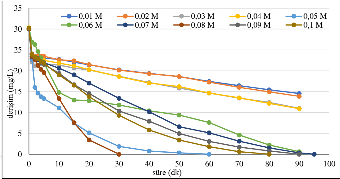
Şekil 6.14. Grafit plaka elektrotlarla, Co:30 mg/L, 155,84 mL/dk akış hızı, 40 A/m 2 akım yoğunluğu, başlangıç pH 0 : 6,08-6,72 arasında, 0,01 M/ 0,02 M/ 0,03 M/ 0,04 M/ 0,05 M/ 0,06 M/ 0,07 M/ 0,08 M/ 0,09 M/ 0,1 M NaCl elektroliti kullanılan koşullarda arıtım verimleri
