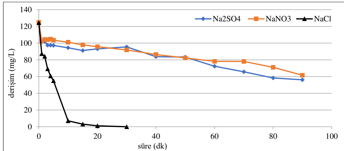
Şekil 6.36. \text{Ti}/\text{IrO}_2 kaplı paralel plaka elektrotlarla, C_0 :125 mg/L \text{Na}_2\text{SO}_4 için; 50 \text{ A/m}^2 akım yoğunluğu, 155,84 mL/dk akış hızı, 0,01 M \text{Na}_2\text{SO}_4 elektrolit miktarı, \text{pH}_{11} olan koşullarda; \text{NaNO}_3 için; 50 \text{ A/m}^2 akım yoğunluğu, 155,84 mL/dk akış hızı, 0,01 M \text{NaNO}_3 elektrolit miktarı, \text{pH}_0 (6,36) olan koşullarda, \text{NaCl} için; 50 \text{ A/m}^2 akım yoğunluğu, 175,7 mL/dk akış hızı, 0,05 M \text{NaCl} elektrolit miktarı, \text{pH}_0 (6,15) olan koşullarda elde edilen arıtım verimleri
