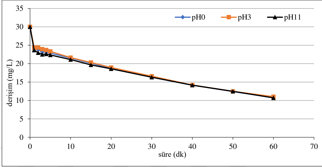
Şekil 6.79. %20 \text{IrO}_2 -%80 \text{RuO}_2 kaplı paralel plaka titanyum elektrotlarla, C_0 :30 mg/L, 400 \text{ A/m}^2 akım yoğunluğunda, 155,84 \text{ mL/dk} akış hızında, 0,01 \text{ M NaNO}_3 derişiminde, \text{pH}_0 (6,20), \text{pH}_3 ve \text{pH}_{11} 'de olan koşullarda elde edilen arıtım verimleri
