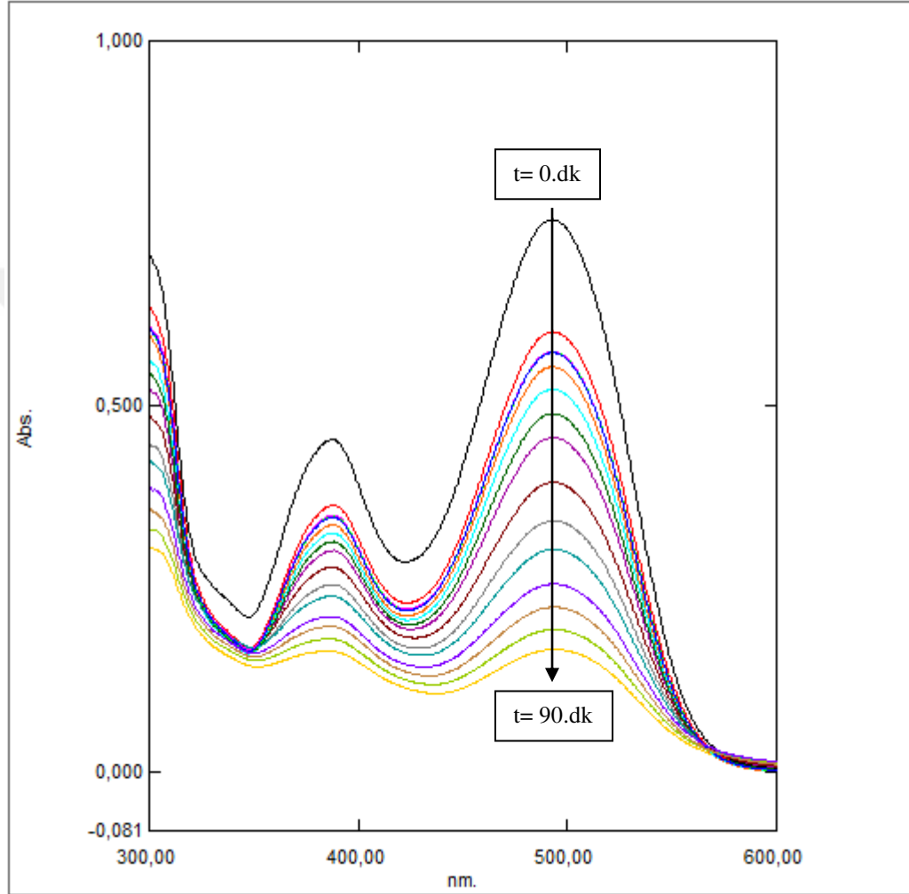
Şekil 6.158. %40IrO 2 -%60RuO 2 kaplı paralel plaka titanyum elektrotlarla, 30 mg/L başlangıç kirlilik derişimi için; 500 A/m 2 akım yoğunluğunda, 155,84 mL/dk akış hızında, 0,01 M NaNO 3 elektrolit miktarı ve pH 0 'da UV-Spektrum grafiği
