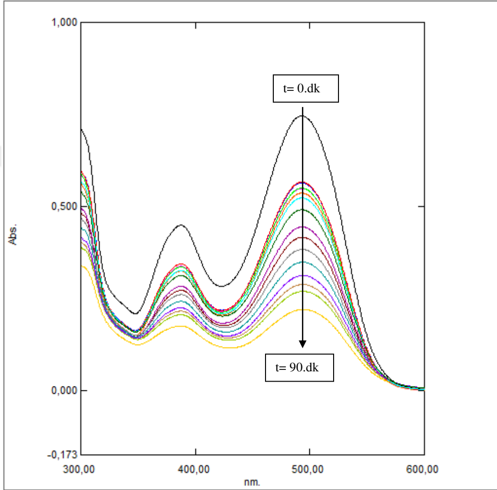
Şekil 6.140. %80IrO 2 -%20RuO 2 kaplı paralel plaka titanyum elektrotlarla, 30 mg/L başlangıç kirlilik derişimi için; 400 A/m 2 akım yoğunluğunda, 155,84 mL/dk akış hızında, 0,01 M NaNO 3 elektrolit miktarı ve pH 0 'de UV-Spektrum grafiğı
