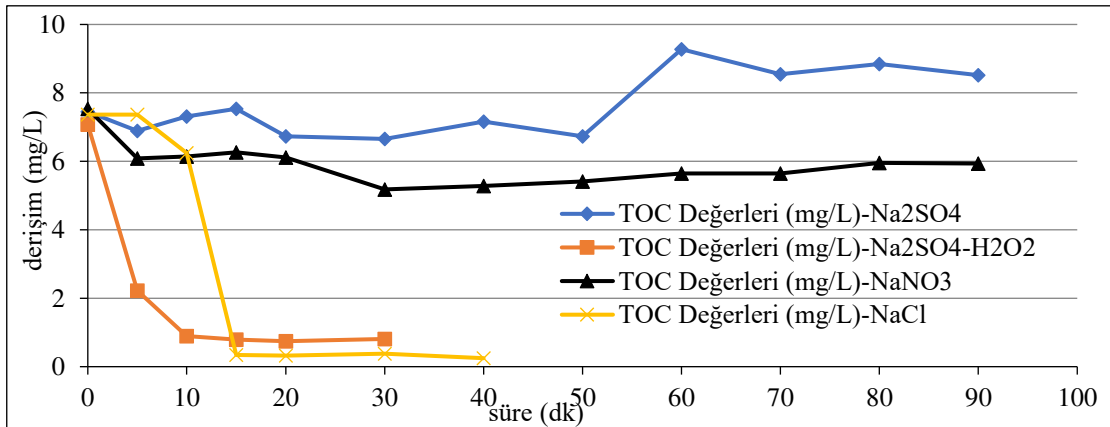
Şekil 6.162. Grafit elektrotlarla, başlangıç kirlilik derişimi 30 mg/L, 8 A/m 2 akım yoğunluğu, 155,84 mL/dk akış hızı, 0,01 M Na 2 SO 4 elektrolit derişimi, pH 11 : 11'de; 8 A/m 2 akım yoğunluğu, 155,84 mL/dk akış hızı, 0,01 M Na 2 SO 4 -0,5 mL H 2 O 2 pH 11'de; 8 A/m 2 akım yoğunluğu, 155,84 mL/dk akış hızı, 0,01 M NaNO 3 elektrolit derişimi, pH 0 'da; 40 A/m 2 akım yoğunluğu, 155,84 mL/dk akış hızı, 0,08 M NaCl elektrolit derişimi, pH 0 olan koşullarda elde edilen TOC sonuçları
