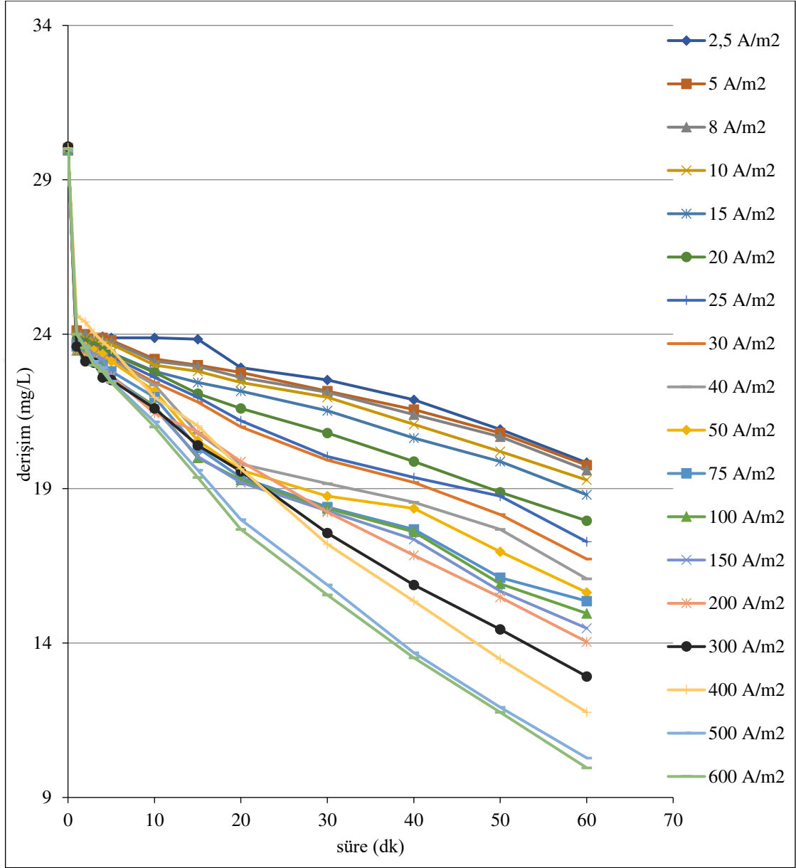
Şekil 6.110. \%40\text{IrO}_2 - \%60\text{RuO}_2 kaplı paralel plaka titanyum elektrotlarla, C_0 :30 mg/L, 2,5/5/8/10/15/20/25/30/40/50/75/100/150/200/300/400/500/600 \text{A/m}^2 akım yoğunluklarında, 155,84 mL/dk akış hızında, 0,01 M \text{NaNO}_3 , \text{pH}_0 : 6,14-6,36 aralığında olan koşullarda elde edilen arıtım verimleri
