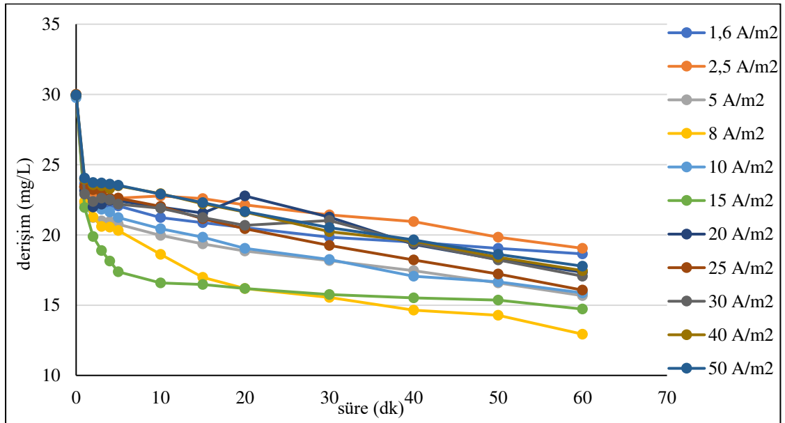
Şekil 6.8. Grafit plaka elektrotlarla, C 0 :30 mg/L, 175,7 mL/dk akış hızında 1,6/2,5/5/8/10/15/20/25/30/40/50 A/m 2 akım yoğunluğu, başlangıç pH 0 : 8,55, 0,01 M NaNO 3 kullanılan koşullarda arıtım verimleri
