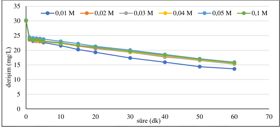
Şekil 6.38. \text{Ti/RuO}_2 kaplı paralel plaka elektrotlarla, C_o :30 mg/L, 150 \text{ A/m}^2 akım yoğunluğunda, 155,84 mL/dk akış hızında, 0,01/0,02/0,03/0,04/0,05/0,1 M \text{Na}_2\text{SO}_4 derişimlerinde, \text{pH}_0 : 6,78-6,97 aralığında olan koşullarda elde edilen arıtım verimleri
