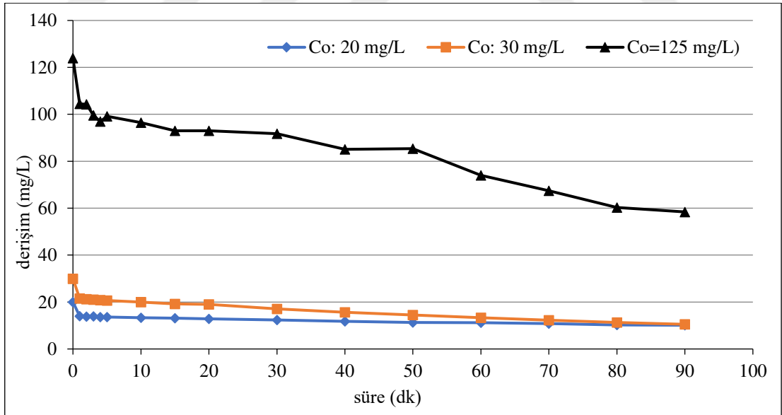
Şekil 6.24. \text{Ti}/\text{IrO}_2 kaplı paralel plaka elektrotlarla, C_0 :30 mg/L, 50 \text{ A/m}^2 akım yoğunluğunda, 155,84 \text{ mL/dk} akış hızında, başlangıç kirlilik derişimi 20 mg/L, 30 mg/L ve 125 mg/L, 0,01 \text{ M Na}_2\text{SO}_4 elektrolit derişiminde, \text{pH}_{11} 'deki koşullarda elde edilen arıtım verimleri
