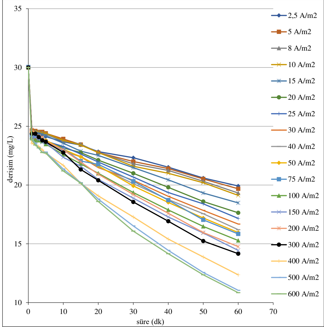
Şekil 6.88. %60IrO 2 -%40RuO 2 kaplı paralel plaka titanyum elektrotlarla, C_o :30 mg/L, 2,5/5/8/10/15/20/25/30/40/50/75/100/150/200/300/400/500/600 A/m 2 akım yoğunluklarında, 155,84 mL/dk akış hızında, 0,01 M Na 2 SO 4 , pH 0 : 6,01-6,31 aralığında olan koşullarda elde edilen arıtım verimleri
