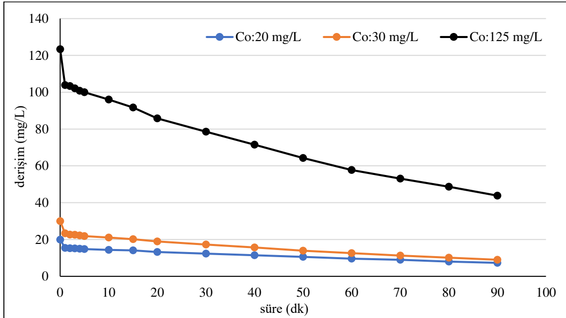
Şekil 6.75. %20IrO 2 -%80RuO 2 kaplı paralel plaka titanyum elektrotlarla, 200 A/m 2 akım yoğunluğunda, 155,84 mL/dk akış hızında, başlangıç kirlilik derişimleri 20 mg/L, 30 mg/L ve 125 mg/L olan 0,01 M Na_2SO_4 elektrolit derişiminde, pH 11 olan koşullarda elde edilen arıtım verimleri
