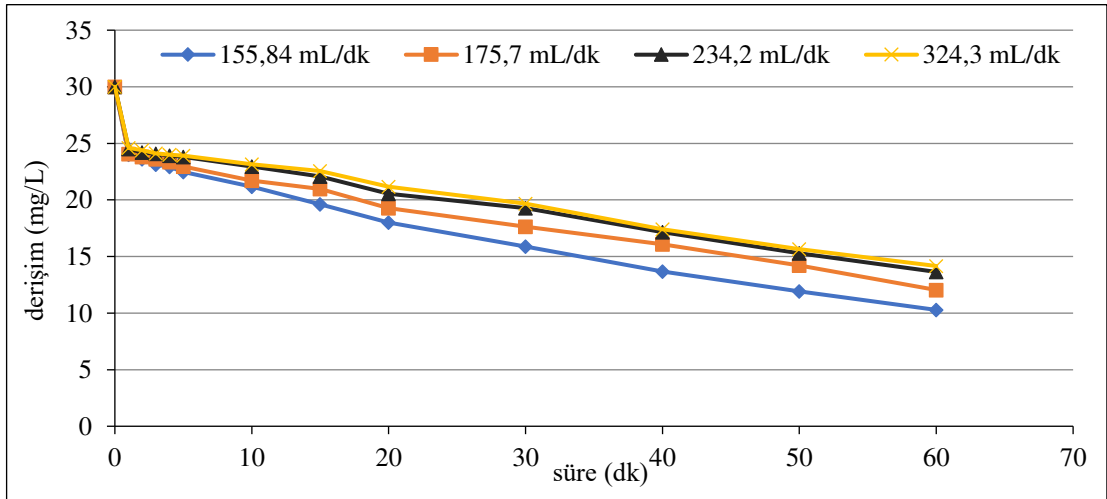
Şekil 6.112. %40 \text{IrO}_2 -%60 \text{RuO}_2 kaplı paralel plaka titanyum elektrotlarla, C_o :30 mg/L, 500 A/m 2 akım yoğunluğu, 155,84 mL/dk, 175,7 mL/dk, 234,2 mL/dk, 324,3 mL/dk akış hızlarında, 0,01 M \text{NaNO}_3 , pH 0 : 6,14-6,21 aralığında olan koşullarda elde edilen arıtım verimleri
