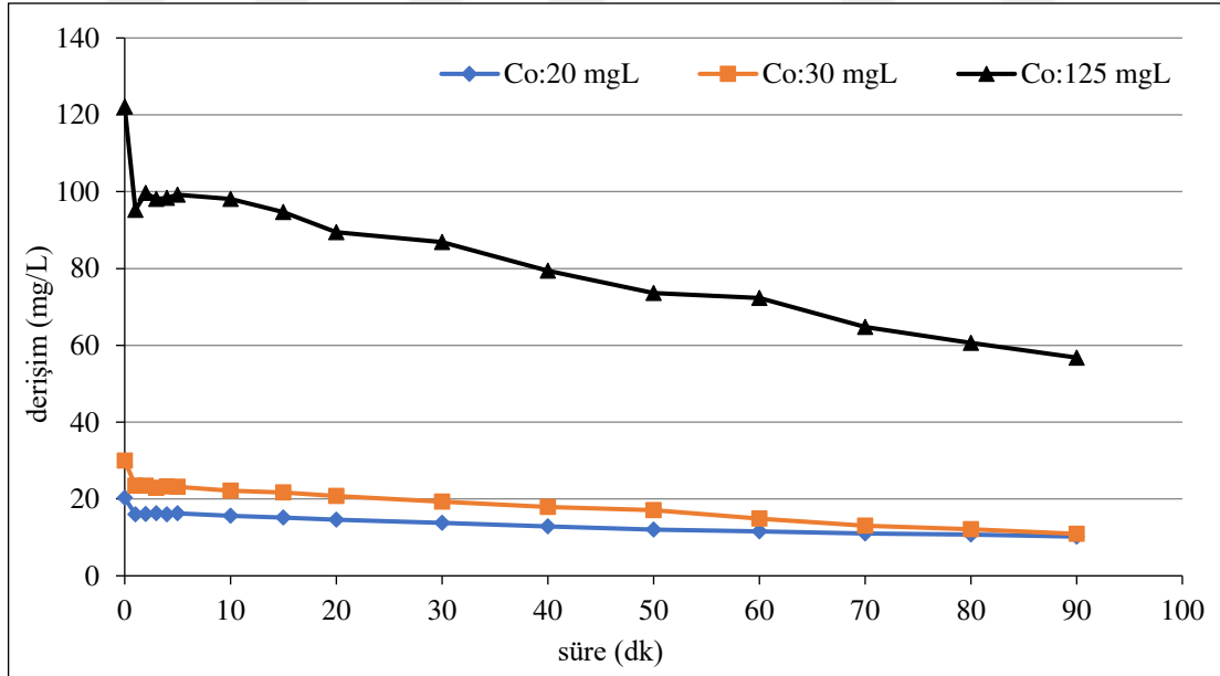
Şekil 6.46. \text{Ti/RuO}_2 kaplı paralel plaka elektrotlarla, 150 \text{ A/m}^2 akım yoğunluğunda, 155,84 \text{ mL/dk} akış hızında, başlangıç kirlilik derişimi 20 mg/L, 30 mg/L ve 125 mg/L olan 0,01 \text{ M NaNO}_3 elektrolit derişiminde, \text{pH}_0 : 6,46-6,66 aralığında olan koşullarda elde edilen arıtım verimleri
