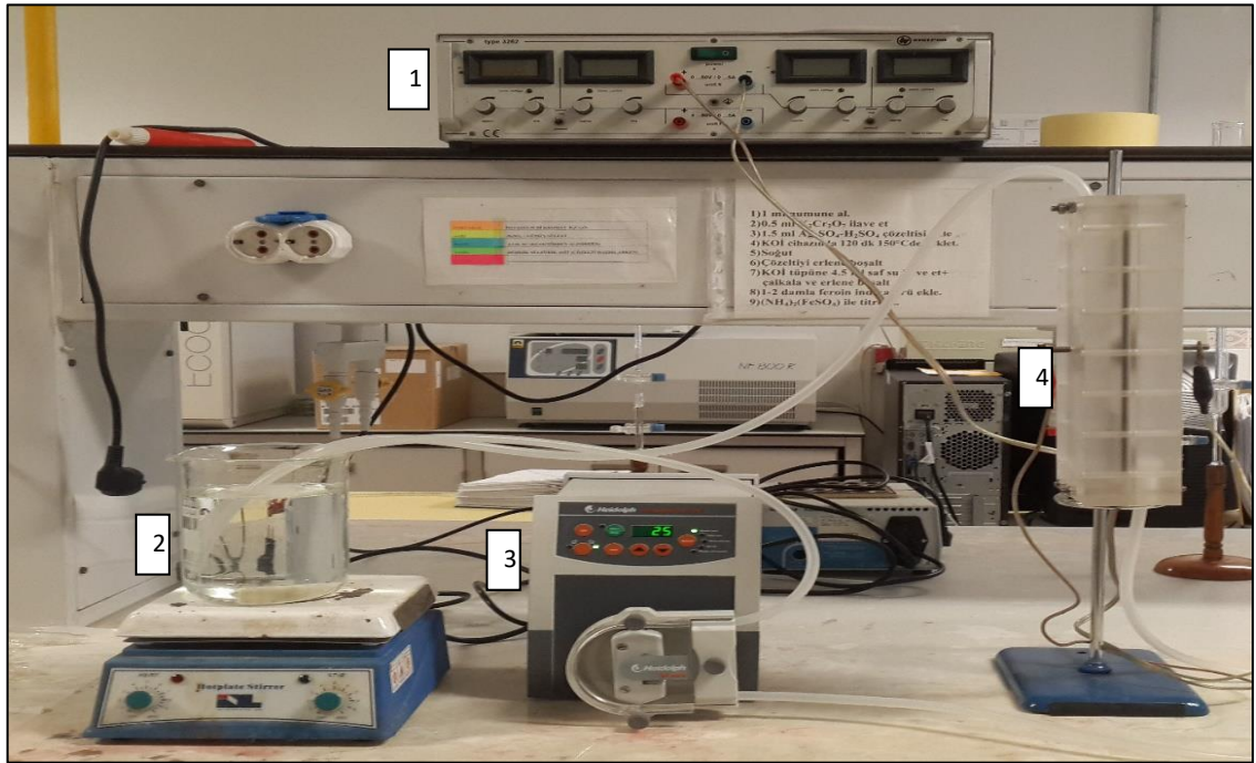
Görsel 5.1. 1, güç kaynağı (Statron Power Supply); 2, kontrollü karıştırıcı ve çalışma için kullanılan çözelti kabı; 3, pompa (Heidolph pump drive 5206); 4, plaka anot ve katot yerleşmeli paralel plaka
