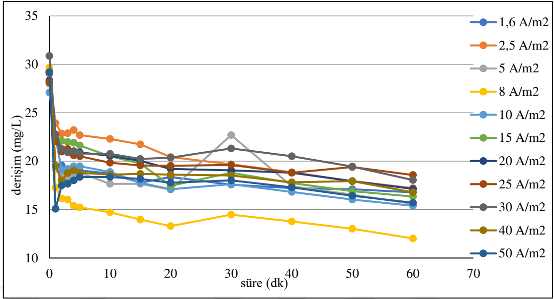
Şekil 6.3. Grafit plaka elektrotlarla, C_0 :30 mg/L, 1,6/2,5/5/8/10/15/20/25/30/40/50 A/m 2 akım yoğunluğu, 155,84 mL/dk akış hızı, başlangıç pH 11 , 0,01 M Na 2 SO 4 kullanılan koşullarda arıtım verimleri
