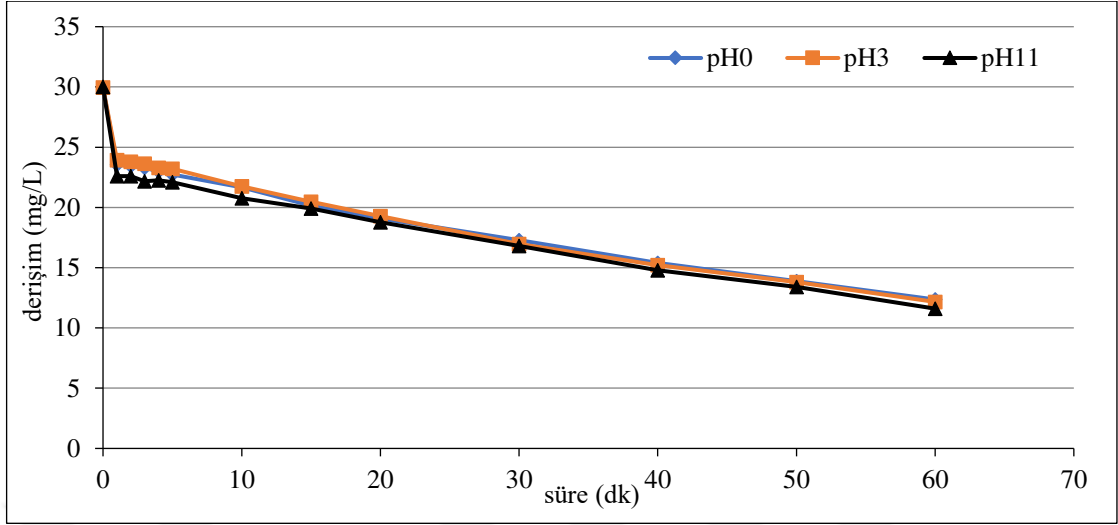
Şekil 6.91. %60IrO 2 -%40RuO 2 kaplı paralel plaka titanyum elektrotlarla, C_0 :30 mg/L, 400 A/m 2 akım yoğunluğunda, 155,84 mL/dk akış hızında, 0,01 M \text{Na}_2\text{SO}_4 derişiminde, pH 0 (6,11), pH 3 ve pH 11 'de olan koşullarda elde edilen arıtım verimleri
