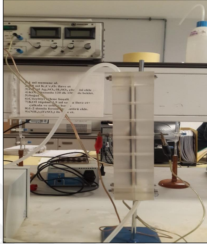
Görsel 5.2. Elektrotların yerleştirildiği paralel plaka düzeneği
