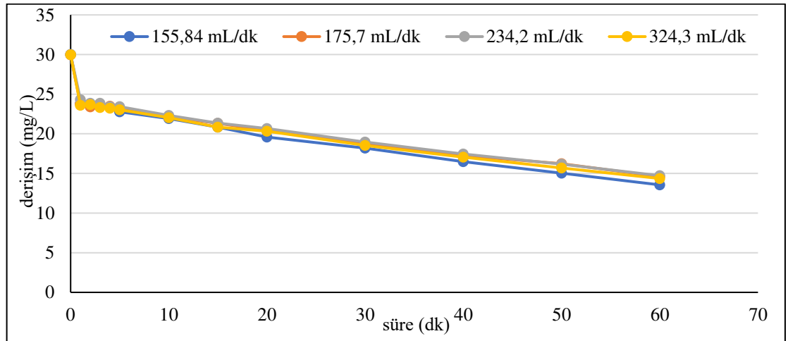
Şekil 6.73. %20 \text{IrO}_2 -%80 \text{RuO}_2 kaplı paralel plaka titanyum elektrotlarla, C_0 :30 mg/L, 200 \text{A/m}^2 akım yoğunluğu, 155,84 mL/dk, 175,7 mL/dk, 234,2 mL/dk, 324,3 mL/dk akış hızlarında, 0,01 M \text{Na}_2\text{SO}_4 , \text{pH}_0 : 5,79-6,15 aralığında olan koşullarda elde edilen arıtım verimleri
