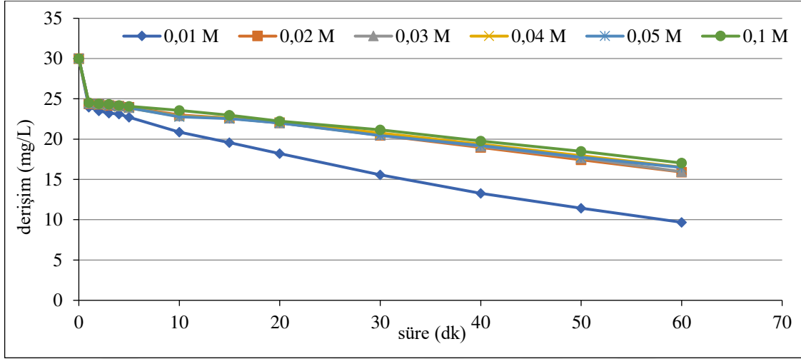
Şekil 6.94. %60IrO 2 -%40RuO 2 kaplı paralel plaka titanyum elektrotlarla, C 0 :30 mg/L, 500 A/m 2 akım yoğunluğunda, 155,84 mL/dk akış hızında, 0,01/0,02/0,03/0,04/0,05/0,1 M NaNO 3 derişimlerinde, pH 0 : 6,18-6,22 aralığında olan koşullarda elde edilen arıtım verimleri
