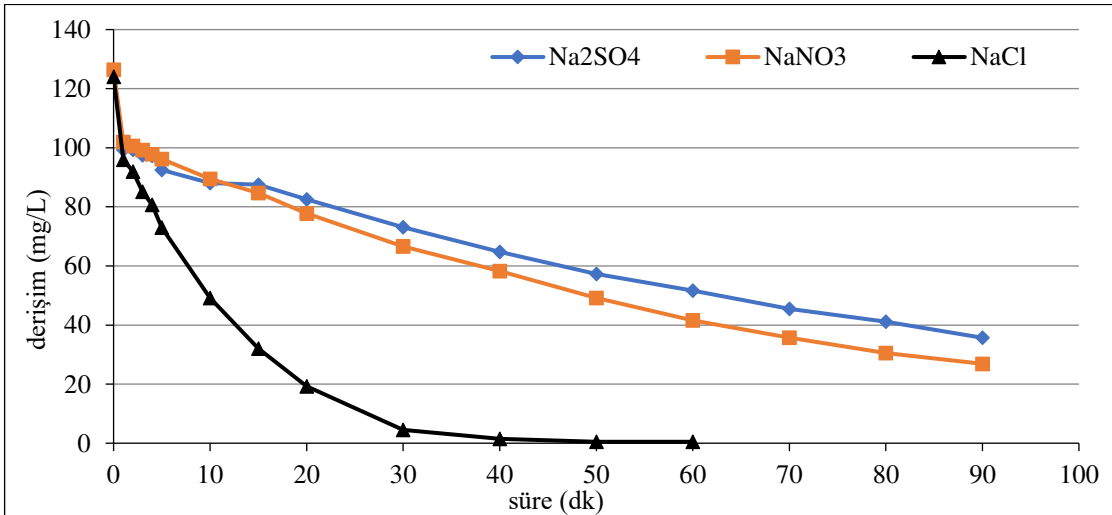
Şekil 6.104. %60 \text{IrO}_2 -%40 \text{RuO}_2 kaplı paralel plaka titanyum elektrotlarla, C_0 :125 mg/L \text{Na}_2\text{SO}_4 için; 400 \text{A/m}^2 akım yoğunluğu, 155,84 mL/dk akış hızı, 0,01 M \text{Na}_2\text{SO}_4 elektrolit miktarı, \text{pH}_{11} olan koşullarda; \text{NaNO}_3 için; 500 \text{A/m}^2 akım yoğunluğu, 155,84 mL/dk akış hızı, 0,01 M \text{NaNO}_3 elektrolit miktarı, \text{pH}_0 (5,80) olan koşullarda, \text{NaCl} için; 75 \text{A/m}^2 akım yoğunluğu, 155,84 mL/dk akış hızı, 0,05 M \text{NaCl} elektrolit miktarı, \text{pH}_0 (6,25) olan koşullarda elde edilen arıtım verimleri
