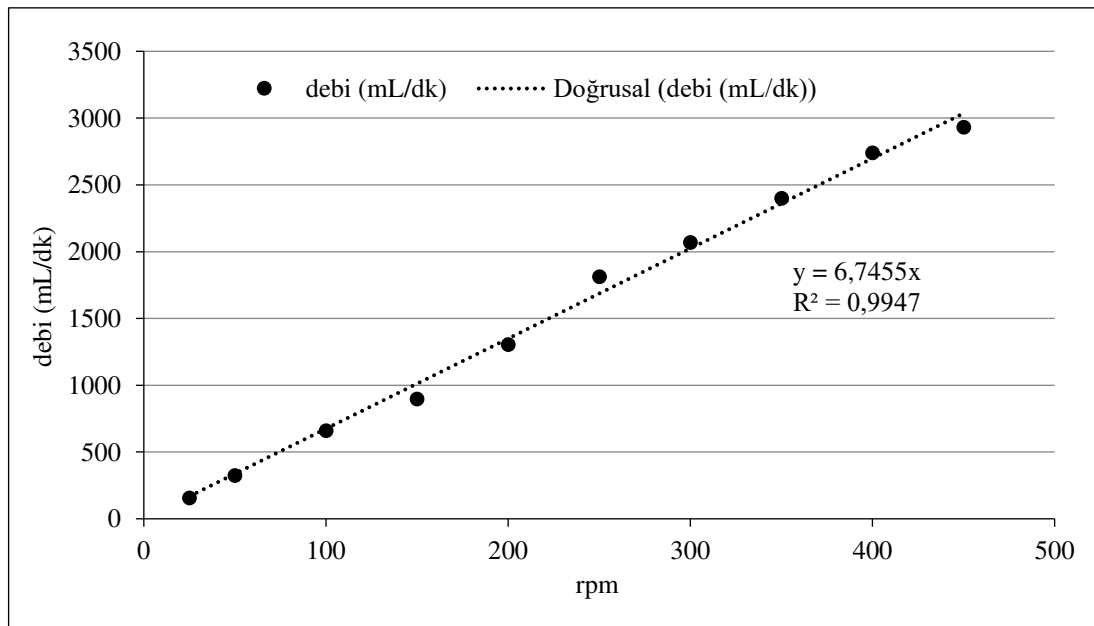
Şekil 6.1. Elektrokimyasal arıtım deney düzeneğinde kullanılan pompanın kalibrasyon eğrisi
