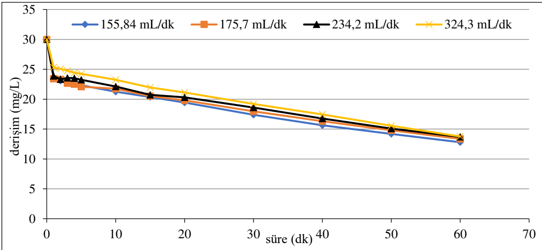
Şekil 6.61. %80 \text{IrO}_2 -%20 \text{RuO}_2 kaplı paralel plaka titanyum elektrotlarla, C_o :30 mg/L, 400 A/m 2 akım yoğunluğu, 155,84 mL/dk, 175,7 mL/dk, 234,2 mL/dk, 324,3 mL/dk akış hızlarında, başlangıç kirlilik derişimi 30 mg/L, 0,01 M \text{NaNO}_3 , \text{pH}_0 : 6,18-6,40 aralığında olan koşullarda elde edilen arıtım verimleri
