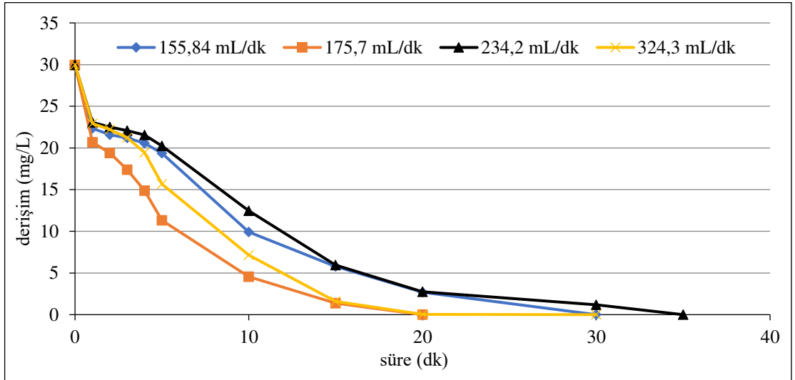
Şekil 6.32. Ti/IrO 2 kaplı paralel plaka elektrotlarla, C o :30 mg/L, 50 A/m 2 akım yoğunluğunda, 155,84 mL/dk, 175,7 mL/dk, 234,2 mL/dk, 324,3 mL/dk akış hızlarında, 0,05 M NaCl, pH 0 : 5,71 olan koşullarda elde edilen arıtım verimleri
