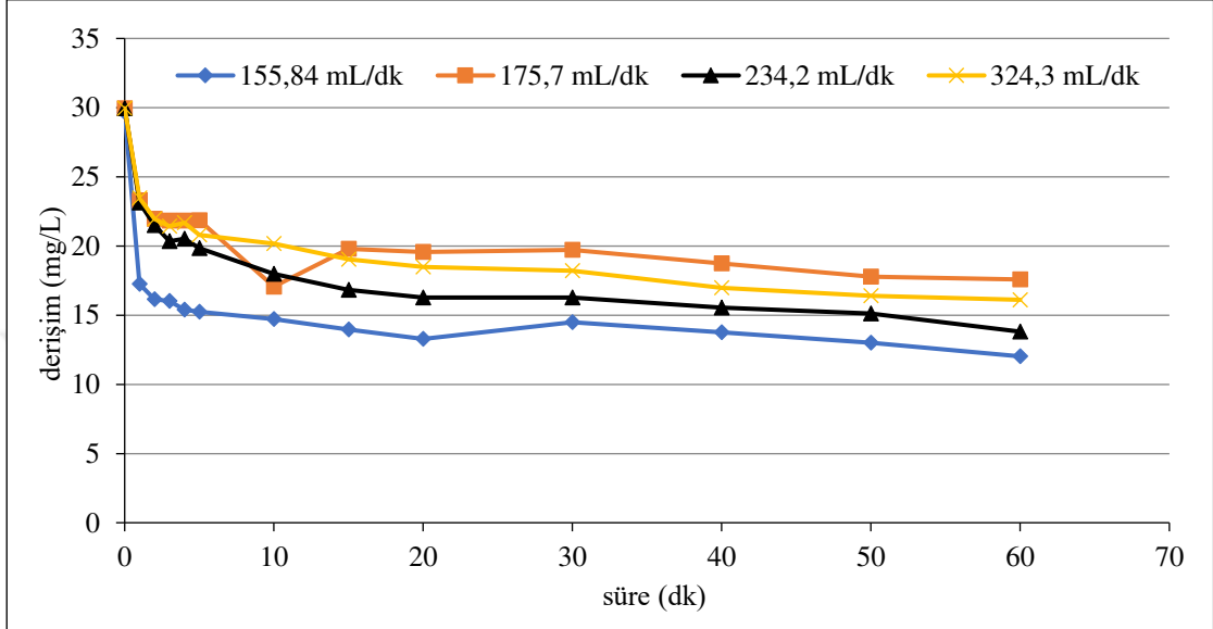
Şekil 6.5. Grafit plaka elektrotlarla, C_0 :30 mg/L, 25, 30, 40, 50 rpm (155,84/175,7/234,2/324,3 mL/dk), 8 A/m 2 akım yoğunluğu, başlangıç pH 11 , 0,01 M Na 2 SO 4 kullanılan koşullarda arıtım verimleri
