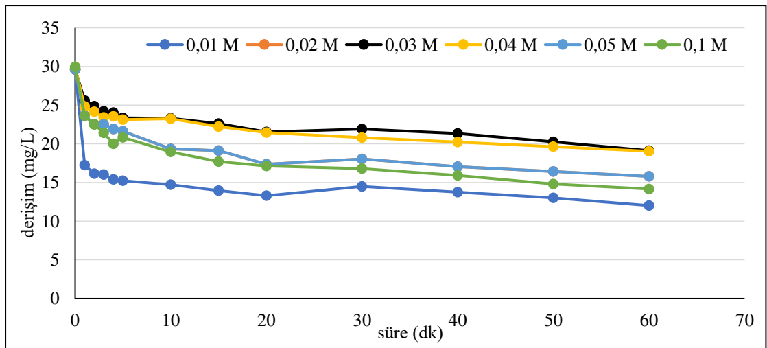
Şekil 6.4. Grafit plaka elektrotlarla, C_0 :30 mg/L, 8 A/m 2 akım yoğunluğu, 155,84 mL/dk akış hızı başlangıç pH 11 , 0,01 M/ 0,02 M/ 0,03 M/ 0,04 M/ 0,05 M/0,1 M Na 2 SO 4 elektroliti kullanılan koşullarda arıtım verimleri
