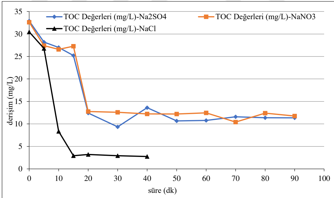
Şekil 6.166. Ti/RuO 2 kaplı paralel plaka elektrotlarla, başlangıç kirlilik derişimi 125 mg/L, 150 A/m 2 akım yoğunluğu, 155,84 mL/dk hızı, 0,01 M Na 2 SO 4 elektrolit derişimi, pH 11 : 11'de; 150 A/m 2 akım yoğunluğu, 155,84 mL/dk akış hızı, 0,01 M NaNO 3 elektrolit derişimi, pH 0 'da; 50 A/m 2 akım yoğunluğu, 155,84 mL/dk akış hızı, 0,06 M NaCl elektrolit derişimi, pH 0 olan koşullarda elde edilen TOC sonuçları
