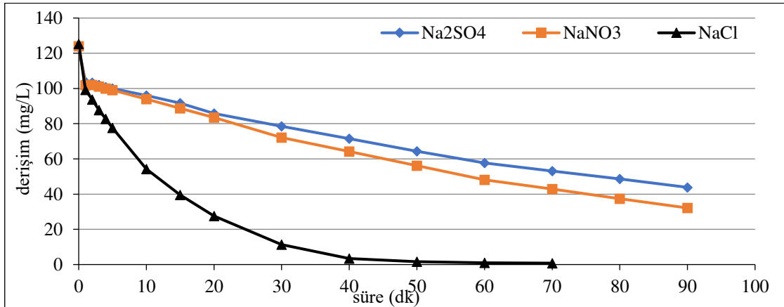
Şekil 6.87. %20 \text{IrO}_2 -%80 \text{RuO}_2 kaplı paralel plaka titanyum elektrotlarla, C_0 :125 mg/L \text{Na}_2\text{SO}_4 için; 200 \text{A/m}^2 akım yoğunluğu, 155,84 mL/dk akış hızı, 0,01 M \text{Na}_2\text{SO}_4 elektrolit miktarı, \text{pH}_{11} olan koşullarda; \text{NaNO}_3 için; 400 \text{A/m}^2 akım yoğunluğu, 155,84 mL/dk akış hızı, 0,01 M \text{NaNO}_3 elektrolit miktarı, \text{pH}_0 (6,31) olan koşullarda, \text{NaCl} için; 75 \text{A/m}^2 akım yoğunluğu, 155,84 mL/dk akış hızı, 0,04 M \text{NaCl} elektrolit miktarı, \text{pH}_0 (6,15) olan koşullarda elde edilen arıtım verimleri
