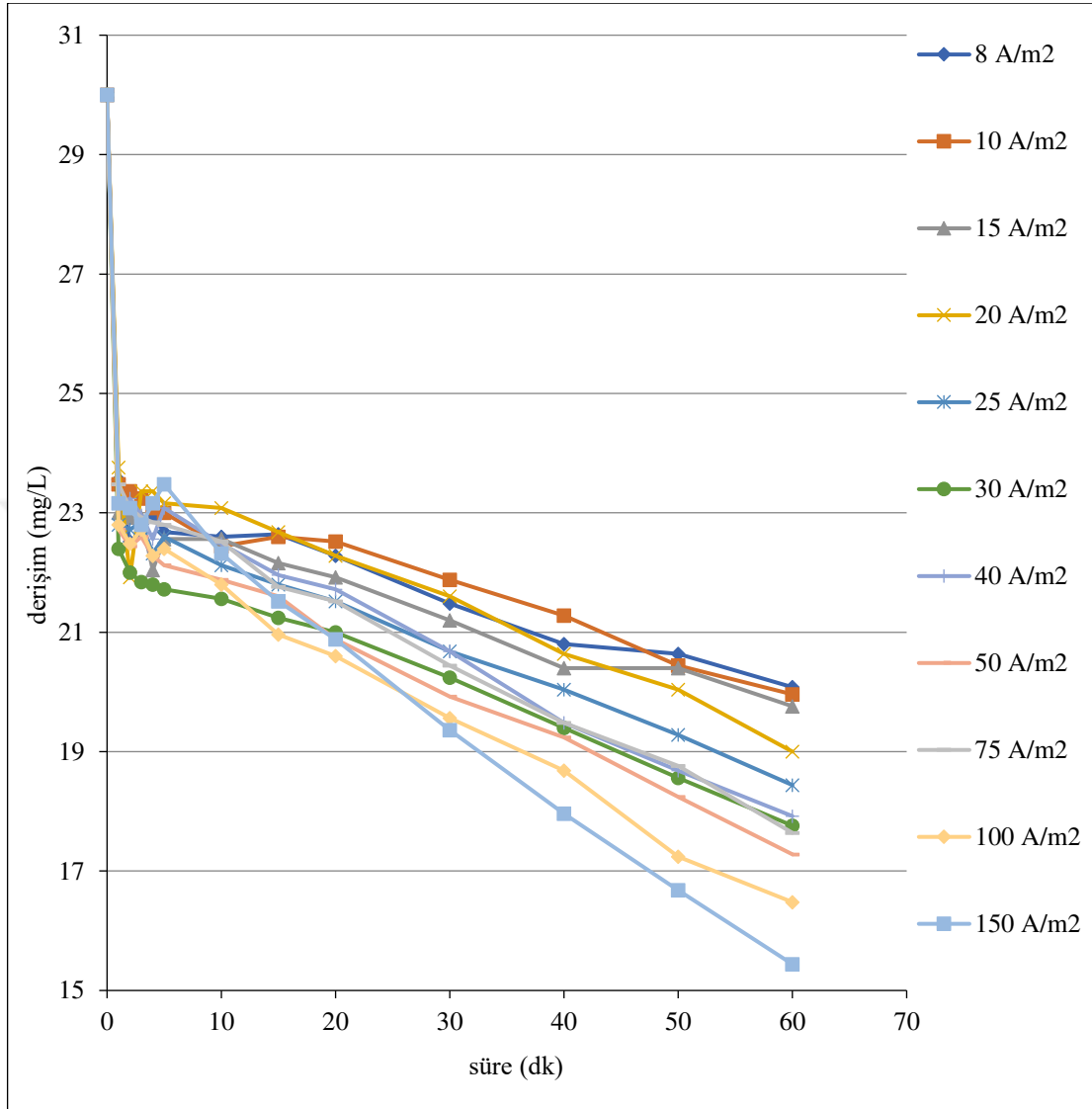
Şekil 6.25. \text{Ti/IrO}_2 kaplı paralel plaka elektrotlarla, C_0 : 30 mg/L 8/10/15/20/25/30/40/50/75/100/150 A/m 2 akım yoğunluklarında, 155,84 mL/dk akış hızında, 0,01 M \text{NaNO}_3 , \text{pH}_0 : 5,80-6,82 olan koşullarda elde edilen arıtım verimleri
