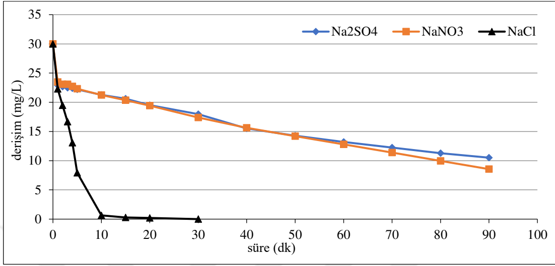
Şekil 6.69. %80 \text{IrO}_2 -%20 \text{RuO}_2 kaplı paralel plaka titanyum elektrotlarla, C_0 :30 mg/L \text{Na}_2\text{SO}_4 için; 200 \text{A/m}^2 akım yoğunluğu, 155,84 mL/dk akış hızı, 0,02 M \text{Na}_2\text{SO}_4 elektrolit miktarı, \text{pH}_{11} olan koşullarda; \text{NaNO}_3 için; 400 \text{A/m}^2 akım yoğunluğu, 155,84 mL/dk akış hızı, 0,01 M \text{NaNO}_3 elektrolit miktarı, \text{pH}_0 (6,24) olan koşullarda, \text{NaCl} için; 75 \text{A/m}^2 akım yoğunluğu, 155,84 mL/dk akış hızı, 0,05 M \text{NaCl} elektrolit miktarı, \text{pH}_0 (6,34) olan koşullarda elde edilen arıtım verimleri
