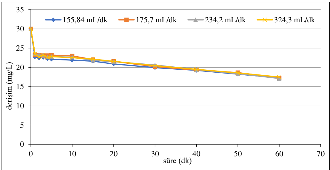
Şekil 6.27. \text{Ti}/\text{IrO}_2 kaplı paralel plaka elektrotlarla, C_0 :30 mg/L, 50 \text{ A/m}^2 akım yoğunluğu, 155,84 mL/dk, 175,7 mL/dk, 234,2 mL/dk, 324,3 mL/dk akış hızlarında, 0,01 M \text{NaNO}_3 , \text{pH}_0 : 5,94-6,44 olan koşullarda elde edilen arıtım verimleri
