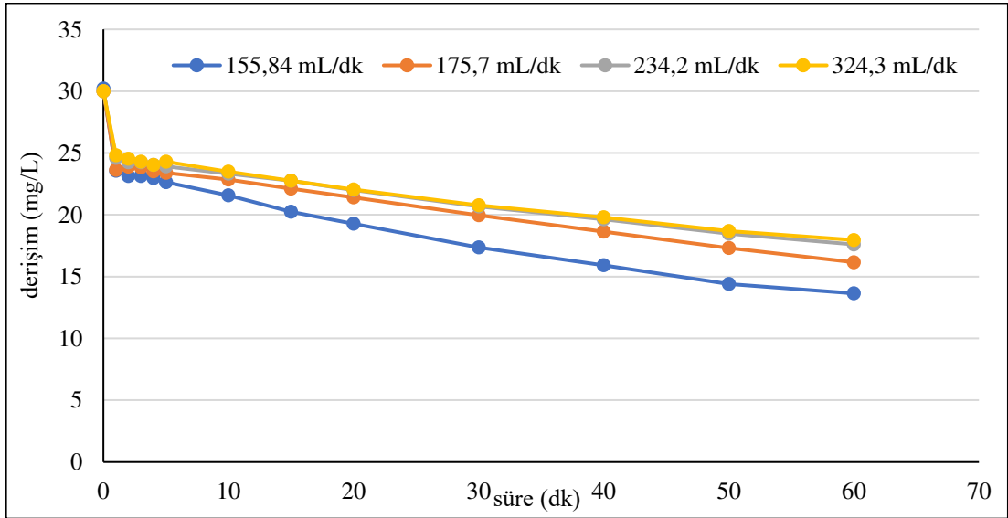
Şekil 6.39. \text{Ti/RuO}_2 kaplı paralel plaka elektrotlarla, C_o :30 mg/L, 150 \text{ A/m}^2 akım yoğunluğu, 155,84 mL/dk, 175,7 mL/dk, 234,2 mL/dk, 324,3 mL/dk akış hızlarında, 0,01 M \text{Na}_2\text{SO}_4 , \text{pH}_0 : 6,55-6,97 aralığında olan koşullarda elde edilen arıtım verimleri
