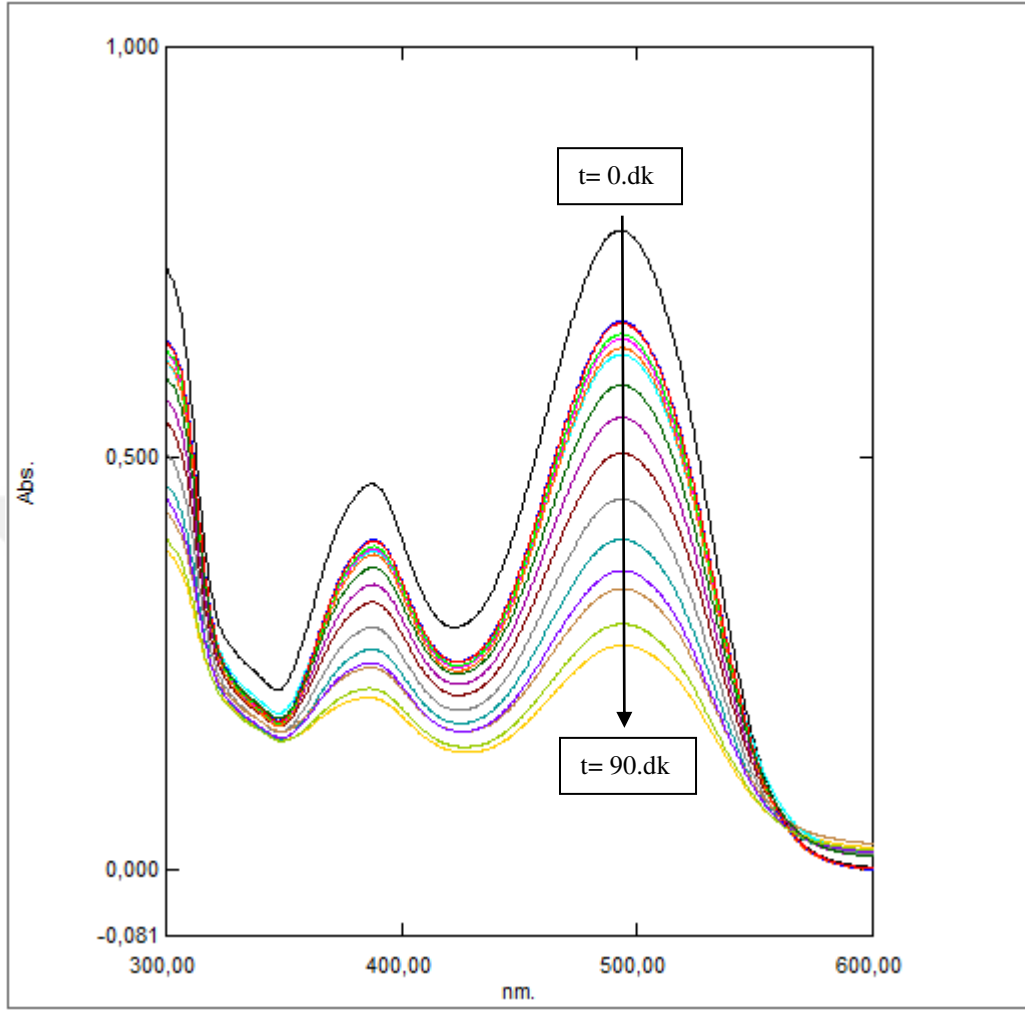
Şekil 6.145. %20IrO 2 -%80RuO 2 kaplı paralel plaka titanyum elektrotlarla, 125 mg/L başlangıç kirlilik derişimi için; 200 A/m 2 akım yoğunluğunda, 155,84 mL/dk akış hızında, 0,01 M Na 2 SO 4 elektrolit miktarı ve pH 11 'de UV-Spektrum grafiğı
