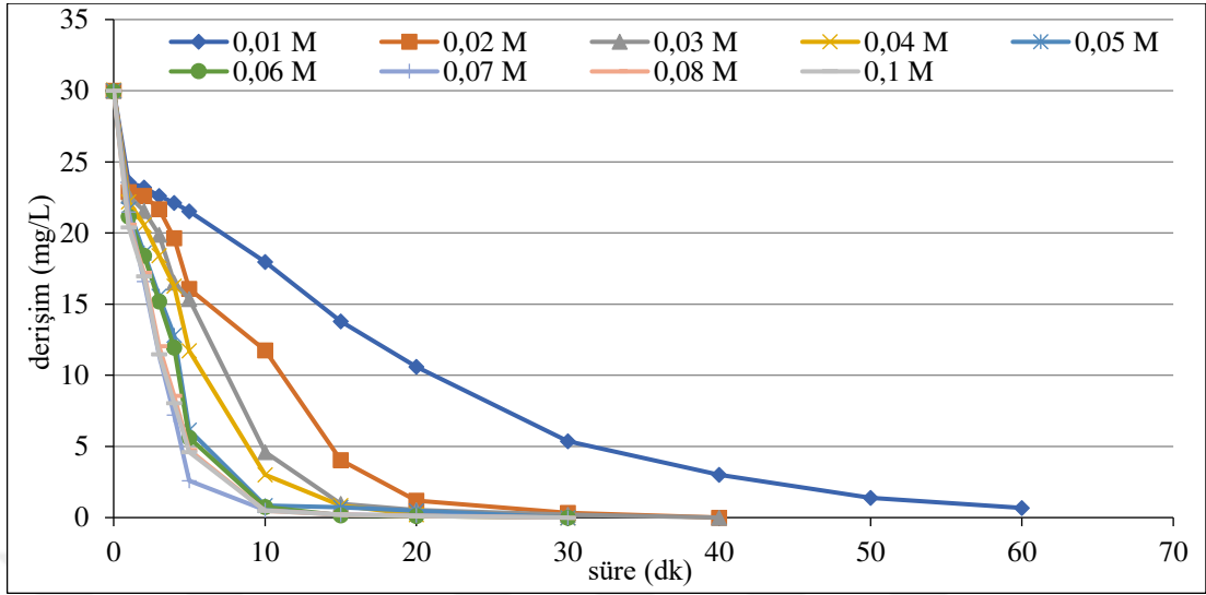
Şekil 6.82. %20IrO 2 -%80RuO 2 kaplı paralel plaka titanyum elektrotlarla, C_o :30 mg/L, 75 A/m 2 akım yoğunluğunda, 155,84 mL/dk akış hızında, 0,01/0,02/0,03/0,04/0,05/0,06M/0,07M/0,08M/0,1 M NaCl derişimlerinde, pH 0 : 6,23-6,29 aralığında olan koşullarda elde edilen arıtım verimleri
