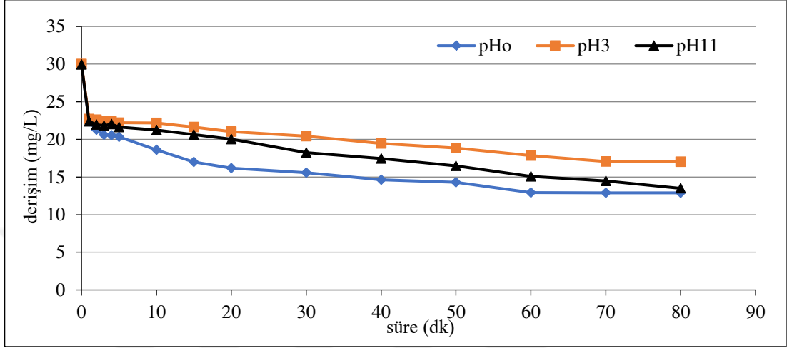
Şekil 6.11. Grafit plaka elektrotlarla, C_o :30 mg/L, 8 A/m 2 akım yoğunluğu, 175,7 mL/dk akış hızı, 0,01 M NaNO 3 , pH 0 (6,21), pH 3 ve pH 11 olan koşullarda arıtım verimleri
