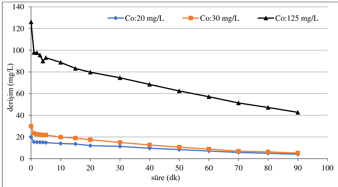
Şekil 6.109. %40IrO 2 -%60RuO 2 kaplı paralel plaka titanyum elektrotlarla, 300 A/m 2 akım yoğunluğunda, 155,84 mL/dk akış hızında, başlangıç kirlilik derişimleri 20 mg/L, 30 mg/L ve 125 mg/L olan 0,01 M \text{Na}_2\text{SO}_4 elektrolit derişiminde, pH 11 olan koşullarda elde edilen arıtım verimleri
