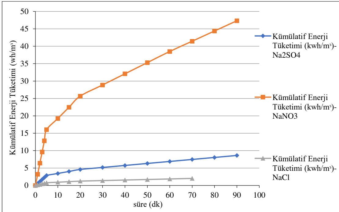
Şekil 6.188. %80IrO 2 -%20RuO 2 kaplı paralel plaka titanyum elektrotlarla, başlangıç kirlilik derişimi 125 mg/L olduđu durumda Na 2 SO 4 , NaNO 3 ve NaCl elektrolitleri ile optimum kořullarda oluřan enerji tüketim grafiđi
