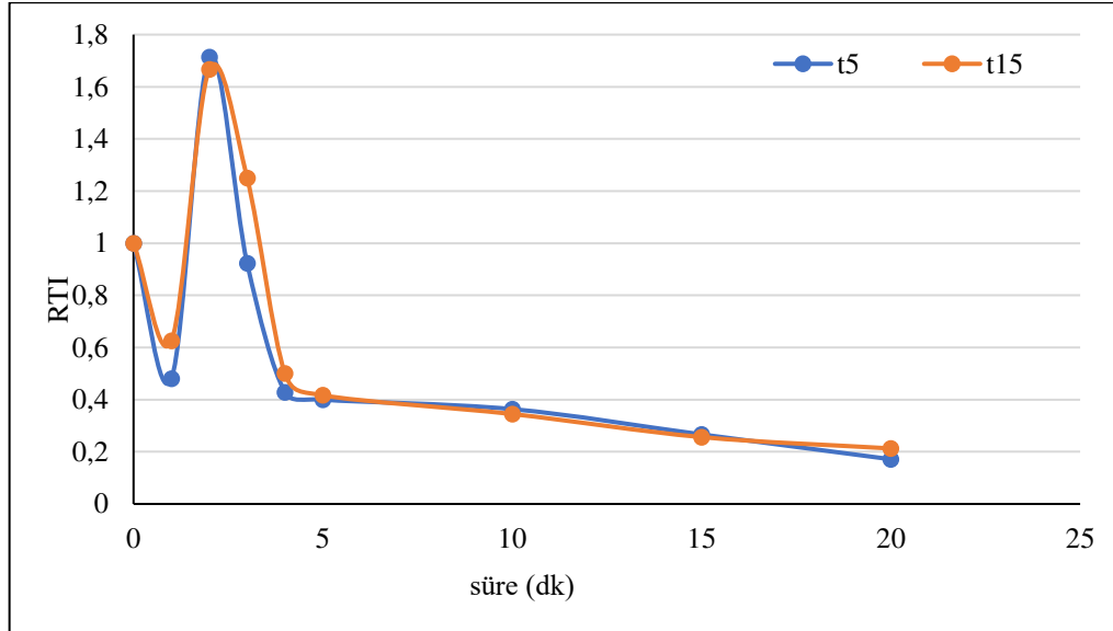
Şekil 6.177. Ti/RuO 2 kaplı elektrotlarla, başlangıç kirlilik derişimi 125 mg/L olduğu durumda NaCl elektroliti kullanılan deneylerde elde edilen toksisite grafiğı
