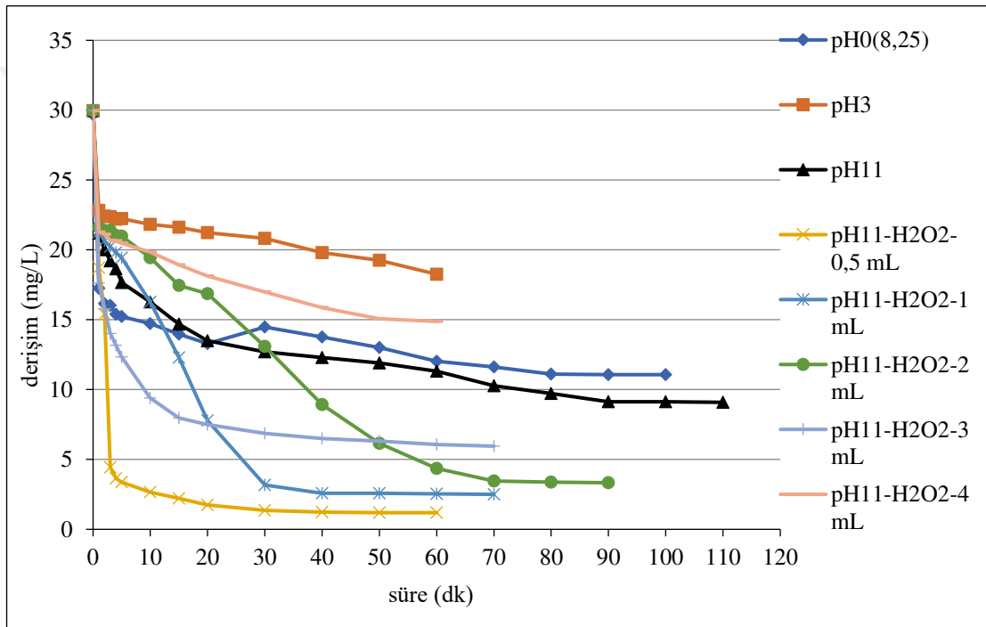
Şekil 6.18. Grafit plaka elektrotlarla, 8 A/m 2 akım yoğunluğu, 155,84 mL/dk akış hızı, başlangıç kirlilik derişimi 30 mg/L, 0,01 M Na_2SO_4 , pH 11 olan koşullarda; 0,5 mL/1 mL/2 mL/3 mL ve 4 mL H_2O_2 varlığında arıtım verimleri
