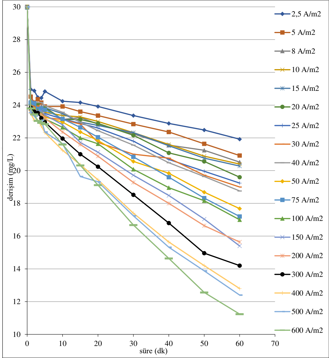
Şekil 6.59. %80IrO 2 -%20RuO 2 kaplı paralel plaka titanyum elektrotlarla, C_o :30 mg/L, 2,5/5/8/10/15/20/25/30/40/50/75/100/150/200/300/400/500/600 A/m 2 akım yoğunluklarında, 155,84 mL/dk akış hızında, 0,01 M Na 2 SO 4 , pH 0 : 6,24-6,47 aralığında olan koşullarda elde edilen arıtım verimleri
