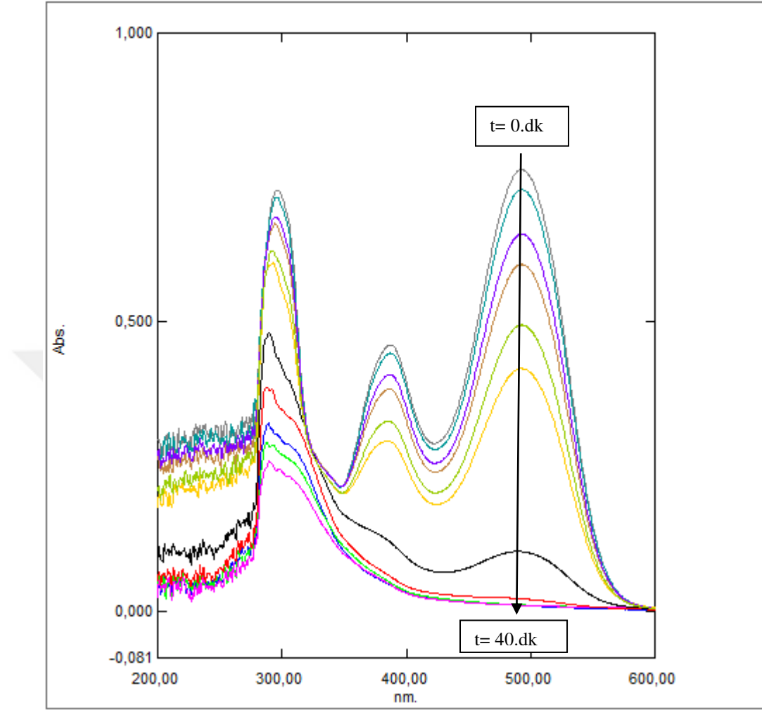
Şekil 6.143. %80IrO 2 -%20RuO 2 kaplı paralel plaka titanyum elektrotlarla, 125 mg/L başlangıç kirlilik derişimi için; 75 A/m 2 akım yoğunluğunda, 155,84 mL/dk akış hızında, 0,05 M NaCl elektrolit miktarı ve pH0'de UV-Spektrum grafiğı
