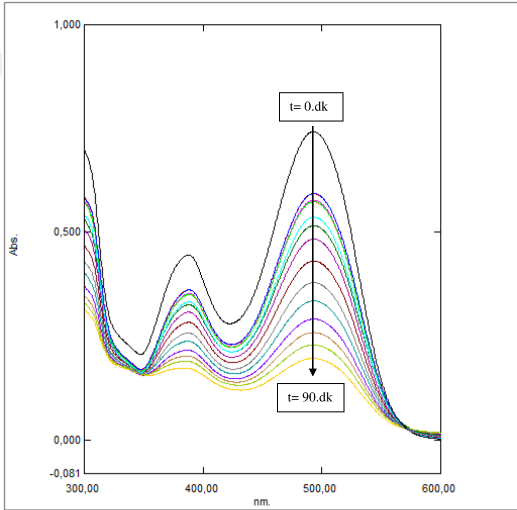
Şekil 6.150. %60IrO 2 -%40RuO 2 kaplı paralel plaka titanyum elektrotlarla, 30 mg/L başlangıç kirlilik derişimi için; 400 A/m 2 akım yoğunluğunda, 155,84 mL/dk akış hızında, 0,01 M Na 2 SO 4 elektrolit miktarı ve pH 11 'de UV-Spektrum grafiği
