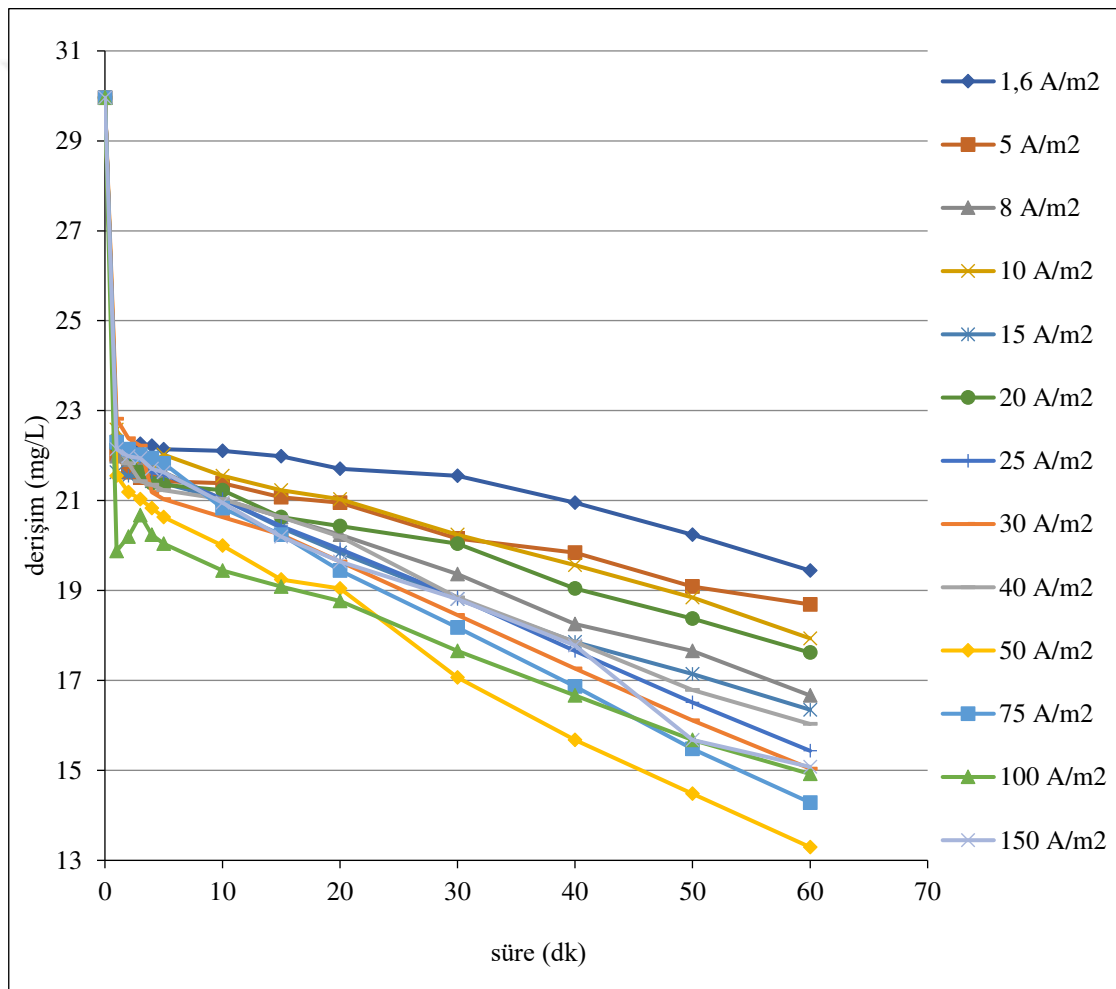
Şekil 6.20. \text{Ti}/\text{IrO}_2 kaplı paralel plaka elektrotlarla, C_0:30 mg/L, 1,6/5/8/10/15/20/25/30/40/50/75/100/150 \text{A}/\text{m}^2 akım yoğunluklarında, 155,84 mL/dk akış hızında, 0,01 M \text{Na}_2\text{SO}_4 , \text{pH}_{11} olan koşullarda elde edilen arıtım verimleri
