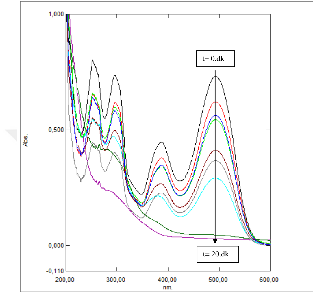
Şekil 6.124. Grafit paralel plaka elektrotlarla, 30 mg/L başlangıç kirlilik derişimi için; 40 A/m 2 akım yoğunluğunda, 155,84 mL/dk akış hızında, 0,08 M NaCl elektrolit miktarı ve pH 0 'de UV-Spektrum grafiğı
