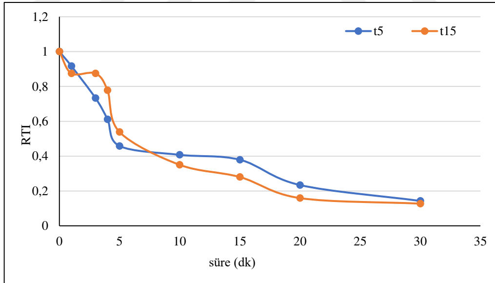
Şekil 6.181. %40Ir-%60RuO 2 kaplı titanyum elektrotlarla, başlangıç kirlilik derişimi 125 mg/L olduğu durumda NaCl elektroliti kullanılan deneylerde elde edilen toksisite grafiğı
