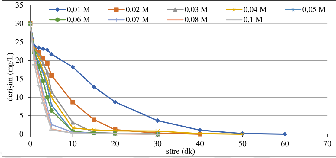
Şekil 6.65. %80IrO 2 -%20RuO 2 kaplı paralel plaka titanyum elektrotlarla, C o :30 mg/L, 75 A/m 2 akım yoğunluğunda, 155,84 mL/dk akış hızında, 0,01/0,02/0,03/0,04/0,05/0,06M/0,07M/0,08M/0,1 M NaCl derişimlerinde, pH 0 : 6,14-6,47 aralığında olan koşullarda elde edilen arıtım verimleri
