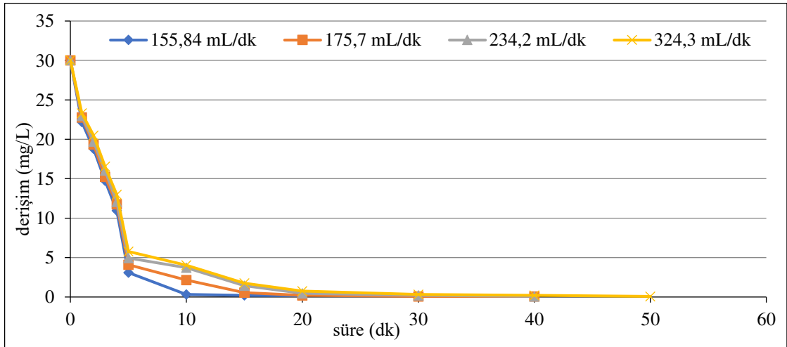
Şekil 6.117. %40IrO 2 -%60RuO 2 kaplı paralel plaka titanyum elektrotlarla, C o :30 mg/L, 75 A/m 2 akım yoğunluğu, 155,84 mL/dk, 175,7 mL/dk, 234,2 mL/dk, 324,3 mL/dk akış hızlarında, 0,05 M NaCl, pH 0 : 6,05-6,24 aralığında olan koşullarda elde edilen arıtım verimleri
