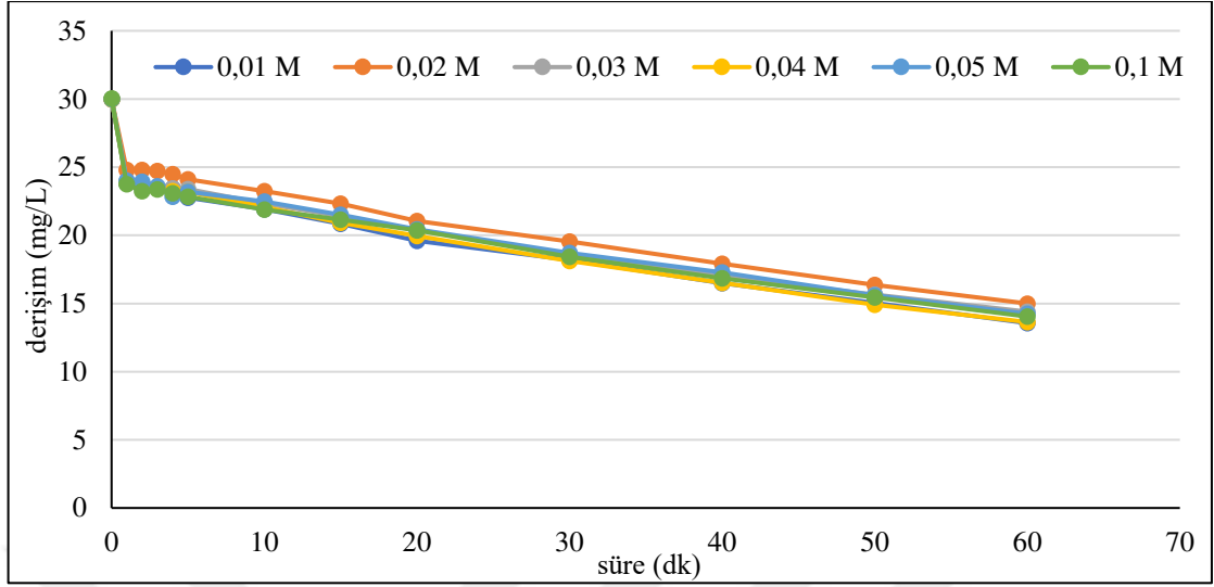
Şekil 6.72. %20 \text{IrO}_2 -%80 \text{RuO}_2 kaplı paralel plaka titanyum elektrotlarla, C_0 :30 mg/L, 200 \text{A/m}^2 akım yoğunluğunda, 155,84 mL/dk akış hızında, 0,01/0,02/0,03/0,04/0,05/0,1 M \text{Na}_2\text{SO}_4 derişimlerinde, \text{pH}_0 : 6,10-6,18 aralığında olan koşullarda elde edilen arıtım verimleri
