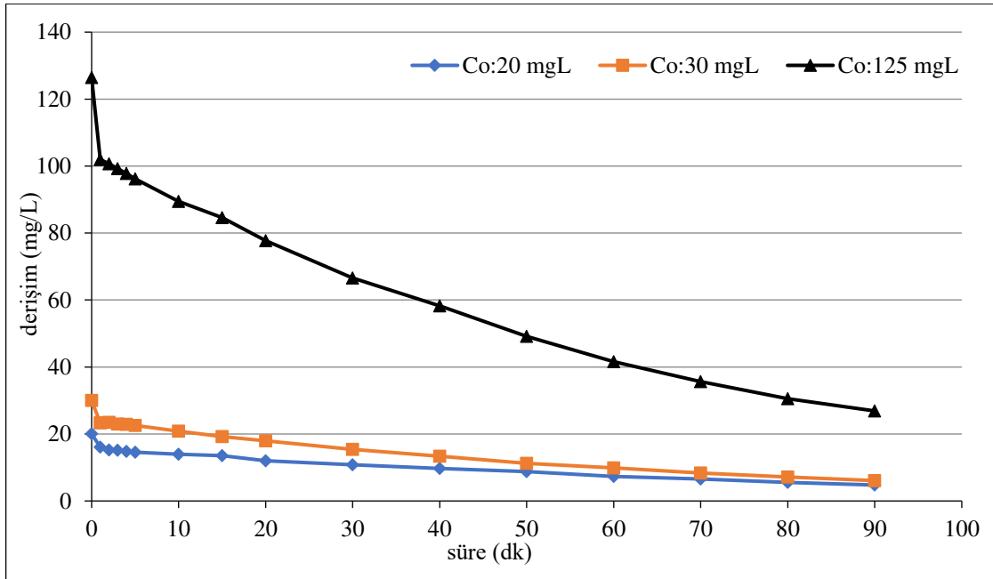
Şekil 6.97. %60IrO 2 -%40RuO 2 kaplı paralel plaka titanyum elektrotlarla, 500 A/m 2 akım yoğunluğunda, 155,84 mL/dk akış hızında, başlangıç kirlilik derişimleri 20 mg/L, 30 mg/L ve 125 mg/L olan 0,01 M \text{NaNO}_3 elektrolit derişiminde, pH 0 (5,80-6,20) olan koşullarda elde edilen arıtım verimleri
