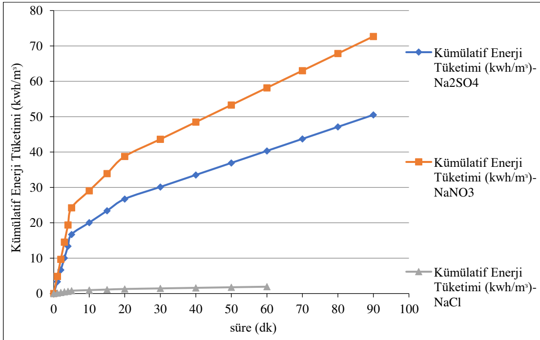
Şekil 6.192. %60IrO 2 -%40RuO 2 kaplı paralel plaka titanyum elektrotlarla, başlangıç kirlilik derişimi 125 mg/L olduđu durumda Na 2 SO 4 , NaNO 3 ve NaCl elektrolitleri ile optimum kořullarda oluřan enerji tüketim grafiđi
