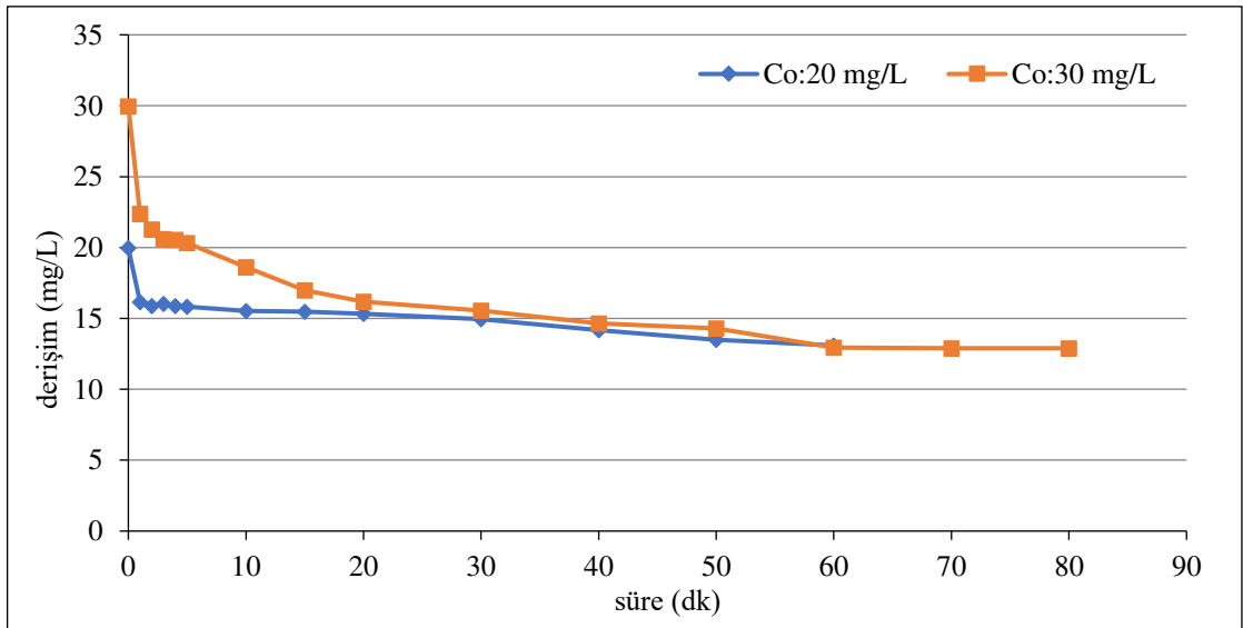
Şekil 6.12. Grafit plaka elektrotlarla, C_o :30 mg/L, 8 A/m 2 akım yoğunluğu, 0,01 M NaNO 3 , 175,7 mL/dk akış hızında pH 0 : 8,55 olan koşullarda başlangıç kirlilik derişimleri 20 ve 30 mg/L'deki arıtım verimleri
