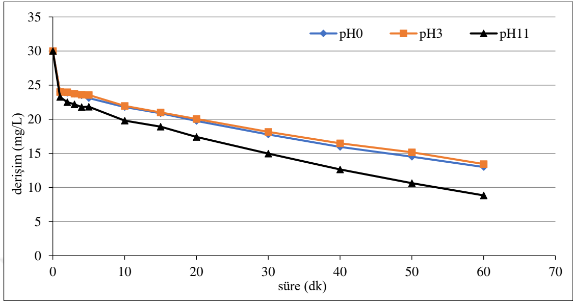
Şekil 6.108. %40IrO 2 -%60RuO 2 kaplı paralel plaka titanyum elektrotlarla, \text{Co} :30 mg/L, 300 A/m 2 akım yoğunluğunda, 155,84 mL/dk akış hızında, 0,01 M \text{Na}_2\text{SO}_4 derişiminde, pH 0 (6,15), pH 3 ve pH 11 ’de olan koşullarda elde edilen arıtım verimleri
