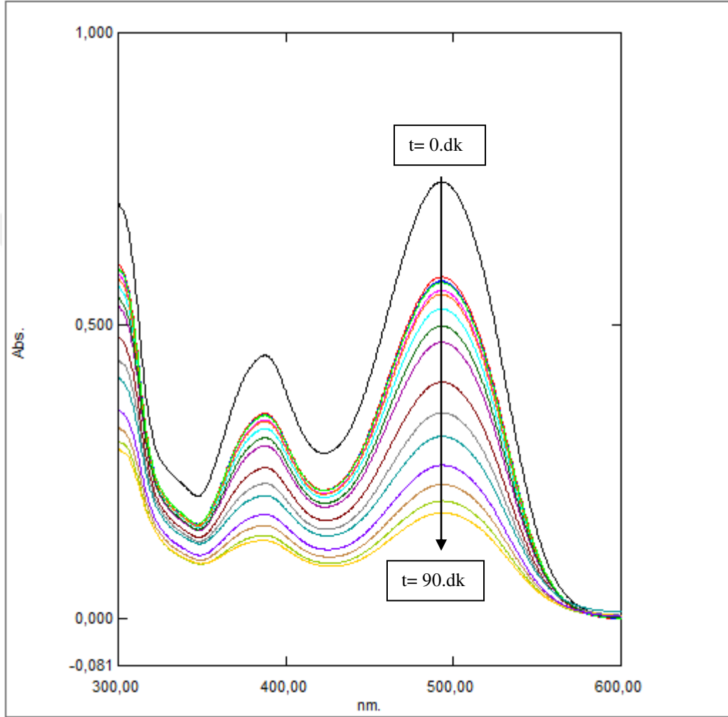
Şekil 6.146. %20IrO 2 -%80RuO 2 kaplı paralel plaka titanyum elektrotlarla, 30 mg/L başlangıç kirlilik derişimi için; 400 A/m 2 akım yoğunluğunda, 155,84 mL/dk akış hızında, 0,01 M NaNO 3 elektrolit miktarı ve pH 0 'de UV-Spektrum grafiği
