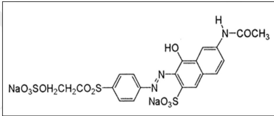
Şekil 5.1. RO16 boyarmaddesinin kimyasal yapısı ( http-5 )
