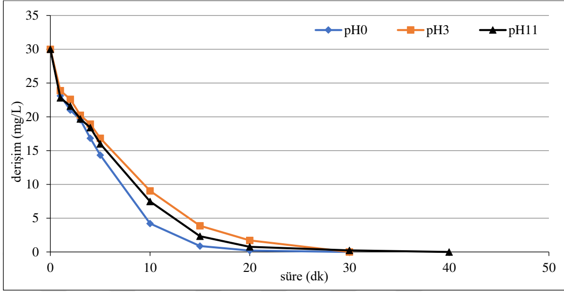
Şekil 6.50. Ti/RuO 2 kaplı paralel plaka elektrotlarla, C_o :30 mg/L, 50 A/m 2 akım yoğunluğunda, 155,84 mL/dk akış hızında, 0,06 M NaCl derişimlerinde, pH 0 (6,12), pH 3 ve pH 11 'de olan koşullarda elde edilen arıtım verimleri
