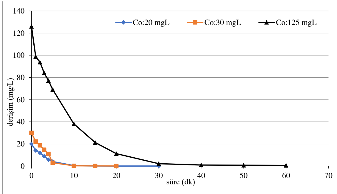
Şekil 6.119. %40IrO 2 -%60RuO 2 kaplı paralel plaka titanyum elektrotlarla, 75 A/m 2 akım yoğunluğunda, 155,84 mL/dk akış hızında, başlangıç kirlilik derişimleri 20 mg/L, 30 mg/L ve 125 mg/L olan 0,05 M NaCl elektrolit derişiminde, pH 0 (6,05-6,24) olan koşullarda elde edilen arıtım verimleri
