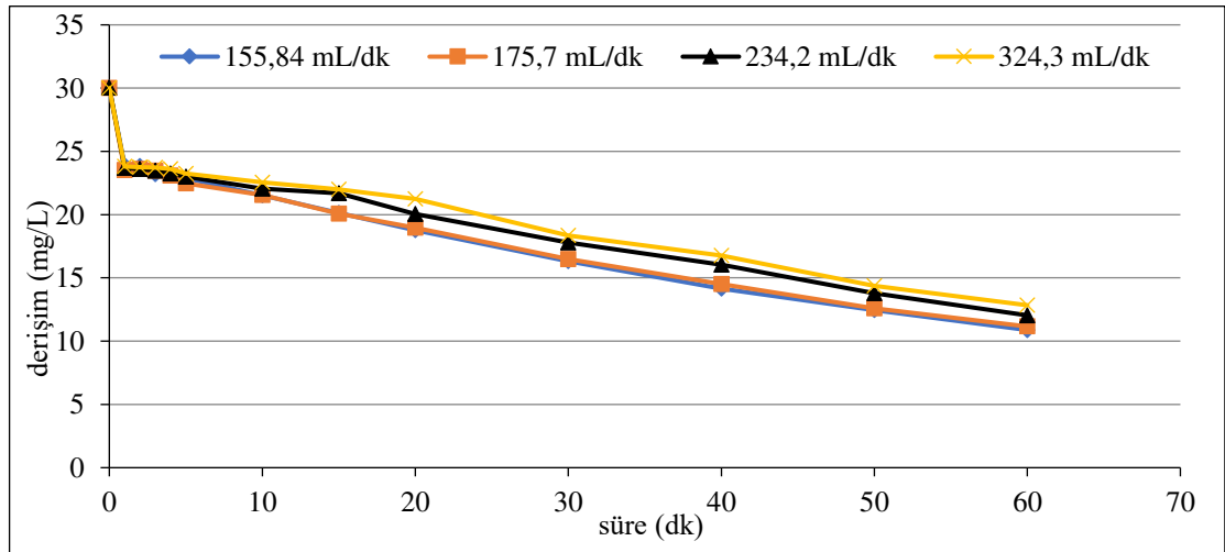
Şekil 6.78. %20 \text{IrO}_2 -%80 \text{RuO}_2 kaplı paralel plaka titanyum elektrotlarla, C_0 :30 mg/L, 400 A/m 2 akım yoğunluğu, 155,84 mL/dk, 175,7 mL/dk, 234,2 mL/dk, 324,3 mL/dk akış hızlarında, 0,01 M \text{NaNO}_3 , \text{pH}_0 : 6,20-6,25 aralığında olan koşullarda elde edilen arıtım verimleri
