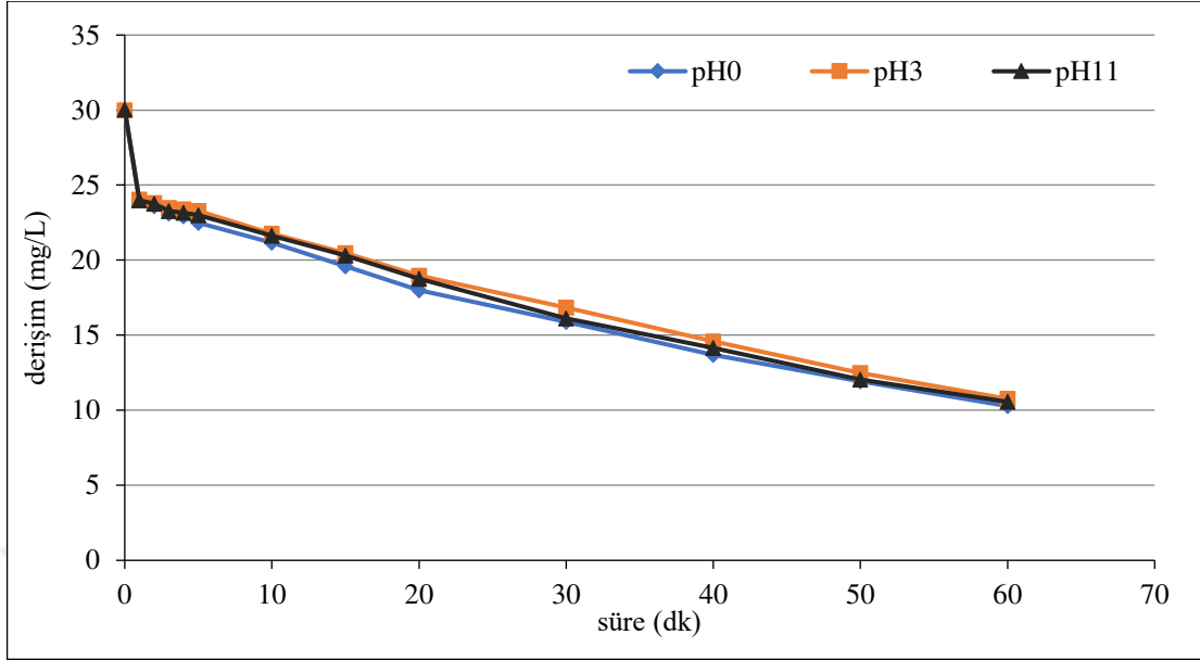
Şekil 6.113. %40IrO 2 -%60RuO 2 kaplı paralel plaka titanyum elektrotlarla, C_0 :30 mg/L, 500 A/m 2 akım yoğunluğunda, 155,84 mL/dk akış hızında, 0,01 M \text{NaNO}_3 derişimlerinde, pH 0 (6,24), pH 3 ve pH 11 ’de olan koşullarda elde edilen arıtım verimleri
