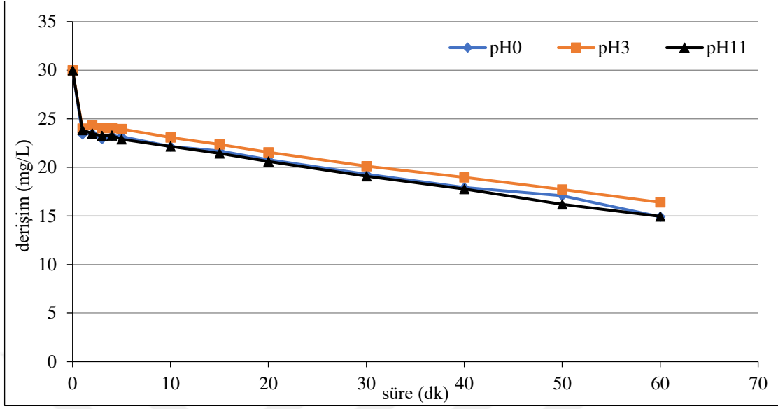
Şekil 6.45. \text{Ti/RuO}_2 kaplı paralel plaka elektrotlarla, C_0 :30 mg/L, 150 \text{ A/m}^2 akım yoğunluğunda, 155,84 \text{ mL/dk} akış hızında, 0,01 \text{ M NaNO}_3 derişiminde, \text{pH}_0 (6,66), \text{pH}_3 ve \text{pH}_{11} 'de olan koşullarda elde edilen arıtım verimleri
