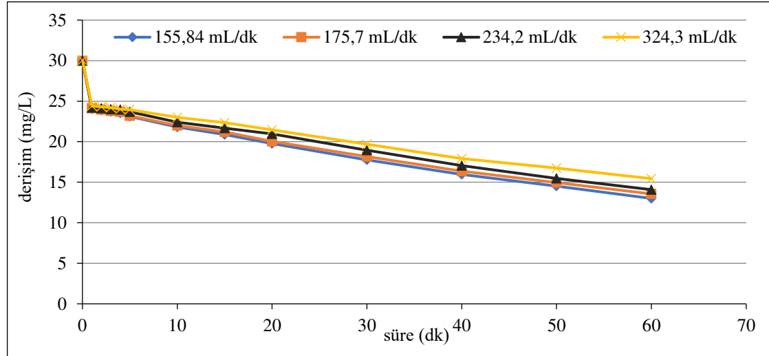
Şekil 6.107. %40IrO 2 -%60RuO 2 kaplı paralel plaka titanyum elektrotlarla, C o :30 mg/L, 300 A/m 2 akım yoğunluğu, 155,84 mL/dk, 175,7 mL/dk, 234,2 mL/dk, 324,3 mL/dk akış hızlarında, 0,01 M Na 2 SO 4 , pH 0 : 6,14-6,16 aralığında olan koşullarda elde edilen arıtım verimleri
