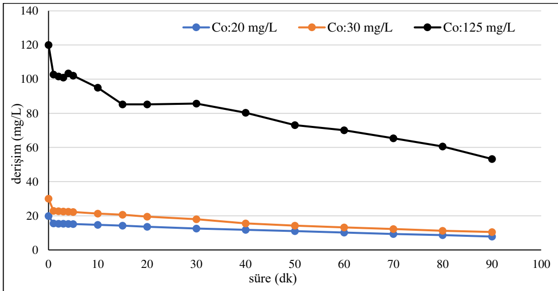
Şekil 6.58. %80IrO 2 -%20RuO 2 kaplı paralel plaka titanyum elektrotlarla, 200 A/m 2 akım yoğunluğunda, 155,84 mL/dk akış hızında, başlangıç kirlilik derişimi 20 mg/L, 30 mg/L ve 125 mg/L olan 0,02 M \text{Na}_2\text{SO}_4 elektrolit derişiminde, pH 11 : 11 olan koşullarda elde edilen arıtım verimleri
