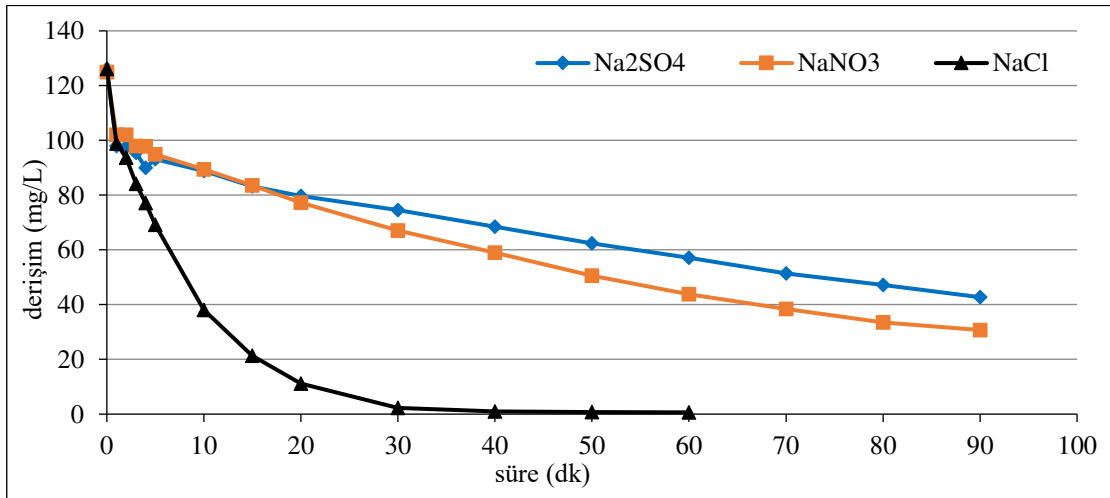
Şekil 6.121. %40 \text{IrO}_2 -%60 \text{RuO}_2 kaplı paralel plaka tiyanyum elektrotlarla, C_0 :125 mg/L \text{Na}_2\text{SO}_4 için; 300 \text{A/m}^2 akım yoğunluğu, 155,84 mL/dk akış hızı, 0,01 M \text{Na}_2\text{SO}_4 elektrolit miktarı, \text{pH}_{11} olan koşullarda; \text{NaNO}_3 için; 500 \text{A/m}^2 akım yoğunluğu, 155,84 mL/dk akış hızı, 0,01 M \text{NaNO}_3 elektrolit miktarı, \text{pH}_0 (6,16) olan koşullarda, \text{NaCl} için; 75 \text{A/m}^2 akım yoğunluğu, 155,84 mL/dk akış hızı, 0,05 M \text{NaCl} elektrolit miktarı, \text{pH}_0 (6,15) olan koşullarda elde edilen arıtım verimleri
