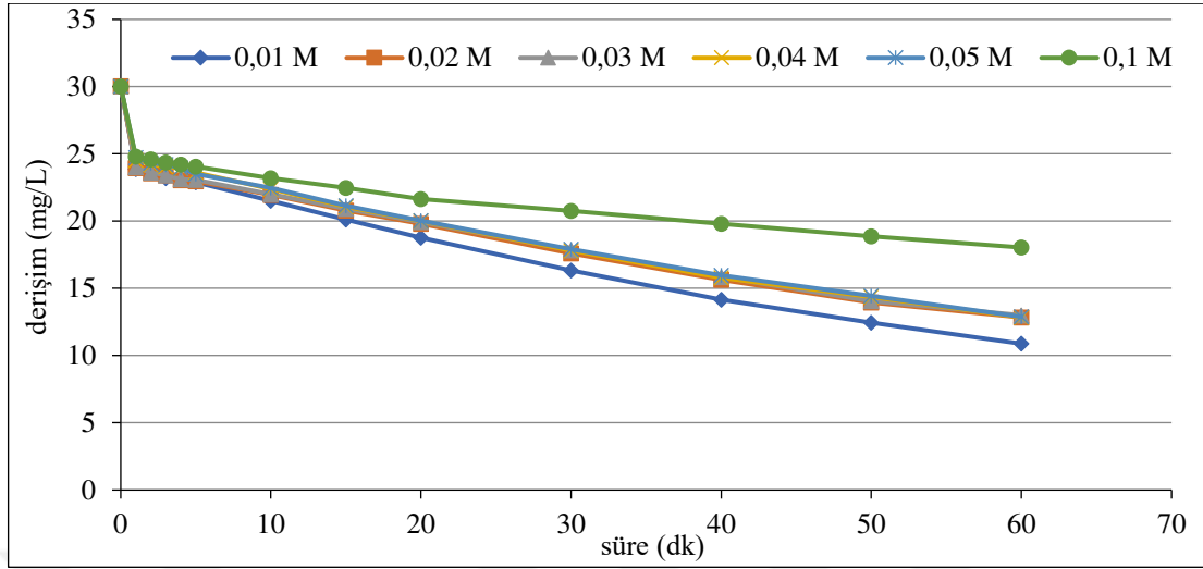
Şekil 6.77. %20 \text{IrO}_2 -%80 \text{RuO}_2 kaplı paralel plaka titanyum elektrotlarla, C_0 :30 mg/L, 400 A/m 2 akım yoğunluğunda, 155,84 mL/dk akış hızında, 0,01/0,02/0,03/0,04/0,05/0,1 M \text{NaNO}_3 derişimlerinde, \text{pH}_0 : 6,20-6,35 aralığında olan koşullarda elde edilen arıtım verimleri
