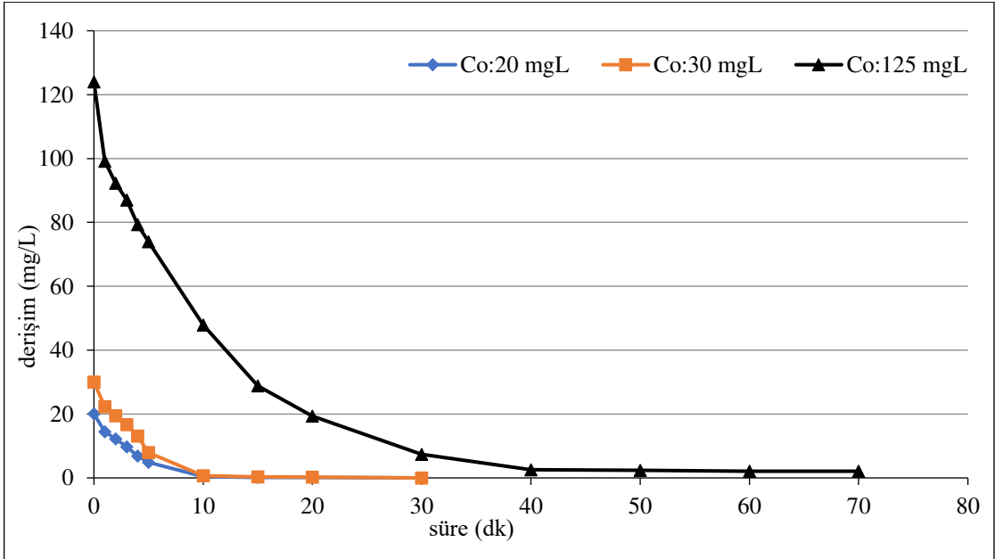
Şekil 6.68. %80IrO 2 -%20RuO 2 kaplı paralel plaka titanyum elektrotlarla, 75 A/m 2 akım yoğunluğunda, 155,84 mL/dk akış hızında, başlangıç kirlilik derişimleri 20 mg/L, 30 mg/L ve 125 mg/L olan 0,05 M NaCl elektrolit derişiminde, pH 0 (6,34-6,78) olan koşullarda elde edilen arıtım verimleri
