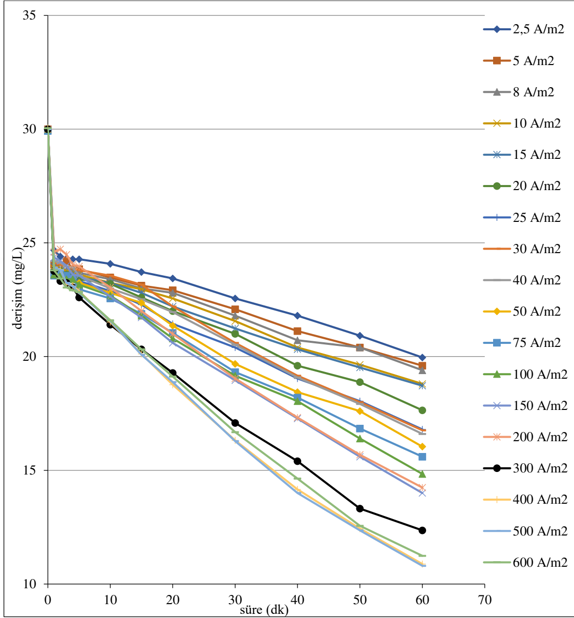
Şekil 6.76. %20 \text{IrO}_2 -%80 \text{RuO}_2 kaplı paralel plaka titanyum elektrotlarla, C_o :30 mg/L, 2,5/5/8/10/15/20/25/30/40/50/75/100/150/200/300/400/500/600 \text{A/m}^2 akım yoğunluklarında, 155,84 mL/dk akış hızında, 0,01 M \text{NaNO}_3 , \text{pH}_0 : 6,15-6,70 aralığında olan koşullarda elde edilen arıtım verimleri
