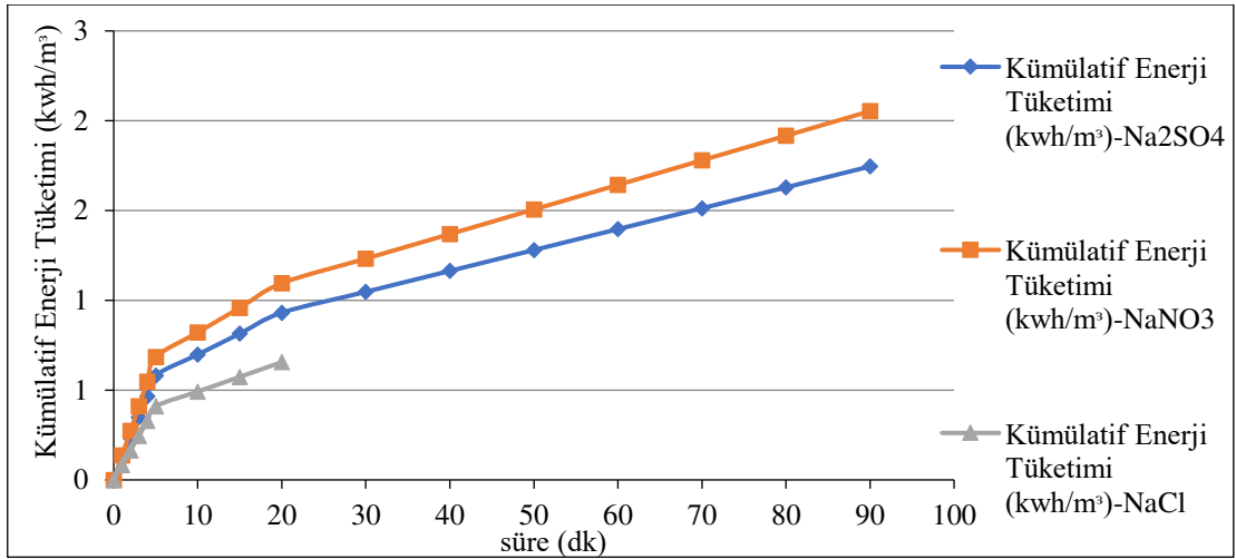
Şekil 6.183. Ti/IrO 2 kaplı paralel plaka elektrotlarla, başlangıç kirlilik derişimi 30 mg/L olduğu durumda Na 2 SO 4 , NaNO 3 ve NaCl elektrolitleri ile optimum koşullarda oluşan, enerji tüketim grafiği
