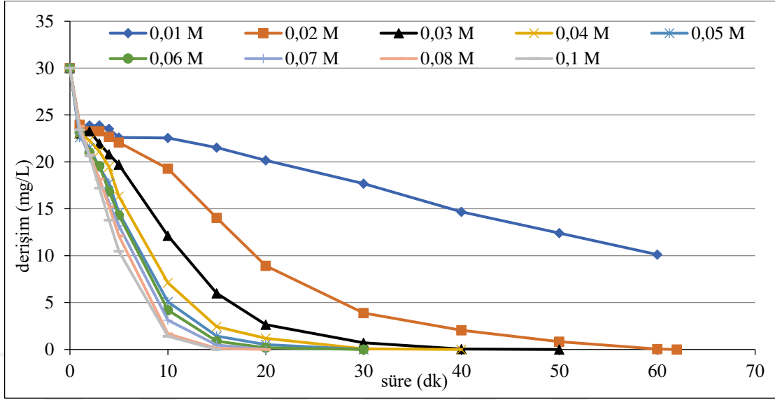
Şekil 6.48. Ti/RuO 2 kaplı paralel plaka elektrotlarla, C o :30 mg/L, 50 A/m 2 akım yoğunluğunda, 155,84 mL/dk akış hızında, 0,01/0,02/0,03/0,04/0,05/0,06/0,07/0,08/0,1 M NaCl elektrolit derişimlerinde, pH 0 : 6-6,28 aralığında olan koşullarında elde edilen arıtım verimleri
