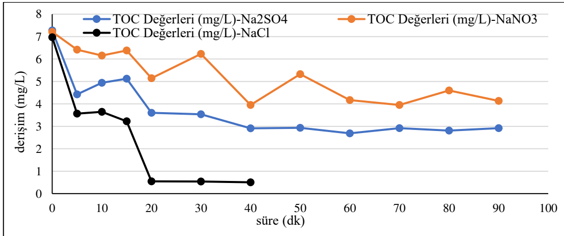
Şekil 6.163. Ti/IrO 2 kaplı paralel plaka elektrotlarla, başlangıç kirlilik derişimi 30 mg/L, 50 A/m 2 akım yoğunluğu, 155,84 mL/dk hızı, 0,01 M Na 2 SO 4 elektrolit derişimi, pH 11 : 11'de; 50 A/m 2 akım yoğunluğu, 155,84 mL/dk akış hızı, 0,01 M NaNO 3 elektrolit derişimi, pH 0 'da; 50 A/m 2 akım yoğunluğu, 155,84 mL/dk akış hızı, 0,05 M NaCl elektrolit derişimi, pH 0 olan koşullarda elde edilen TOC sonuçları
