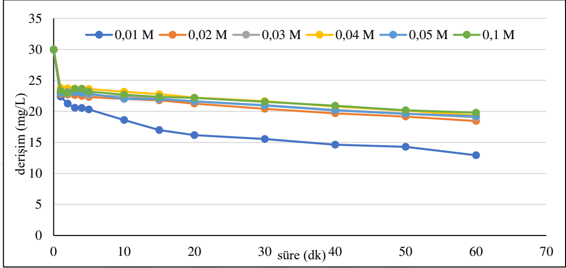
Şekil 6.9. Grafit plaka elektrotlarla, C_o :30 mg/L, 8 \text{ A/m}^2 akım yoğunluğu, 175,7 mL/dk akış hızında, başlangıç \text{pH}_0 : 8,55, 0,01 M/ 0,02 M/ 0,03 M/ 0,04 M/ 0,05 M/ 0,1 M \text{NaNO}_3 elektroliti kullanılan koşullarda arıtım verimleri
