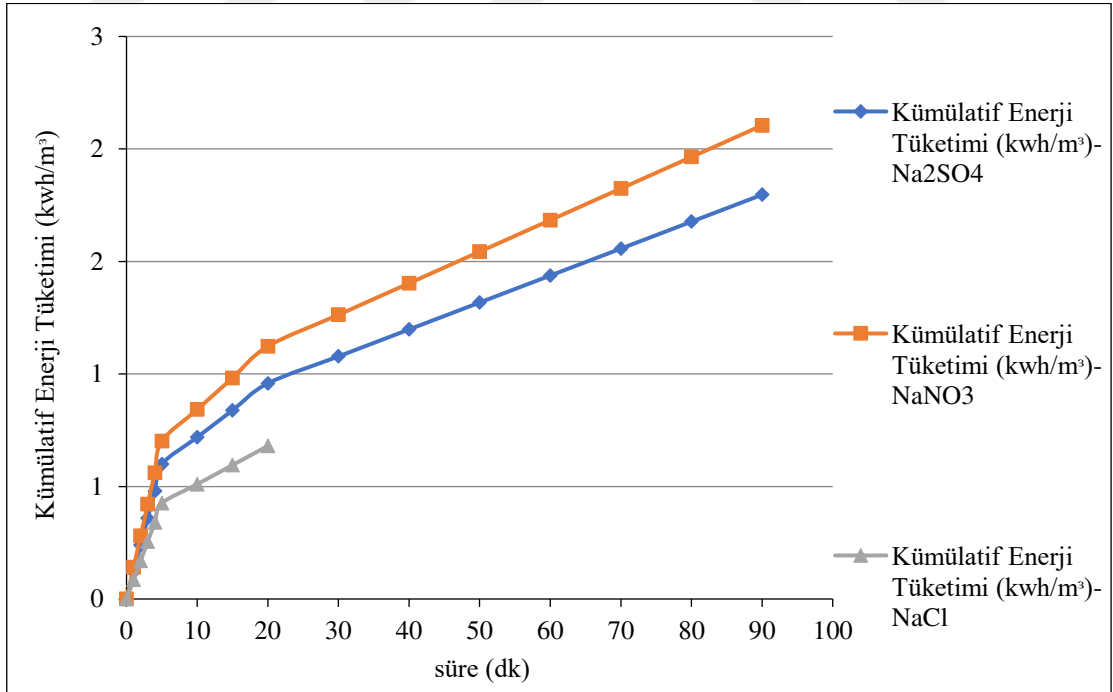
Şekil 6.184. Ti/IrO 2 kaplı paralel plaka elektrotlarla, başlangıç kirlilik derişimi 125 mg/L olduğu durumda Na 2 SO 4 , NaNO 3 ve NaCl elektrolitleri ile optimum koşullarda oluşan enerji tüketim grafiği
