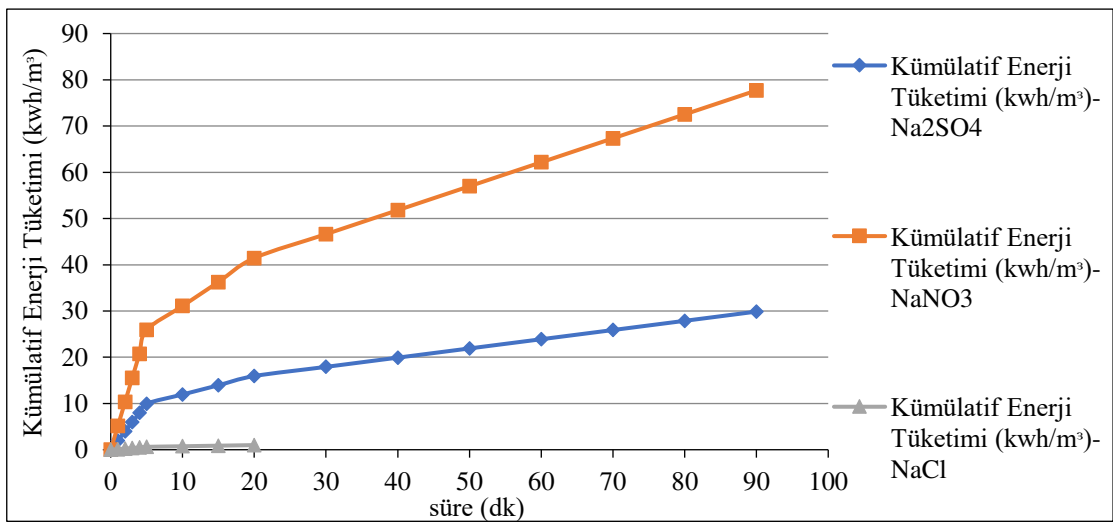
Şekil 6.193. %40IrO 2 -%60RuO 2 kaplı paralel plaka titanyum elektrotlarla, başlangıç kirlilik derişimi 30 mg/L olduğu durumda Na 2 SO 4 , NaNO 3 ve NaCl elektrolitleri ile optimum koşullarda oluşan enerji tüketim grafiği
