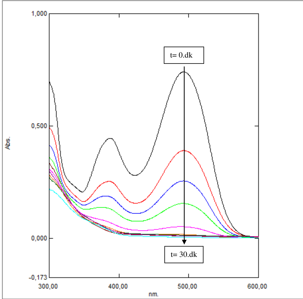
Şekil 6.142. %80IrO 2 -%20RuO 2 kaplı paralel plaka titanyum elektrotlarla, 30 mg/L başlangıç kirlilik derişimi için; 75 A/m 2 akım yoğunluğunda, 155,84 mL/dk akış hızında, 0,05 M NaCl elektrolit miktarı ve pH 0 'de UV-Spektrum grafiğı
