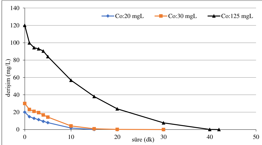
Şekil 6.51. Ti/RuO 2 kaplı paralel plaka elektrotlarla, 50 A/m 2 akım yoğunluğunda, 155,84 mL/dk akış hızında, başlangıç kirlilik derişimi 20 mg/L, 30 mg/L ve 125 mg/L olan 0,06 M NaCl elektrolit derişimlerinde, pH 0 : 6-6,20'deki koşullarda elde edilen arıtım verimleri
