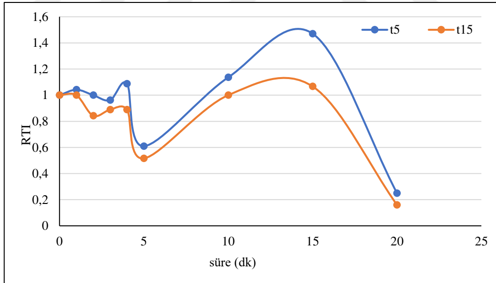
Şekil 6.179. %20Ir-%80RuO 2 kaplı titanyum elektrotlarla, başlangıç kirlilik derişimi 125 mg/L olduğu durumda NaCl elektroliti kullanılan deneylerde elde edilen toksisite grafiğı
