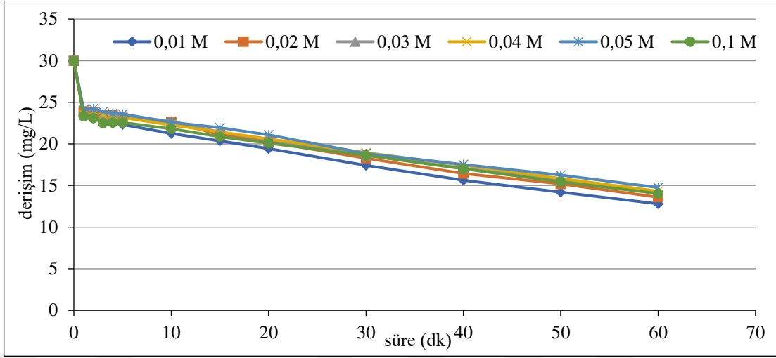
Şekil 6.60. %80 \text{IrO}_2 -%20 \text{RuO}_2 kaplı paralel plaka titanyum elektrotlarla, C_o :30 mg/L, 400 A/m 2 akım yoğunluğunda, 155,84 mL/dk akış hızında, 0,01/0,02/0,03/0,04/0,05/0,1 M \text{NaNO}_3 derişimlerinde, \text{pH}_0 : 6,30-6,47 aralığında olan koşullarda elde edilen arıtım verimleri
