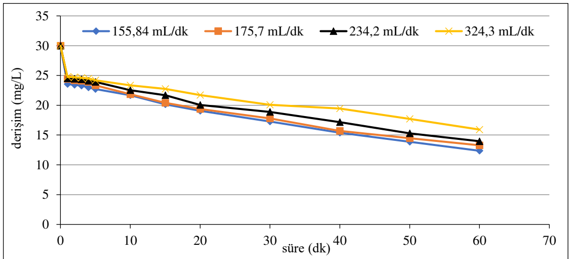
Şekil 6.90. %60IrO 2 -%40RuO 2 kaplı paralel plaka titanyum elektrotlarla, C_0 :30 mg/L, 400 A/m 2 akım yoğunluğu, 155,84 mL/dk, 175,7 mL/dk, 234,2 mL/dk, 324,3 mL/dk akış hızlarında, 0,01 M \text{Na}_2\text{SO}_4 , pH 0 : 6,08-6,11 aralığında olan koşullarda elde edilen arıtım verimleri
