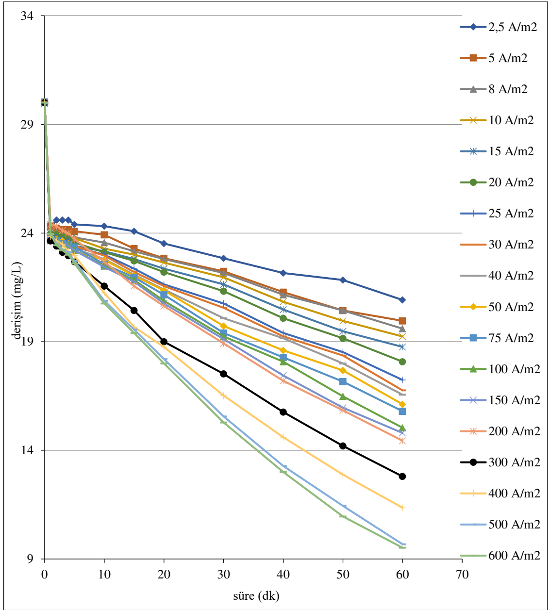
Şekil 6.93. %60IrO 2 -%40RuO 2 kaplı paralel plaka titanyum elektrotlarla, C_o :30 mg/L, 2,5/5/8/10/15/20/25/30/40/50/75/100/150/200/300/400/500/600 A/m 2 akım yoğunluklarında, 155,84 mL/dk akış hızında, 0,01 M NaNO 3 , pH 0 : 5,94-6,21 aralığında olan koşullarda elde edilen arıtım verimleri
