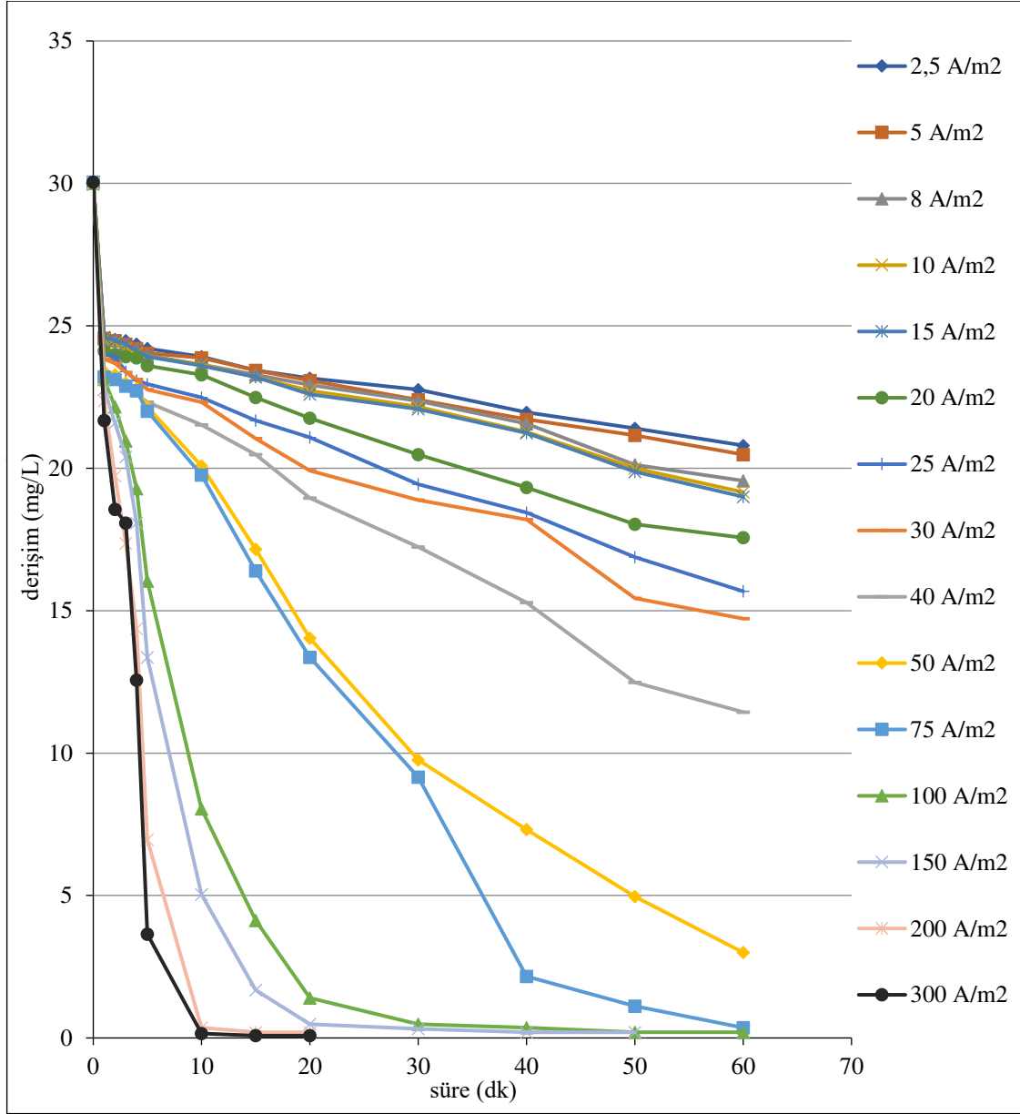
Şekil 6.115. %40IrO 2 -%60RuO 2 kaplı paralel plaka titanyum elektrotlarla, C 0 :30 mg/L, 2,5/5/8/10/15/20/25/30/40/50/75/100/150/200/300 A/m 2 akım yoğunluklarında, 155,84 mL/dk akış hızında, 0,01 M NaCl, pH 0 : 6,14-6,33 aralığında olan koşullarda elde edilen arıtım verimleri
