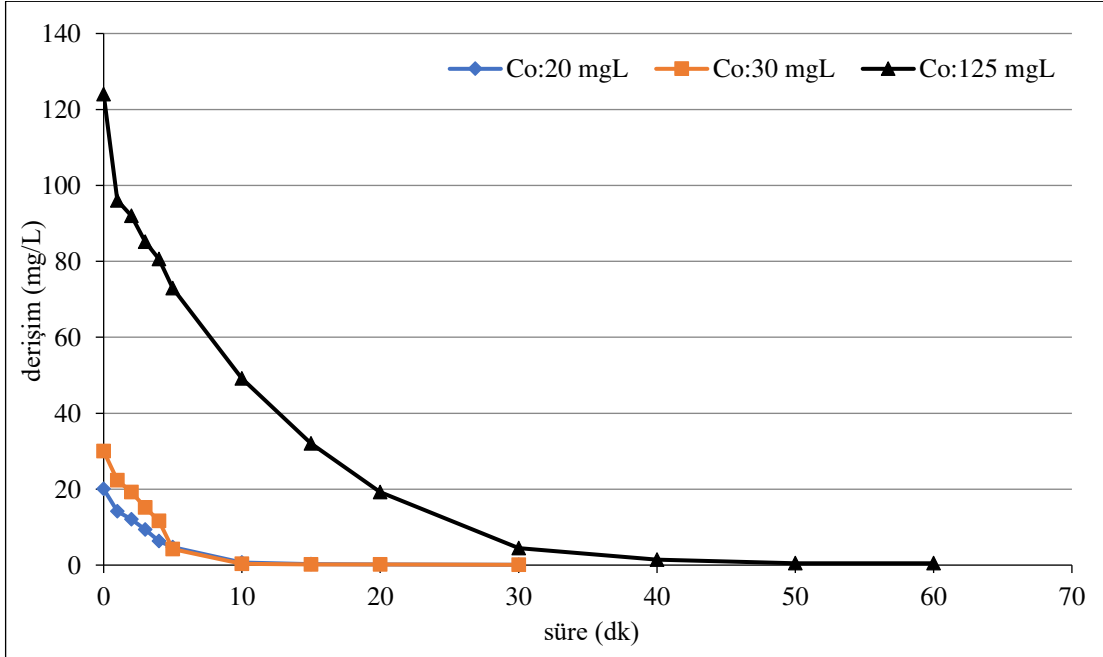
Şekil 6.102. %60IrO 2 -%40RuO 2 kaplı paralel plaka titanyum elektrotlarla, 75 A/m 2 akım yoğunluğunda, 155,84 mL/dk akış hızında, başlangıç kirlilik derişimleri 20 mg/L, 30 mg/L ve 125 mg/L olan 0,05 M NaCl elektrolit derişiminde, pH 0 (6,21-6,26) olan koşullarda elde edilen arıtım verimleri
