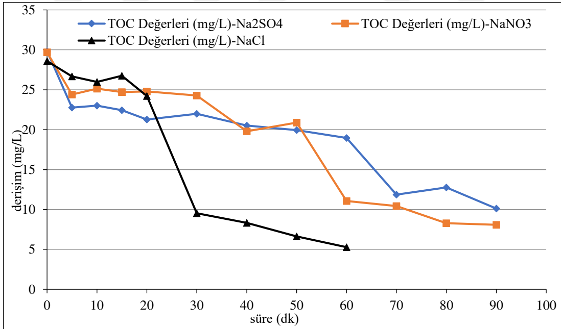
Şekil 6.172. %60IrO 2 -%40RuO 2 kaplı paralel plaka titanyum elektrotlarla, başlangıç kirlilik derişimi 125 mg/L, 400 A/m 2 akım yoğunluğu, 155,84 mL/dk akış hızı, 0,01 M Na 2 SO 4 elektrolit derişimi, pH 11 : 11'de; 500 A/m 2 akım yoğunluğu, 155,84 mL/dk akış hızı, 0,01 M NaNO 3 elektrolit derişimi, pH 0 'da; 75 A/m 2 akım yoğunluğu, 155,84 mL/dk akış hızı, 0,05 M NaCl elektrolit derişimi, pH 0 olan koşullarda elde edilen TOC sonuçları
