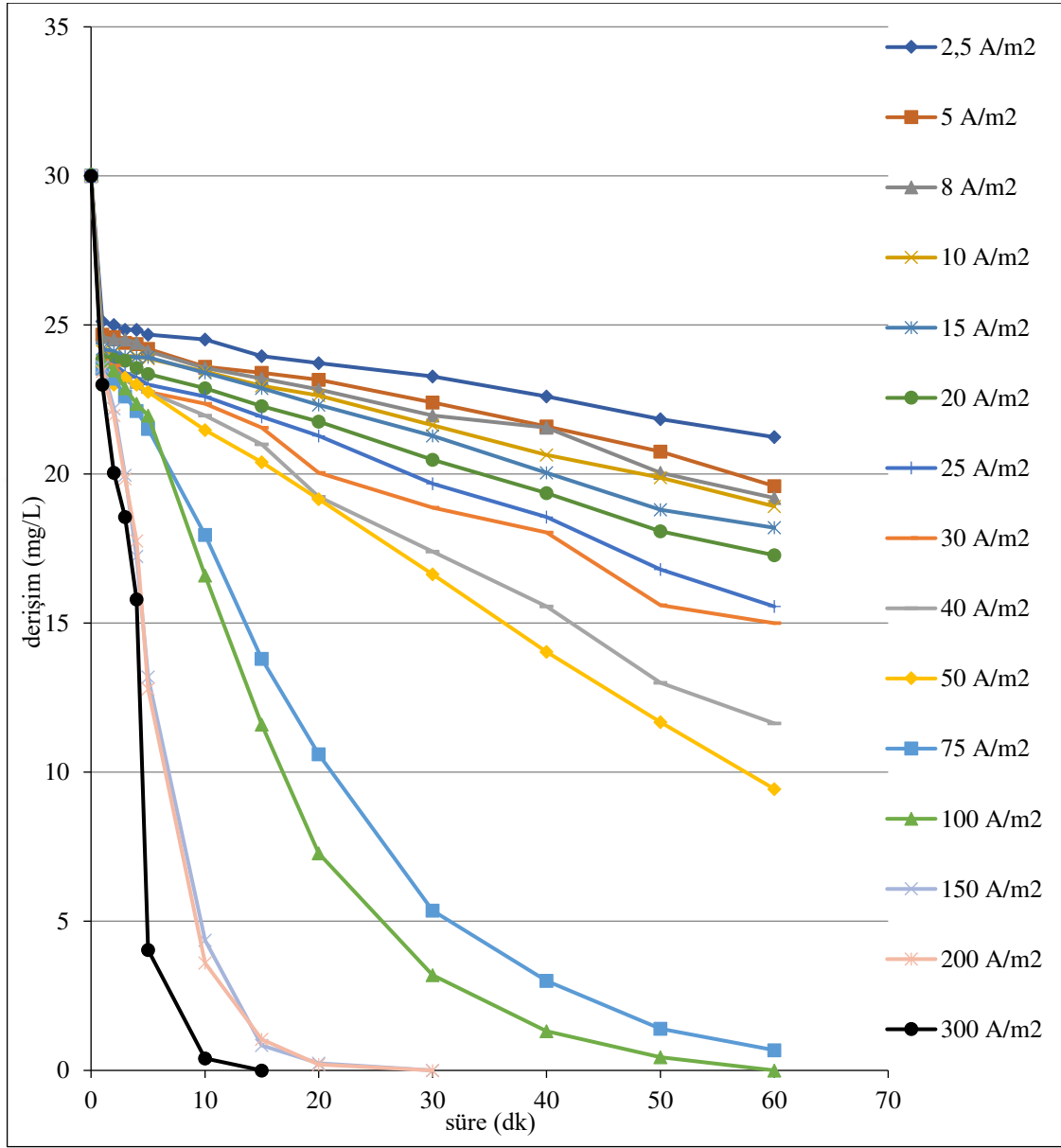
Şekil 6.81. %20IrO 2 -%80RuO 2 kaplı paralel plaka titanyum elektrotlarla, C o :30 mg/L, 2,5/5/8/10/15/20/25/30/40/50/75/100/150/200/300 A/m 2 akım yoğunluklarında, 155,84 mL/dk akış hızında, 0,01 M NaCl, pH 0 : 6,19-6,29 aralığında olan koşullarda elde edilen arıtım verimleri
