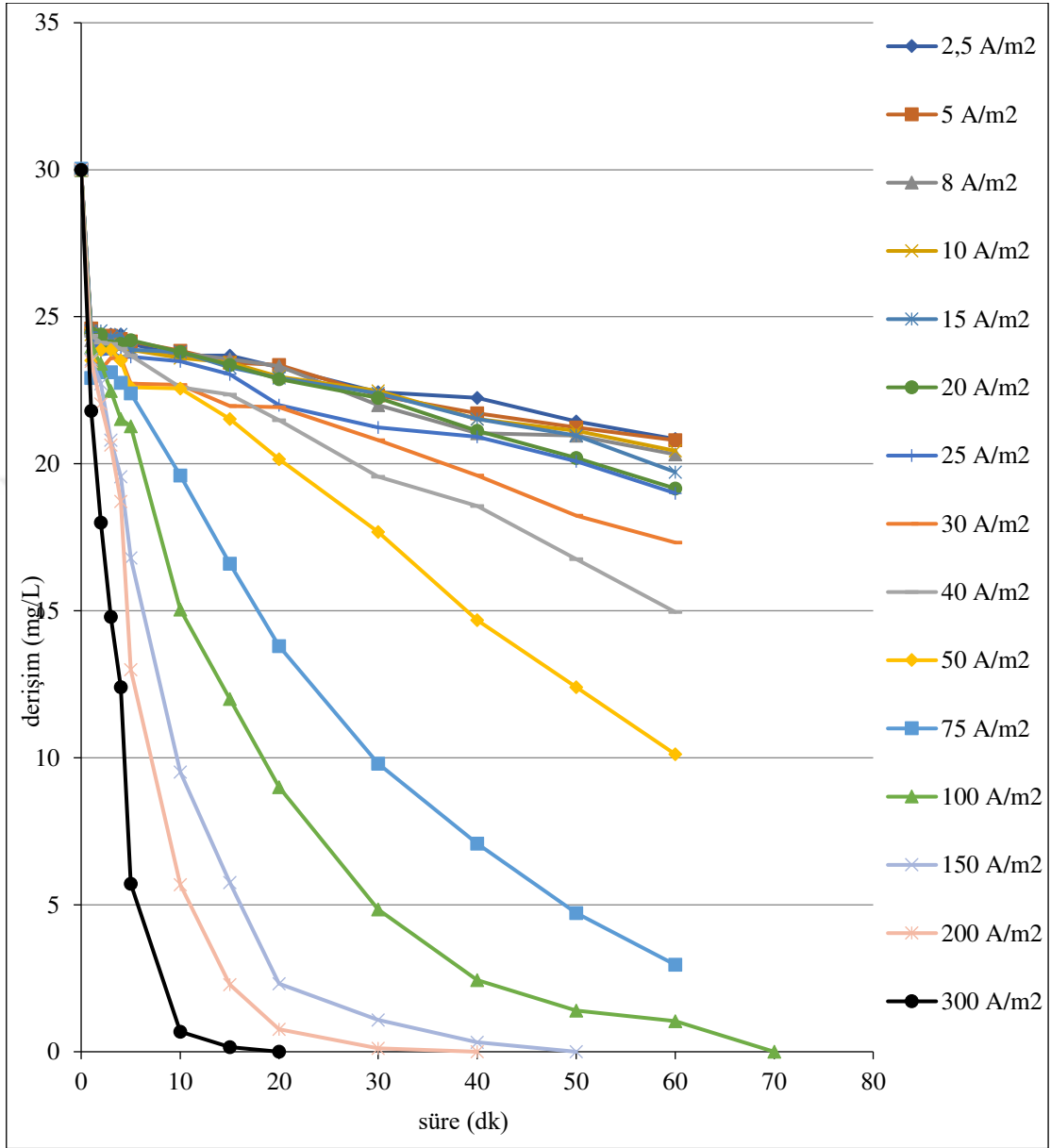
Şekil 6.47. Ti/RuO 2 kaplı paralel plaka elektrotlarla, C o :30 mg/L, 2,5/5/8/10/15/20/25/30/40/50/75/100/150/200/300 A/m 2 akım yoğunluklarında, 155,84 mL/dk akış hızında, 0,01 M NaCl, pH 0 : 5,13-6,51 aralığında olan koşullarda elde edilen arıtım verimleri
