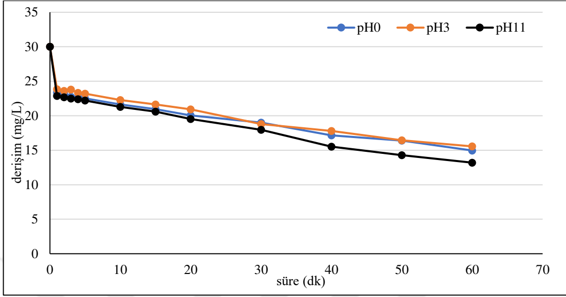
Şekil 6.57. %80IrO 2 -%20RuO 2 kaplı paralel plaka titanyum elektrotlarla, C_0 :30 mg/L, 200 A/m 2 akım yoğunluğunda, 155,84 mL/dk akış hızında, 0,02 M \text{Na}_2\text{SO}_4 derişiminde, pH 0 (6,04), pH 3 ve pH 11 'de olan koşullarda elde edilen arıtım verimleri
