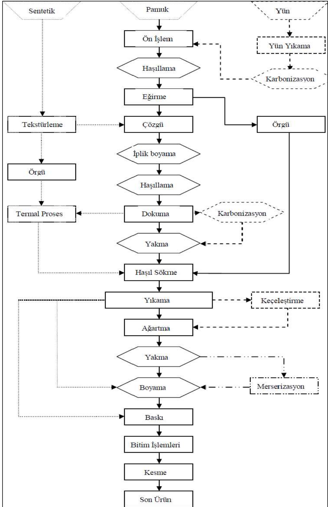
Şekil 3.1. Tekstil endüstrisinde yer alan genel proses basamakları (Cırık, 2010)
