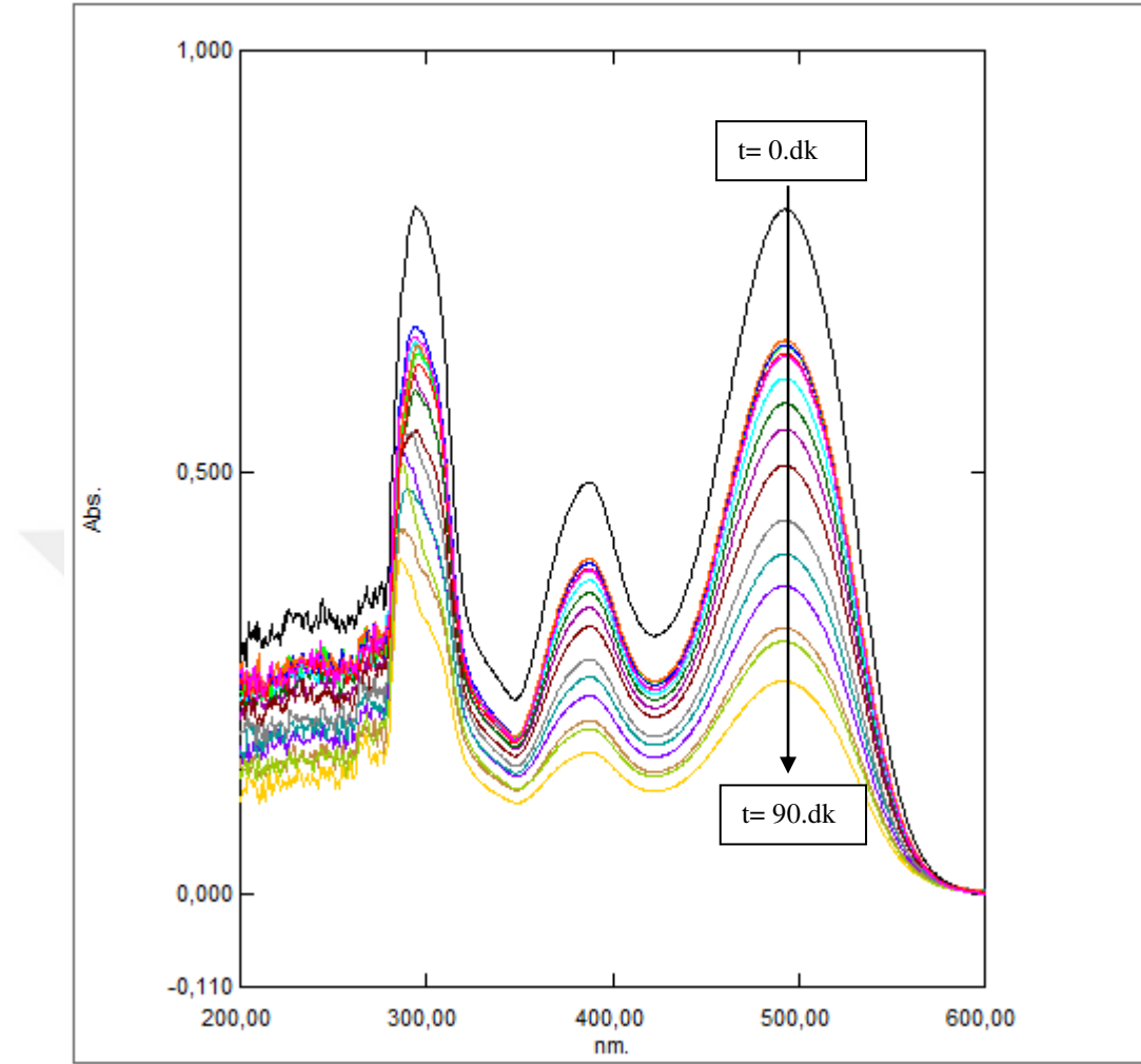
Şekil 6.135. Ti/RuO 2 kaplı paralel plaka elektrotlarla, 125 mg/L başlangıç kirlilik derişimi için; 150 A/m 2 akım yoğunluğunda, 155,84 mL/dk akış hızında, 0,01 M NaNO 3 elektrolit miktarı ve pH 0 'de UV-Spektrum grafiğı
