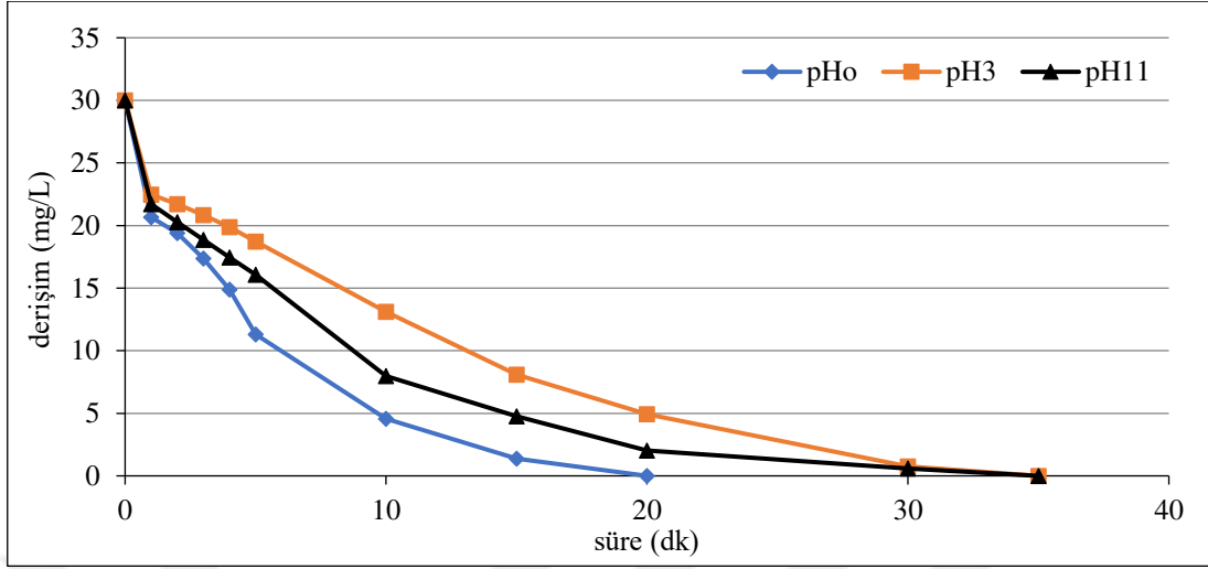
Şekil 6.33. Ti/IrO 2 kaplı paralel plaka elektrotlarla, C 0 :30 mg/L, 50 A/m 2 akım yoğunluğunda, 175,7 mL/dk akış hızında, 0,05 M NaCl derişiminde, pH 0 (5,71), pH 3 ve pH 11 'de olan koşullarda elde edilen arıtım verimleri
