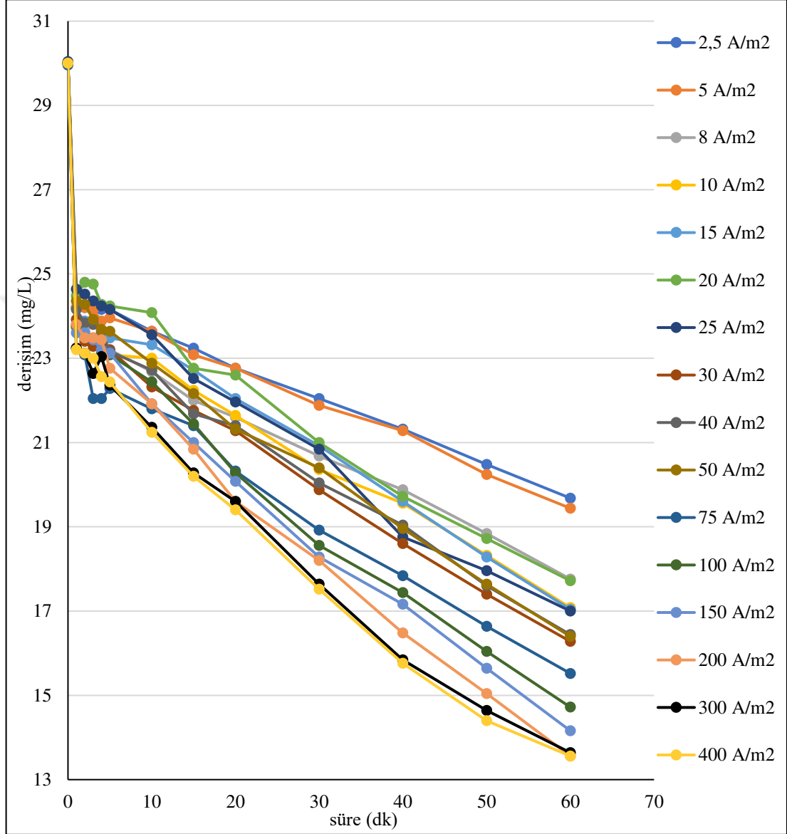
Şekil 6.71. %20IrO 2 -%80RuO 2 kaplı paralel plaka titanyum elektrotlarla, C_0 :30 mg/L, 2,5/5/8/10/15/20/25/30/40/50/75/100/150/200/300/400 A/m 2 akım yoğunluklarında, 155,84 mL/dk akış hızında, 0,01 M Na 2 SO 4 , pH 0 : 6,15-6,70 aralığında olan koşullarda elde edilen arıtım verimleri
