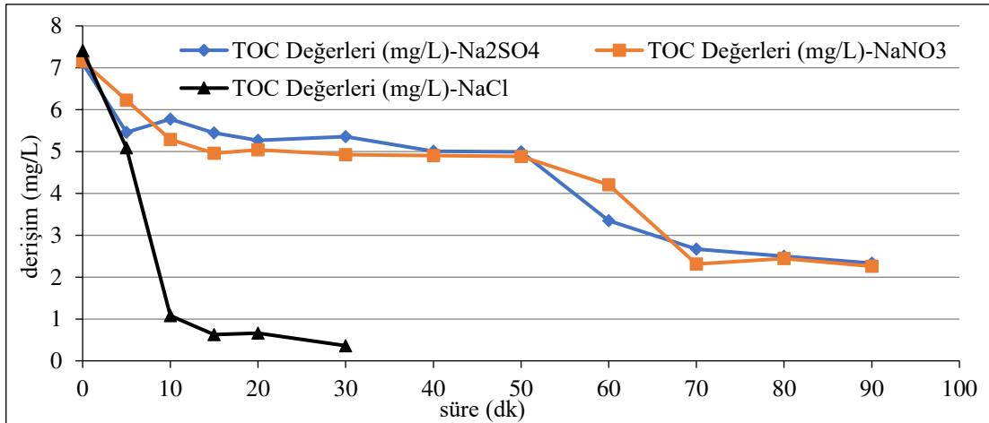
Şekil 6.171. %60IrO 2 -%40RuO 2 kaplı paralel plaka titanyum elektrotlarla, başlangıç kirlilik derişimi 30 mg/L, 400 A/m 2 akım yoğunluğu, 155,84 mL/dk akış hızı, 0,01 M Na 2 SO 4 elektrolit derişimi, pH 11 : 11'de; 500 A/m 2 akım yoğunluğu, 155,84 mL/dk akış hızı, 0,01 M NaNO 3 elektrolit derişimi, pH 0 'da; 75 A/m 2 akım yoğunluğu, 155,84 mL/dk akış hızı, 0,05 M NaCl elektrolit derişimi, pH 0 olan koşullarda elde edilen TOC sonuçları
