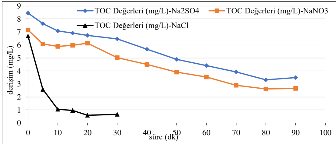
Şekil 6.173. %40IrO 2 -%60RuO 2 kaplı paralel plaka titanyum elektrotlarla, başlangıç kirlilik derişimi 30 mg/L, 300 A/m 2 akım yoğunluğu, 155,84 mL/dk akış hızı, 0,01 M Na 2 SO 4 elektrolit derişimi, pH 11 : 11'de; 500 A/m 2 akım yoğunluğu, 155,84 mL/dk akış hızı, 0,01 M NaNO 3 elektrolit derişimi, pH 0 'da; 75 A/m 2 akım yoğunluğu, 155,84 mL/dk akış hızı, 0,05 M NaCl elektrolit derişimi, pH 0 olan koşullarda elde edilen TOC sonuçları
