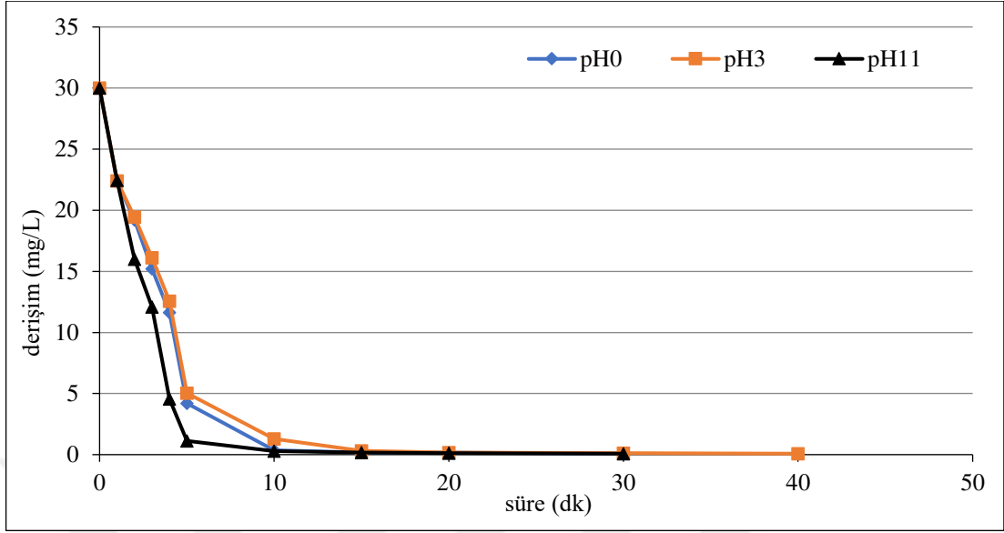
Şekil 6.101. %60IrO 2 -%40RuO 2 kaplı paralel plaka titanyum elektrotlarla, C o :30 mg/L, 75 A/m 2 akım yoğunluğunda, 155,84 mL/dk akış hızında, 0,05 M NaCl derişimlerinde, pH 0 (6,26), pH 3 ve pH 11 ’de olan koşullarda elde edilen arıtım verimleri
