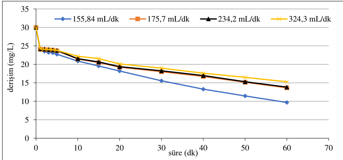
Şekil 6.95. %20IrO 2 -%80RuO 2 kaplı paralel plaka titanyum elektrotlarla, C 0 :30 mg/L, 500 A/m 2 akım yoğunluğu, 155,84 mL/dk, 175,7 mL/dk, 234,2 mL/dk, 324,3 mL/dk akış hızlarında, 0,01 M NaNO 3 , pH 0 : 6,14-6,16 aralığında olan koşullarda elde edilen arıtım verimleri
