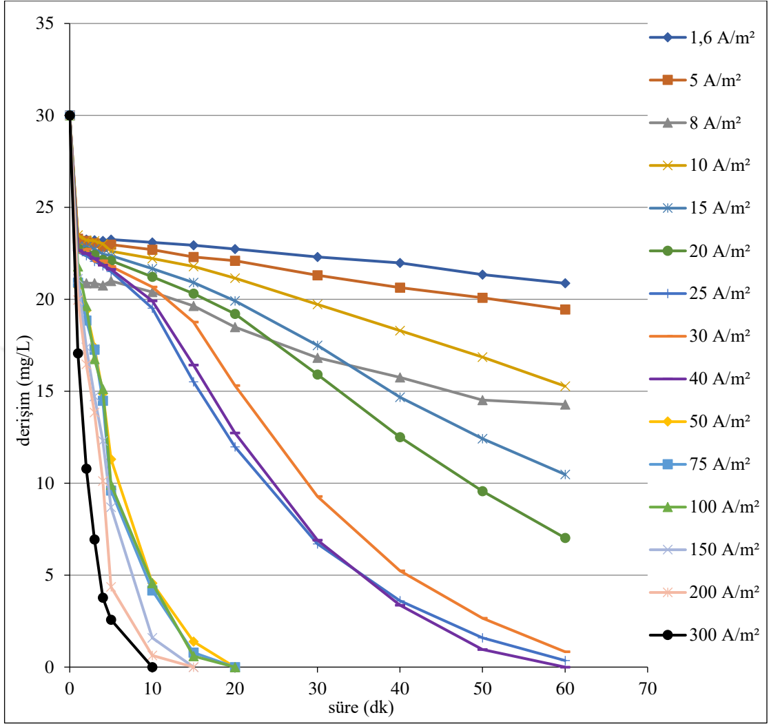
Şekil 6.30. Ti/IrO 2 kaplı paralel plaka elektrotlarla, C 0 :30 mg/L, 1,6/5/8/10/15/20/25/30/40/50/75/100/150/200/300 A/m 2 akım yoğunluklarında, 175,7 mL/dk akış hızında, 0,05 M NaCl, pH 0 : 5,16-6,10 olan koşullarda elde edilen arıtım verimleri
