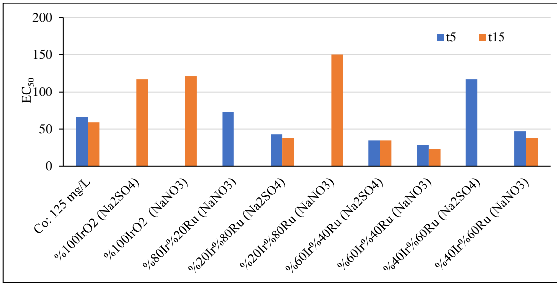
Şekil 6.175. IrO 2 /RuO 2 kaplı titanyum elektrotlarla, başlangıç kirlilik derişimi 125 mg/L olduğu durumda Na 2 SO 4 ve NaNO 3 elektrolitleri ile optimum koşullarda elde edilen numunelerin toksisite grafiğı (Grafik her bir deneyin 90.dk'sı ile elde edilen numunelerin toksisite değerlerini göstermektedir. 1. Sütun t 5 ve 2. Sütun t 15 değerlerine karşılık gelmektedir.)
