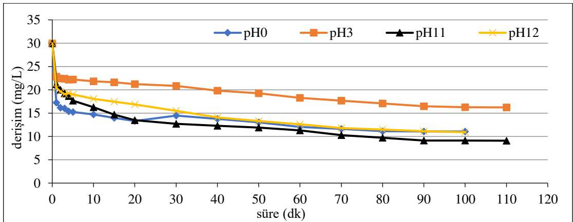
Şekil 6.6. Grafit plaka elektrotlarla, C_0 :30 mg/L, 8 A/m 2 akım yoğunluğu, 0,01 M Na 2 SO 4 , 155,84 mL/dk akış hızında pH 0 (6,29), pH 3 , pH 11 ve pH 12 olan koşullarda arıtım verimleri
