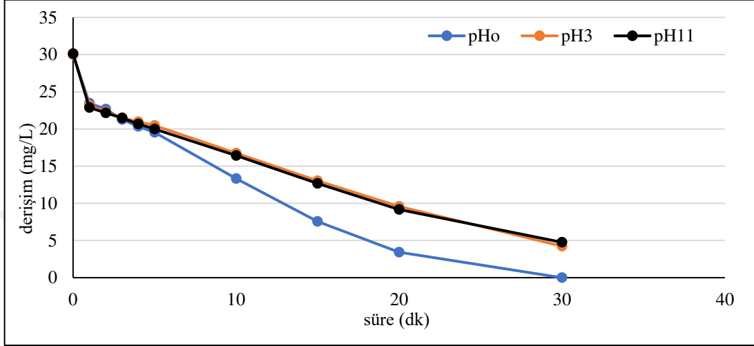
Şekil 6.16. Grafit plaka elektrotlarla, Co:30 mg/L, 40 A/m 2 akım yoğunluğu, 155,84 mL/dk akış hızı, 0,08 M NaCl, pH 0 (6,19), pH 3 ve pH 11 olan koşullarda arıtım verimleri
