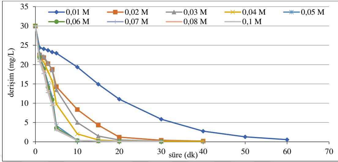
Şekil 6.99. %60IrO 2 -%40RuO 2 kaplı paralel plaka titanyum elektrotlarla, C_o :30 mg/L, 75 A/m 2 akım yoğunluğunda, 155,84 mL/dk akış hızında, 0,01/0,02/0,03/0,04/0,05/0,06/0,07/0,08/0,1 M NaCl derişimlerinde, pH 0 : 6,15-6,29 aralığında olan koşullarda elde edilen arıtım verimleri
