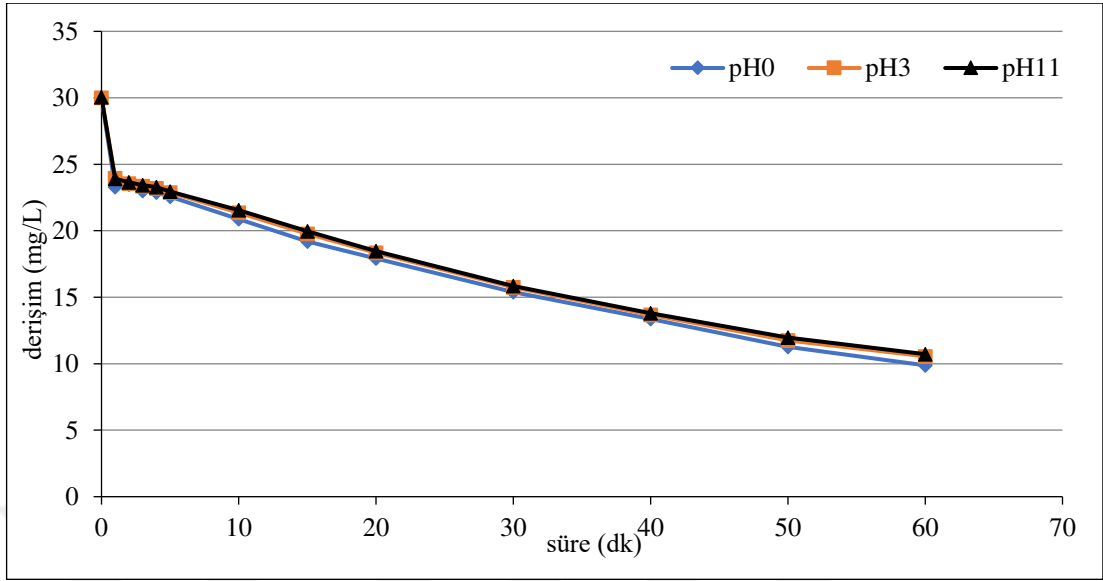
Şekil 6.96. %60IrO 2 -%40RuO 2 kaplı paralel plaka titanyum elektrotlarla, C_0 :30 mg/L, 500 A/m 2 akım yoğunluğunda, 155,84 mL/dk akış hızında, 0,01 M \text{NaNO}_3 derişiminde, pH 0 (6,19), pH 3 ve pH 11 'de olan koşullarda elde edilen arıtım verimleri
