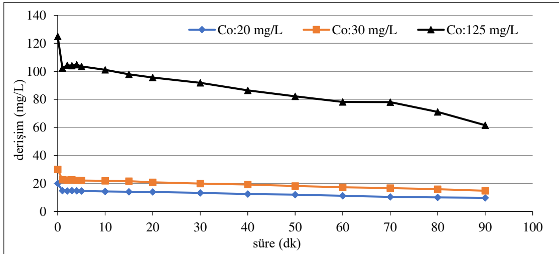
Şekil 6.29. \text{Ti/IrO}_2 kaplı paralel plaka elektrotlarla, 50 \text{ A/m}^2 akım yoğunluğunda, 155,84 mL/dk akış hızında, başlangıç kirlilik derişimleri 20 mg/L, 30 mg/L ve 125 mg/L, 0,01 M \text{NaNO}_3 elektrolit derişiminde, \text{pH}_0 : 5,94-6,15'teki koşullarda elde edilen arıtım verimleri
