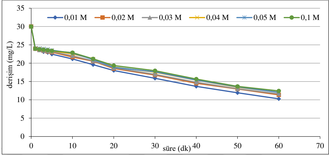
Şekil 6.111. %40 \text{IrO}_2 -%60 \text{RuO}_2 kaplı paralel plaka titanyum elektrotlarla, C_o :30 mg/L, 500 A/m 2 akım yoğunluğunda, 155,84 mL/dk akış hızında, 0,01/0,02/0,03/0,04/0,05/0,1 M \text{NaNO}_3 derişimlerinde, pH 0 : 6,14-6,24 aralığında olan koşullarda elde edilen arıtım verimleri
