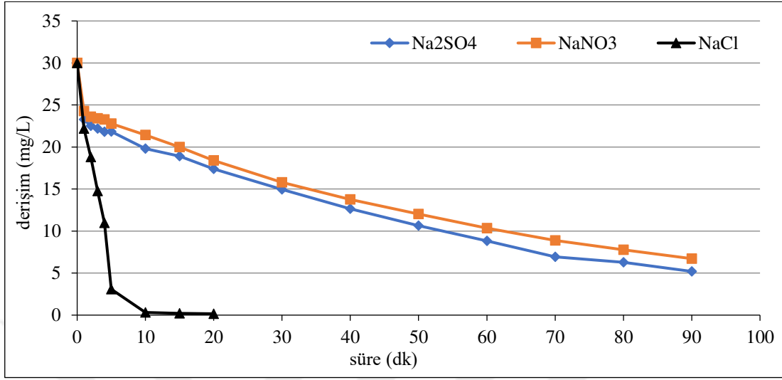
Şekil 6.120. %40 \text{IrO}_2 -%60 \text{RuO}_2 kaplı paralel plaka titanyum elektrotlarla, C_0 :30 mg/L \text{Na}_2\text{SO}_4 için; 300 \text{A/m}^2 akım yoğunluğu, 155,84 mL/dk akış hızı, 0,01 M \text{Na}_2\text{SO}_4 elektrolit miktarı, \text{pH}_{11} olan koşullarda; \text{NaNO}_3 için; 500 \text{A/m}^2 akım yoğunluğu, 155,84 mL/dk akış hızı, 0,01 M \text{NaNO}_3 elektrolit miktarı, \text{pH}_0 (6,14) olan koşullarda, \text{NaCl} için; 75 \text{A/m}^2 akım yoğunluğu, 155,84 mL/dk akış hızı, 0,05 M \text{NaCl} elektrolit miktarı, \text{pH}_0 (6,05) olan koşullarda elde edilen arıtım verimleri
