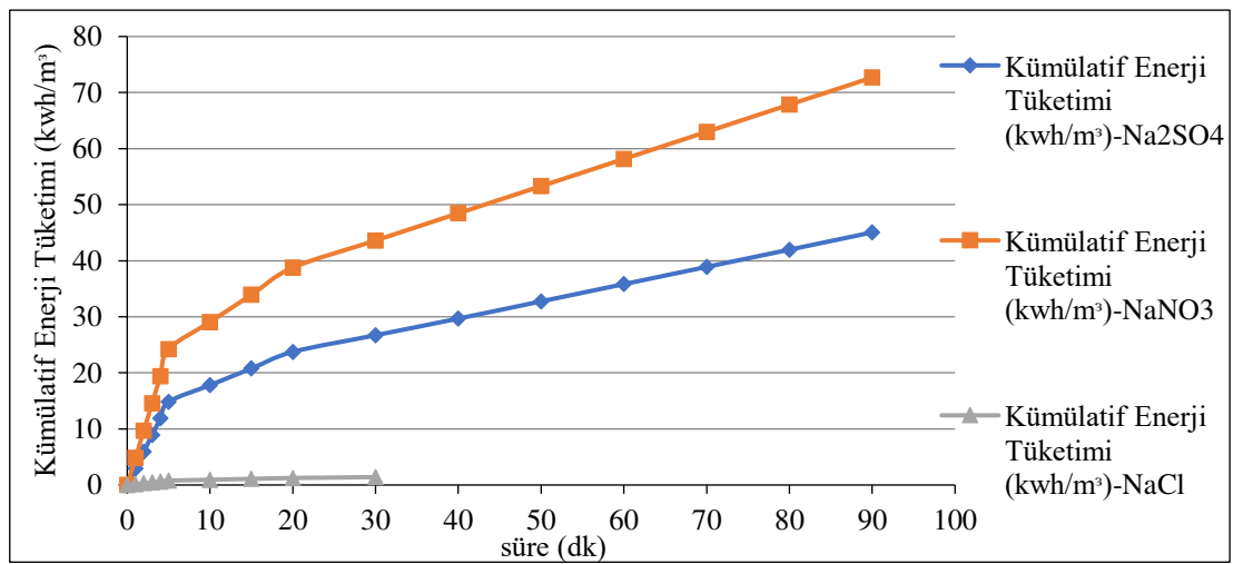
Şekil 6.191. %60IrO 2 -%40RuO 2 kaplı paralel plaka titanyum elektrotlarla, başlangıç kirlilik derişimi 30 mg/L olduğu durumda Na 2 SO 4 , NaNO 3 ve NaCl elektrolitleri ile optimum koşullarda oluşan enerji tüketim grafiği
