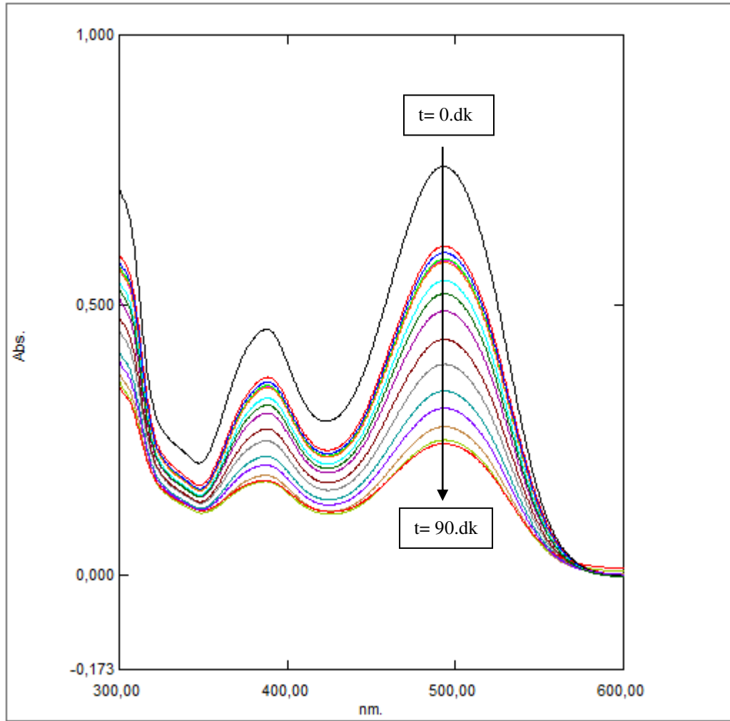
Şekil 6.144. %20IrO 2 -%80RuO 2 kaplı paralel plaka titanyum elektrotlarla, 30 mg/L başlangıç kirlilik derişimi için; 200 A/m 2 akım yoğunluğunda, 155,84 mL/dk akış hızında, 0,01 M Na 2 SO 4 elektrolit miktarı ve pH 11 'de UV-Spektrum grafiği
