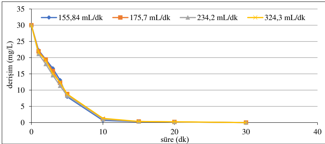
Şekil 6.66. %80IrO 2 -%20RuO 2 kaplı paralel plaka titanyum elektrotlarla, C o :30 mg/L, 75 A/m 2 akım yoğunluğu, 155,84 mL/dk, 175,7 mL/dk, 234,2 mL/dk, 324,3 mL/dk akış hızlarında, 0,05 M NaCl, pH 0 : 6,34-6,45 aralığında olan koşullarda elde edilen arıtım verimleri
