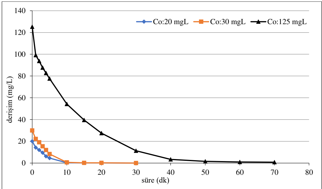
Şekil 6.85. %20IrO 2 -%80RuO 2 kaplı paralel plaka titanyum elektrotlarla, 75 A/m 2 akım yoğunluğunda, 155,84 mL/dk akış hızında, başlangıç kirlilik derişimleri 20 mg/L, 30 mg/L ve 125 mg/L olan 0,04 M NaCl elektrolit derişiminde, pH 0 (6,14-6,27) olan koşullarda elde edilen arıtım verimleri
