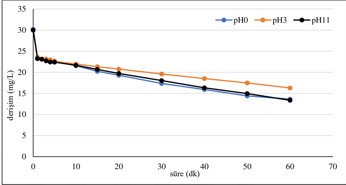
Şekil 6.40. \text{Ti/RuO}_2 kaplı paralel plaka elektrotlarla, C_0 :30 mg/L, 150 \text{ A/m}^2 akım yoğunluğunda, 155,84 \text{ mL/dk} akış hızında, 0,01 \text{ M Na}_2\text{SO}_4 derişiminde, \text{pH}_0 (6,78), \text{pH}_3 ve \text{pH}_{11} 'de olan koşullarda elde edilen arıtım verimleri
