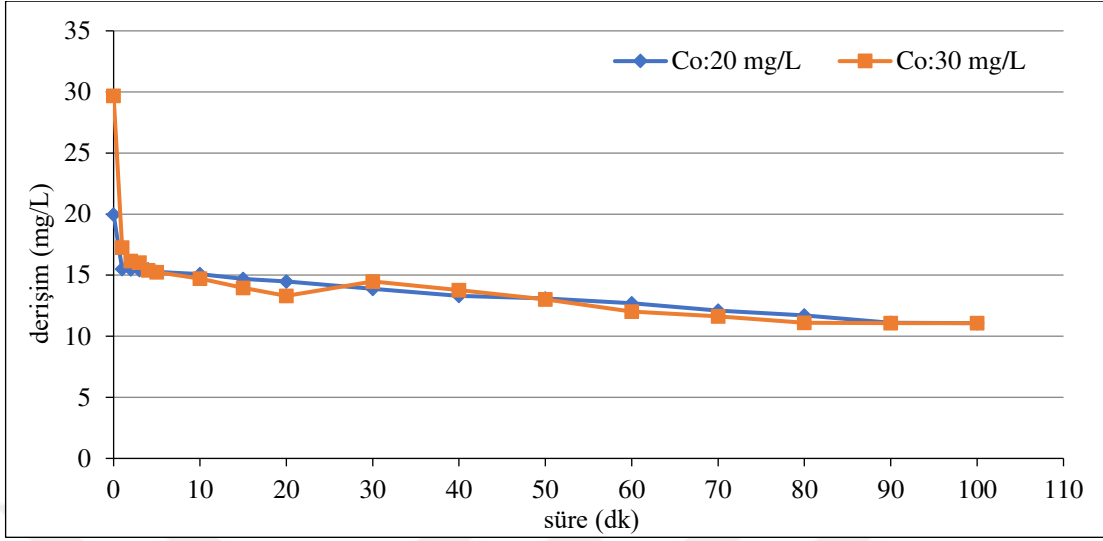
Şekil 6.7. Grafit plaka elektrotlarla, 8 A/m 2 akım yoğunluğu, 0,01 M Na 2 SO 4 , 155,84 mL/dk akış hızında pH 11 olan koşullarda başlangıç kirlilik derişimi 20 ve 30 mg/L'deki arıtım verimleri
