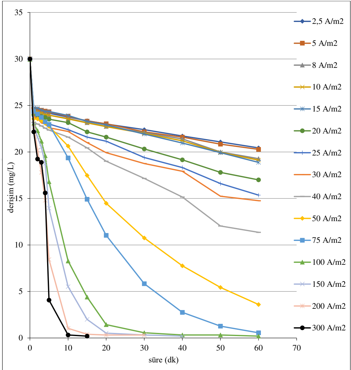
Şekil 6.98. %60IrO 2 -%40RuO 2 kaplı paralel plaka titanyum elektrotlarla, C 0 :30 mg/L, 2,5/5/8/10/15/20/25/30/40/50/75/100/150/200/300 A/m 2 akım yoğunluklarında, 155,84 mL/dk akış hızında, 0,01 M NaCl, pH 0 : 6,01-6,27 aralığında olan koşullarda elde edilen arıtım verimleri
