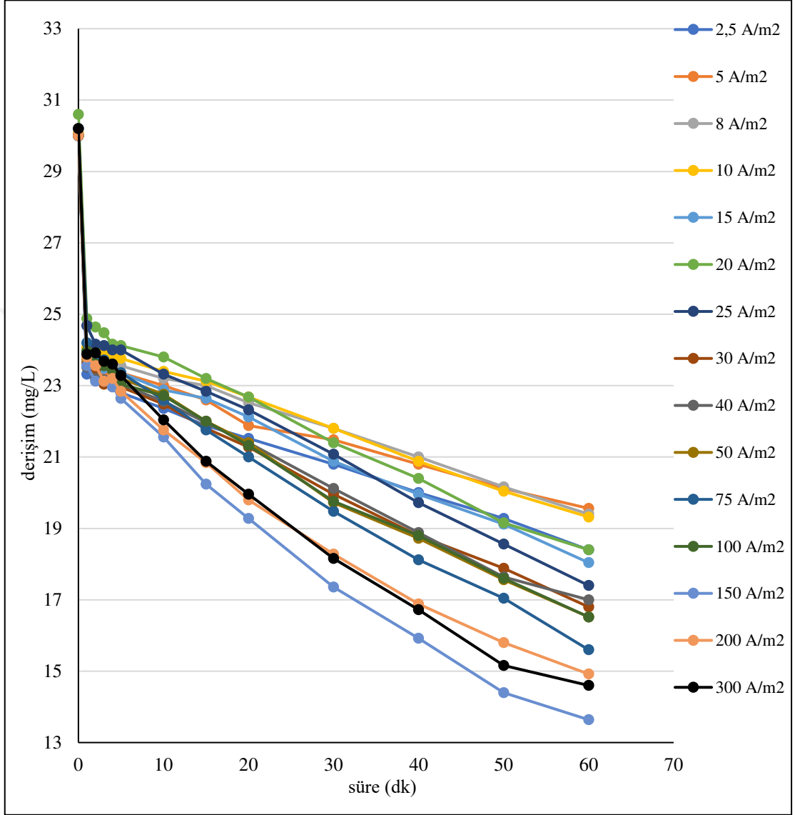
Şekil 6.37. Ti/RuO 2 kaplı paralel plaka elektrotlarla, C 0 :30 mg/L, 2,5/5/8/10/15/20/25/30/40/50/75/100/150/200/300 A/m 2 akım yoğunluklarında, 155,84 mL/dk akış hızında, 0,01 M Na 2 SO 4 , pH 0 : 6,12-6,87 aralığında olan koşullarda elde edilen arıtım verimleri
