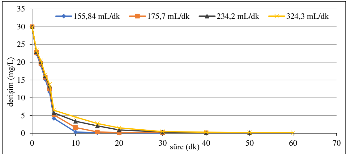
Şekil 6.100. %60IrO 2 -%40RuO 2 kaplı paralel plaka titanyum elektrotlarla, C_o :30 mg/L, 75 A/m 2 akım yoğunluğu, 155,84 mL/dk, 175,7 mL/dk, 234,2 mL/dk, 324,3 mL/dk akış hızlarında, 0,05 M NaCl, pH 0 : 6,23-6,26 aralığında olan koşullarda elde edilen arıtım verimleri
