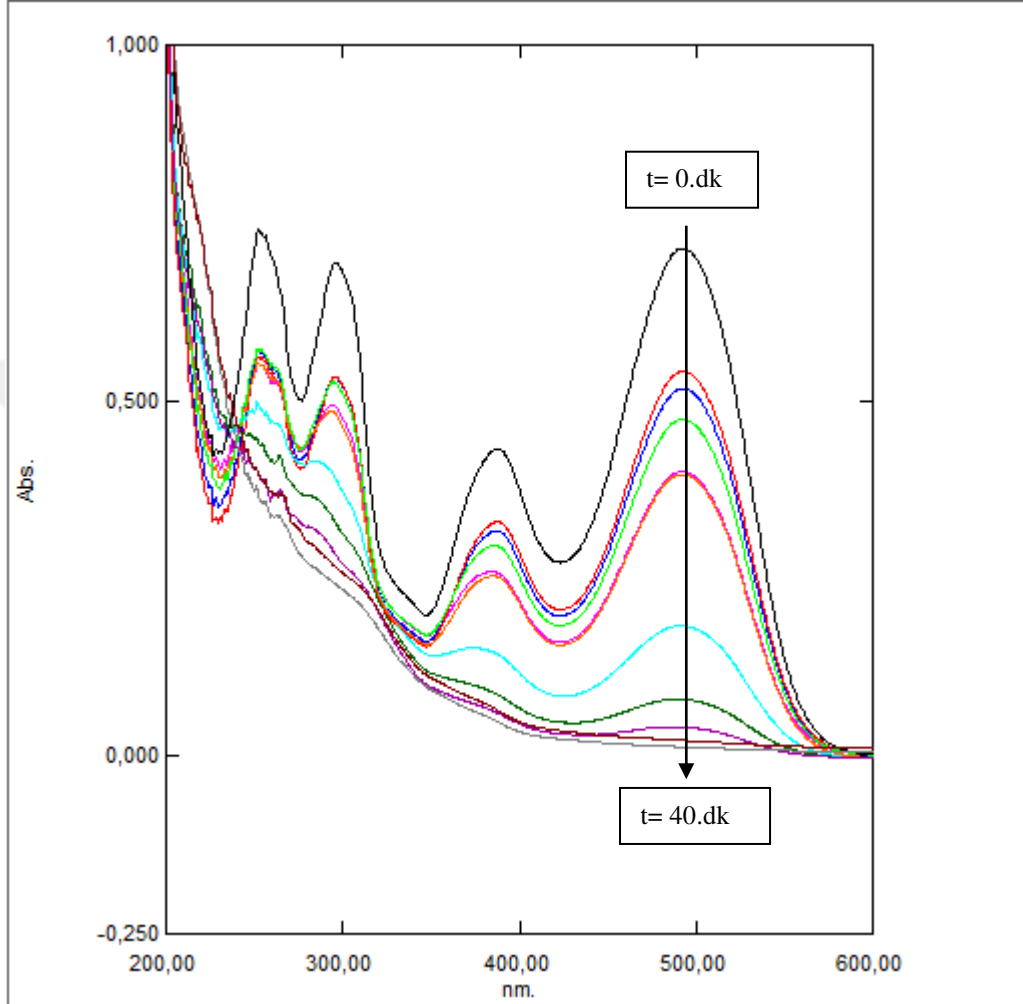
Şekil 6.130. Ti/IrO 2 kaplı paralel plaka elektrotlarla, 30 mg/L başlangıç kirlilik derişimi için; 50 A/m 2 akım yoğunluğunda, 175,7 mL/dk akış hızında, 0,05 M NaCl elektrolit miktarı ve pH 0 'de UV-Spektrum grafiği
