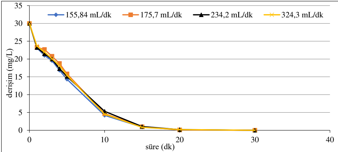
Şekil 6.49. Ti/RuO 2 kaplı paralel plaka elektrotlarla, C o :30 mg/L, 50 A/m 2 akım yoğunluğu, 155,84 mL/dk, 175,7 mL/dk, 234,2 mL/dk, 324,3 mL/dk akış hızlarında, 0,06 M NaCl, pH 0 : 6-6,27 aralığında olan koşullarda elde edilen arıtım verimleri
