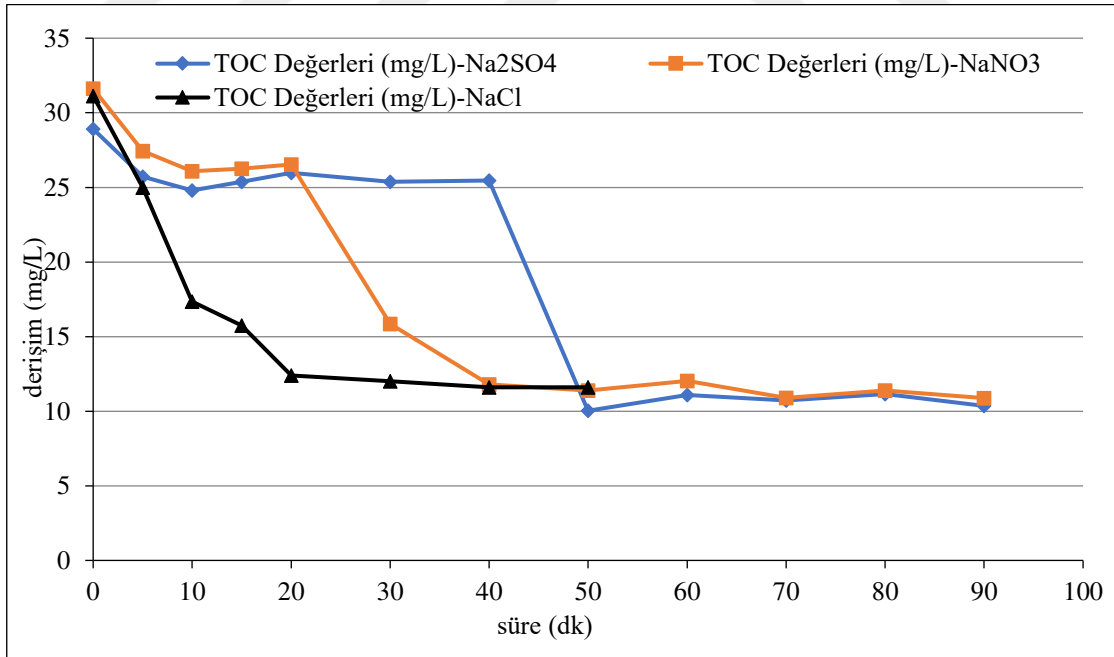
Şekil 6.168. %80IrO 2 -%20RuO 2 kaplı paralel plaka titanyum elektrotlarla, başlangıç kirlilik derişimi 125 mg/L, 200 A/m 2 akım yoğunluğu, 155,84 mL/dk akış hızı, 0,02 M Na 2 SO 4 elektrolit derişimi, pH 11 : 11'de; 400 A/m 2 akım yoğunluğu, 155,84 mL/dk akış hızı, 0,01 M NaNO 3 elektrolit derişimi, pH 0 'da; 75 A/m 2 akım yoğunluğu, 155,84 mL/dk akış hızı, 0,05 M NaCl elektrolit derişimi, pH 0 olan koşullarda elde edilen TOC sonuçları
