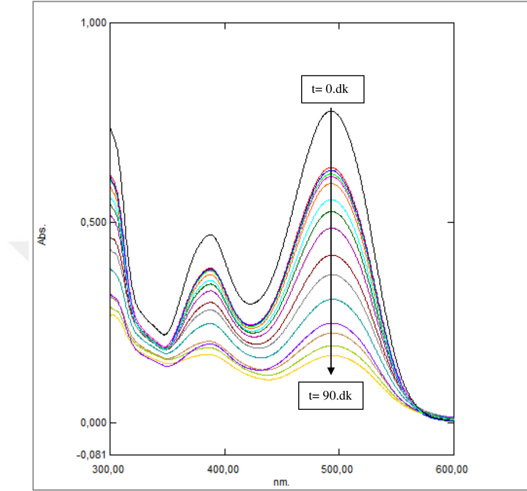
Şekil 6.153. %60IrO 2 -%40RuO 2 kaplı paralel plaka titanyum elektrotlarla, 125 mg/L başlangıç kirlilik derişimi için; 500 A/m 2 akım yoğunluğunda, 155,84 mL/dk akış hızında, 0,01 M NaNO 3 elektrolit miktarı ve pH 0 'da UV-Spektrum grafiğı
