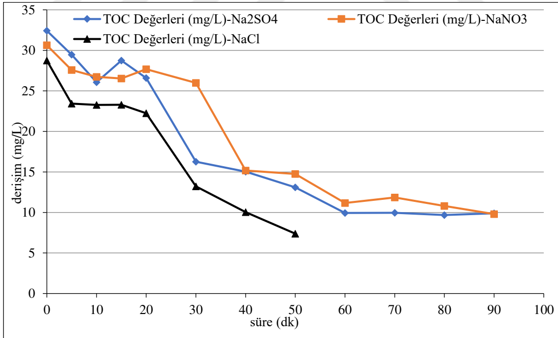
Şekil 6.170. %20IrO 2 -%80RuO 2 kaplı paralel plaka titanyum elektrotlarla, başlangıç kirlilik derişimi 125 mg/L, 200 A/m 2 akım yoğunluğu, 155,84 mL/dk akış hızı, 0,01 M Na 2 SO 4 elektrolit derişimi, pH 11 : 11'de; 400 A/m 2 akım yoğunluğu 155,84 mL/dk akış hızı, 0,01 M NaNO 3 elektrolit derişimi, pH 0 'da; 75 A/m 2 akım yoğunluğu, 155,84 mL/dk akış hızı, 0,04 M NaCl elektrolit derişimi, pH 0 olan koşullarda elde edilen TOC sonuçları
