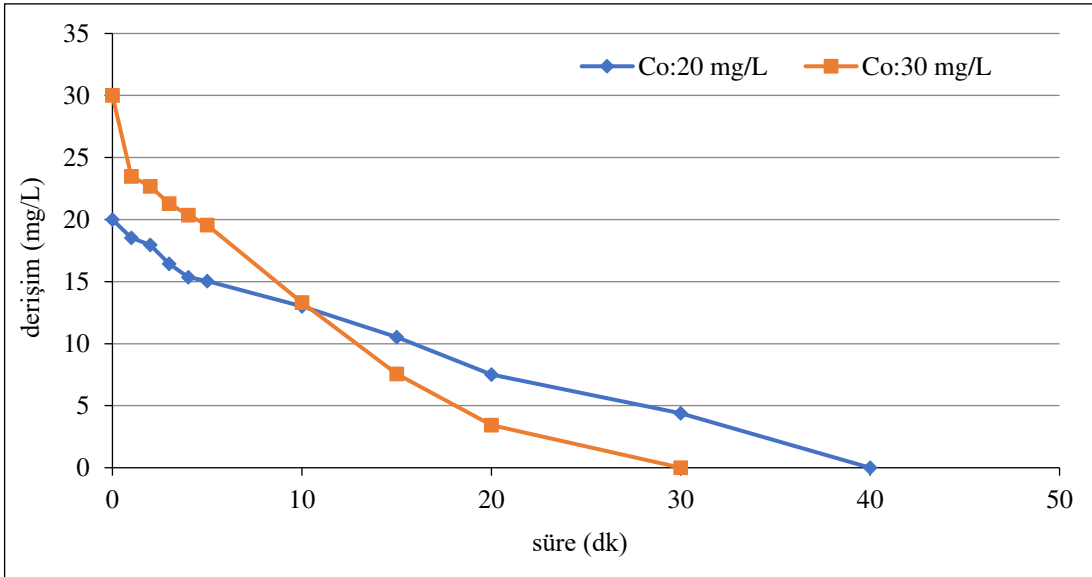
Şekil 6.17. Grafit plaka elektrotlarla, 40 A/m 2 akım yoğunluğu, 155,84 mL/dk akış hızı, 0,08 M NaCl, pH 0 'da (6,19-6,25) başlangıç kirlilik derişimi Co: 20 mg/L ve Co: 30 mg/L olan koşullarda arıtım verimleri
