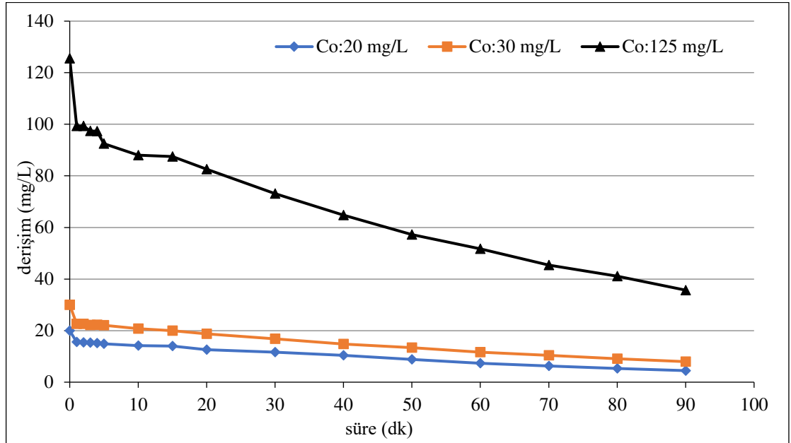
Şekil 6.92. %60IrO 2 -%40RuO 2 kaplı paralel plaka titanyum elektrotlarla, 400 A/m 2 akım yoğunluğunda, 155,84 mL/dk akış hızında, başlangıç kirlilik derişimleri 20 mg/L, 30 mg/L ve 125 mg/L olan 0,01 M \text{Na}_2\text{SO}_4 elektrolit derişiminde, pH 11 olan koşullarda elde edilen arıtım verimleri
