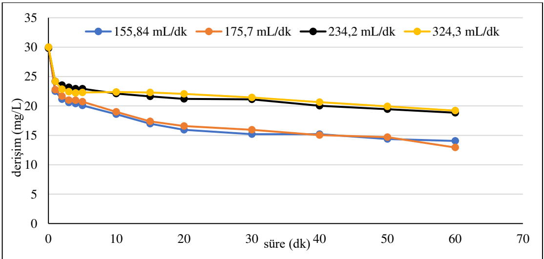
Şekil 6.10. Grafit plaka elektrotlarla, C_o :30 mg/L, 8 \text{ A/m}^2 akım yoğunluğu, 0,01 M \text{NaNO}_3 , 155,84 mL/dk, 175,7 mL/dk, 234,2 mL/dk, 324,3 mL/dk akış hızlarında \text{pH}_0 : 8,55 olan koşullarda arıtım verimleri
