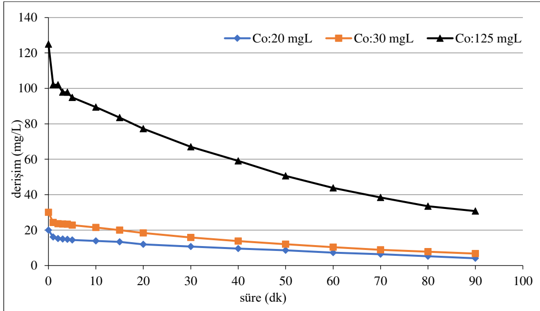
Şekil 6.114. %40IrO 2 -%60RuO 2 kaplı paralel plaka titanyum elektrotlarla, 500 A/m 2 akım yoğunluğunda, 155,84 mL/dk akış hızında, başlangıç kirlilik derişimleri 20 mg/L, 30 mg/L ve 125 mg/L olan 0,01 M \text{NaNO}_3 elektrolit derişiminde, pH 0 (6,13-6,16) olan koşullarda elde edilen arıtım verimleri
