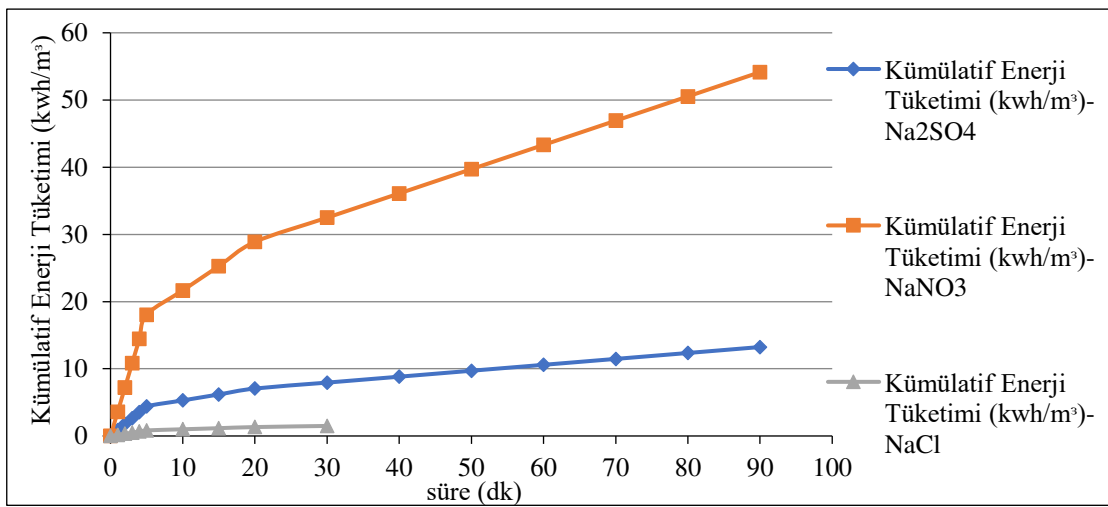
Şekil 6.189. %20IrO 2 -%80RuO 2 kaplı paralel plaka titanyum elektrotlarla, başlangıç kirlilik derişimi 30 mg/L olduğu durumda Na 2 SO 4 , NaNO 3 ve NaCl elektrolitleri ile optimum koşullarda oluşan enerji tüketim grafiği
