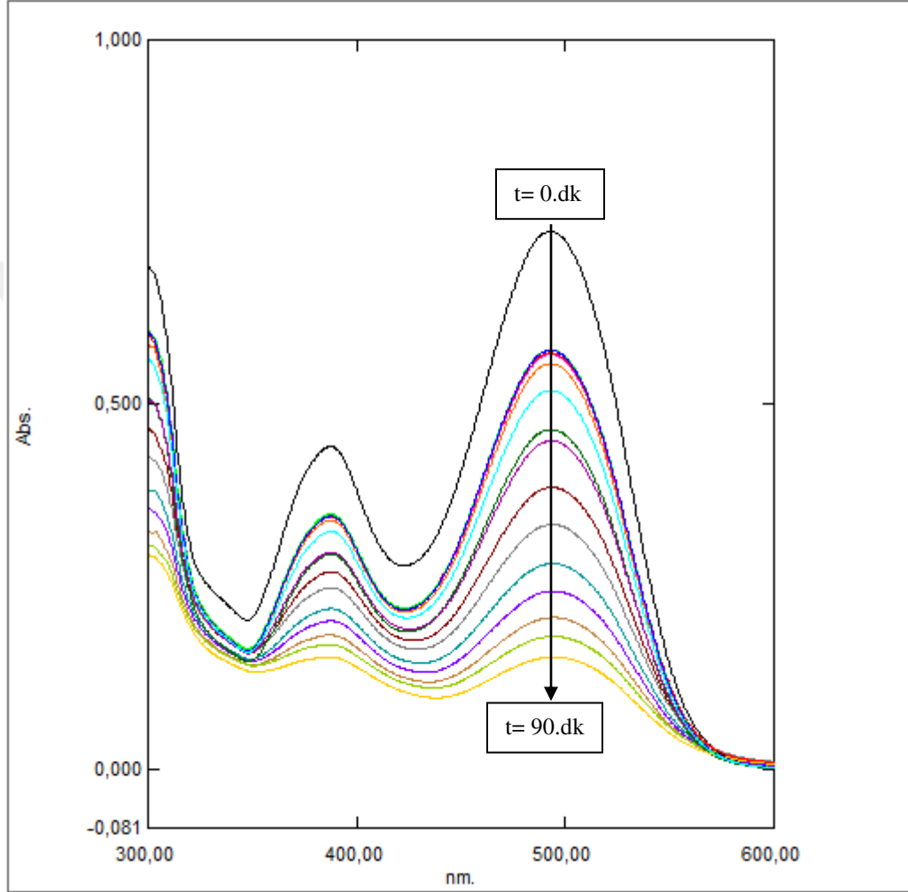
Şekil 6.152. %60IrO 2 -%40RuO 2 kaplı paralel plaka titanyum elektrotlarla, 30 mg/L başlangıç kirlilik derişimi için; 500 A/m 2 akım yoğunluğunda, 155,84 mL/dk akış hızında, 0,01 M NaNO 3 elektrolit miktarı ve pH 0 'da UV-Spektrum grafiğı
