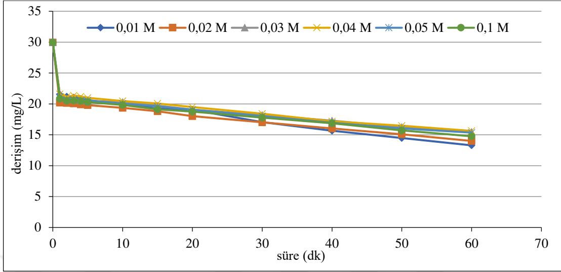
Şekil 6.21. Ti/IrO 2 kaplı paralel plaka elektrotlarla, C 0 :30 mg/L, 50 A/m 2 akım yoğunluğunda, 155,84 mL/dk akış hızında, 0,01/0,02/0,03/0,04/0,05/0,1 M Na 2 SO 4 derişimlerinde, pH 11 olan koşullarda elde edilen arıtım verimleri
