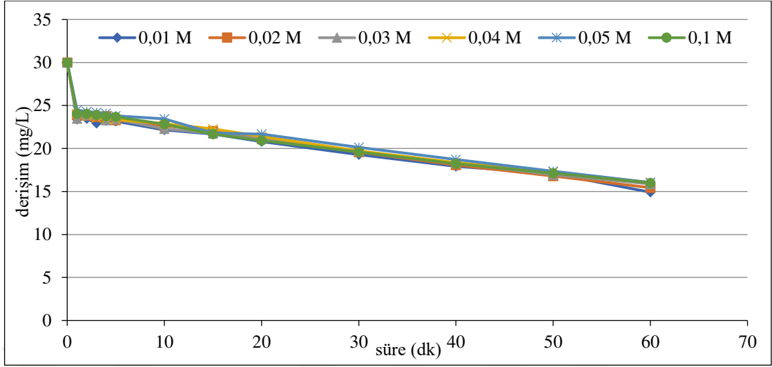
Şekil 6.43. Ti/RuO 2 kaplı paralel plaka elektrotlarla, C 0 :30 mg/L, 150 A/m 2 akım yoğunluğunda, 155,84 mL/dk akış hızında, 0,01/0,02/0,03/0,04/0,05/0,1 M NaNO 3 derişimlerinde, pH 0 : 6,64-7,01 aralığında olan koşullarda elde edilen arıtım verimleri
