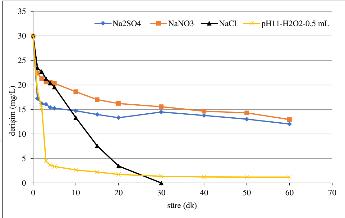
Şekil 6.19. Grafit plaka elektrotlarla, C_o :30 mg/L \text{Na}_2\text{SO}_4 için; 8 A/m 2 akım yoğunluğu, 155,84 mL/dk akış hızı, 0,01 M \text{Na}_2\text{SO}_4 elektrolit miktarı, pH 11 olan koşullarda; \text{Na}_2\text{SO}_4 -H 2 O 2 için; 8 A/m 2 akım yoğunluğu, 155,84 mL/dk akış hızı, 0,01 M \text{Na}_2\text{SO}_4 -0,5 mL H 2 O 2 elektrolit miktarı, pH 11 olan koşullarda \text{NaNO}_3 için; 8 A/m 2 akım yoğunluğu, 175,7 mL/dk akış hızı, 0,01 M \text{NaNO}_3 elektrolit miktarı, pH 0 : 8,25 olan koşullarda, \text{NaCl} için; 40 A/m 2 akım yoğunluğu, 155,84 mL/dk akış hızı, 0,08 M \text{NaCl} elektrolit miktarı, pH 0 : 6,08 olan koşullarda elde edilen arıtım verimleri
