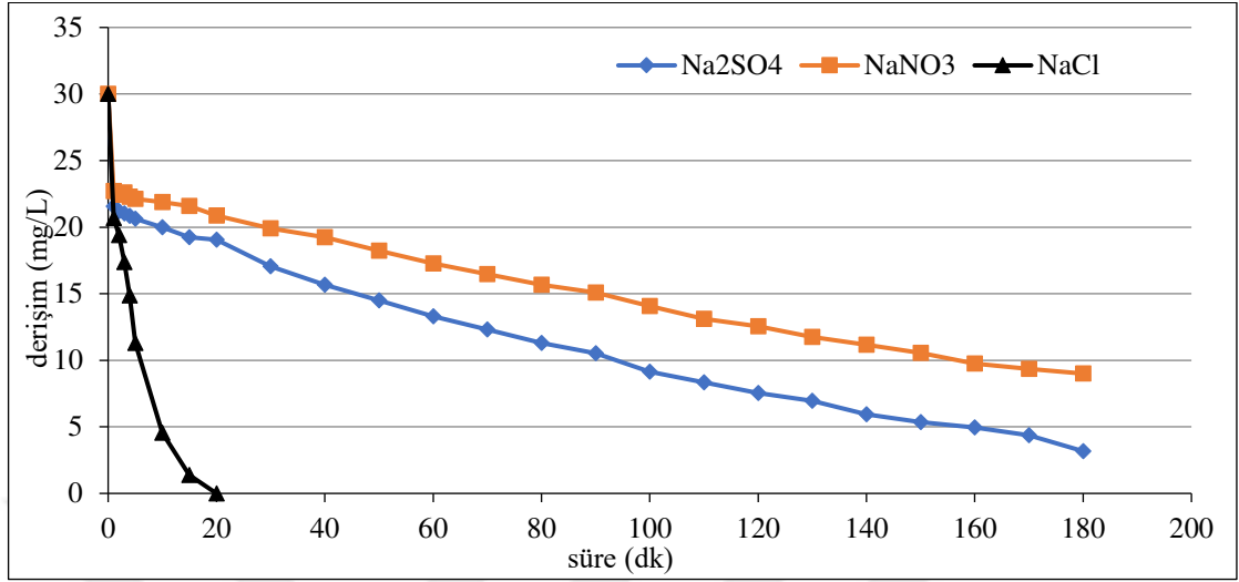
Şekil 6.35. \text{Ti}/\text{IrO}_2 kaplı paralel plaka elektrotlarla, C_0 :30 mg/L \text{Na}_2\text{SO}_4 için; 50 \text{ A/m}^2 akım yoğunluğu, 155,84 mL/dk akış hızı, 0,01 M \text{Na}_2\text{SO}_4 elektrolit miktarı, \text{pH}_{11} olan koşullarda; \text{NaNO}_3 için; 50 \text{ A/m}^2 akım yoğunluğu, 155,84 mL/dk akış hızı, 0,01 M \text{NaNO}_3 elektrolit miktarı, \text{pH}_0 (5,94) olan koşullarda, \text{NaCl} için; 50 \text{ A/m}^2 akım yoğunluğu, 175,7 mL/dk akış hızı, 0,05 M \text{NaCl} elektrolit miktarı, \text{pH}_0 (5,71) olan koşullarda elde edilen arıtım verimleri
