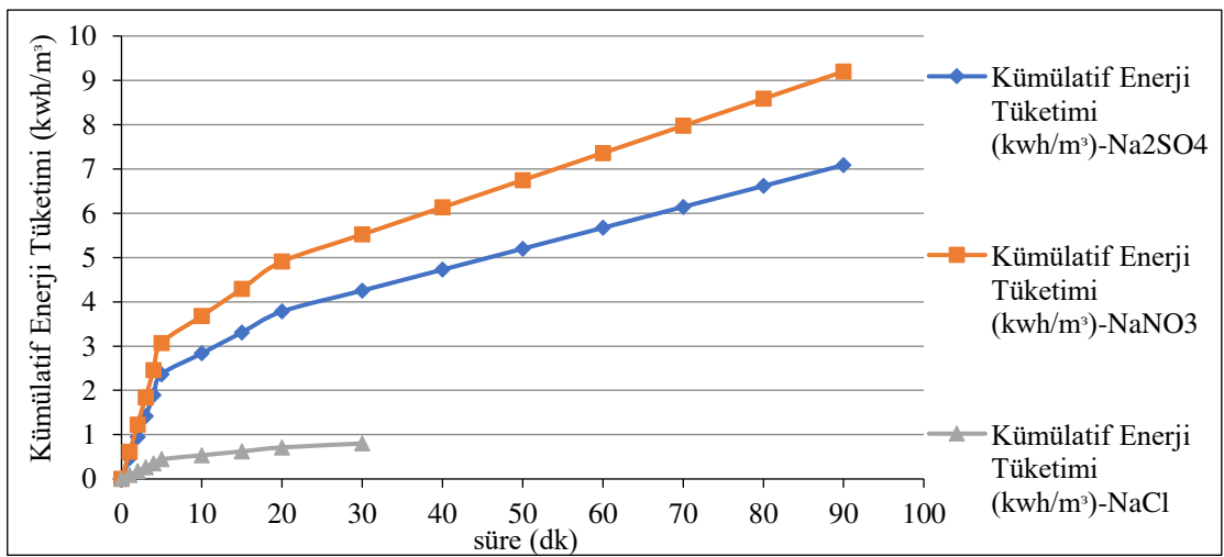
Şekil 6.185. Ti/RuO 2 kaplı paralel plaka elektrotlarla, başlangıç kirlilik derişimi 30 mg/L olduğu durumda Na 2 SO 4 , NaNO 3 ve NaCl elektrolitleri ile optimum koşullarda oluşan enerji tüketim grafiği
