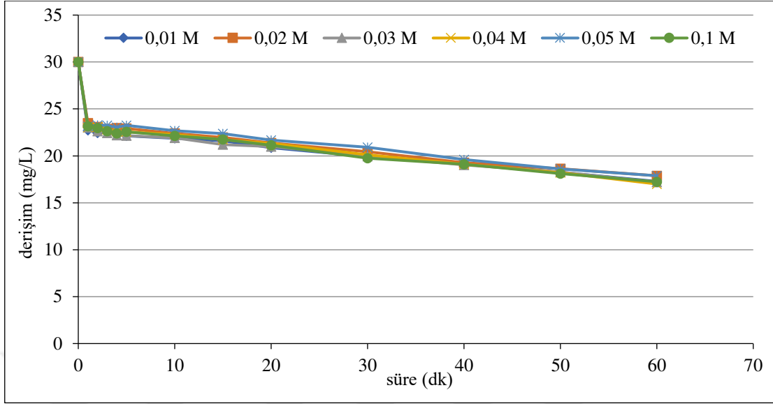
Şekil 6.26. \text{Ti}/\text{IrO}_2 kaplı paralel plaka elektrotlarla, C_0 :30 mg/L, 50 \text{ A/m}^2 akım yoğunluğunda, 155,84 mL/dk akış hızında, 0,01/0,02/0,03/0,04/0,05/0,1 M \text{NaNO}_3 derişimlerinde, \text{pH}_0 : 5,94-6,41 olan koşullarda elde edilen arıtım verimleri
