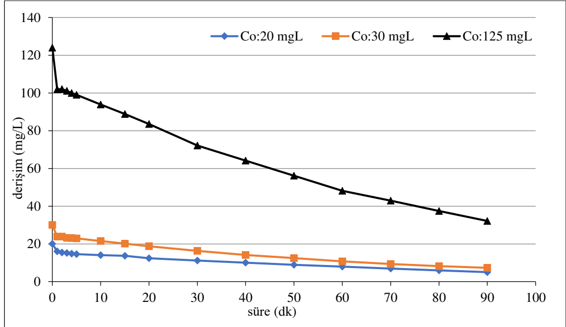
Şekil 6.80. %20 \text{IrO}_2 -%80 \text{RuO}_2 kaplı paralel plaka titanyum elektrotlarla, 400 \text{ A/m}^2 akım yoğunluğunda, 155,84 \text{ mL/dk} akış hızında, başlangıç kirlilik derişimleri 20 mg/L, 30 mg/L ve 125 mg/L olan 0,01 \text{ M NaNO}_3 elektrolit derişiminde, \text{pH}_0 (6,20-6,31) olan koşullarda elde edilen arıtım verimleri
