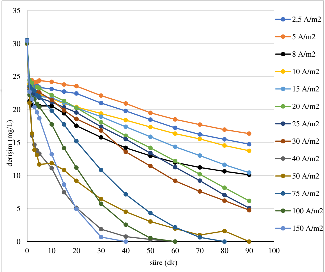
Şekil 6.13. Grafit plaka elektrotlarla, \text{Co} :30 mg/L, 155,84 mL/dk akış hızında 2,5/5/8/10/15/20/25/30/40/50/75/100/150 A/m 2 akım yoğunluğu, başlangıç pH 0 : 5,86-6,53 arasında, 0,05 M NaCl kullanılan koşullarda arıtım verimleri
