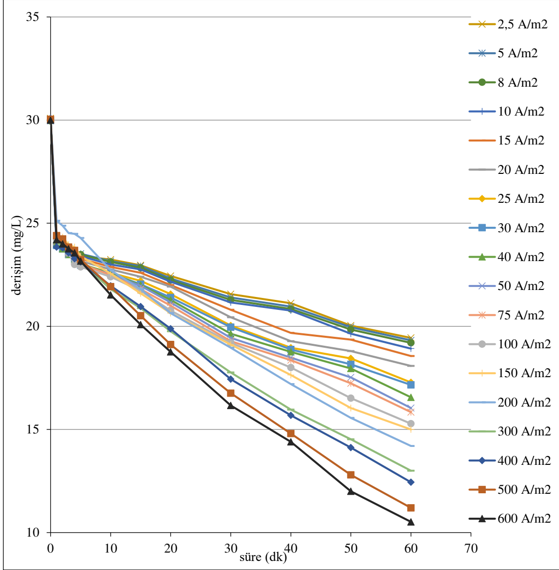
Şekil 6.105. %40IrO 2 -%60RuO 2 kaplı paralel plaka titanyum elektrotlarla, C_0 :30 mg/L, 2,5/5/8/10/15/20/25/30/40/50/75/100/150/200/300/400/500/600 A/m 2 akım yoğunluklarında, 155,84 mL/dk akış hızında, 0,01 M Na 2 SO 4 , pH 0 : 6,09-6,31 aralığında olan koşullarda elde edilen arıtım verimleri
