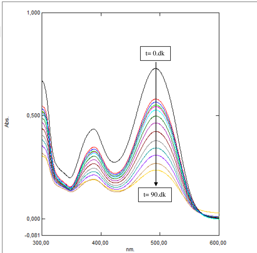
Şekil 6.156. %40IrO 2 -%60RuO 2 kaplı paralel plaka titanyum elektrotlarla, 30 mg/L başlangıç kirlilik derişimi için; 300 A/m 2 akım yoğunluğunda, 155,84 mL/dk akış hızında, 0,01 M Na 2 SO 4 elektrolit miktarı ve pH 11 'de UV-Spektrum grafiği
