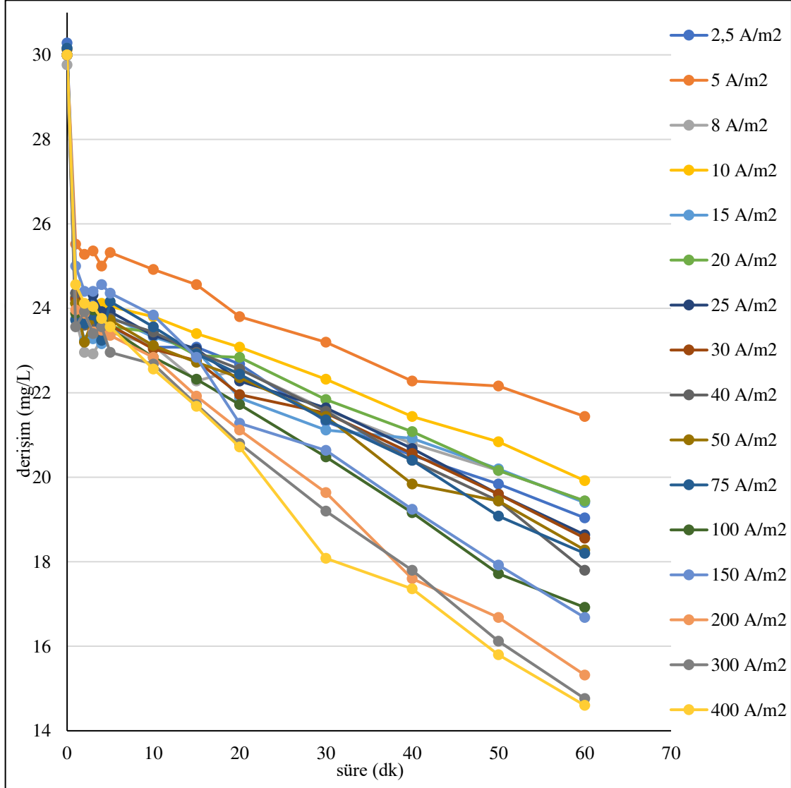
Şekil 6.54. %80IrO 2 -%20RuO 2 kaplı paralel plaka titanyum elektrotlarla, C_o :30 mg/L, 2,5/5/8/10/15/20/25/30/40/50/75/100/150/200/300/400 A/m 2 akım yoğunluklarında, 155,84 mL/dk akış hızında, 0,01 M Na 2 SO 4 , pH 0 : 6,06-6,40 aralığında olan koşullarda elde edilen arıtım verimleri
