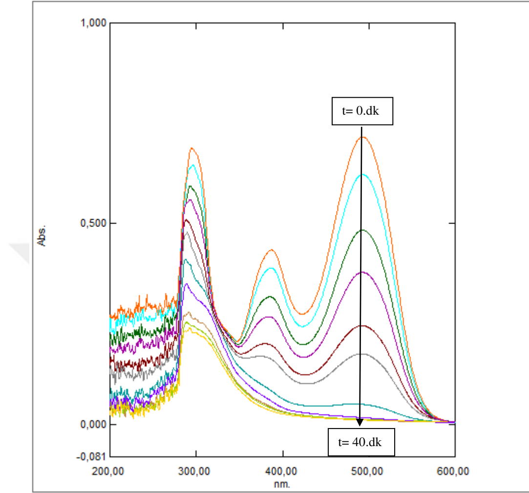
Şekil 6.149. %20IrO 2 -%80RuO 2 kaplı paralel plaka titanyum elektrotlarla, 125 mg/L başlangıç kirlilik derişimi için; 75 A/m 2 akım yoğunluğunda, 155,84 mL/dk akış hızında, 0,04 M NaCl elektrolit miktarı ve pH 0 'de UV-Spektrum grafiğı
