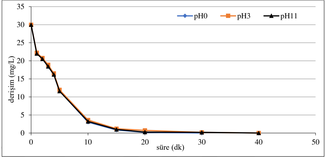
Şekil 6.84. %20IrO 2 -%80RuO 2 kaplı paralel plaka titanyum elektrotlarla, C 0 :30 mg/L, 75 A/m 2 akım yoğunluğunda, 155,84 mL/dk akış hızında, 0,04 M NaCl derişimlerinde, pH 0 (6,27), pH 3 ve pH 11 ’de olan koşullarda elde edilen arıtım verimleri
