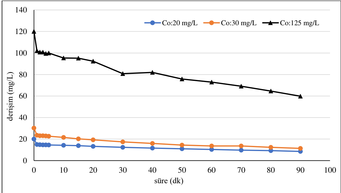
Şekil 6.41. \text{Ti/RuO}_2 kaplı paralel plaka elektrotlarla, 150 \text{ A/m}^2 akım yoğunluğunda, 155,84 \text{ mL/dk} akış hızında, başlangıç kirlilik derişimi 20 mg/L, 30 mg/L ve 125 mg/L olan 0,01 \text{ M Na}_2\text{SO}_4 elektrolit derişiminde, \text{pH}_0 : 6,49-6,78 aralığında olan koşullarda elde edilen arıtım verimleri
