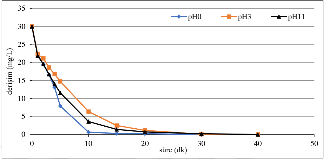
Şekil 6.67. %80IrO 2 -%20RuO 2 kaplı paralel plaka titanyum elektrotlarla, C 0 :30 mg/L, 75 A/m 2 akım yoğunluğunda, 155,84 mL/dk akış hızında, 0,05 M NaCl derişiminde, pH 0 (6,34), pH 3 ve pH 11 'de olan koşullarda elde edilen arıtım verimleri
