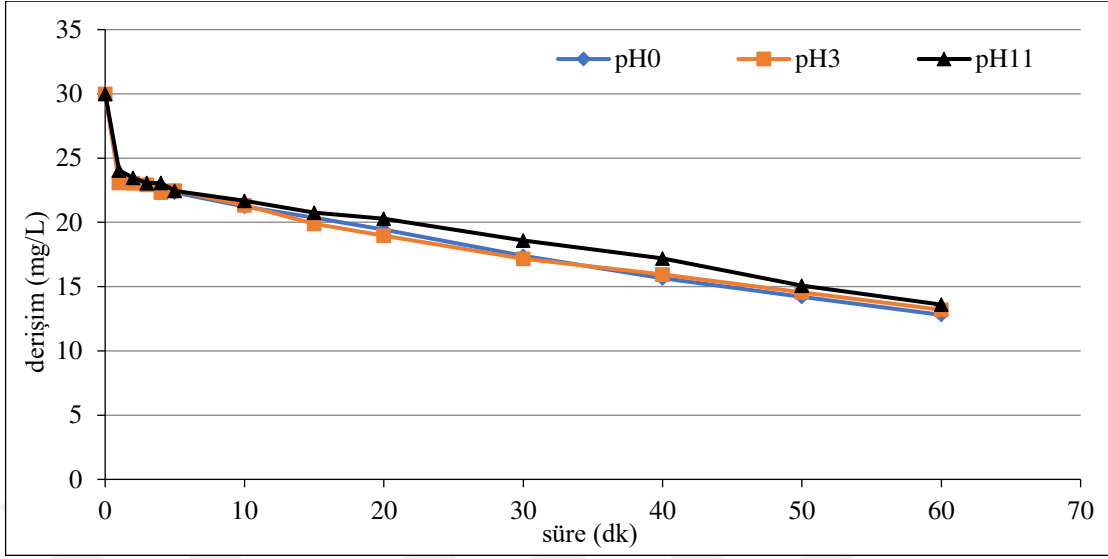
Şekil 6.62. %80IrO 2 -%20RuO 2 kaplı paralel plaka titanyum elektrotlarla, C_0 :30 mg/L, 400 A/m 2 akım yoğunluğunda, 155,84 mL/dk akış hızında, 0,01 M \text{NaNO}_3 derişimlerinde, pH 0 (6,24), pH 3 ve pH 11 'de olan koşullarda elde edilen arıtım verimleri
