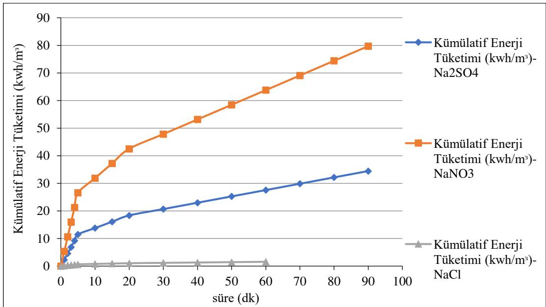
Şekil 6.194. %40IrO 2 -%60RuO 2 kaplı paralel plaka titanyum elektrotlarla, başlangıç kirlilik derişimi 125 mg/L olduđu durumda Na 2 SO 4 , NaNO 3 ve NaCl elektrolitleri ile optimum kořullarda oluřan, enerji tüketim grafiđi
