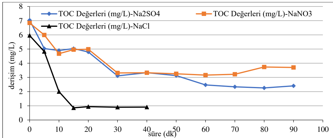
Şekil 6.165. Ti/RuO 2 kaplı paralel plaka elektrotlarla, başlangıç kirlilik derişimi 30 mg/L, 150 A/m 2 akım yoğunluğu, 155,84 mL/dk hızı, 0,01 M Na 2 SO 4 elektrolit derişimi, pH 11 : 11 'de; 150 A/m 2 akım yoğunluğu, 155,84 mL/dk akış hızı, 0,01 M NaNO 3 elektrolit derişimi, pH 0 'da; 50 A/m 2 akım yoğunluğu, 155,84 mL/dk akış hızı, 0,06 M NaCl elektrolit derişimi, pH 0 olan koşullarda elde edilen TOC sonuçları
