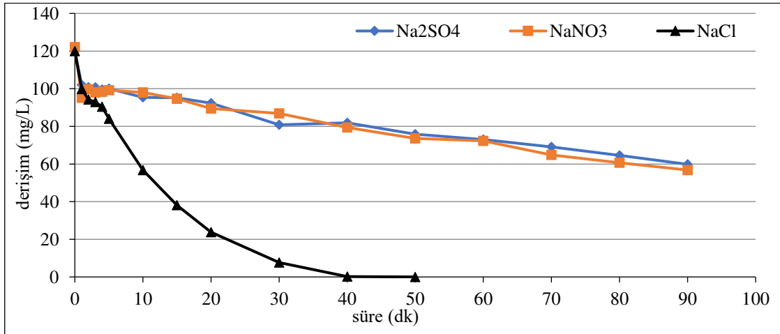
Şekil 6.53. \text{Ti/RuO}_2 kaplı paralel plaka elektrotlarla, C_0 :125 mg/L \text{Na}_2\text{SO}_4 için; 150 A/m 2 akım yoğunluğu, 155,84 mL/dk akış hızı, 0,01 M \text{Na}_2\text{SO}_4 elektrolit miktarı, \text{pH}_{11} olan koşullarda; \text{NaNO}_3 için; 150 A/m 2 akım yoğunluğu, 155,84 mL/dk akış hızı, 0,01 M \text{NaNO}_3 elektrolit miktarı, \text{pH}_0 (6,46) olan koşullarda, \text{NaCl} için; 50 A/m 2 akım yoğunluğu, 155,84 mL/dk akış hızı, 0,06 M \text{NaCl} elektrolit miktarı, \text{pH}_0 (6,03) olan koşullarda elde edilen arıtım verimleri
