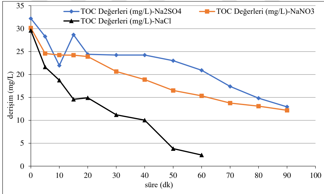
Şekil 6.174. %40IrO 2 -%60RuO 2 kaplı paralel plaka titanyum elektrotlarla, başlangıç kirlilik derişimi 125 mg/L, 300 A/m 2 akım yoğunluğu, 155,84 mL/dk akış hızı, 0,01 M Na 2 SO 4 elektrolit derişimi, pH 11 : 11'de; 500 A/m 2 akım yoğunluğu, 155,84 mL/dk akış hızı, 0,01 M NaNO 3 elektrolit derişimi, pH 0 'da; 75 A/m 2 akım yoğunluğu, 155,84 mL/dk akış hızı, 0,05 M NaCl elektrolit derişimi, pH 0 olan koşullarda elde edilen TOC sonuçları
