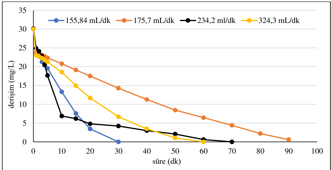
Şekil 6.15. Grafit plaka elektrotlarla, Co:30 mg/L, 40 A/m 2 akım yoğunluğu, 0,08 M NaCl, 155,84 mL/dk, 175,7 mL/dk, 234,2 mL/dk, 324,3 mL/dk akış hızlarında pH 0 : 6,11-6,83 arasında olan koşullarda arıtım verimleri
