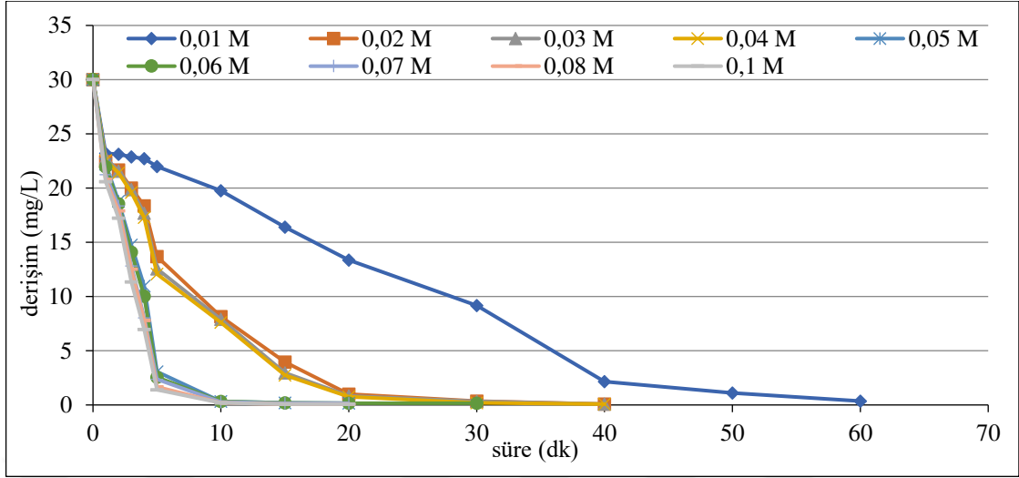
Şekil 6.116. %40IrO 2 -%60RuO 2 kaplı paralel plaka titanyum elektrotlarla, C o :30 mg/L, 75 A/m 2 akım yoğunluğunda, 155,84 mL/dk akış hızında, 0,01/0,02/0,03/0,04/0,05/0,06M/0,07M/0,08M/0,1 M NaCl derişimlerinde, pH 0 : 6,05-6,25 aralığında olan koşullarda elde edilen arıtım verimleri
