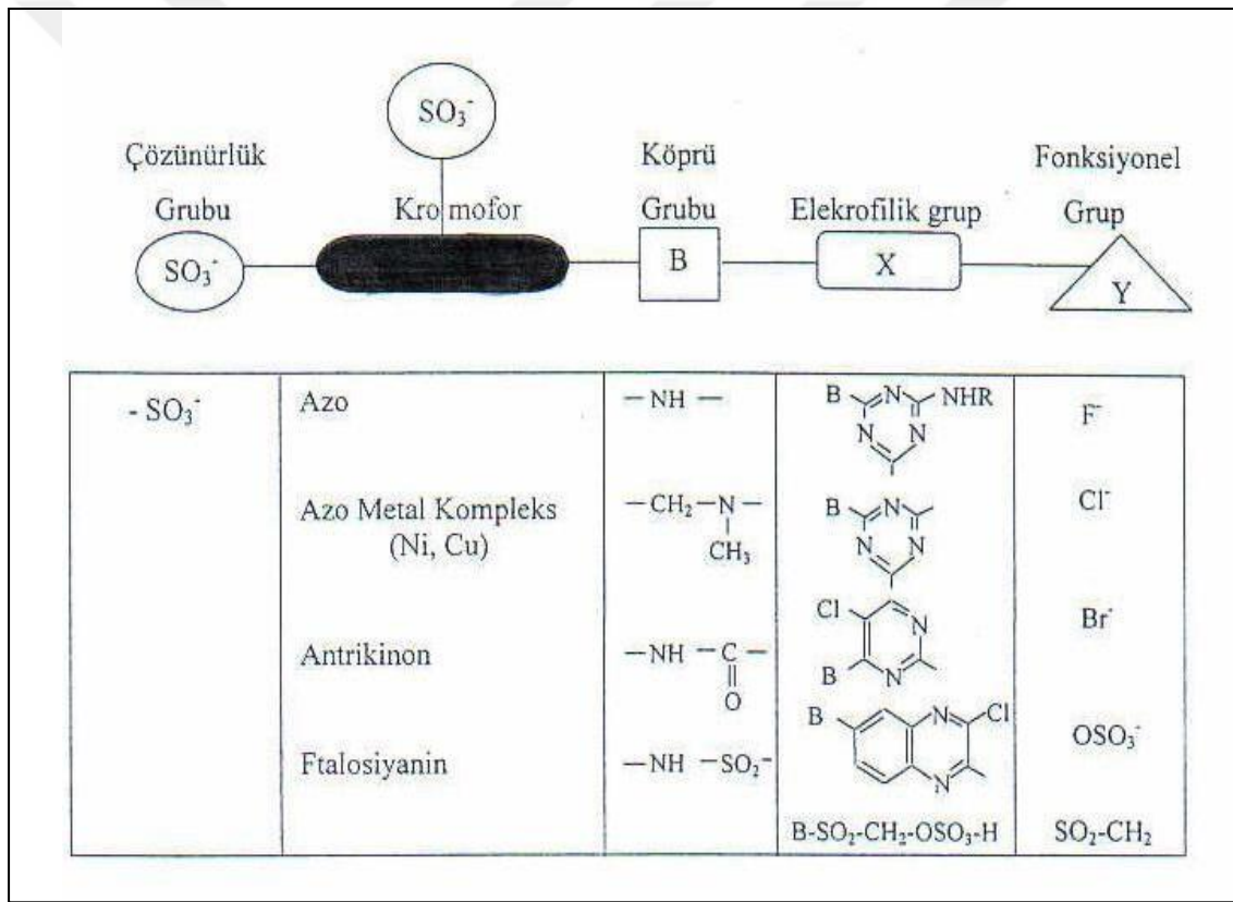
Şekil 3.2. Reaktif Boyarmaddelerin Genel Yapısı (Vigo, 1994)
