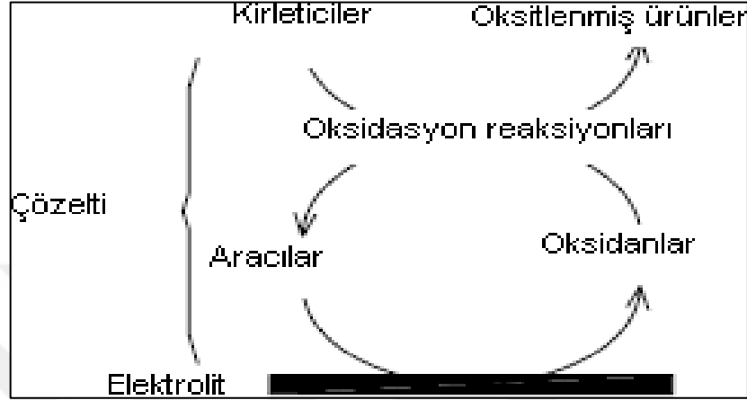
Görsel 3.5. Dolaylı oksidasyon sırasında oluşan tepkimeler (Deng ve Englehardt, 2007)
