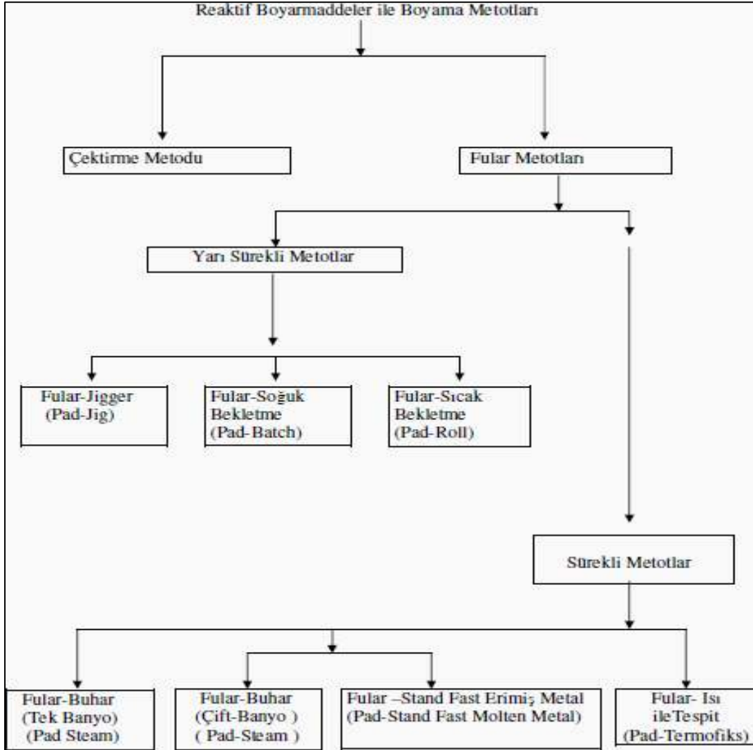
Şekil 3.3. Reaktif boyar maddeler ile boyama metotları (Vardar, 2006)
