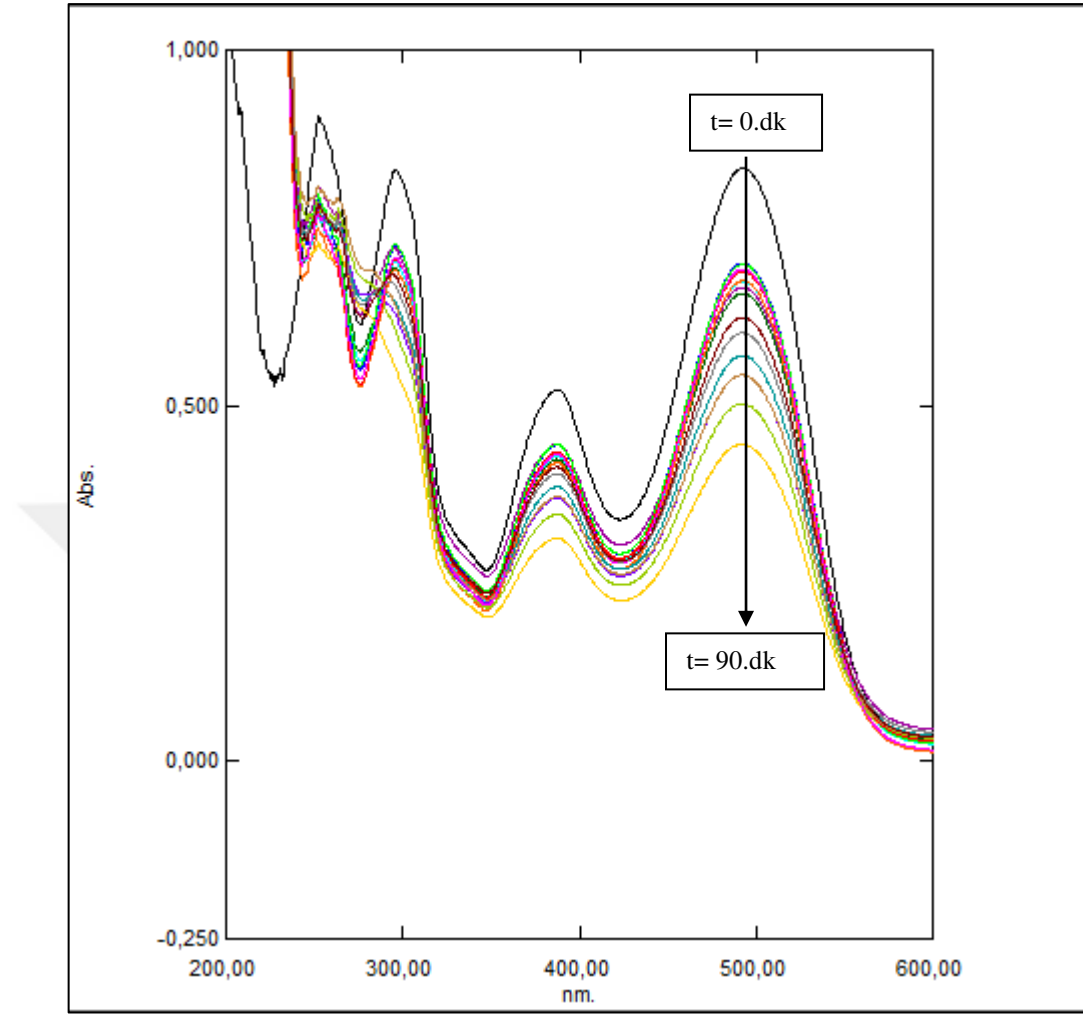
Şekil 6.129. Ti/IrO 2 kaplı paralel plaka elektrotlarla, 125 mg/L başlangıç kirlilik derişimi için; 50 A/m 2 akım yoğunluğunda, 155,84 mL/dk akış hızında, 0,01 M NaNO 3 elektrolit miktarı ve pH 0 'de UV-Spektrum grafiğı
