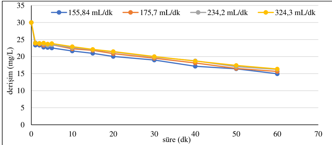
Şekil 6.56. %80IrO 2 -%20RuO 2 kaplı paralel plaka titanyum elektrotlarla, C_o :30 mg/L, 200 A/m 2 akım yoğunluğu, 155,84 mL/dk, 175,7 mL/dk, 234,2 mL/dk, 324,3 mL/dk akış hızlarında, 0,02 M \text{Na}_2\text{SO}_4 , pH 0 : 6,04-6,20 aralığında olan koşullarda elde edilen arıtım verimleri
