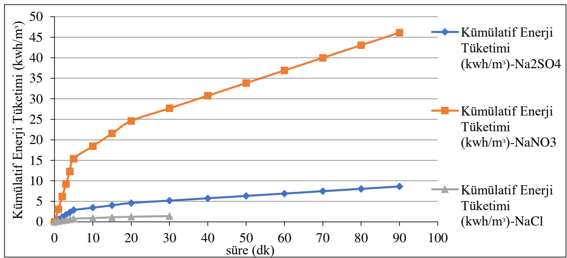
Şekil 6.187. %80IrO 2 -%20RuO 2 kaplı paralel plaka titanyum elektrotlarla, başlangıç kirlilik derişimi 30 mg/L olduğu durumda Na 2 SO 4 , NaNO 3 ve NaCl elektrolitleri ile optimum koşullarda oluşan enerji tüketim grafiği
