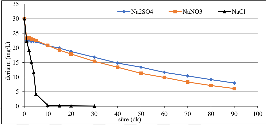
Şekil 6.103. %60 \text{IrO}_2 -%40 \text{RuO}_2 kaplı paralel plaka titanyum elektrotlarla, C_0 :30 mg/L \text{Na}_2\text{SO}_4 için; 400 \text{A/m}^2 akım yoğunluğu, 155,84 mL/dk akış hızı, 0,01 M \text{Na}_2\text{SO}_4 elektrolit miktarı, \text{pH}_{11} olan koşullarda; \text{NaNO}_3 için; 500 \text{A/m}^2 akım yoğunluğu, 155,84 mL/dk akış hızı, 0,01 M \text{NaNO}_3 elektrolit miktarı, \text{pH}_0 (6,16) olan koşullarda, \text{NaCl} için; 75 \text{A/m}^2 akım yoğunluğu, 155,84 mL/dk akış hızı, 0,05 M \text{NaCl} elektrolit miktarı, \text{pH}_0 (6,26) olan koşullarda elde edilen arıtım verimleri
