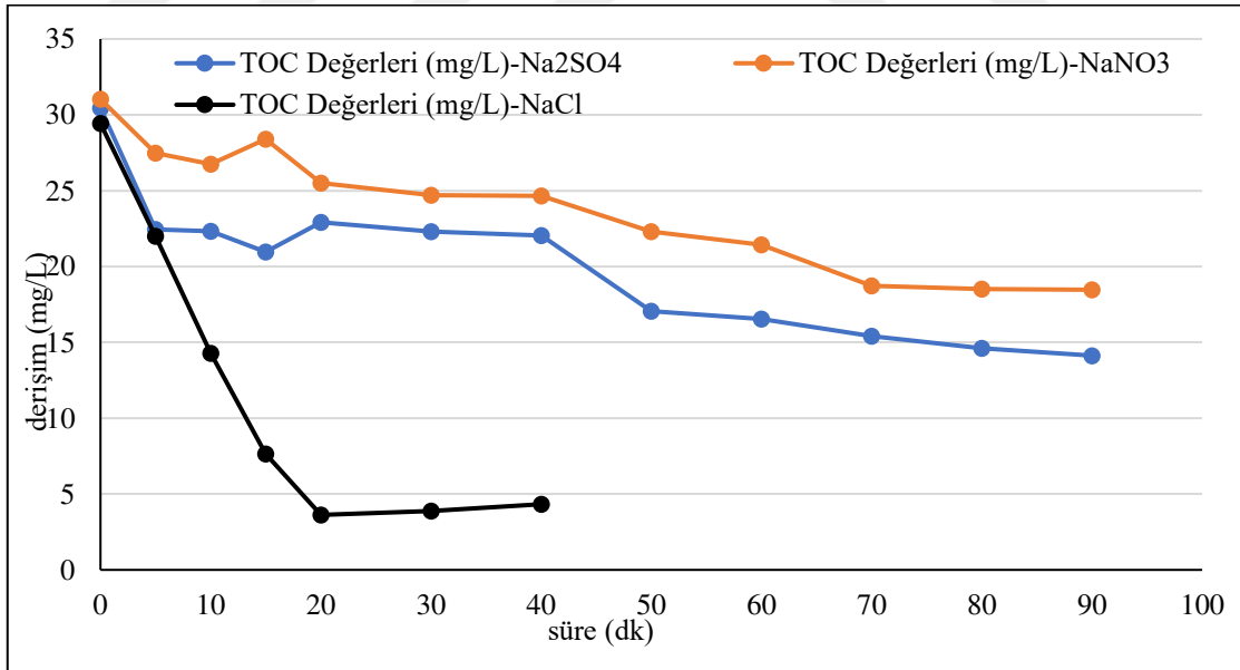
Şekil 6.164. Ti/IrO 2 kaplı paralel plaka elektrotlarla, başlangıç kirlilik derişimi 125 mg/L, 50 A/m 2 akım yoğunluğu, 155,84 mL/dk hızı, 0,01 M Na 2 SO 4 elektrolit derişimi, pH 11 : 11 'de; 50 A/m 2 akım yoğunluğu, 155,84 mL/dk akış hızı, 0,01 M NaNO 3 elektrolit derişimi, pH 0 'da; 50 A/m 2 akım yoğunluğu, 155,84 mL/dk akış hızı, 0,05 M NaCl elektrolit derişimi, pH 0 olan koşullarda elde edilen TOC sonuçları
