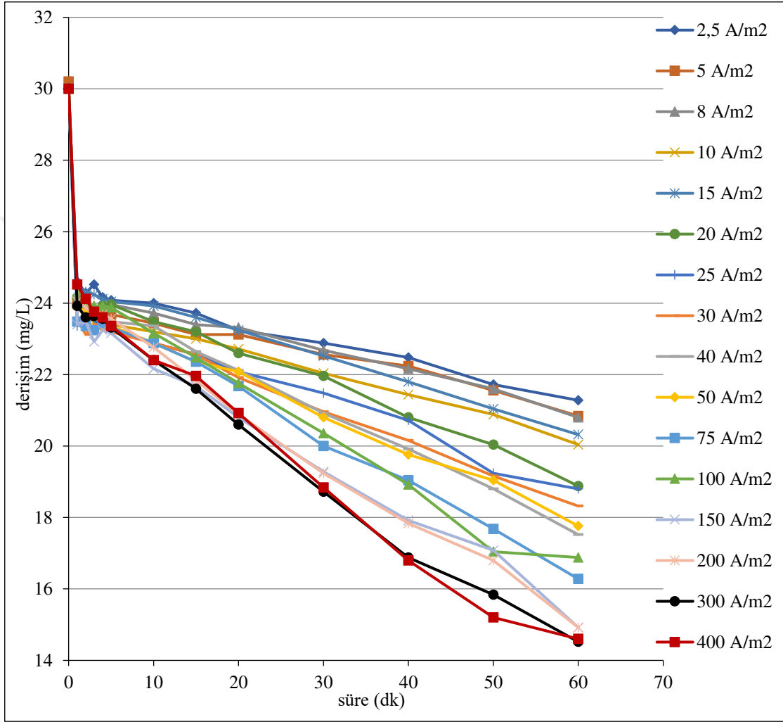
Şekil 6.42. Ti/RuO 2 kaplı paralel plaka elektrotlarla, C 0 :30 mg/L, 2,5/5/8/10/15/20/25/30/40/50/75/100/150/200/300/400 A/m 2 akım yoğunluklarında, 155,84 mL/dk akış hızında, 0,01 M NaNO 3 , pH 0 : 6,51-7,02 olan koşullarda elde edilen arıtım verimleri
