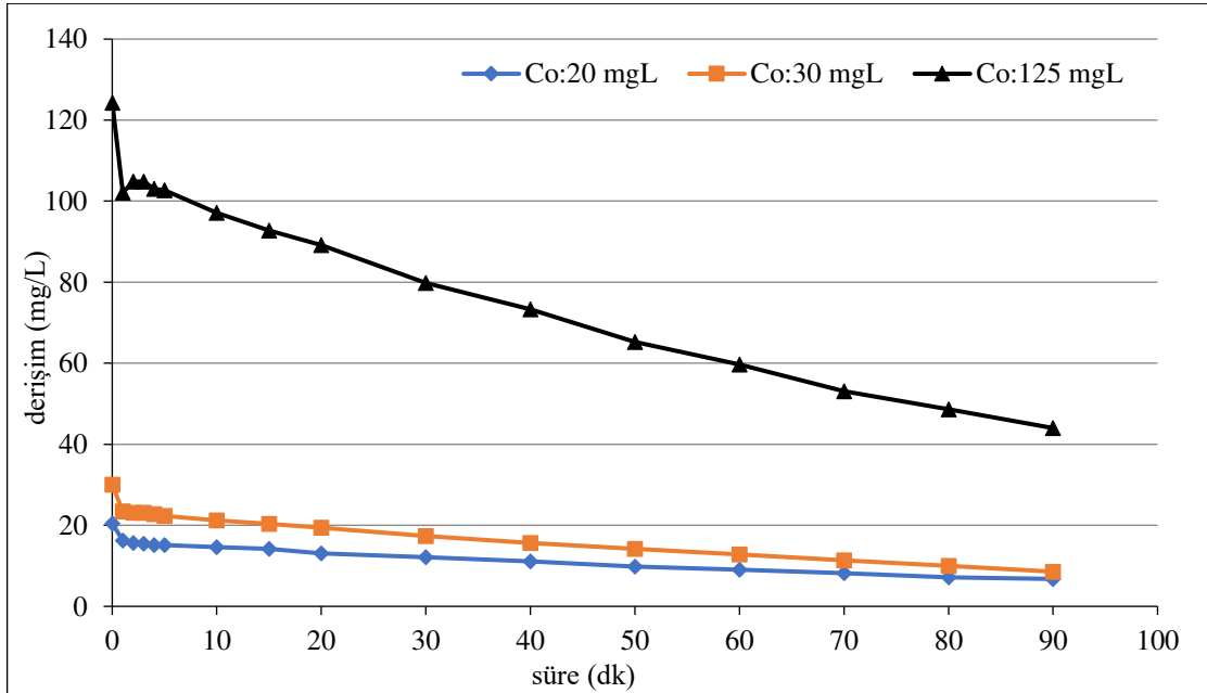
Şekil 6.63. %80IrO 2 -%20RuO 2 kaplı paralel plaka titanyum elektrotlarla, 400 A/m 2 akım yoğunluğunda, 155,84 mL/dk akış hızında, başlangıç kirlilik derişimleri 20 mg/L, 30 mg/L ve 125 mg/L olan 0,01 M \text{NaNO}_3 elektrolit derişiminde, pH 0 (6,24-6,33) olan koşullarda elde edilen arıtım verimleri
