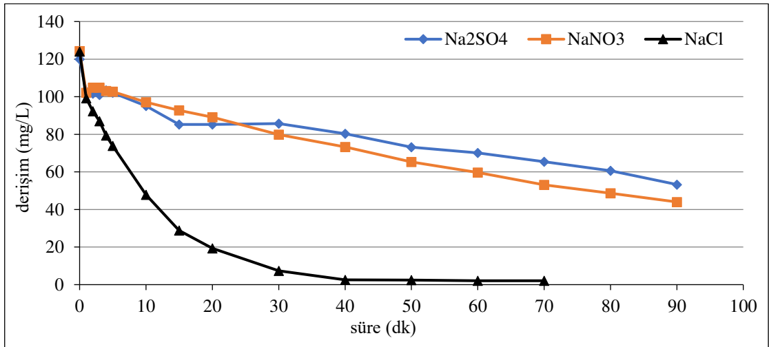
Şekil 6.70. %80 \text{IrO}_2 -%20 \text{RuO}_2 kaplı paralel plaka titanyum elektrotlarla, C_0 :125 mg/L \text{Na}_2\text{SO}_4 için; 200 \text{A/m}^2 akım yoğunluğu, 155,84 mL/dk akış hızı, 0,02 M \text{Na}_2\text{SO}_4 elektrolit miktarı, \text{pH}_{11} olan koşullarda; \text{NaNO}_3 için; 400 \text{A/m}^2 akım yoğunluğu, 155,84 mL/dk akış hızı, 0,01 M \text{NaNO}_3 elektrolit miktarı, \text{pH}_0 (6,33) olan koşullarda, \text{NaCl} için; 75 \text{A/m}^2 akım yoğunluğu, 155,84 mL/dk akış hızı, 0,05 M \text{NaCl} elektrolit miktarı, \text{pH}_0 (6,78) olan koşullarda elde edilen arıtım verimleri
