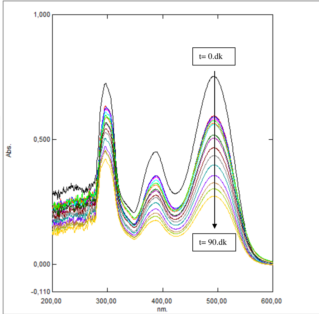
Şekil 6.134. Ti/RuO 2 kaplı paralel plaka elektrotlarla, 30 mg/L başlangıç kirlilik derişimi için; 150 A/m 2 akım yoğunluğunda, 155,4 mL/dk akış hızında, 0,01 M NaNO 3 elektrolit miktarı ve pH 0 'de UV-Spektrum grafiğı
