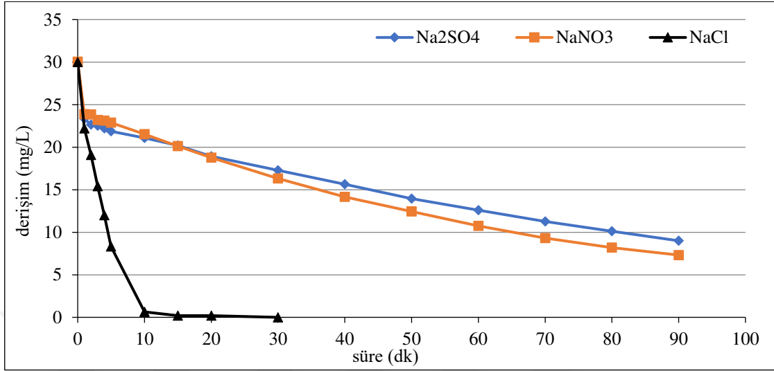
Şekil 6.86. %20 \text{IrO}_2 -%80 \text{RuO}_2 kaplı paralel plaka titanyum elektrotlarla, C_0 :30 mg/L \text{Na}_2\text{SO}_4 için; 200 \text{A/m}^2 akım yoğunluğu, 155,84 mL/dk akış hızı, 0,01 M \text{Na}_2\text{SO}_4 elektrolit miktarı, \text{pH}_{11} olan koşullarda; \text{NaNO}_3 için; 400 \text{A/m}^2 akım yoğunluğu, 155,84 mL/dk akış hızı, 0,01 M \text{NaNO}_3 elektrolit miktarı, \text{pH}_0 (6,20) olan koşullarda, \text{NaCl} için; 75 \text{A/m}^2 akım yoğunluğu, 155,84 mL/dk akış hızı, 0,04 M \text{NaCl} elektrolit miktarı, \text{pH}_0 (6,27) olan koşullarda elde edilen arıtım verimleri
