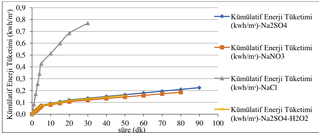
Şekil 6.182. Grafit plaka elektrotlarla, başlangıç kirlilik derişimi 30 mg/L olduğu durumda Na 2 SO 4 , Na 2 SO 4 -H 2 O 2 , NaNO 3 ve NaCl elektrolitleri ile optimum koşullarda oluşan enerji tüketim grafiği
