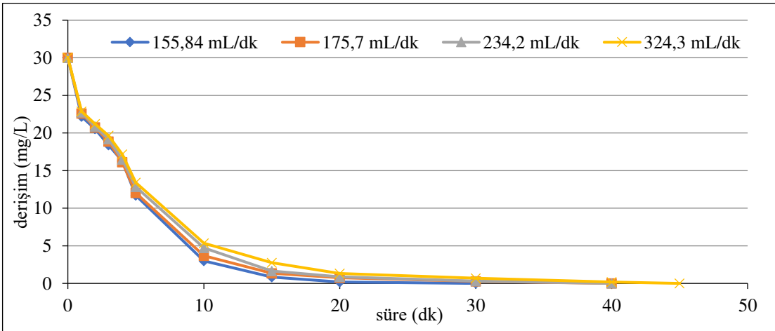
Şekil 6.83. %20IrO 2 -%80RuO 2 kaplı paralel plaka titanyum elektrotlarla, C_o :30 mg/L, 75 A/m 2 akım yoğunluğu, 155,84 mL/dk, 175,7 mL/dk, 234,2 mL/dk, 324,3 mL/dk akış hızlarında, 0,04 M NaCl, pH 0 : 6,23-6,27 aralığında olan koşullarda elde edilen arıtım verimleri
