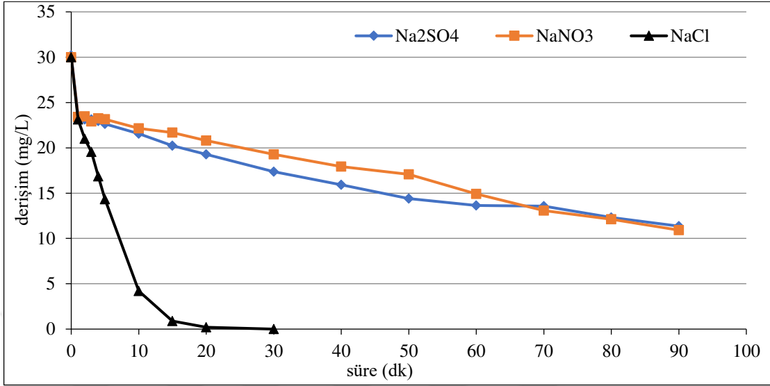
Şekil 6.52. \text{Ti/RuO}_2 kaplı paralel plaka elektrotlarla, C_0 :30 mg/L \text{Na}_2\text{SO}_4 için; 150 A/m 2 akım yoğunluğu, 155,84 mL/dk akış hızı, 0,01 M \text{Na}_2\text{SO}_4 elektrolit miktarı, \text{pH}_{11} olan koşullarda; \text{NaNO}_3 için; 150 A/m 2 akım yoğunluğu, 155,84 mL/dk akış hızı, 0,01 M \text{NaNO}_3 elektrolit miktarı, \text{pH}_0 (6,66) olan koşullarda, \text{NaCl} için; 50 A/m 2 akım yoğunluğu, 155,84 mL/dk akış hızı, 0,06 M \text{NaCl} elektrolit miktarı, \text{pH}_0 (6,12) olan koşullarda elde edilen arıtım verimleri
