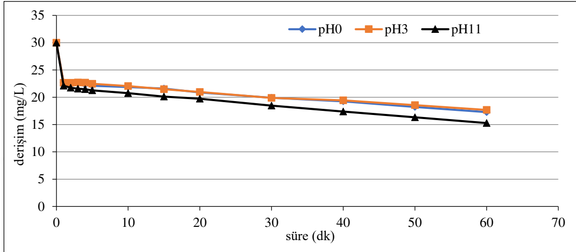
Şekil 6.28. \text{Ti/IrO}_2 kaplı paralel plaka elektrotlarla, C_0 :30 mg/L, 50 \text{ A/m}^2 akım yoğunluğunda, 155,84 mL/dk akış hızında, 0,01 M \text{NaNO}_3 derişiminde, \text{pH}_0 (5,94), \text{pH}_3 ve \text{pH}_{11} 'de olan koşullarda elde edilen arıtım verimleri
