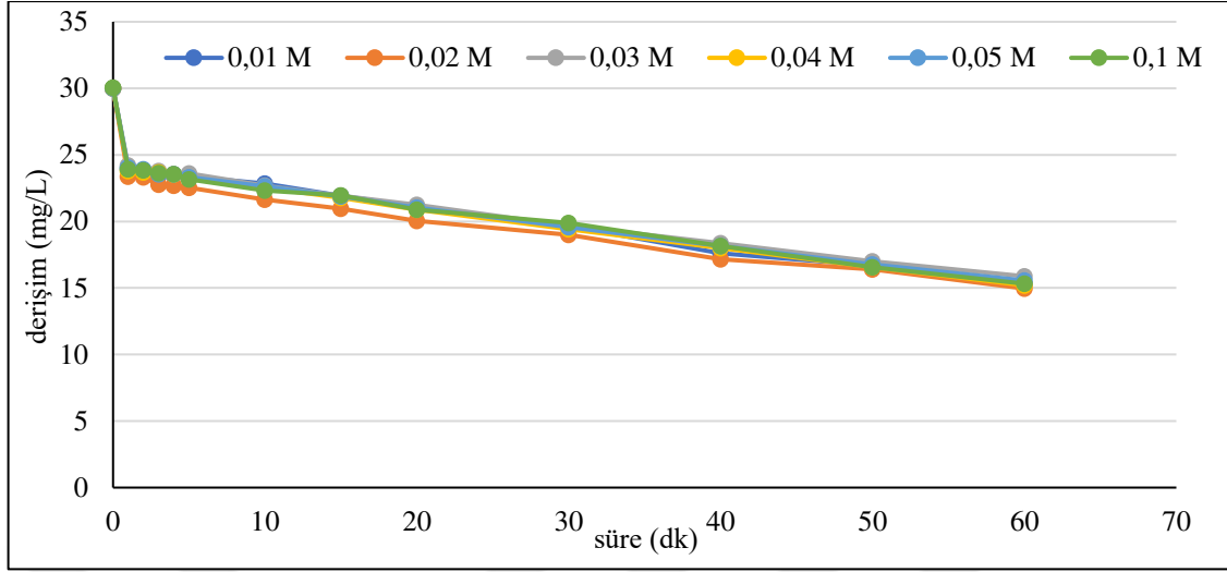
Şekil 6.55. %80IrO 2 -%20RuO 2 kaplı paralel plaka titanyum elektrotlarla, C_o :30 mg/L, 200 A/m 2 akım yoğunluğunda, 155,84 mL/dk akış hızında, 0,01/0,02/0,03/0,04/0,05/0,1 M \text{Na}_2\text{SO}_4 derişimlerinde, pH 0 : 6,01-6,22 aralığında olan koşullarda elde edilen arıtım verimleri
