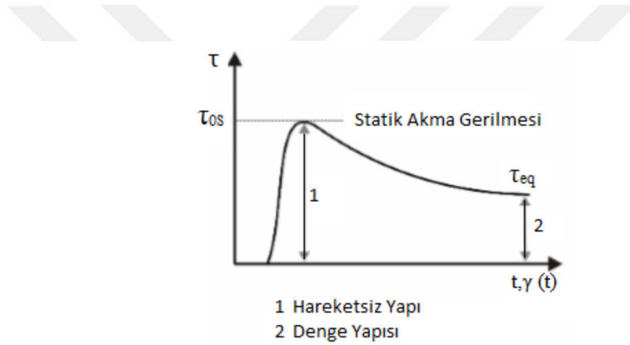
Şekil 1.3: Kayma gerilmesi \tau çok düşük bir sabit kayma hızında ve statik akma gerilmesi \tau_{0s} .
