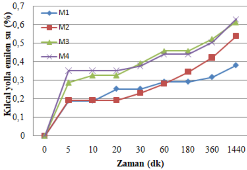
Şekil 4.3: 90 günlük kılcallık atış yüzdesi-zaman grafiği.
