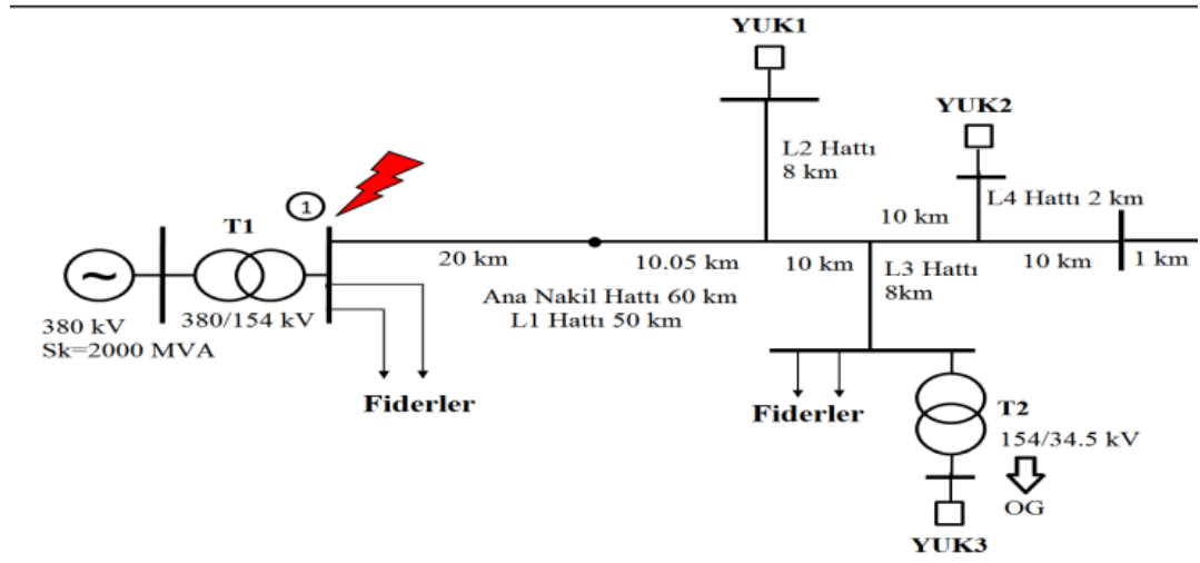
Şekil 1.2. İletim hatları tek hat şeması örneği (Enerji İletim ve Dağıtım, n.d.)
